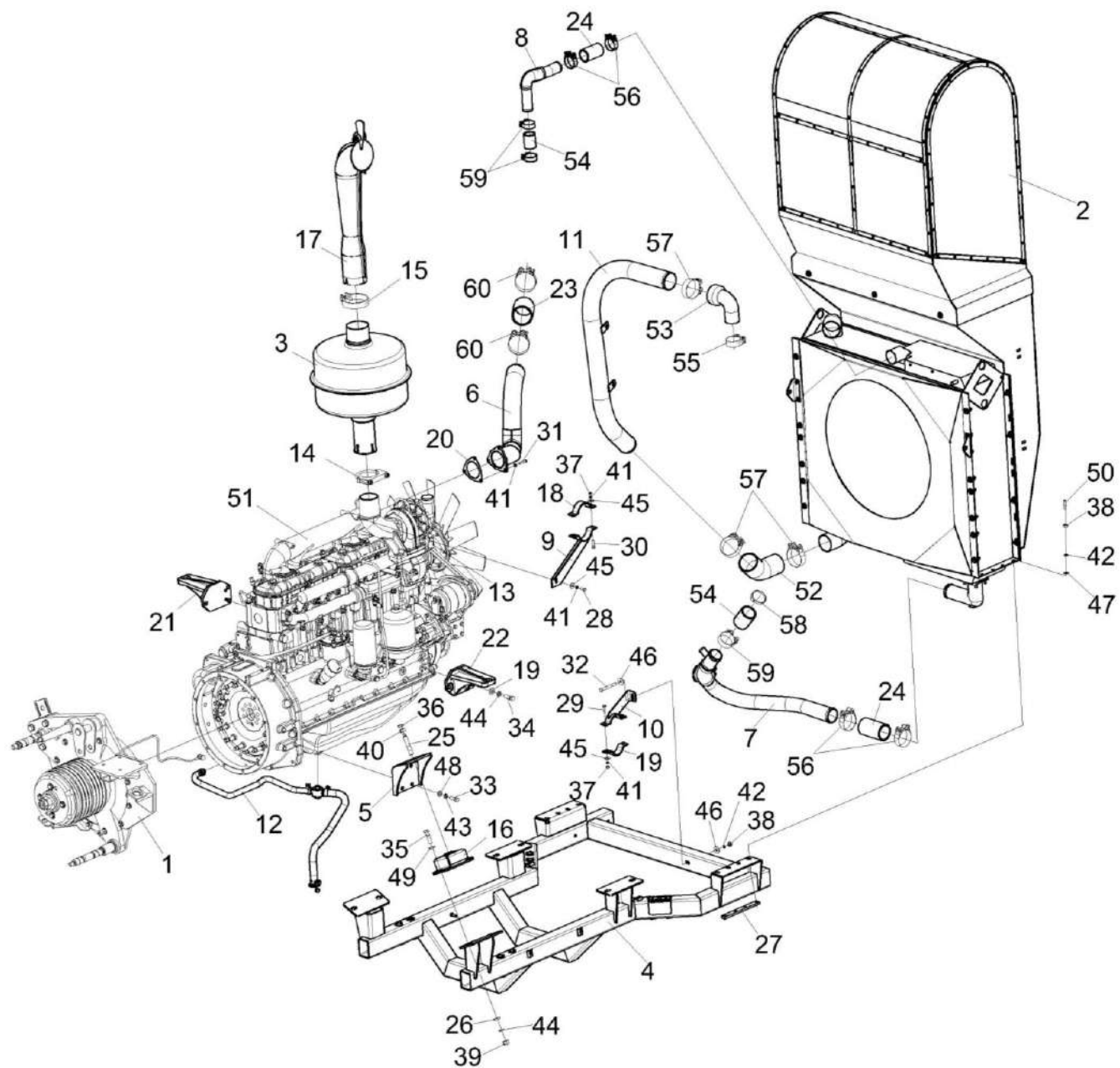
Рисунок 85 – Установка радиатора КП-4-0106040
