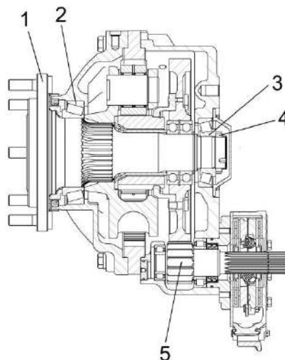
Рисунок 2.22 – Редуктор бортовой (разрез)
