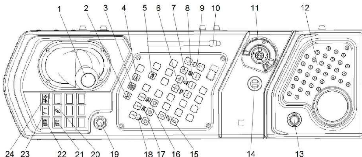
Рисунок 1.34 – Пульт управления комбайна
