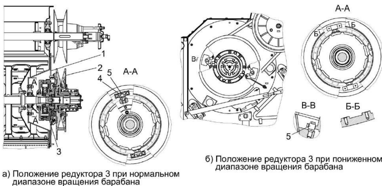
Рисунок 2.12 – Разблокировка понижающего редуктора
