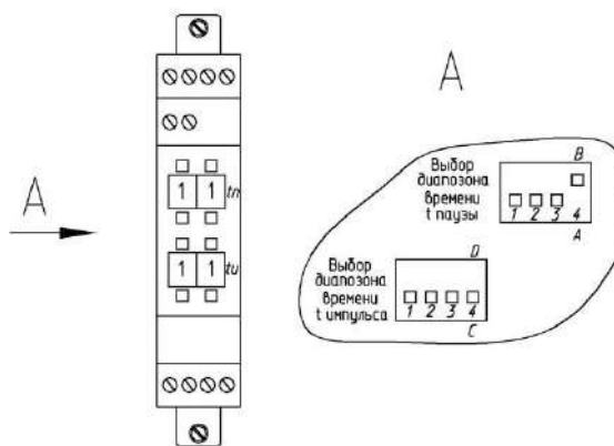
Рисунок 1.32 – Реле времени
