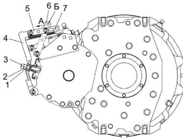
Рисунок 2.21 – Редуктор бортовой
