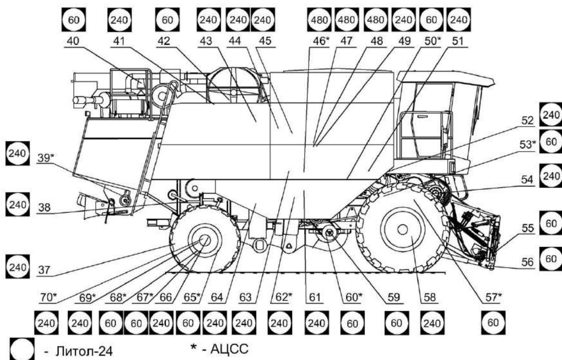
Рисунок 3.2 – Смазка комбайна (вид справа)
