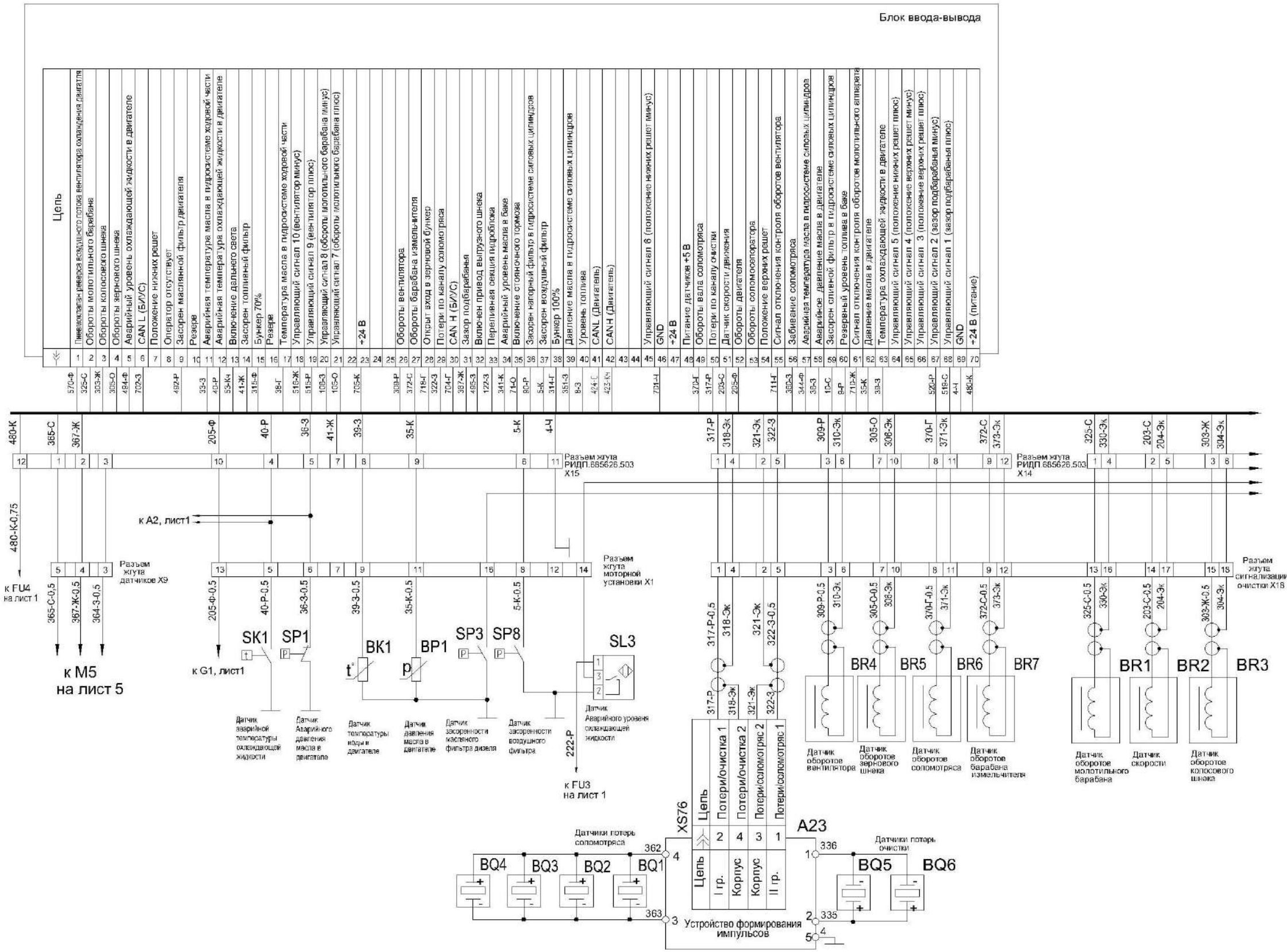
Рисунок Б.6 – Схема электрическая принципиальная комбайна (лист 6.1)
