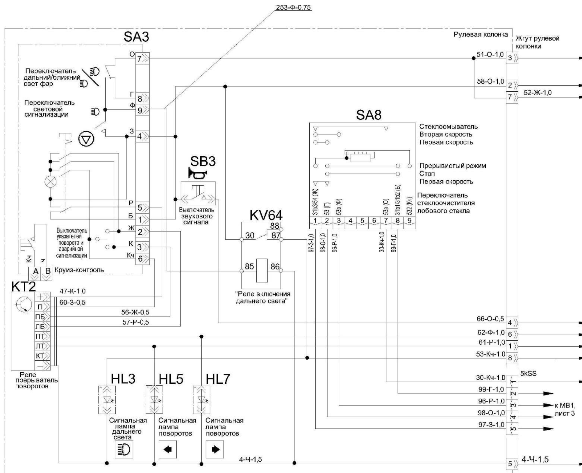
Рисунок Б.2 – Схема электрическая принципиальная комбайна (лист 2.1)
