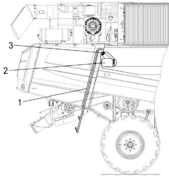
Рисунок 2.7 – Заправка топливного бака
