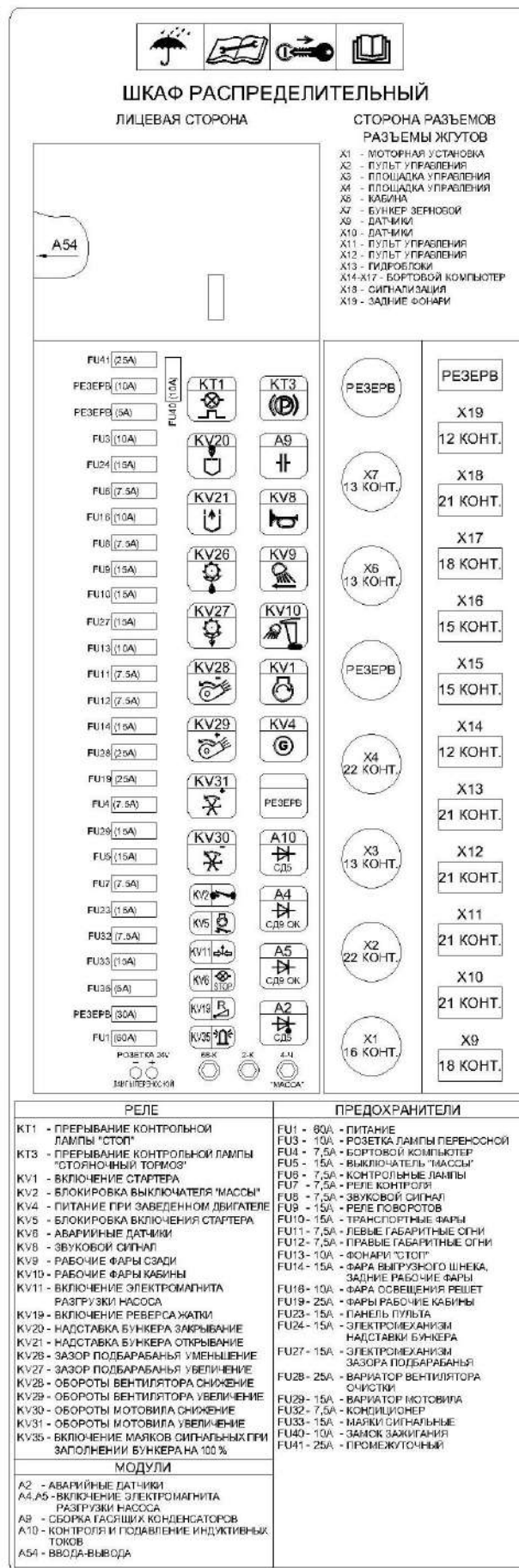
Рисунок 1.24 – Схема соединений шкафа распределительного
