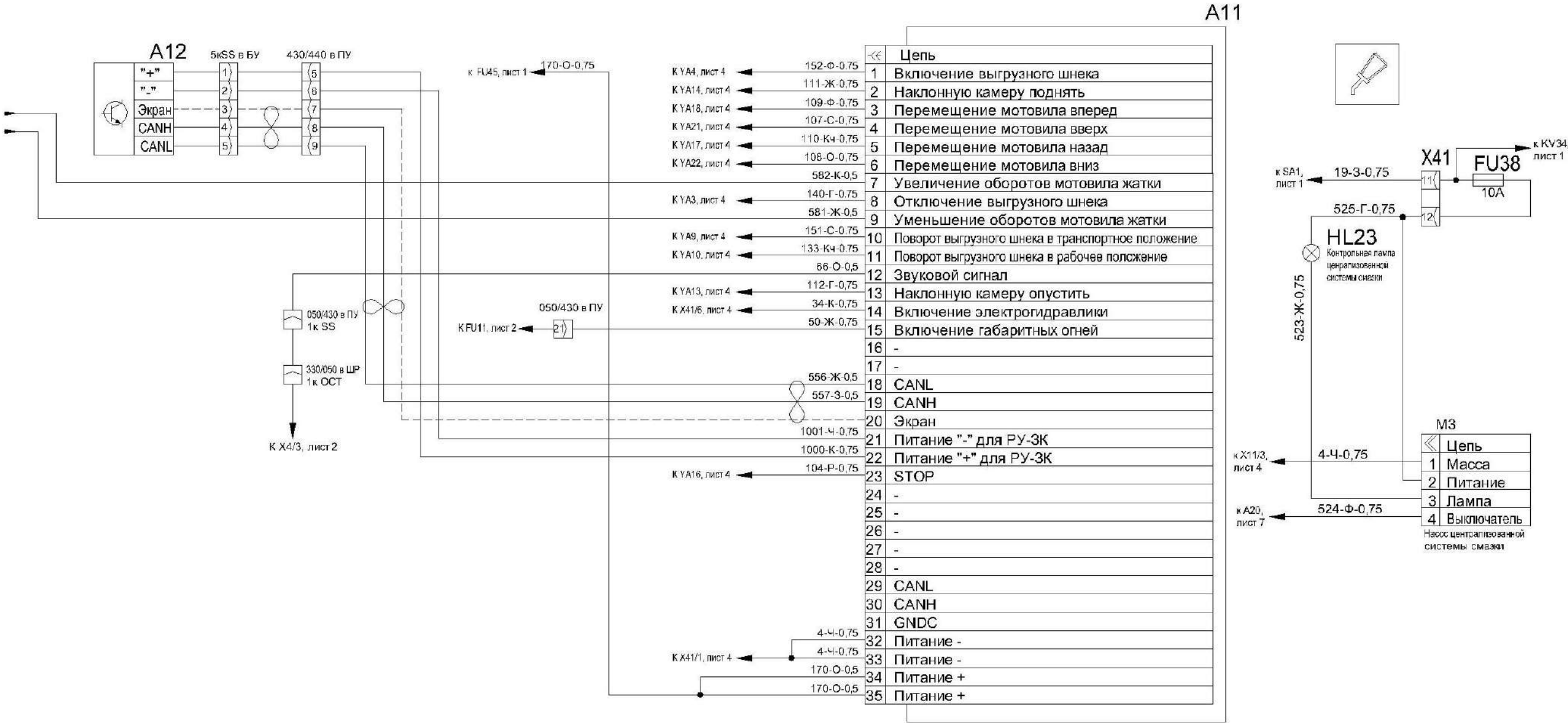
Рисунок Б.5 – Схема электрическая принципиальная комбайна (лист 5.2)
