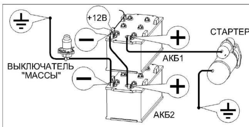
Рисунок 2.5 – Подключение аккумуляторных батарей
