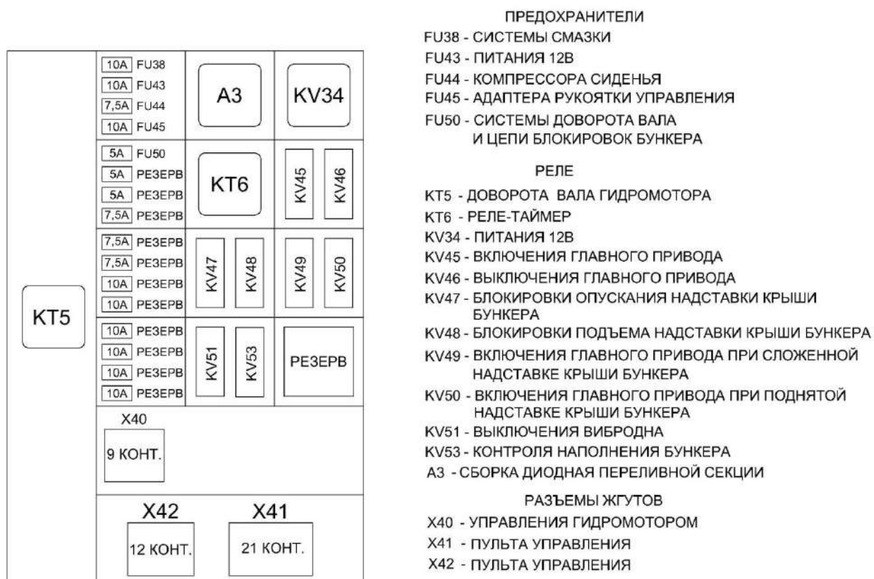
Рисунок 1.35 – Реле и предохранители пульта управления
