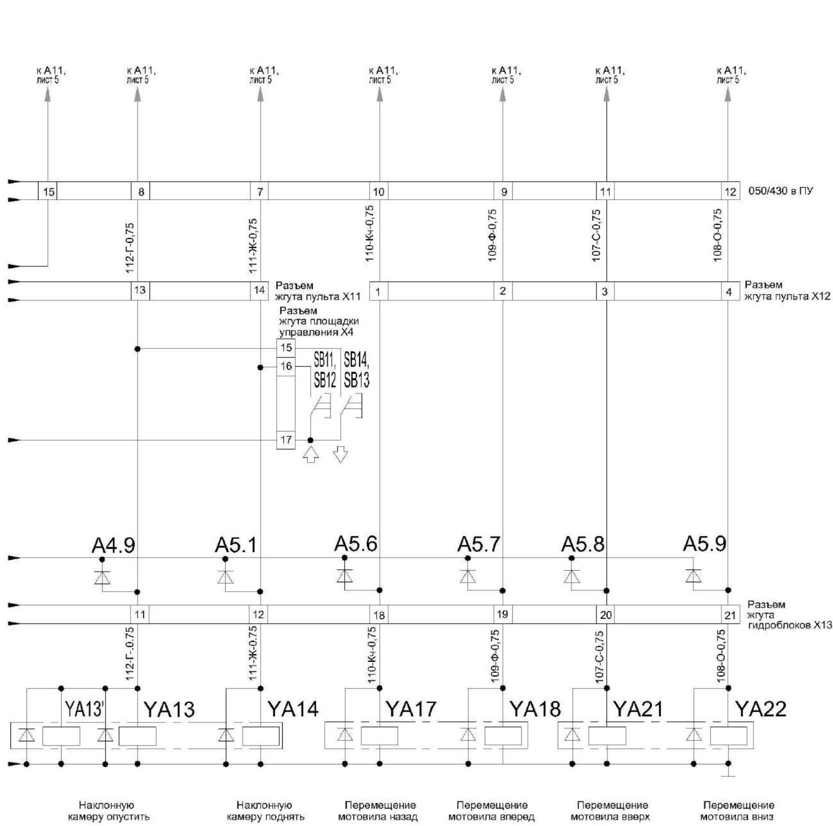
Рисунок Б.4 – Схема электрическая принципиальная комбайна (лист 4.3)
