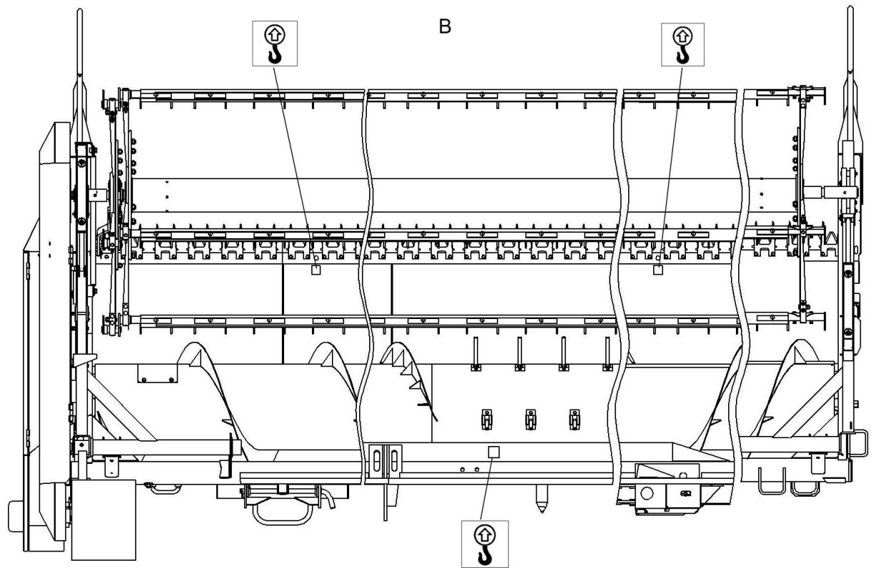
Расположение на жатке предупредительных и указательных знаков и табличек безопасности (вид справа)
