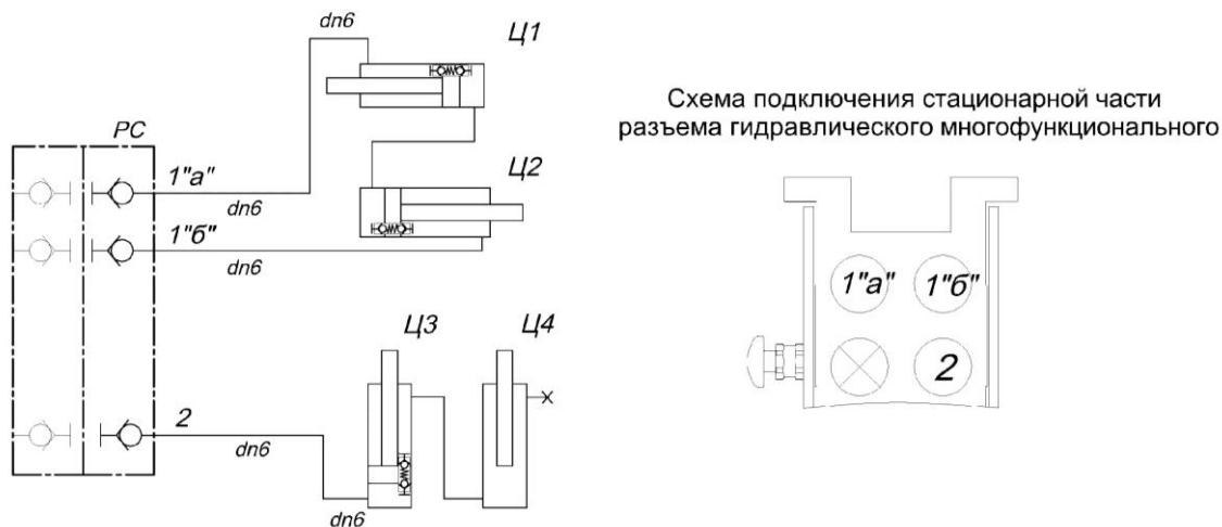
а) с многофункциональным разъемом
