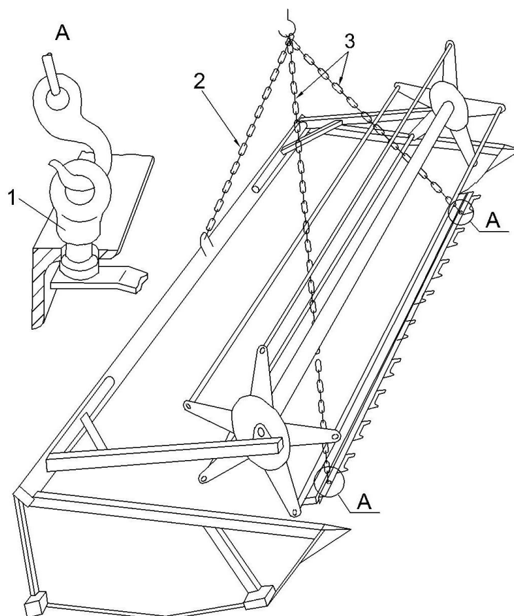
1 – рым болт; 2, 3 – стропы
