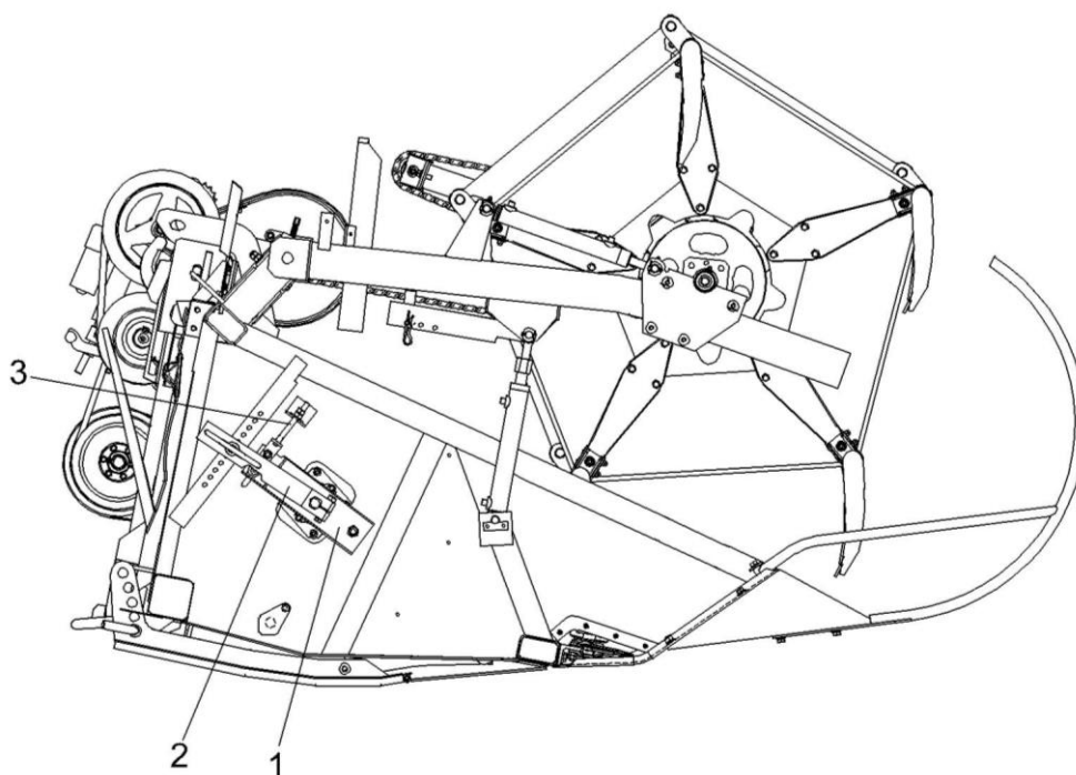
1 – опора шнека; 2 – рычаг; 3 – тяга
