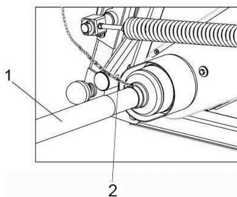
Рисунок 2.8– Подсоединение энергосистем жатки
