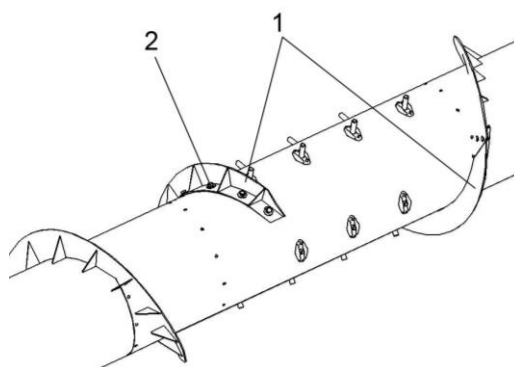
1 - витки; 2 – крепеж
