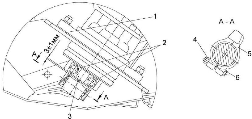
Рисунок 3.6 – Угловая передача
