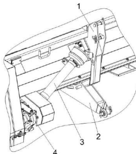
Рисунок 2.3 – Навеска жатки для трав
