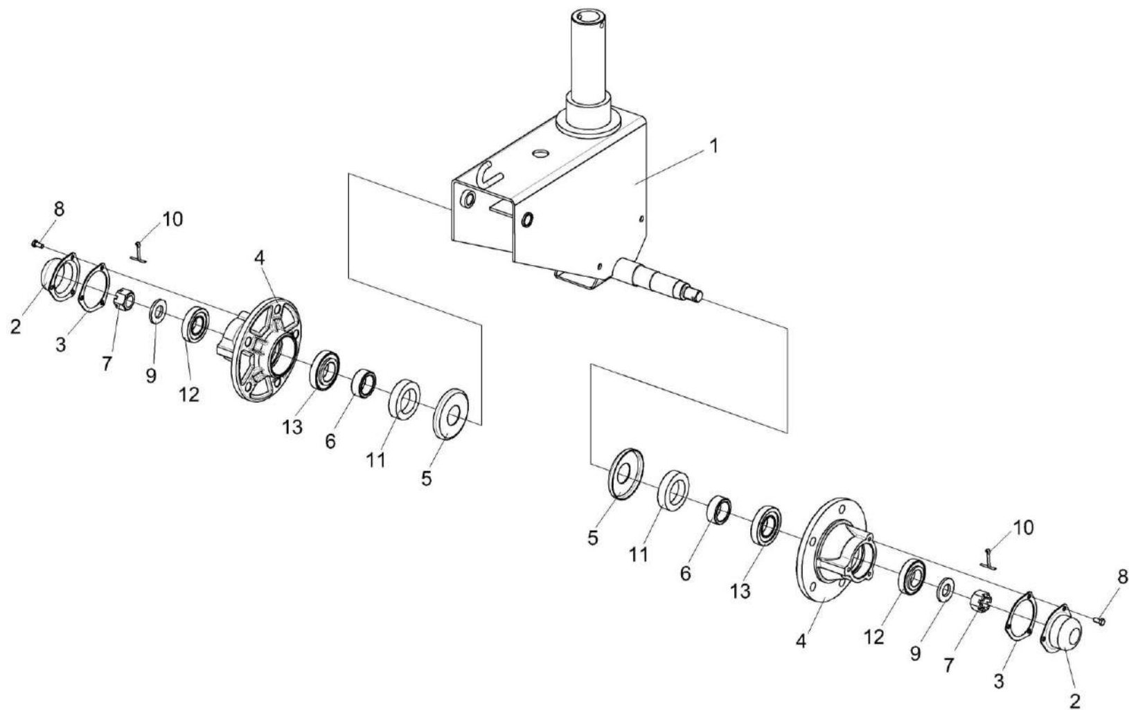
Рисунок 35 – Ось передняя КЗР 1593000
