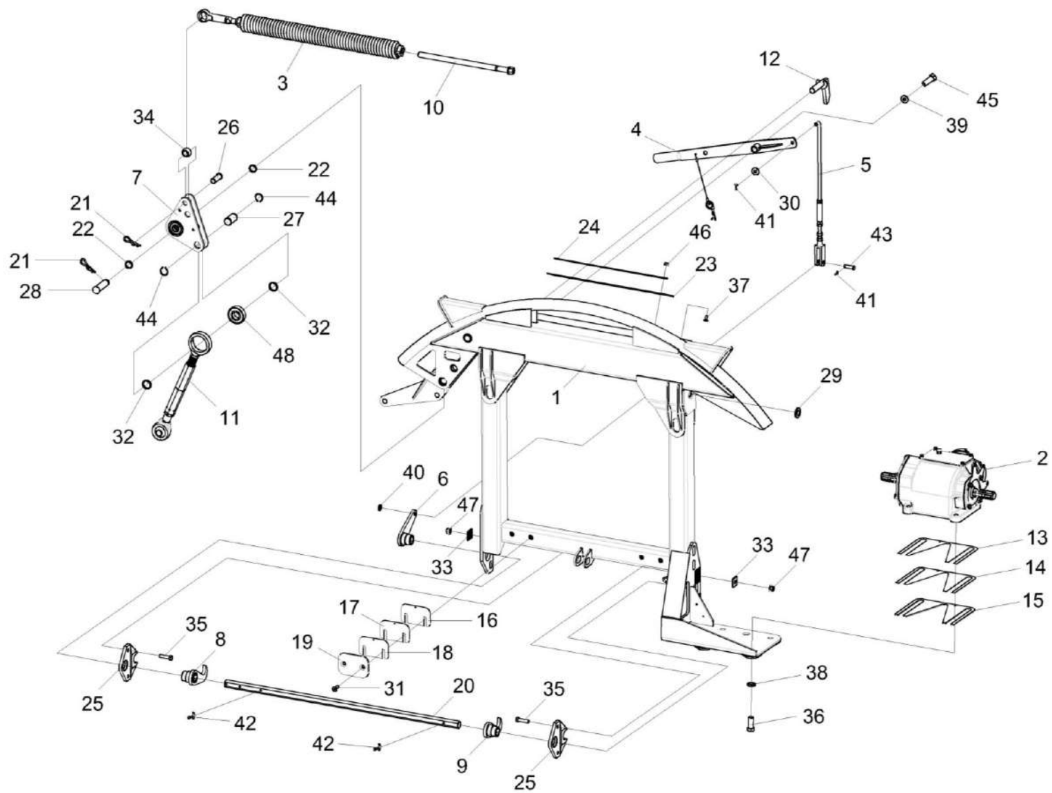
Рисунок 26 – Рамка переходная ЖРТ-6-0120000А
