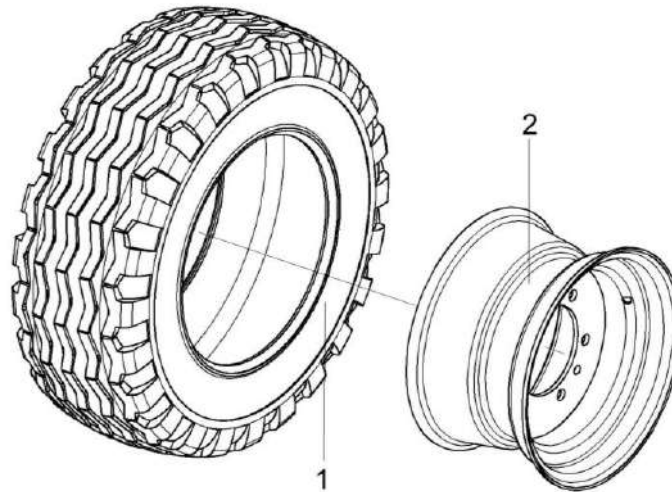
Рисунок 37 – Колесо КЛ 0109500
