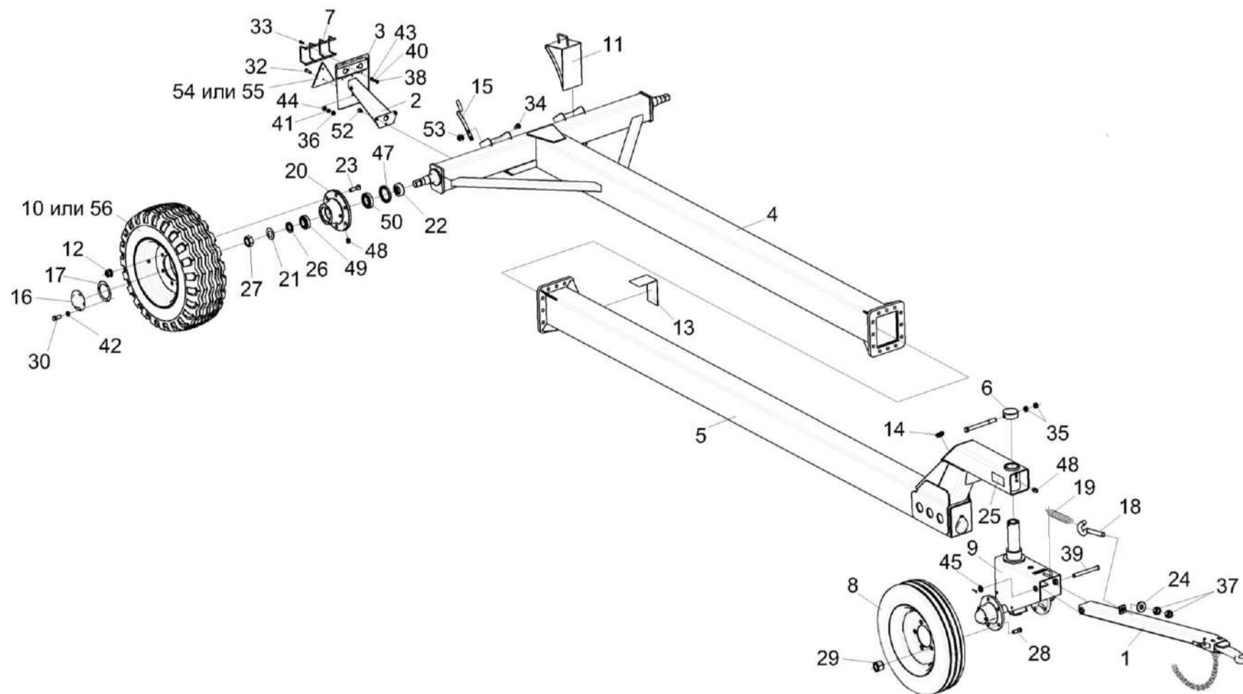
Рисунок 34 – Тележка транспортная (установка колес)
