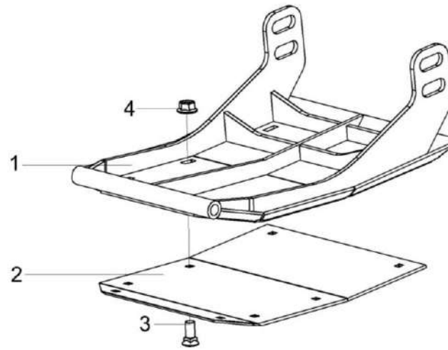
Рисунок 25 – Башмак КВК-1-0518000А-01
