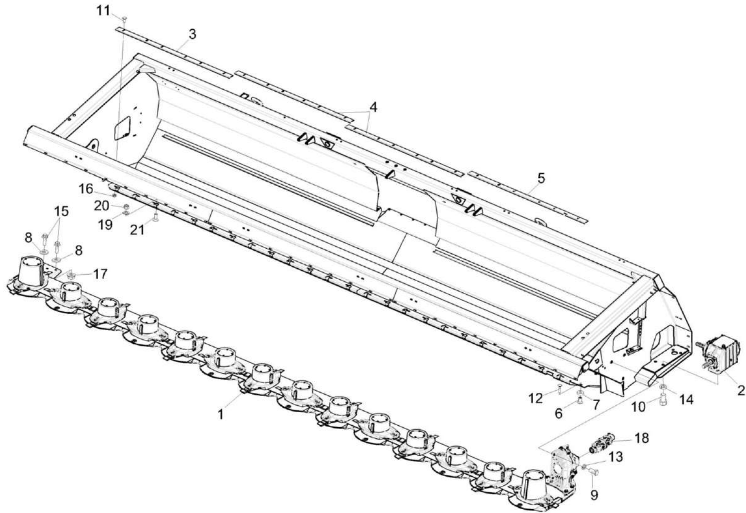
Рисунок 5 – Жатка для трав ЖРТ-6-0100000 (лист 4)
