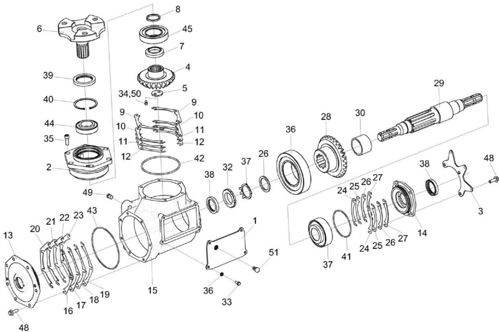
Рисунок 27 – Редуктор ЖРТ-6-0125000
