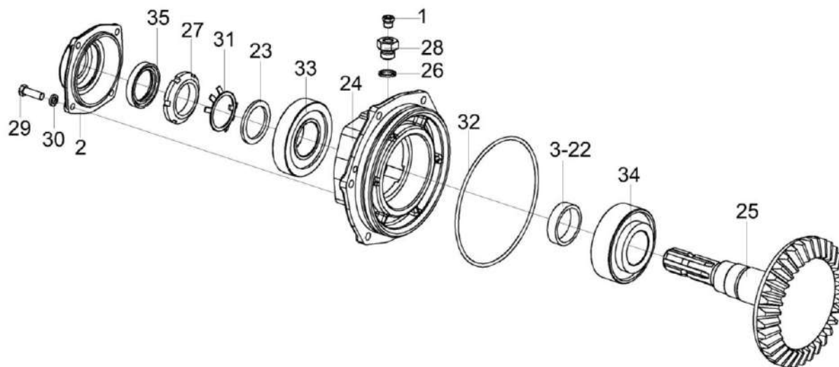
Рисунок 22 – Стакан КВК-1-0506010
