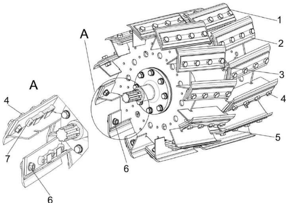
1 - прижим ножа; 2, 3 - ножи; 4 – болт; 5 – опора; 6 – гайка; 7 - планка
