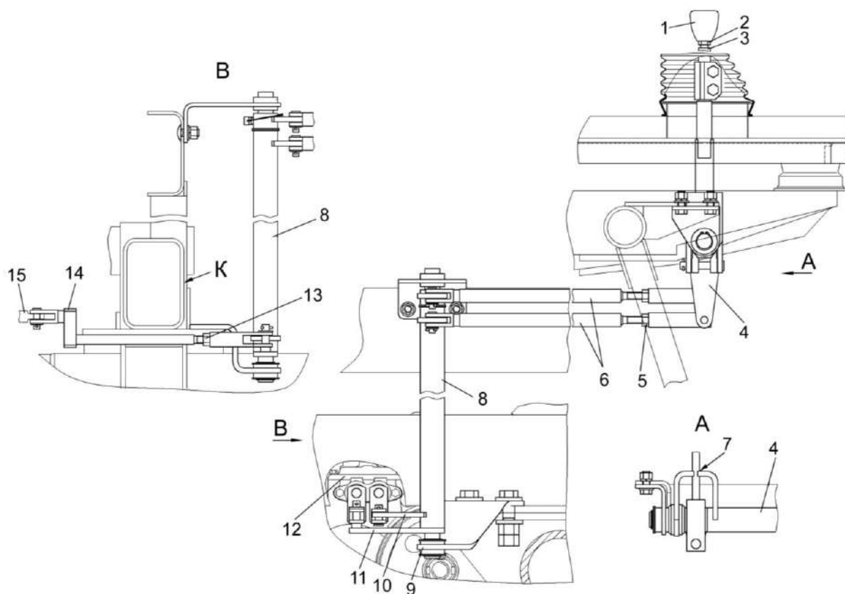
1 – рукоятка механизма переключения передач; 2 – гайка; 3 – рычаг рукоятки механизма переключения передач; 4 – блок переключения; 5, 13 – контргайки; 6, 14 – тяги; 7 – пазы кулис блока переключения; 8 – вал; 9 – опора; 10, 11 – рычаги; 12 – коробка перемены передач; 15 – штоки коробки перемены передач
