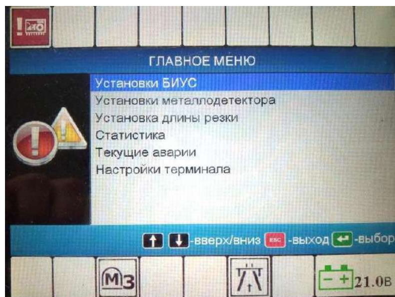
Рисунок Ж.8 – Раздел установок БИУС
