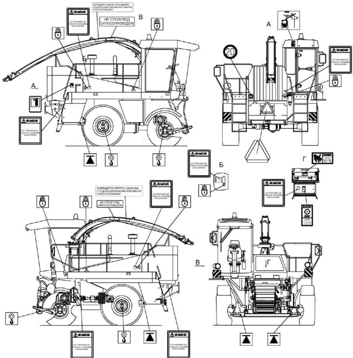
Комбайн
