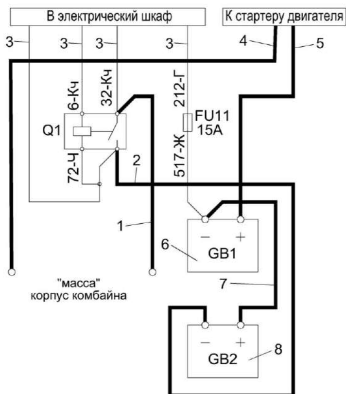
Рисунок 2.2 – Схема установки аккумуляторных батарей
