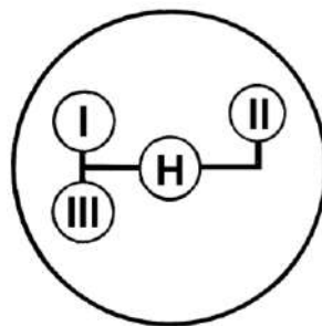
Рисунок 1.26 – Схема переключения передач
