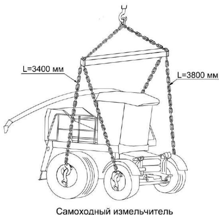
Рисунок 6.1 – Схема строповки комбайна
