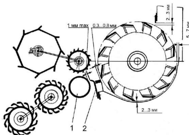
1 – гладкий валец; 2 – чистик
