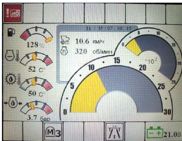
Рисунок Ж.6 – Экран транспортирования
