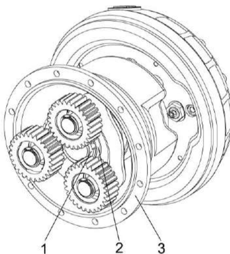
Рисунок 2.28 - Редуктор бортовой
