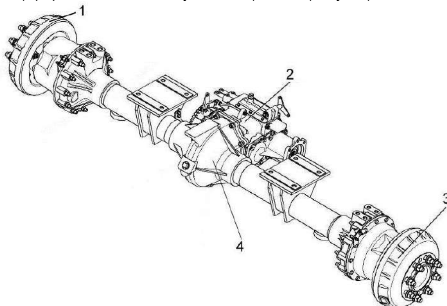
Рисунок 1.13 – Мост ведущих колес
