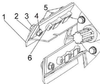
Рисунок 4.3 – Замена ножа
