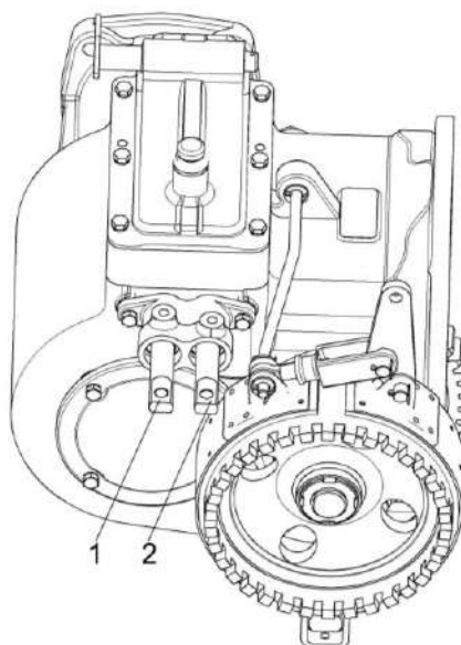
1 - шток переключения 1-й и 3-й передач; 2 - шток переключения 2-й передачи Рисунок 2.30 - Коробка передач
