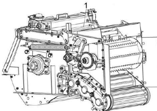
Рисунок 4.2– Питающе-измельчающий аппарат
