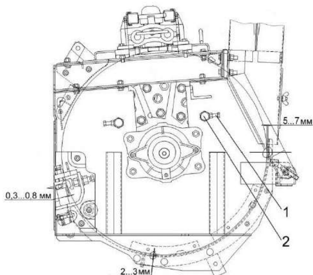
1 – стопорный болт; 2 – бонка
