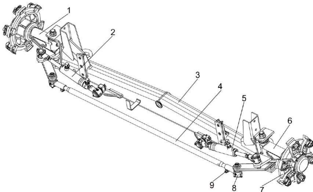
Рисунок 1.12 – Мост управляемых колес
