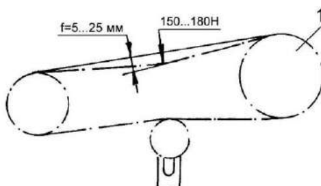
Рисунок 2.23 – Схемы натяжения цепных передач
