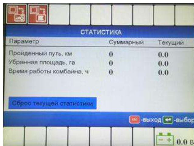
Рисунок Ж.14 – Экран статистики
