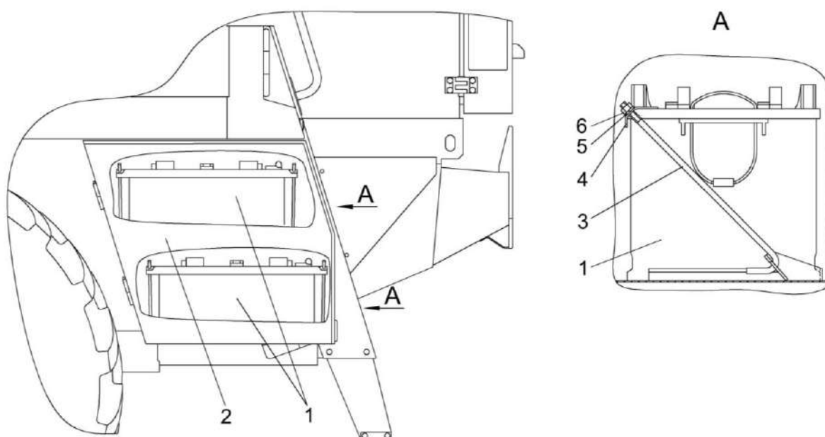
Рисунок 2.2 – Схема установки аккумуляторных батарей
