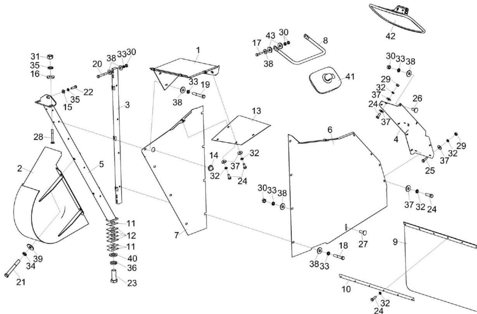
Рисунок 193 – Установка ограждений КВС-80-8-0100100 (лист 2)
