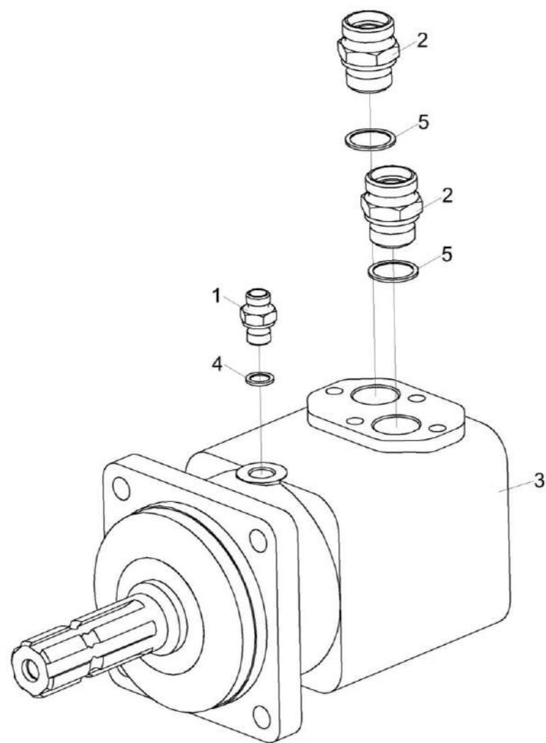
Рисунок 229 – Гидромотор привода режущего аппарата КС-200-0688210
