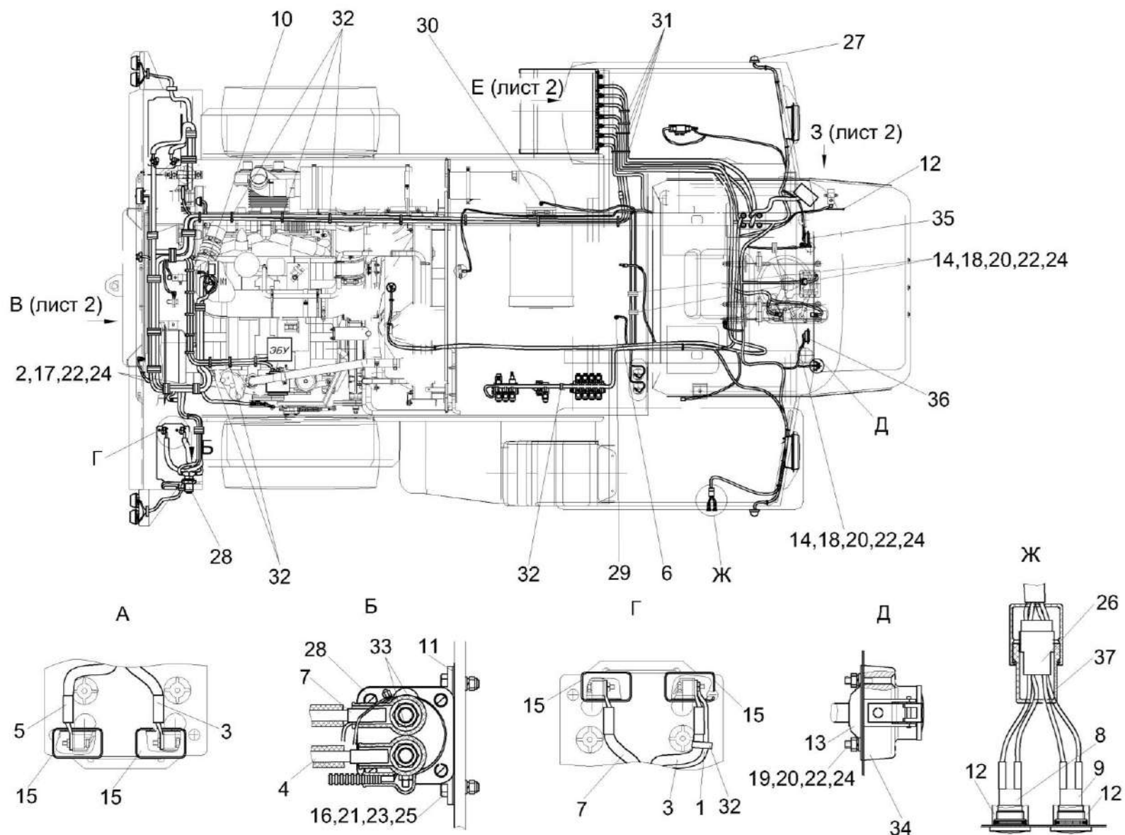
Рисунок 246 – Установка электрооборудования КВС-80-7-0721000 (лист 1)
