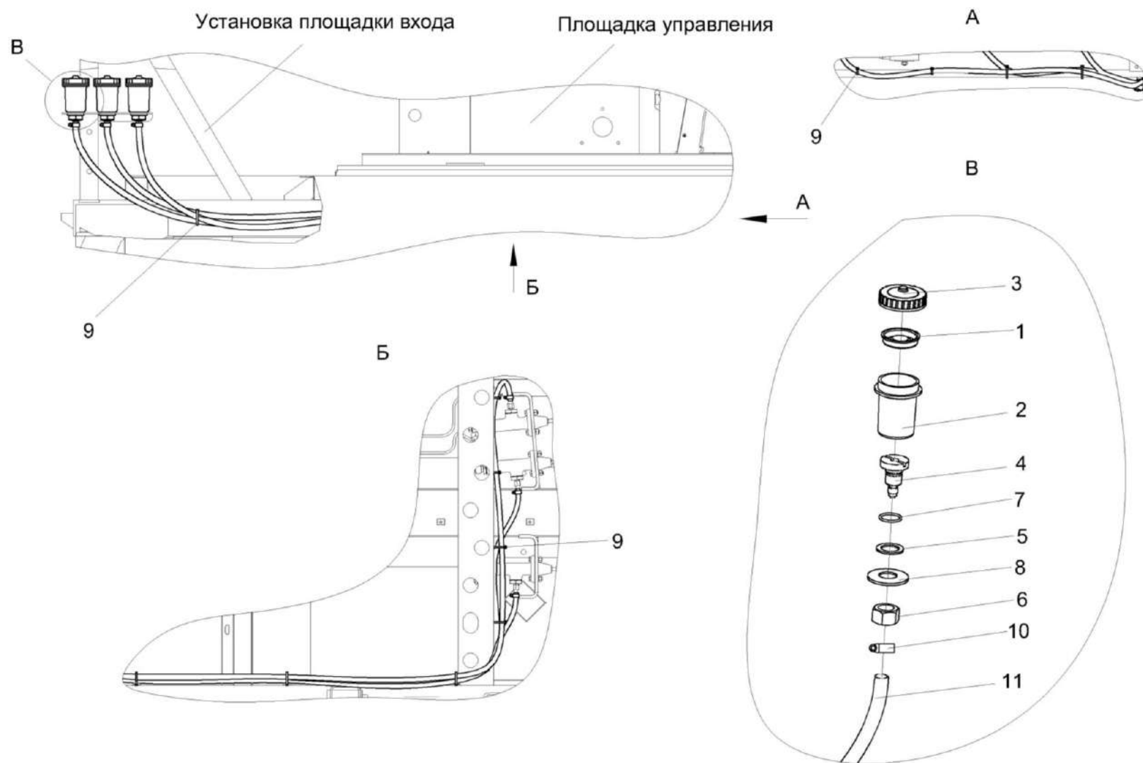
Рисунок 156 – Установка тормозных бачков КВС-80-8-0119660
