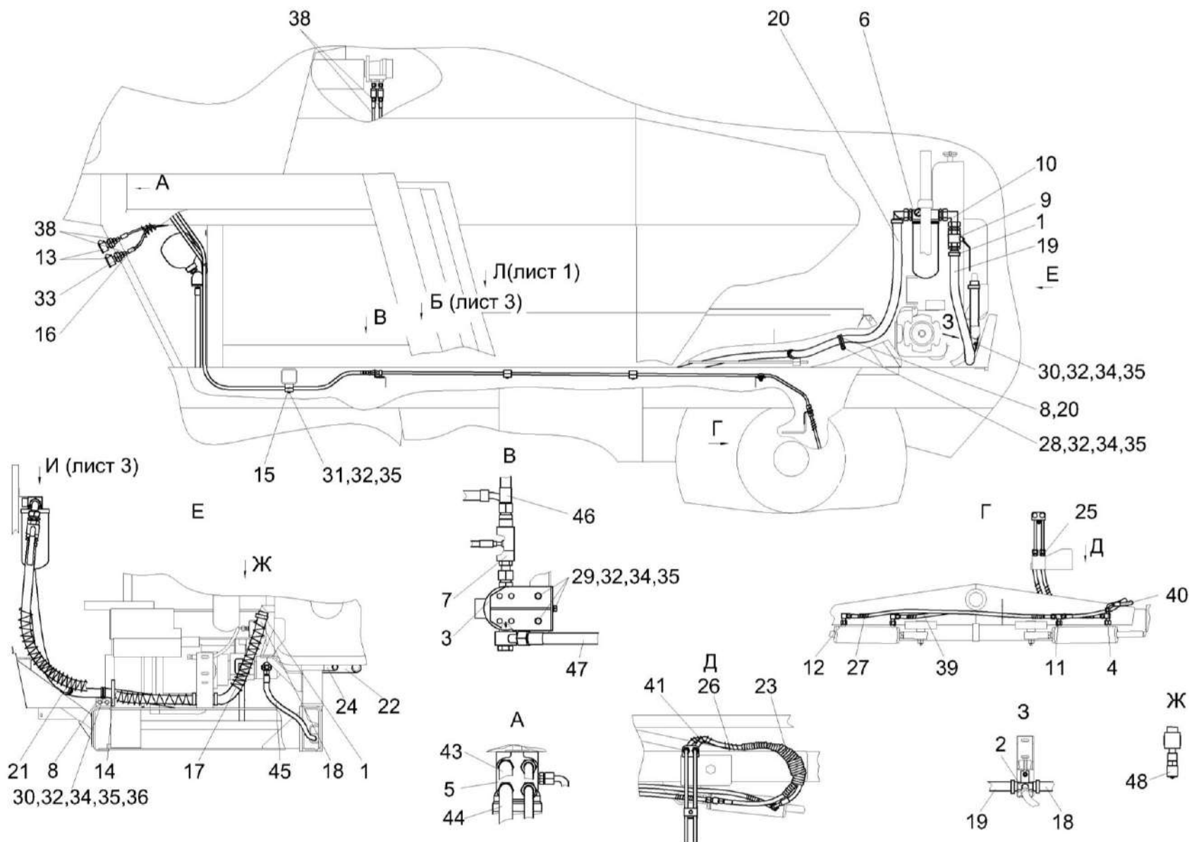
Рисунок 211 – Гидросистема рабочих органов и рулевого управления КВС-5-0602000-01 (лист 2)
