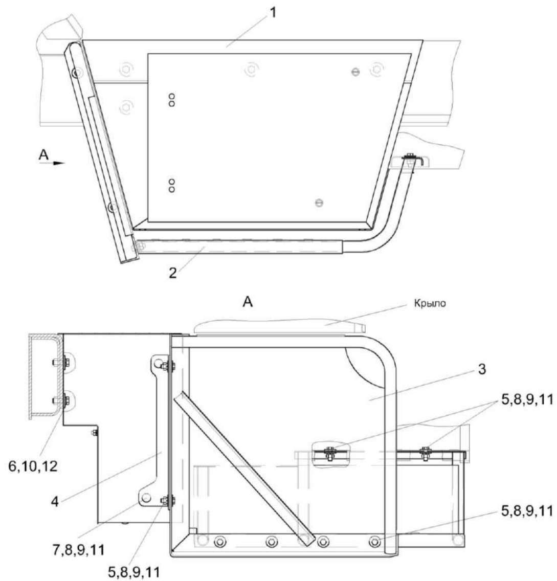
Рисунок 190 – Установка ящика КВС-8-0173000
