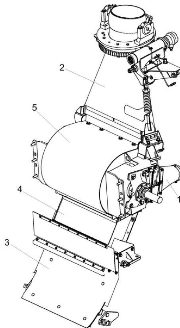
Рисунок 123 – Установка технологического тракта КВС-80-8-0140000 (общий вид)
