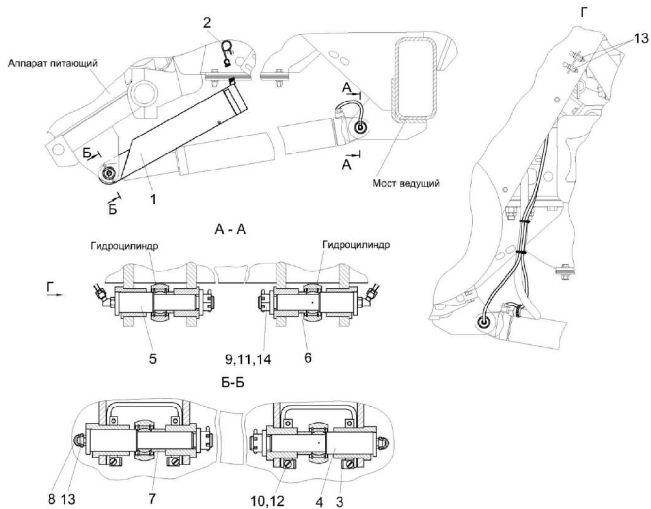
Рисунок 26 – Механизм вывешивания КВС-1-0105000А
