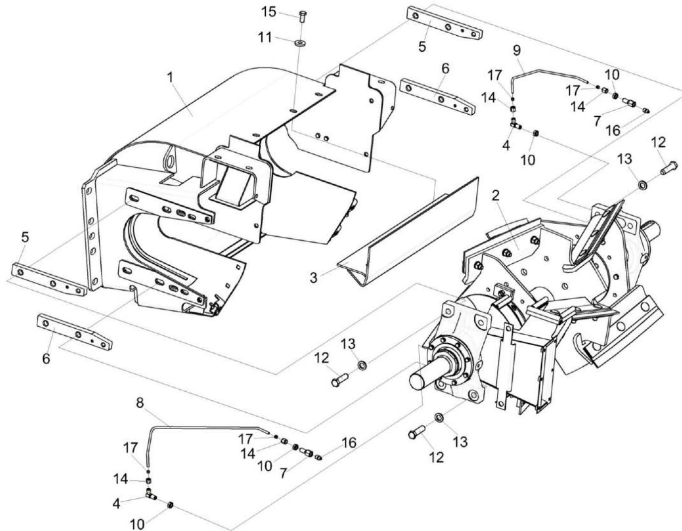
Рисунок 128 – Ускоритель выброса КВС-2-0142000 (лист 2)
