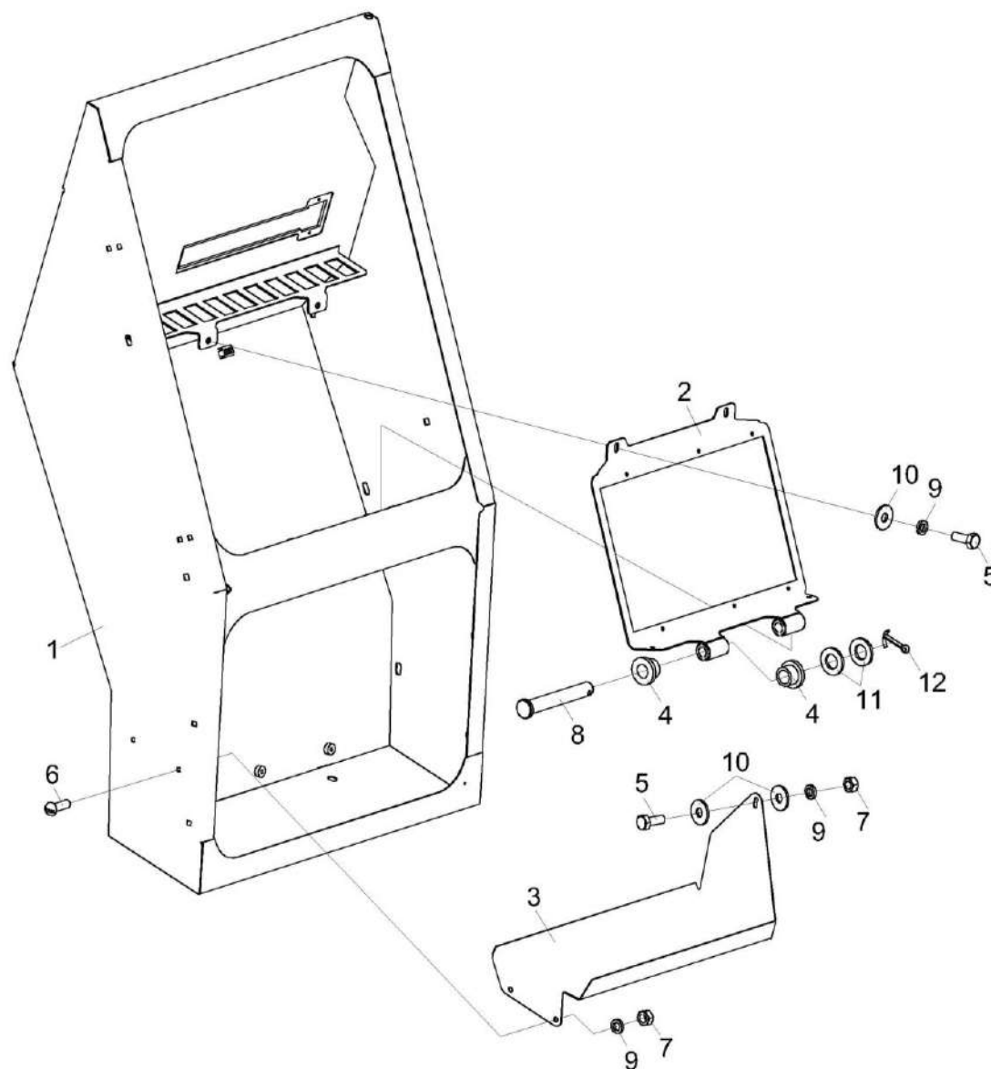
Рисунок 255 – Электрощкаф КВС-8-0702010 (лист 2)
