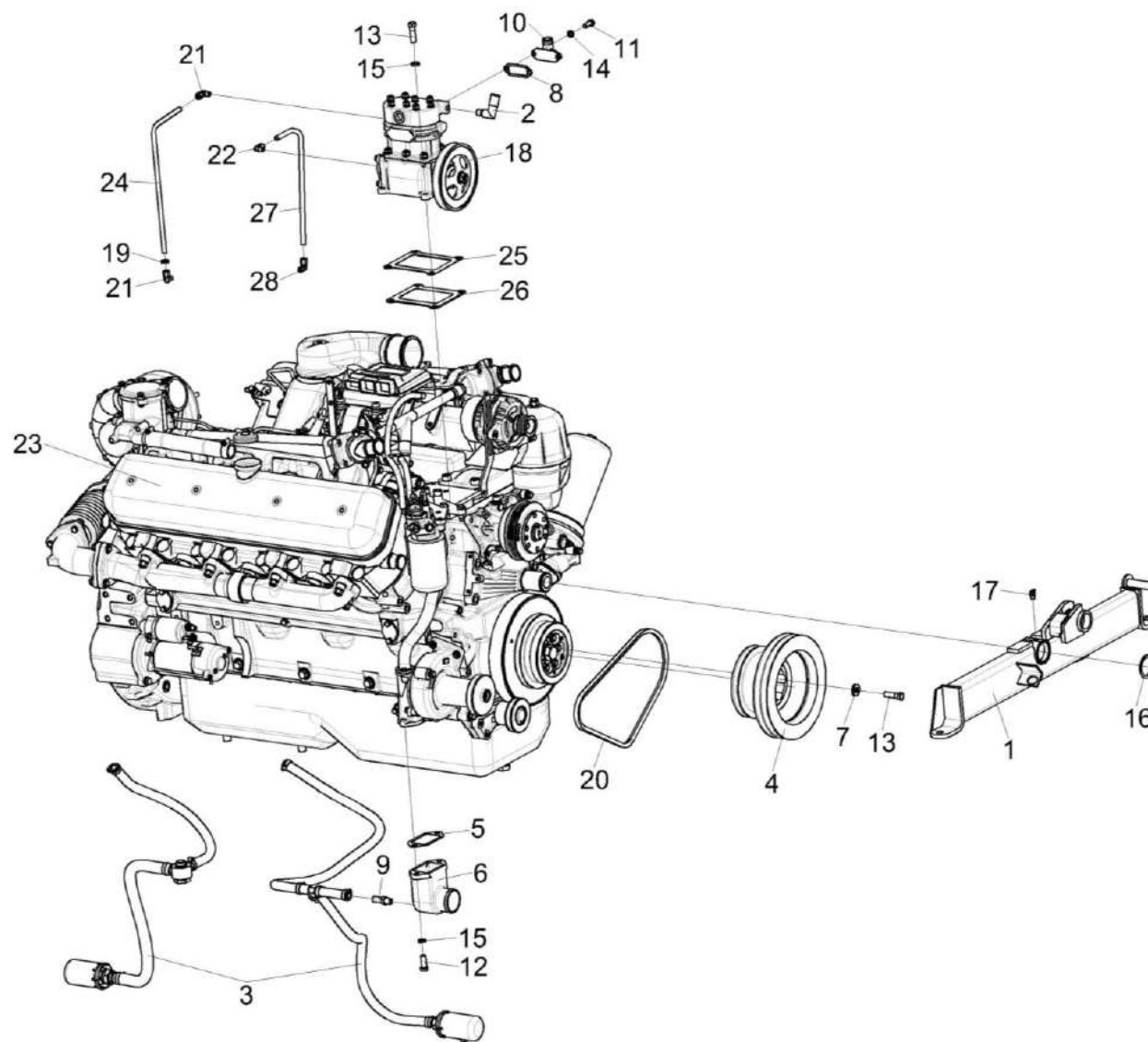
Рисунок 33 – Двигатель КВС-80-7-0150010 (лист 2)
