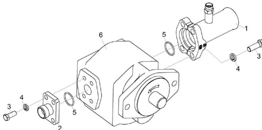
Рисунок 237 – Гидронасос шестеренный КВС-5-0624320
