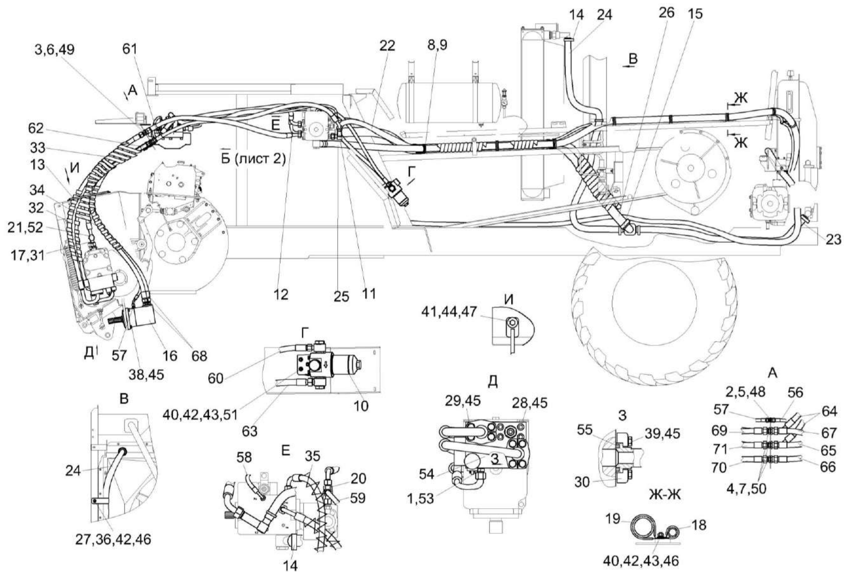
Рисунок 232 – Гидросистема привода питающего аппарата и адаптеров КВС-5-0624000 (лист 1)
