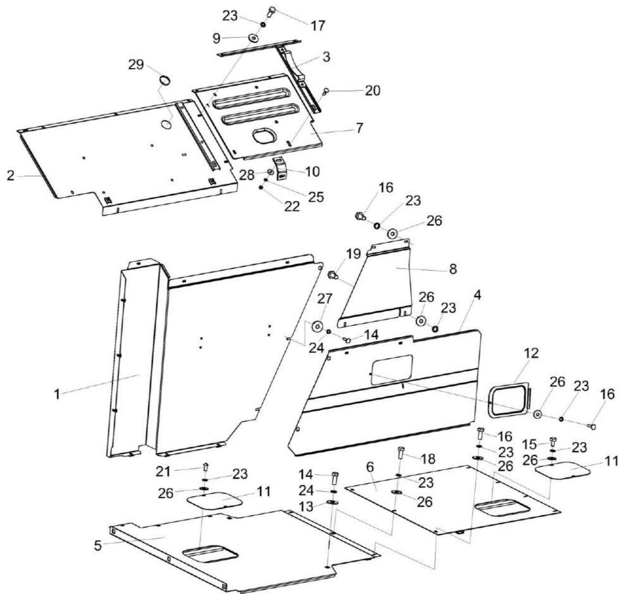
Рисунок 188 – Установка настилов и ограждений КВС-2-0169000-03
