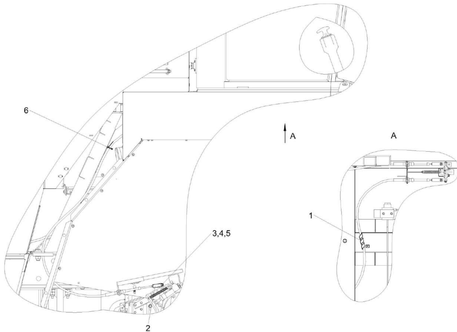
Рисунок 157 – Установка тросов стояночного тормоза КВС-80-8-0119610
