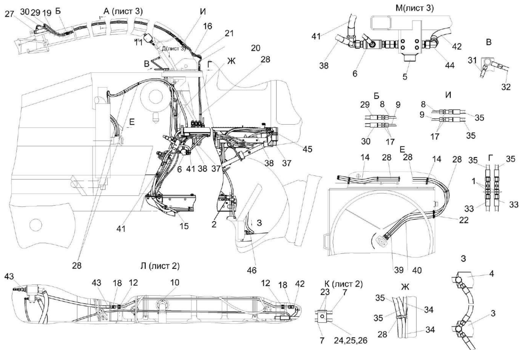
Рисунок 210 – Гидросистема рабочих органов и рулевого управления КВС-5-0602000-01 (лист 1)
