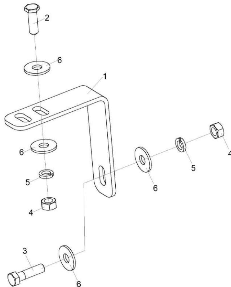
Рисунок 176 – Установка конденсатора КВС-8-0121080
