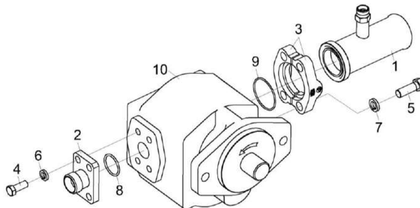
Рисунок 238 – Гидронасос шестеренный КВС-5-0624330
