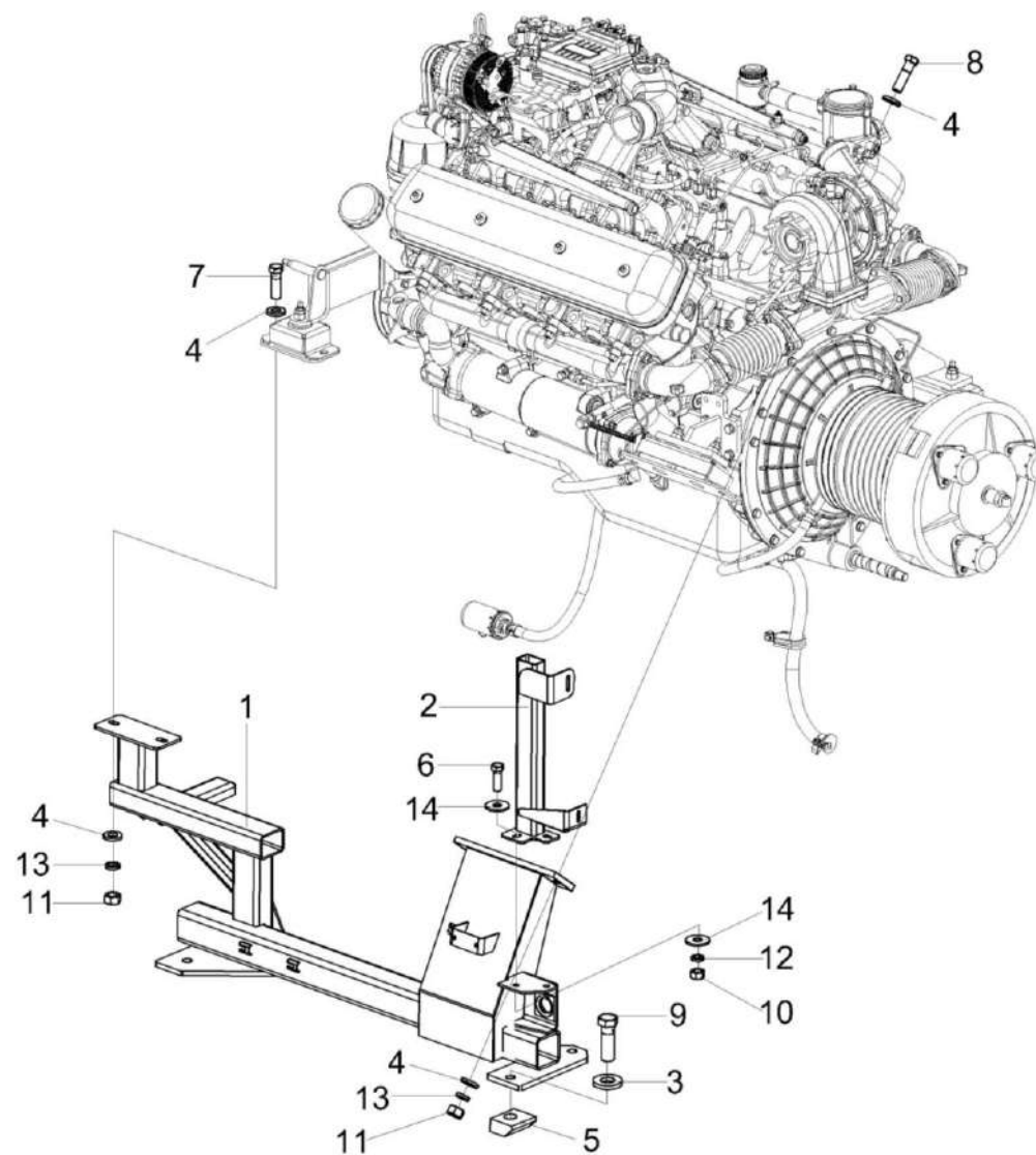
Рисунок 30 – Установка двигателя КВС-80-7-0150000 (лист 3)
