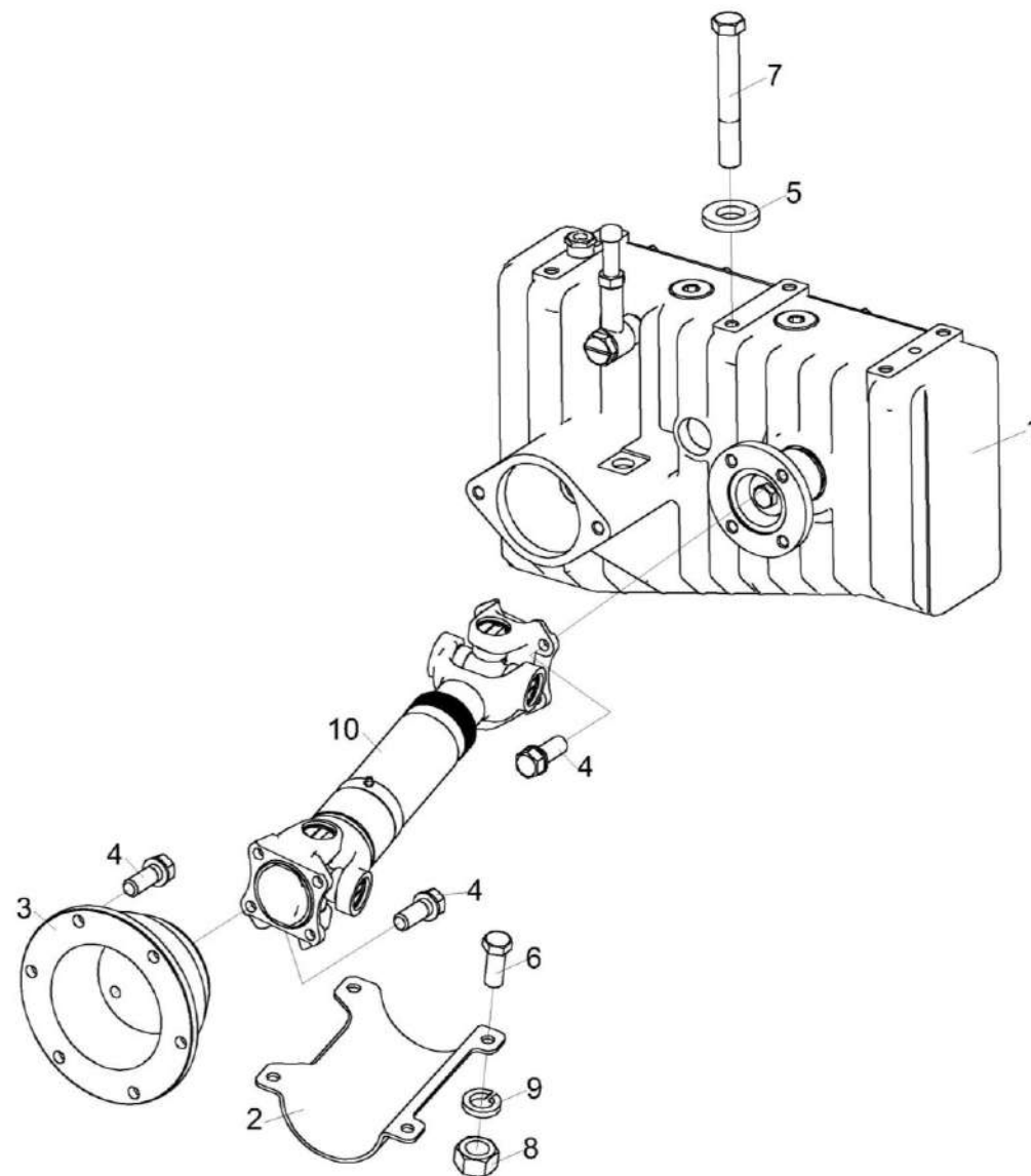
Рисунок 94 – Установка редуктора КВС-80-8-0131500
