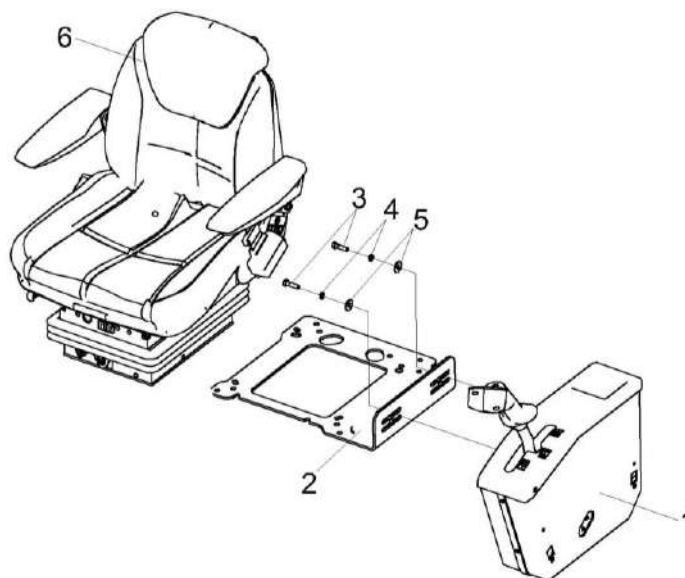
Рисунок 142 – Сиденье КВС-80-8-0119290
