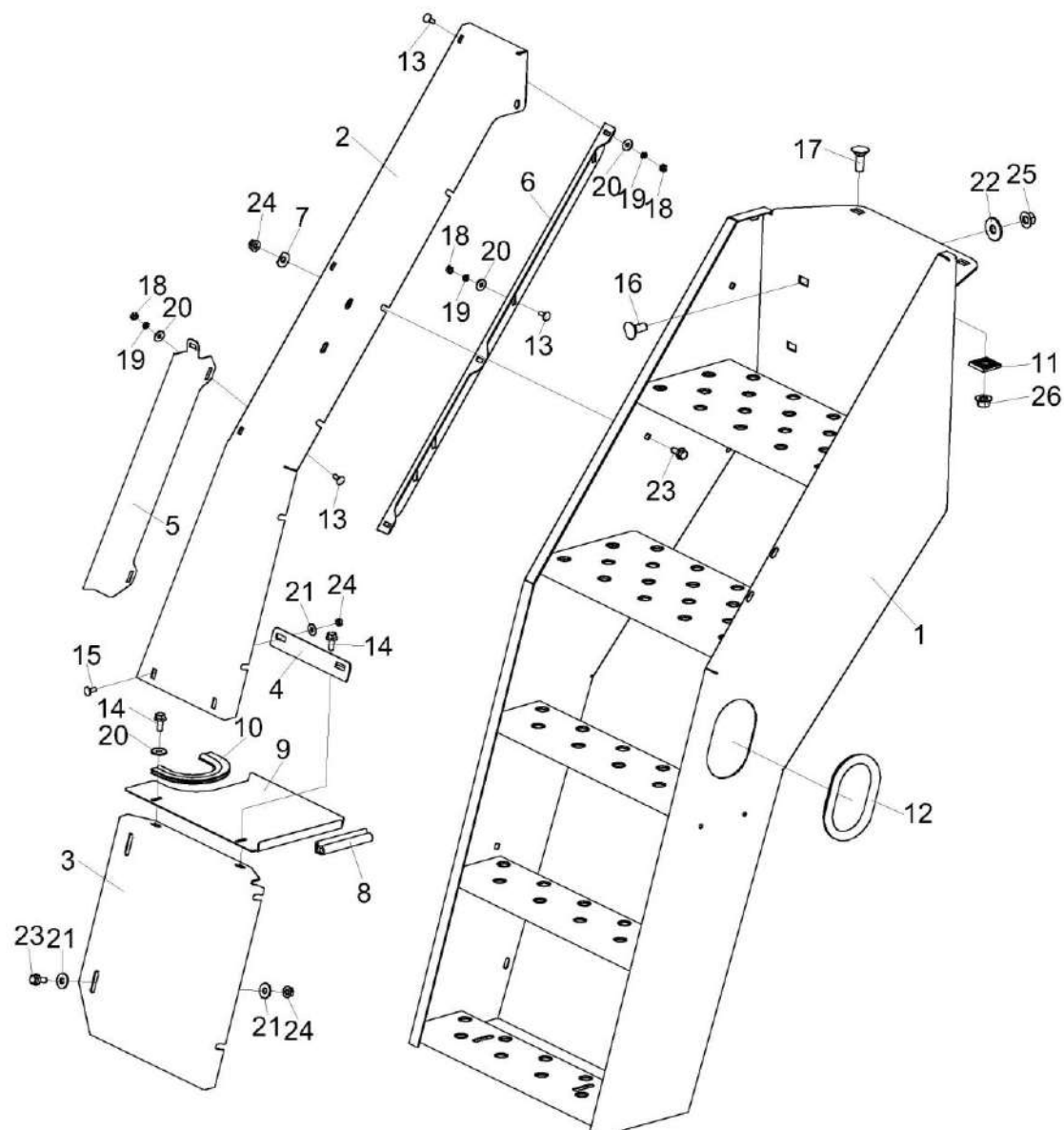
Рисунок 189 – Установка трапа КВС-80-8-0175000
