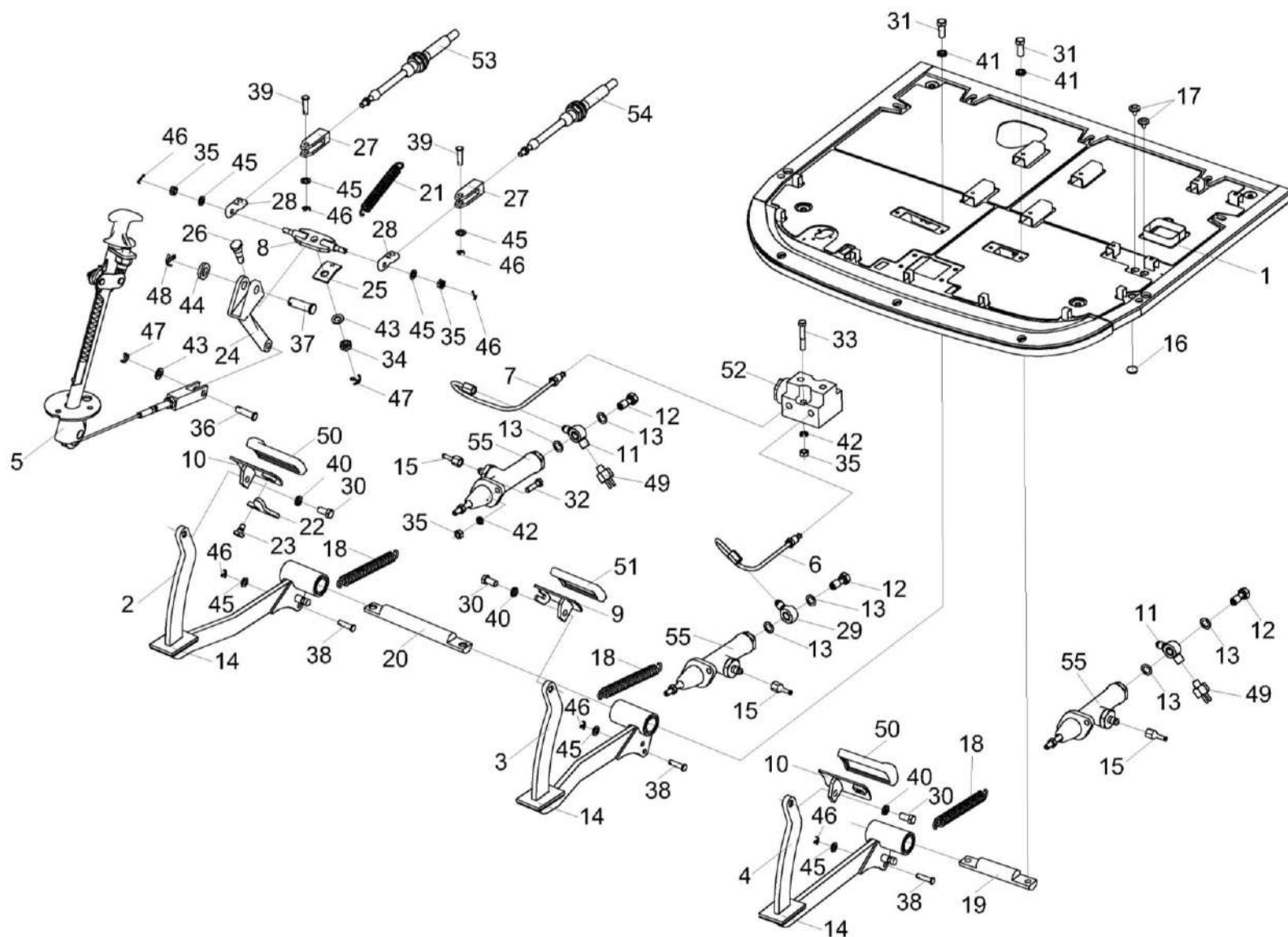
Рисунок 141 – Площадка управления КВС-80-8-0119000 (лист 2)
