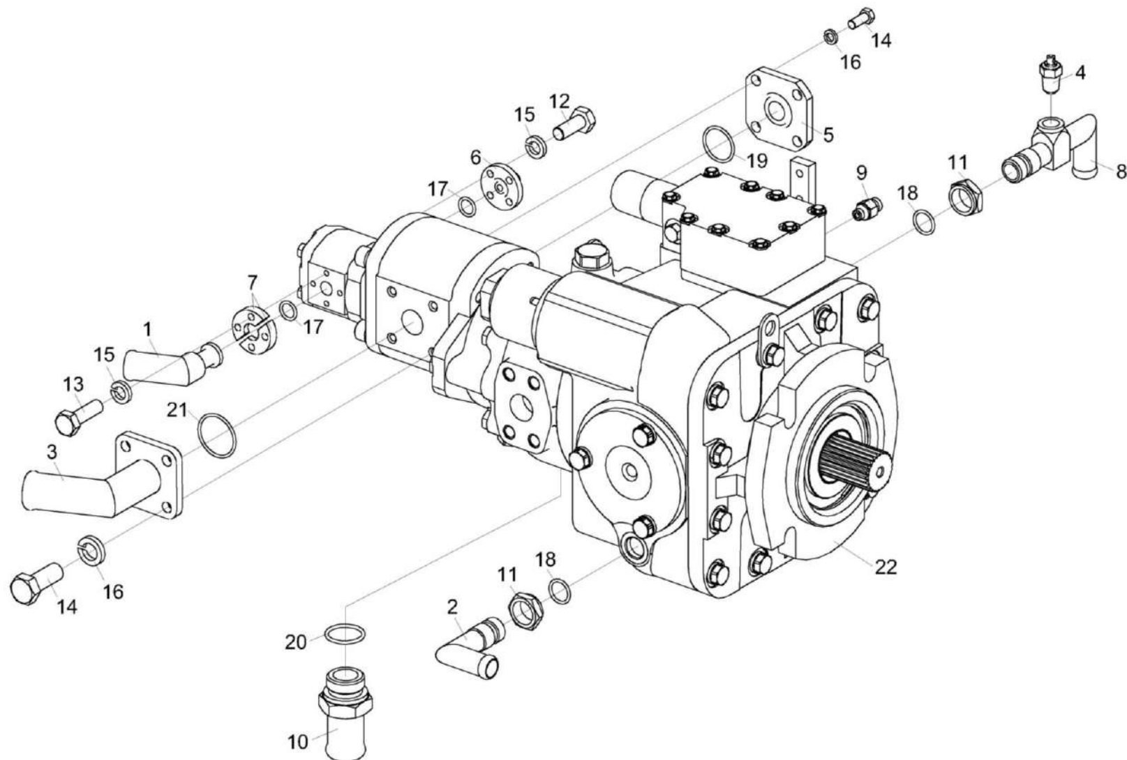
Рисунок 224 – Насос трехсекционный КВС-8-0600100
