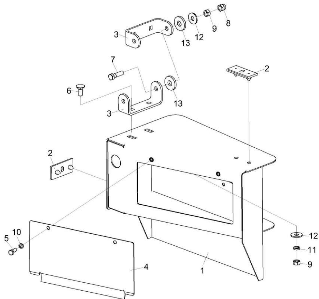
Рисунок 196 – Корпус фонарей КВС-2-0101480А и КВС-2-0101480А-01
