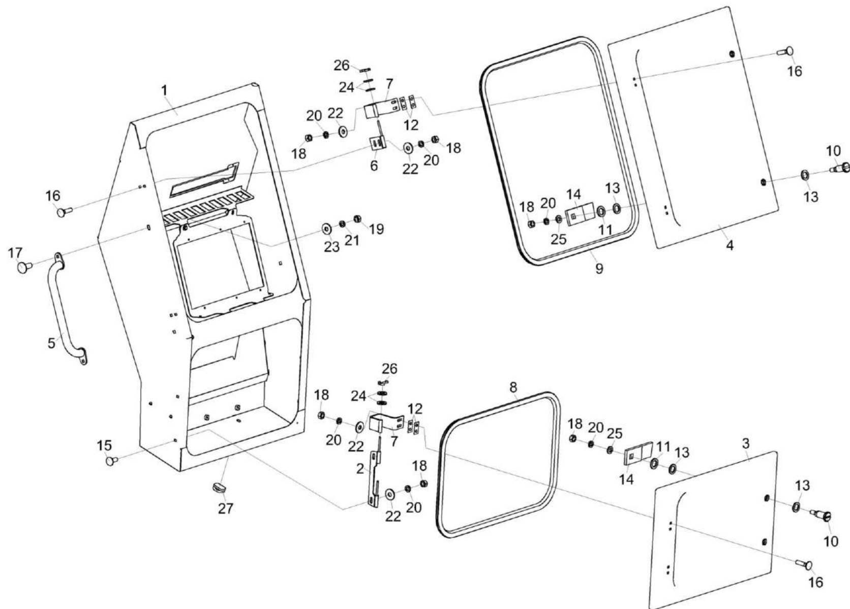
Рисунок 254 – Электрощкаф КВС-8-0702010 (лист 1)
