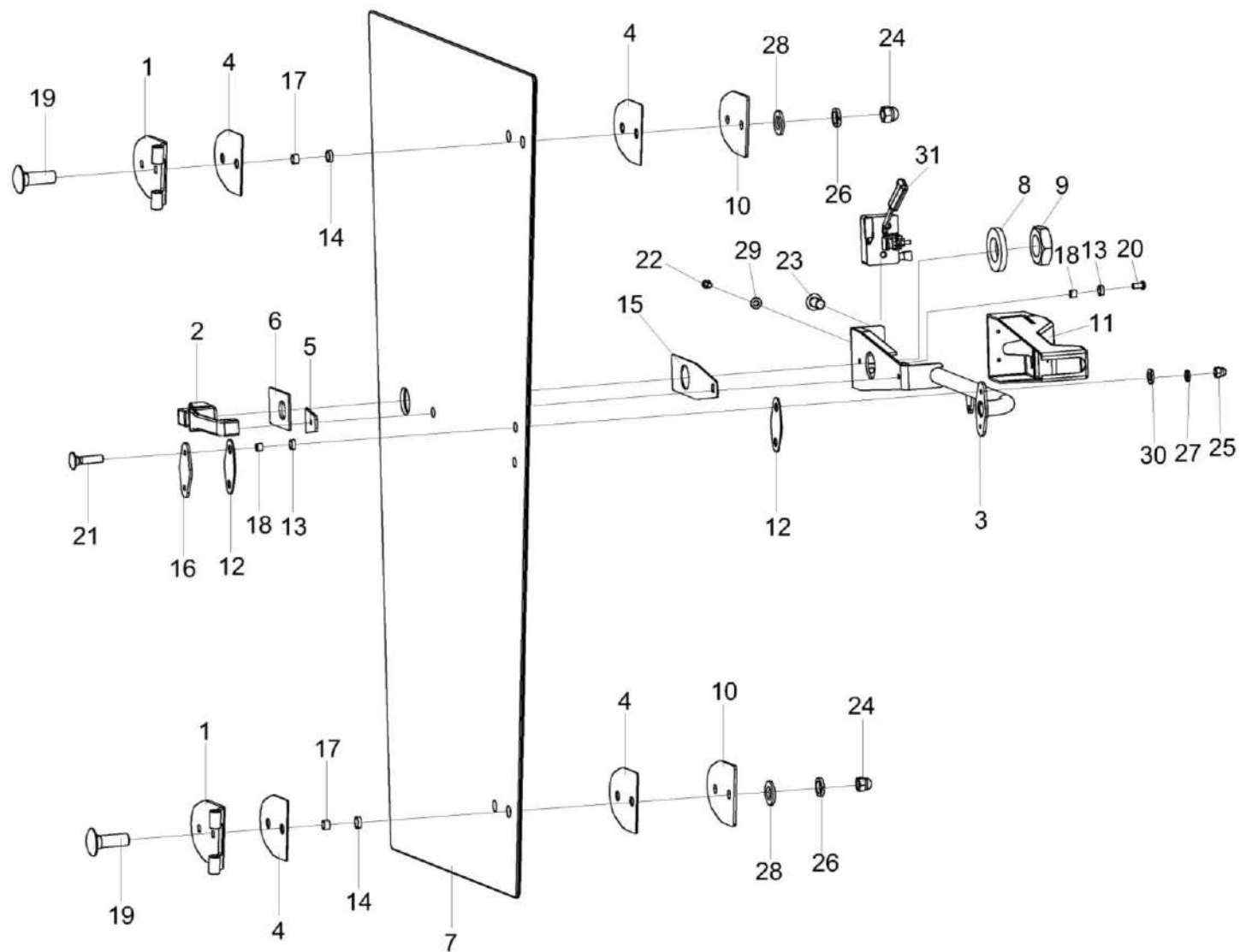
Рисунок 170 – Дверь КЗК-12-0131070-01
