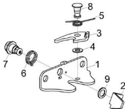
Рисунок 184 – Замок КВС-1-0160240
