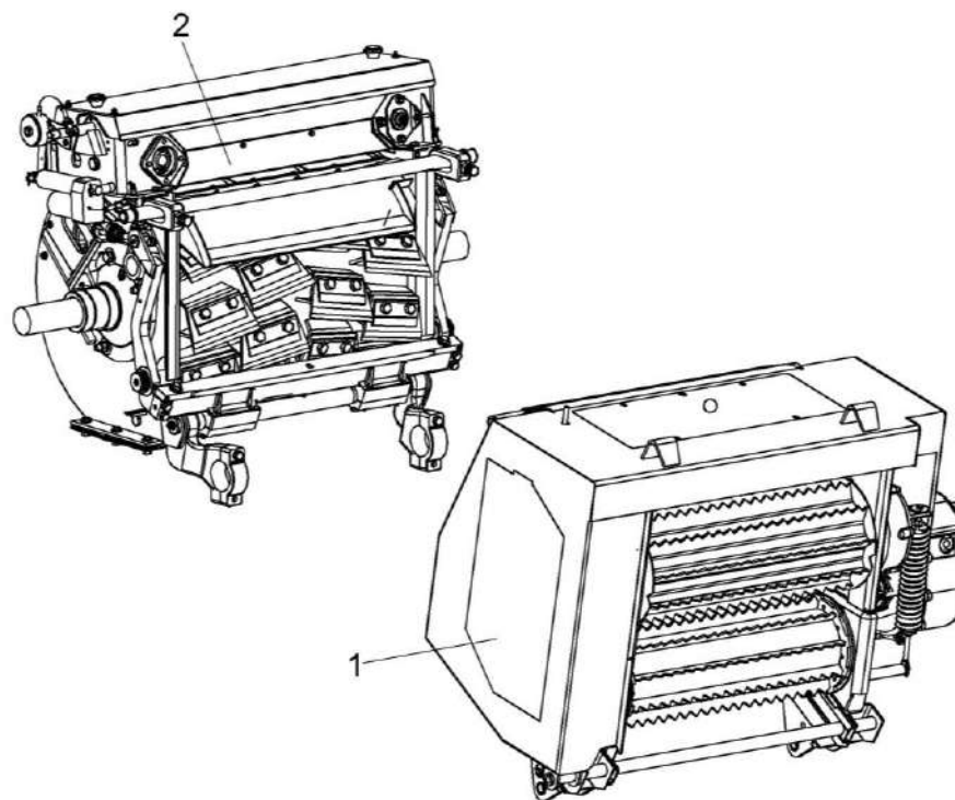
Рисунок 59 – Аппарат питающе-измельчающий КВС-8-0110000-01
