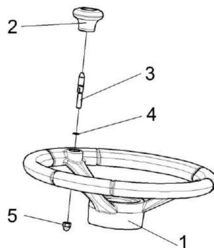
Рисунок 153 – Колесо рулевое КЗК-12-0122300
