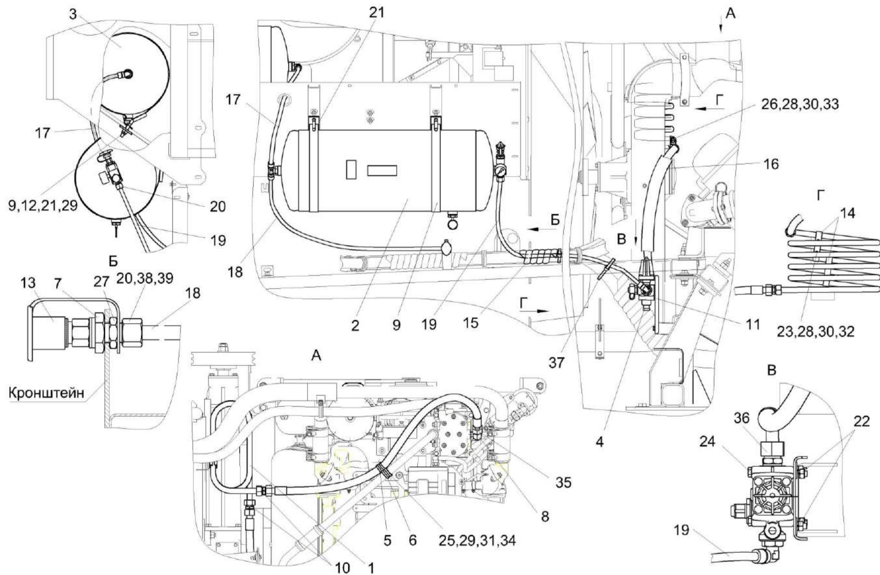
Рисунок 240 – Пневмосистема КВС-7-0800000
