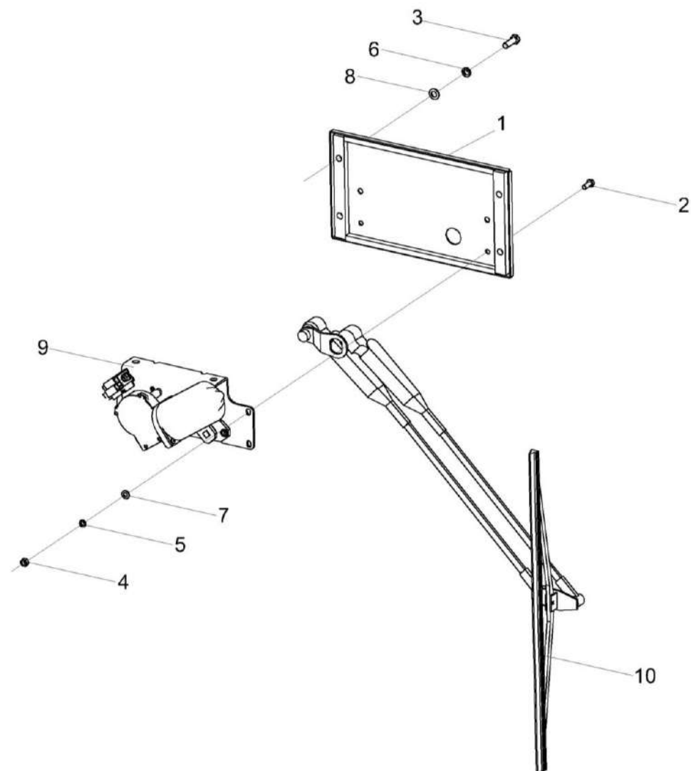
Рисунок 167 – Установка стеклоочистителя КВС-80-8-0120090
