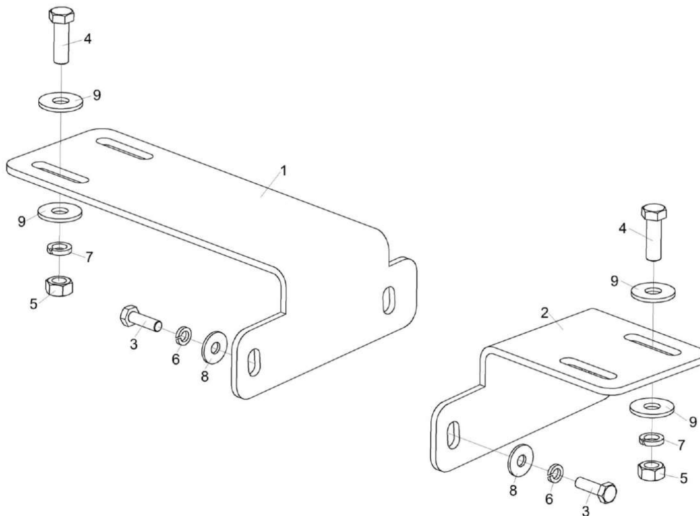
Рисунок 179 – Установка блока испарительного-отопительного КВС-8-0121090
