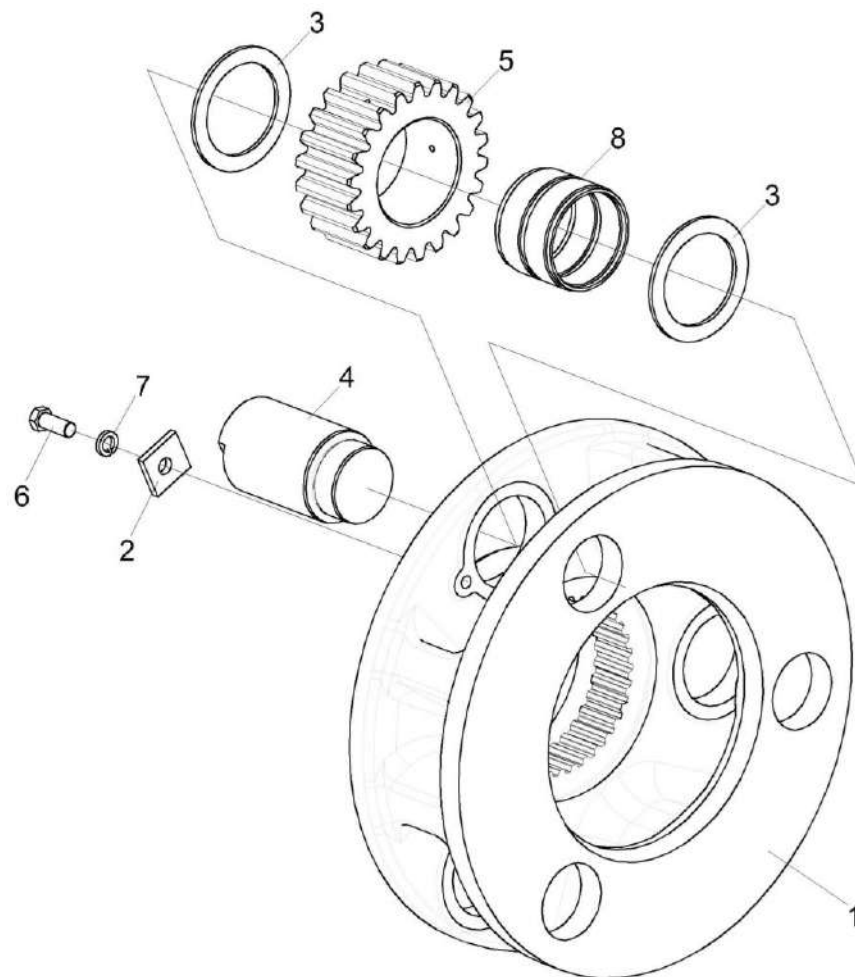
Рисунок 14 – Водило КЗК-12А-12-0107210
