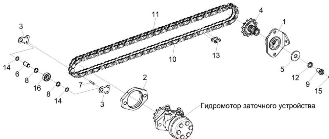
Рисунок 86 – Привод каретки КВС-2-0116650
