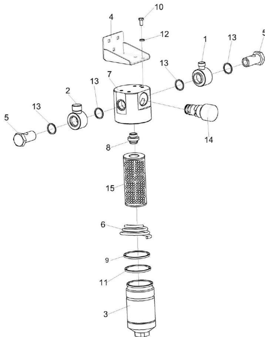
Рисунок 227 – Фильтр напорный КВС-5-0604360
