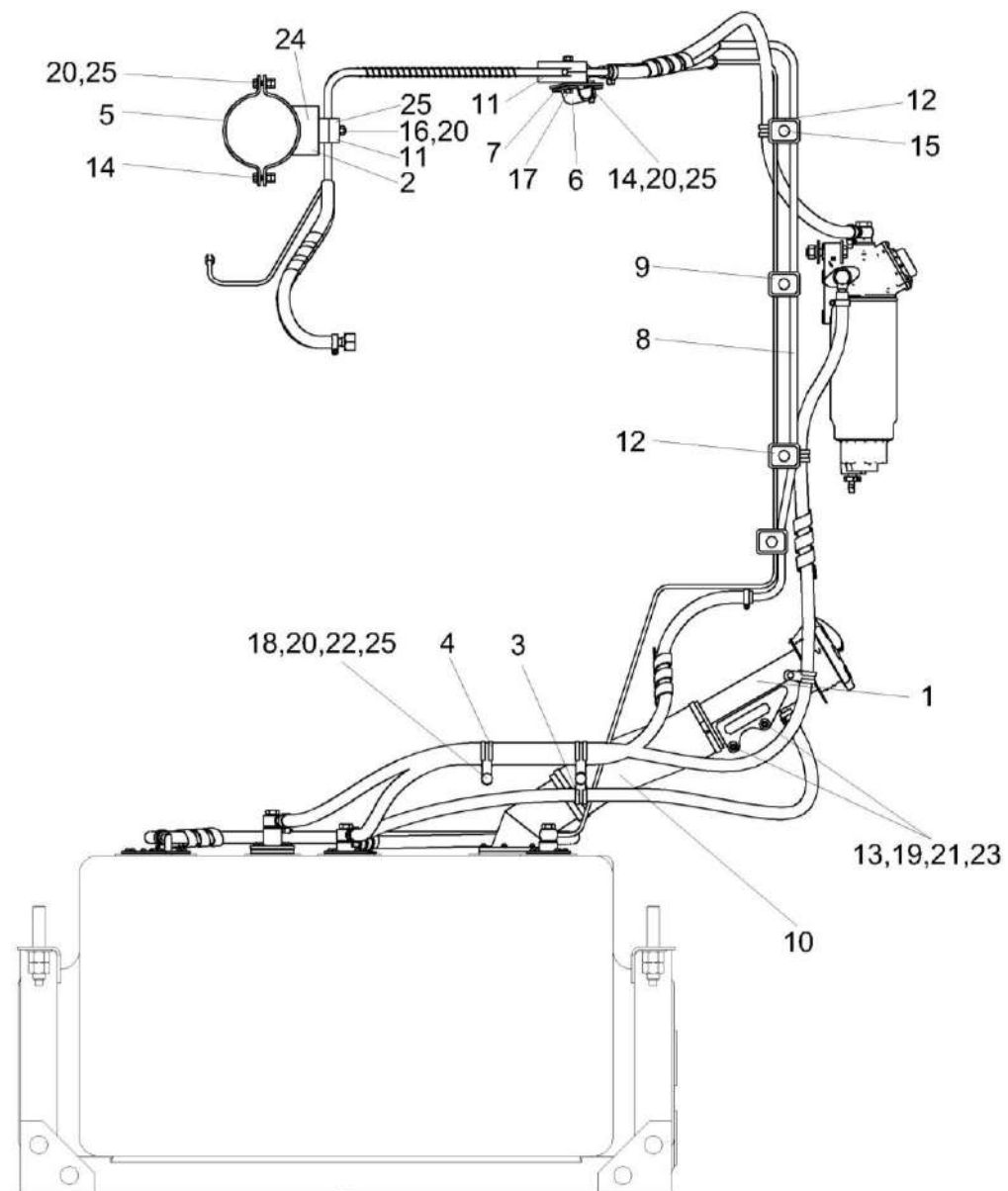
Рисунок 202 – Установка топливного оборудования КВС-7-0103700 (лист 3)
