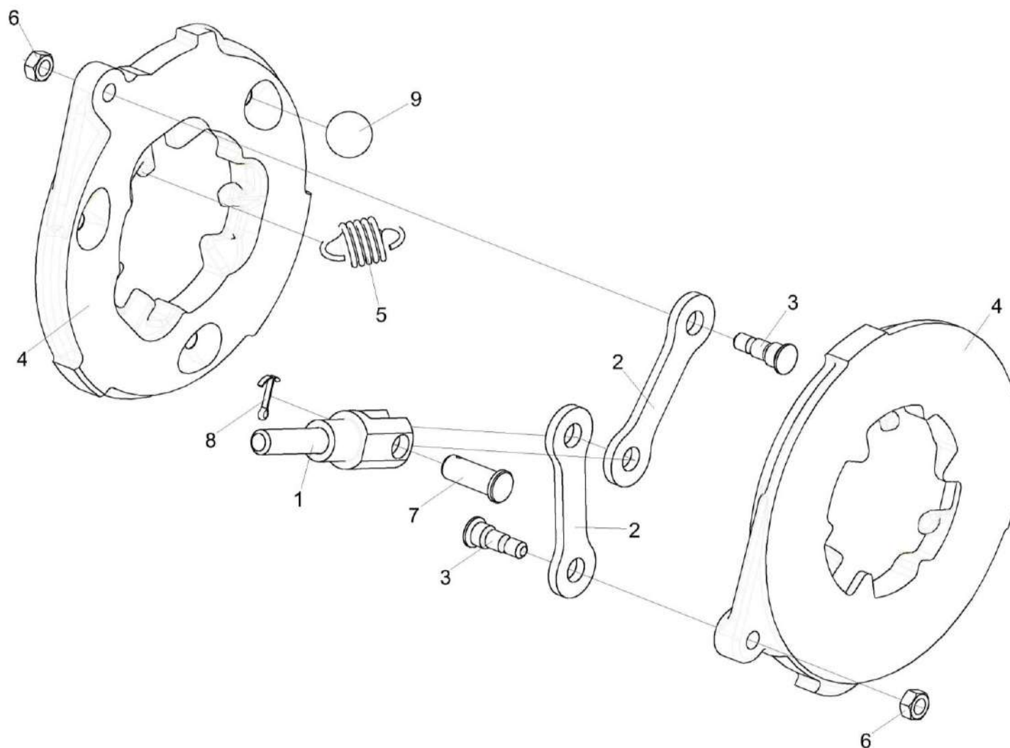
Рисунок 13 – Диски нажимные МК-23М.03.030А
