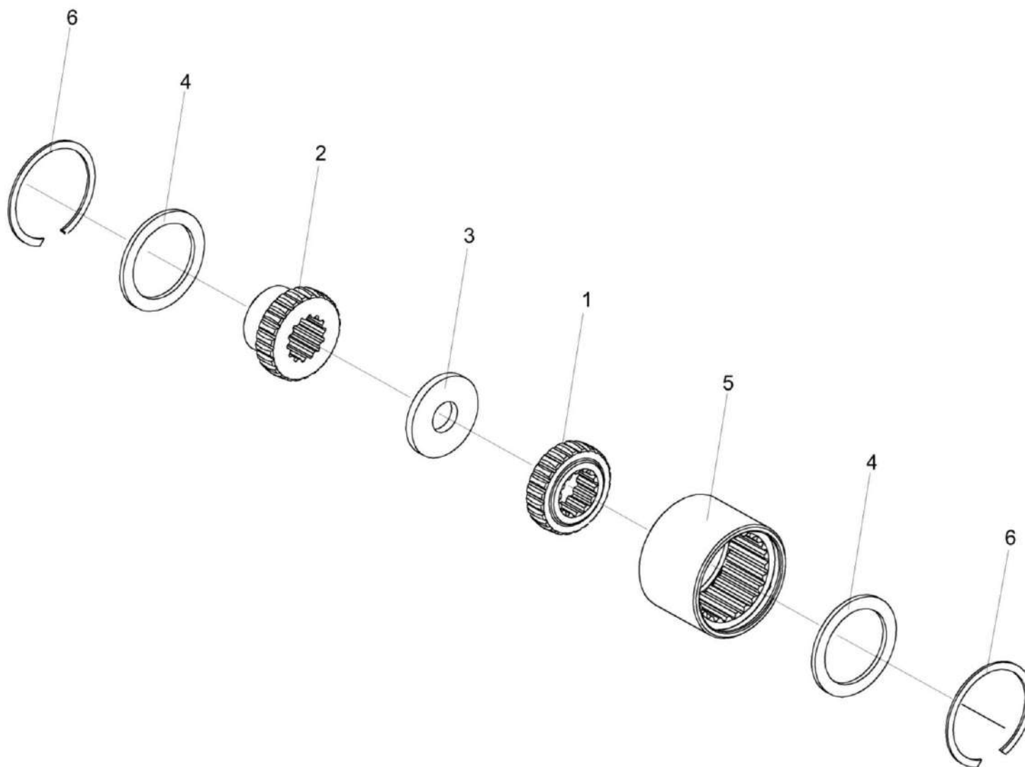
Рисунок 239 – Муфта КГС 0100110 и КГС 0100140
