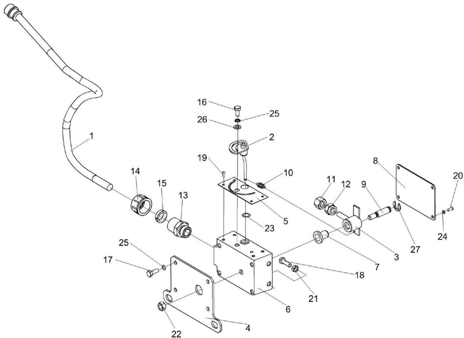
Рисунок 75 – Датчик камнедетектора КВС-1-0111070-01
