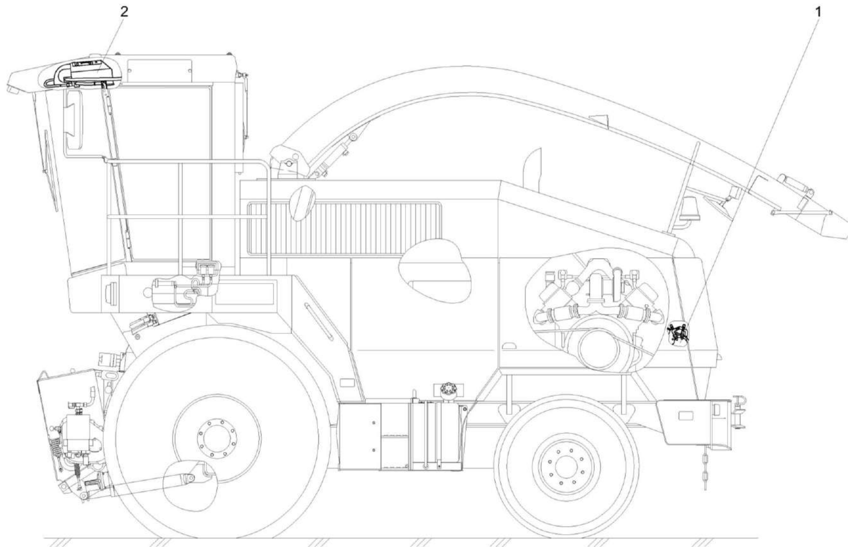
Рисунок 173 – Установка климатическая КВС-80-7-0121000 и КВС-80-7-0121000-01
