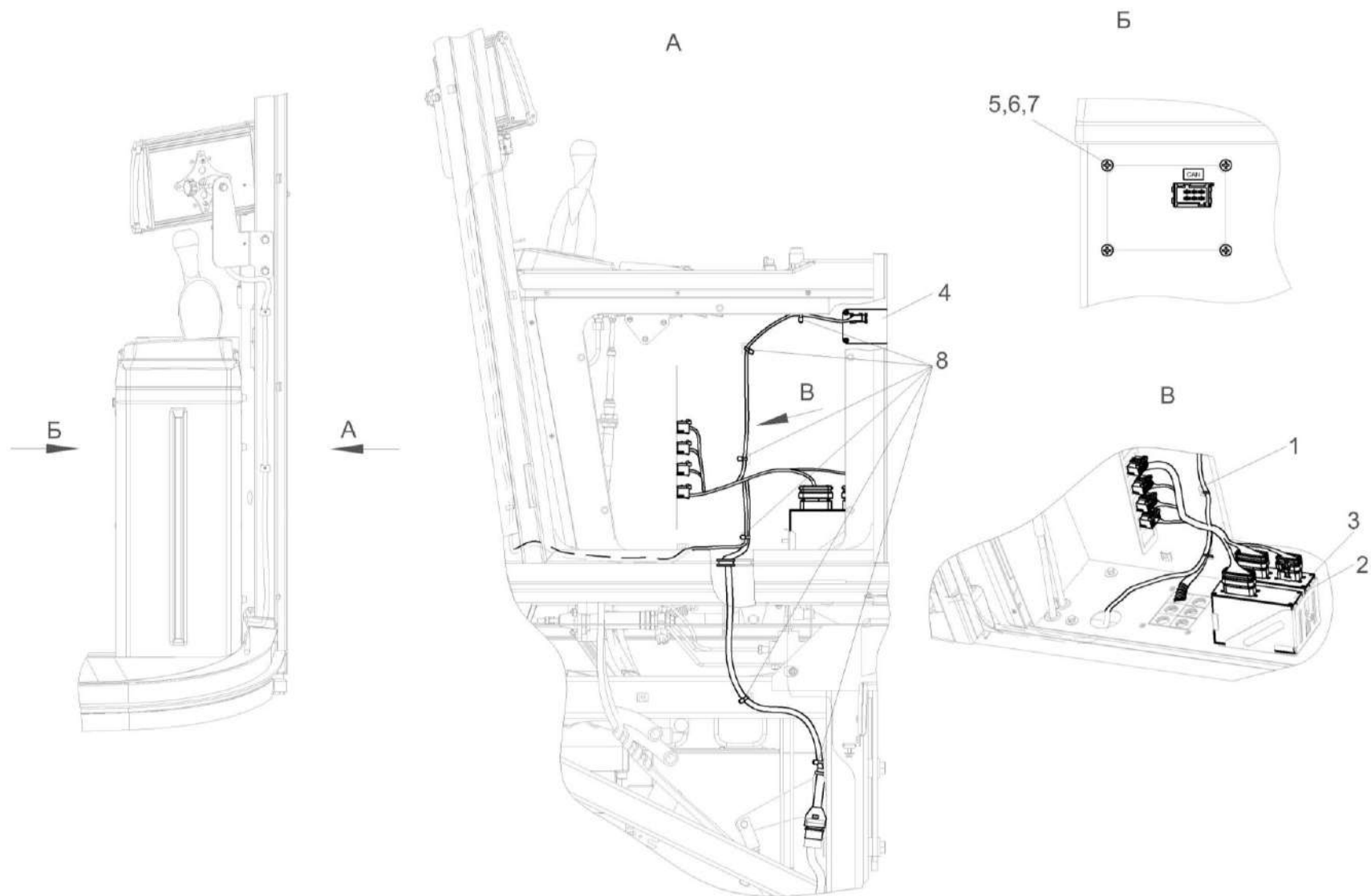
Рисунок 149 – Установка автоматики пульта КВС-80-8-0701750
