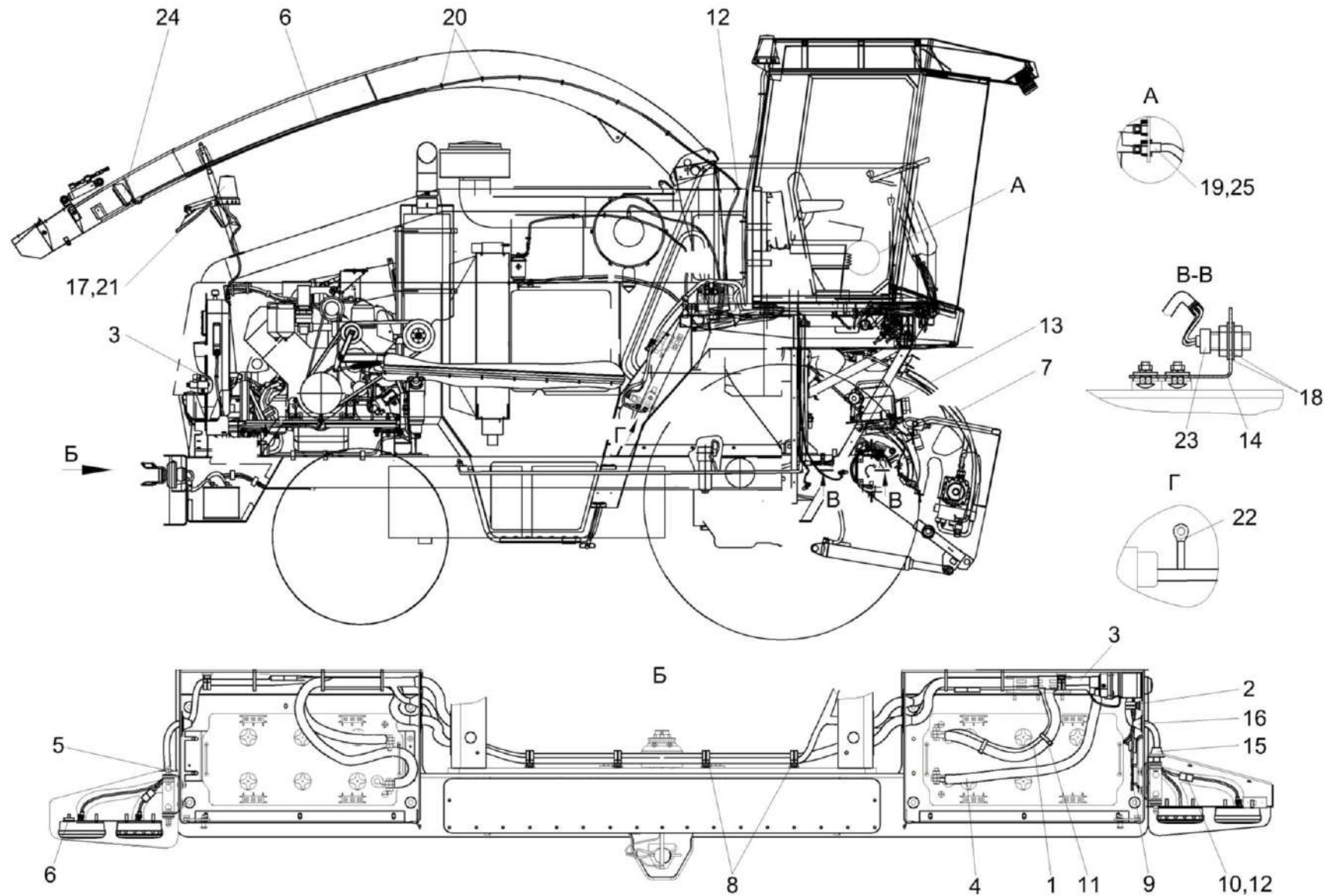
Рисунок 249 – Установка электрооборудования КВС-80-7-0721000 (лист 4)
