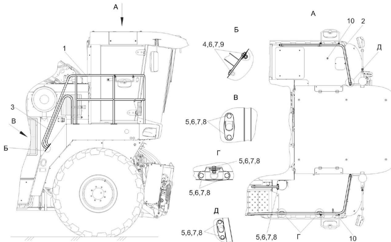
Рисунок 162 – Установка поручней КВС-80-8-0125000
