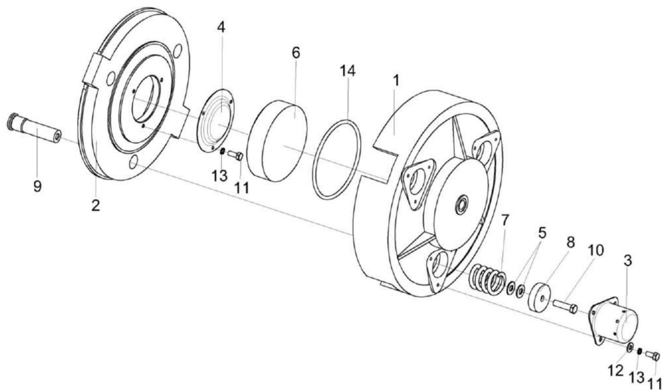
Рисунок 37 – Механизм нажимной КВК 0151040
