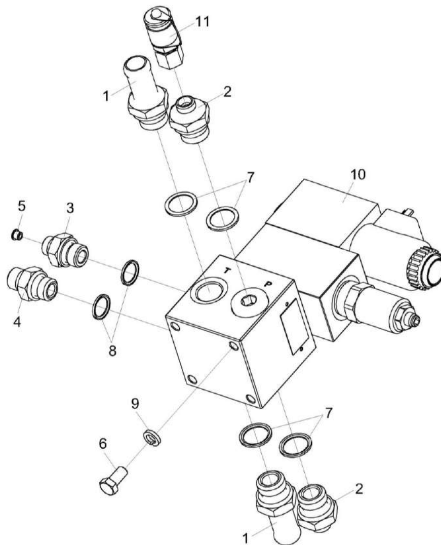
Рисунок 219 – Гидроблок воздухозаборника КВС-5-0602310А
