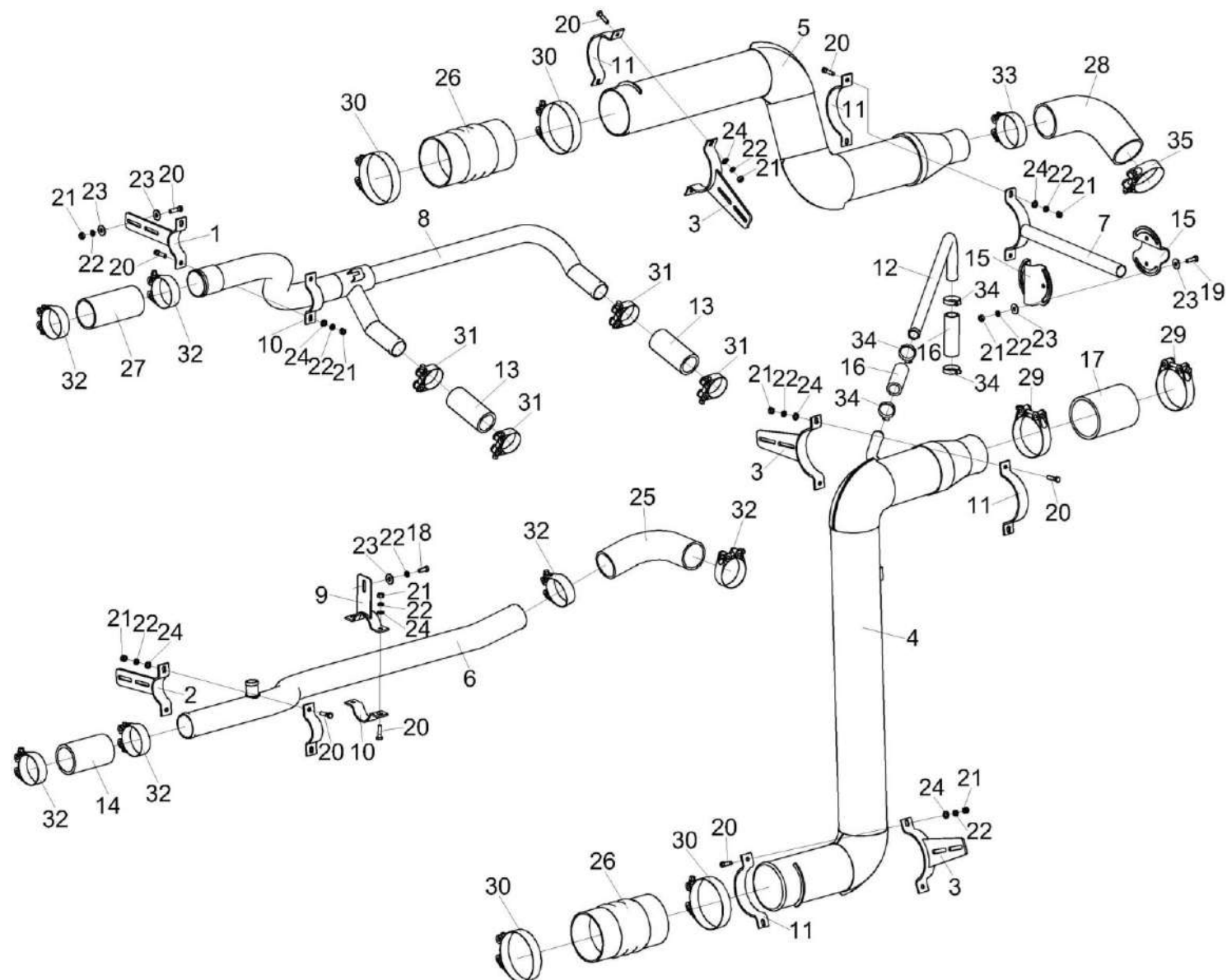
Рисунок 52 – Установка труб КВС-80-7-0150300
