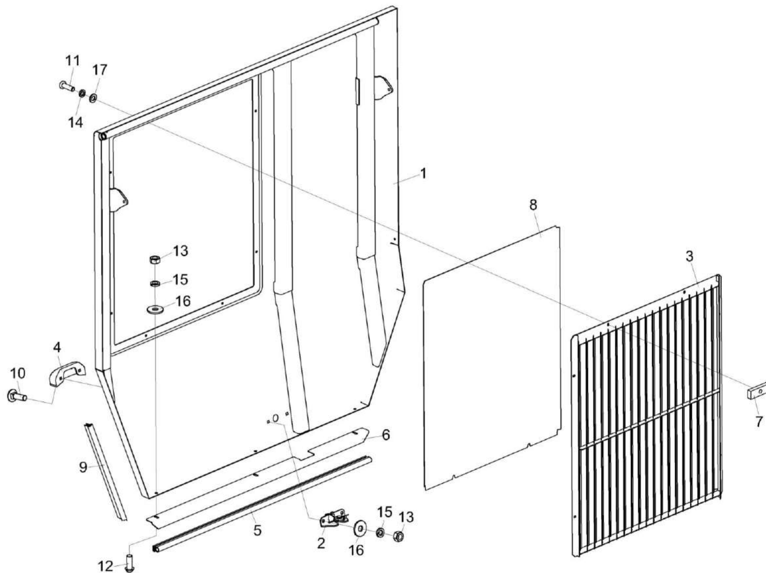
Рисунок 183 – Капот КВС-80-8-0160100-01
