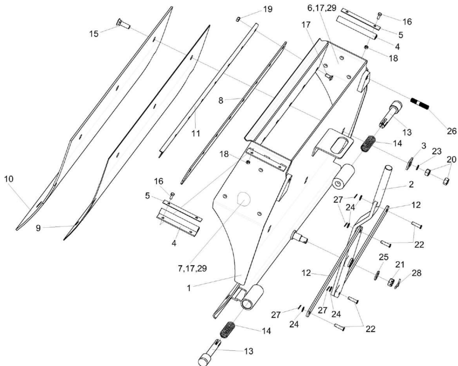
Рисунок 126 – Камера приемная КВС-1-0147000А
