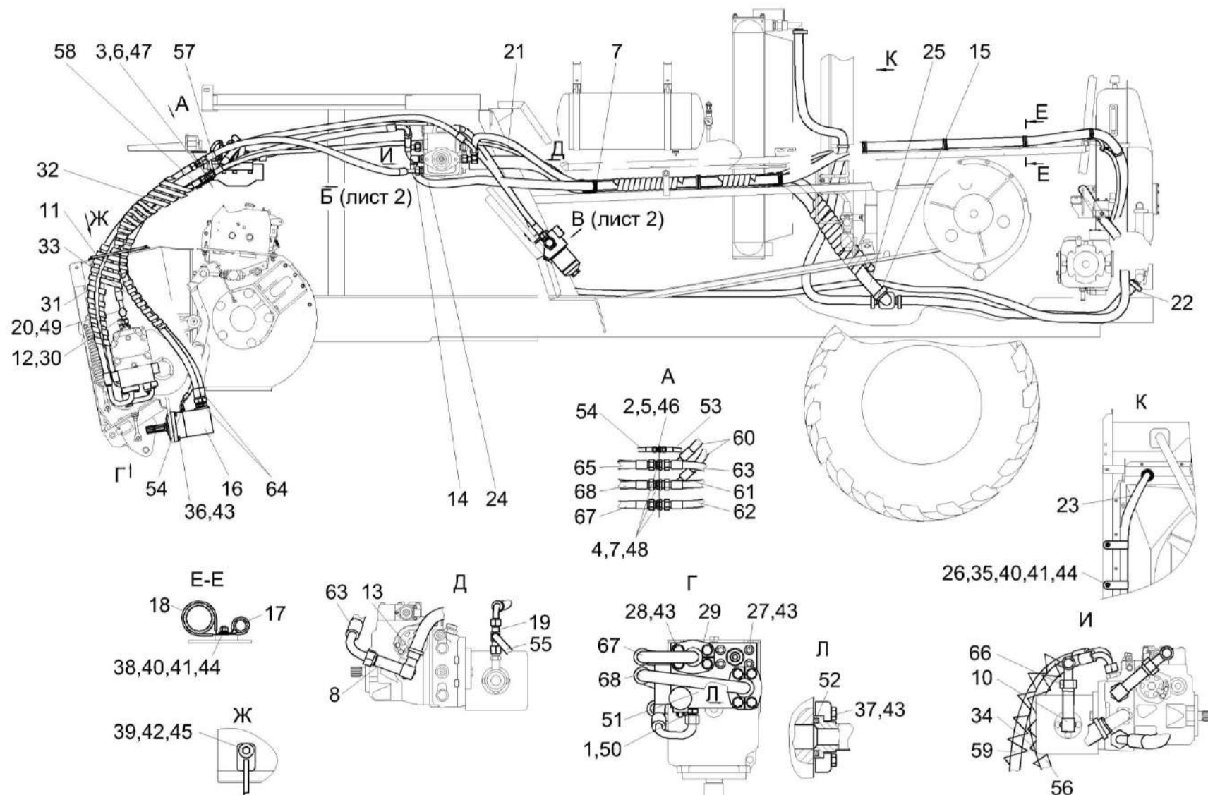
Рисунок 230 – Гидросистема привода питающего аппарата и адаптеров КВС-5-0614000 (лист 1)
