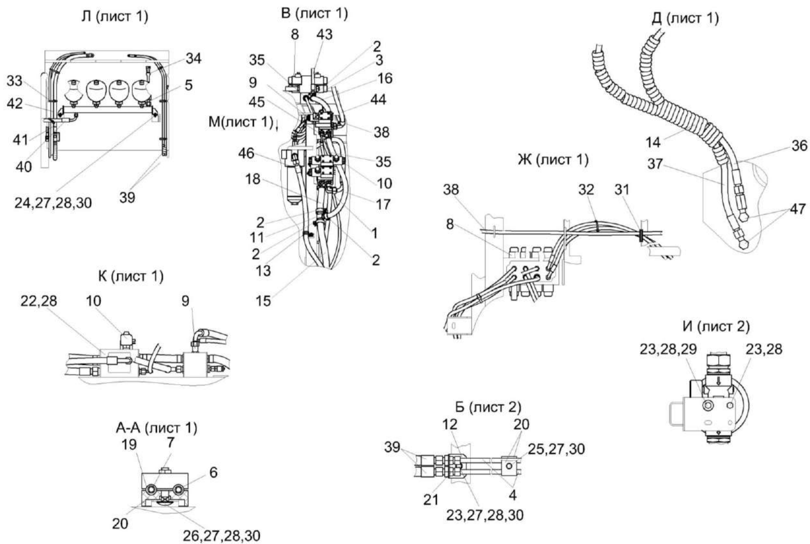
Рисунок 212 – Гидросистема рабочих органов и рулевого управления КВС-5-0602000-01 (лист 3)
