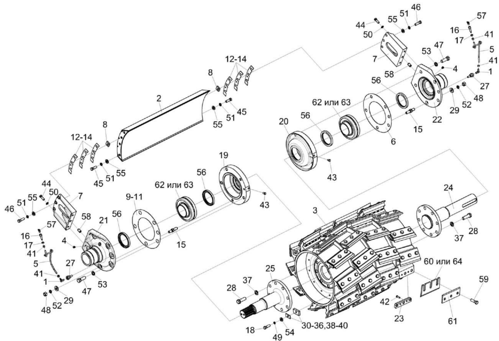
Рисунок 82 – Установка барабана КВС-2-0115430
