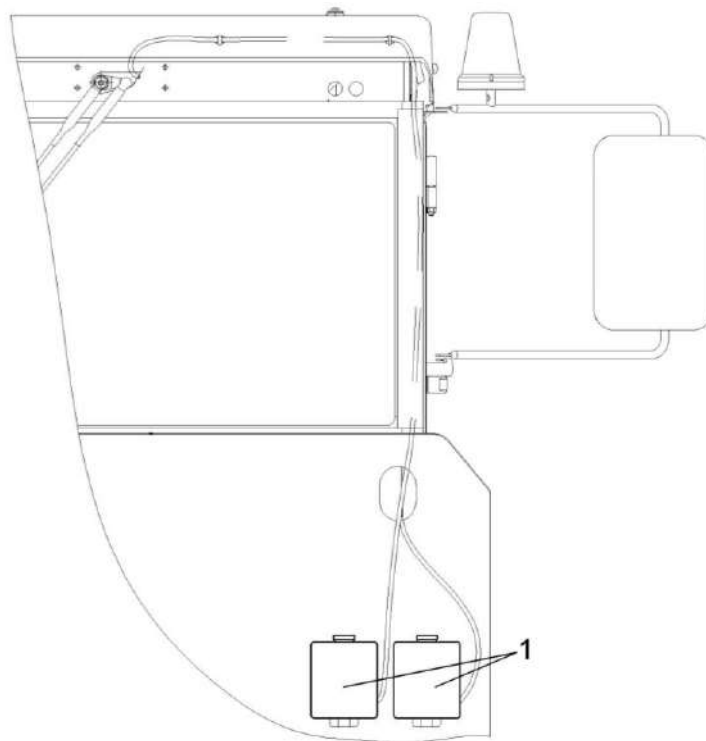
Рисунок 172 – Установка стеклоомывателей КВС-2-0122030
