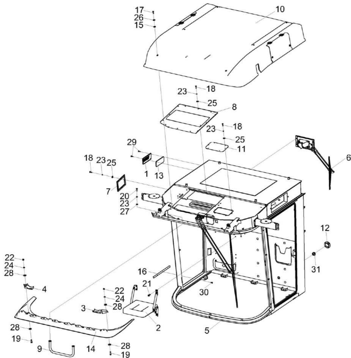
Рисунок 165 – Кабина КВС-80-8-0120010 (лист 2)
