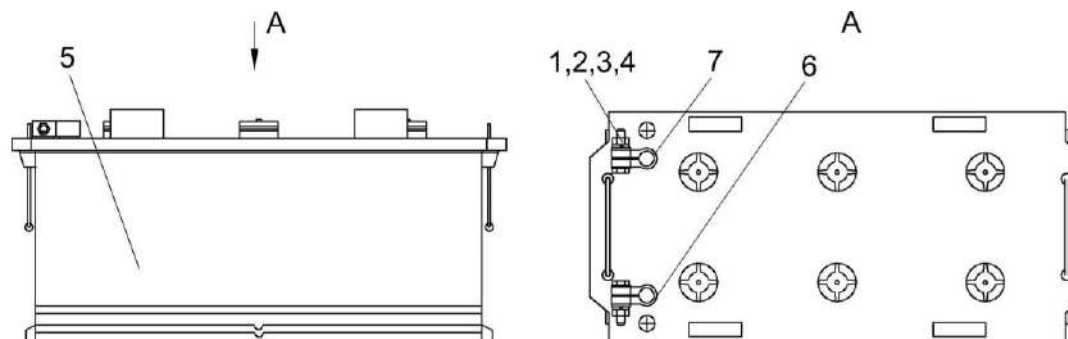
Рисунок 252 – Батарея аккумуляторная с переходниками КЗК 0705190
