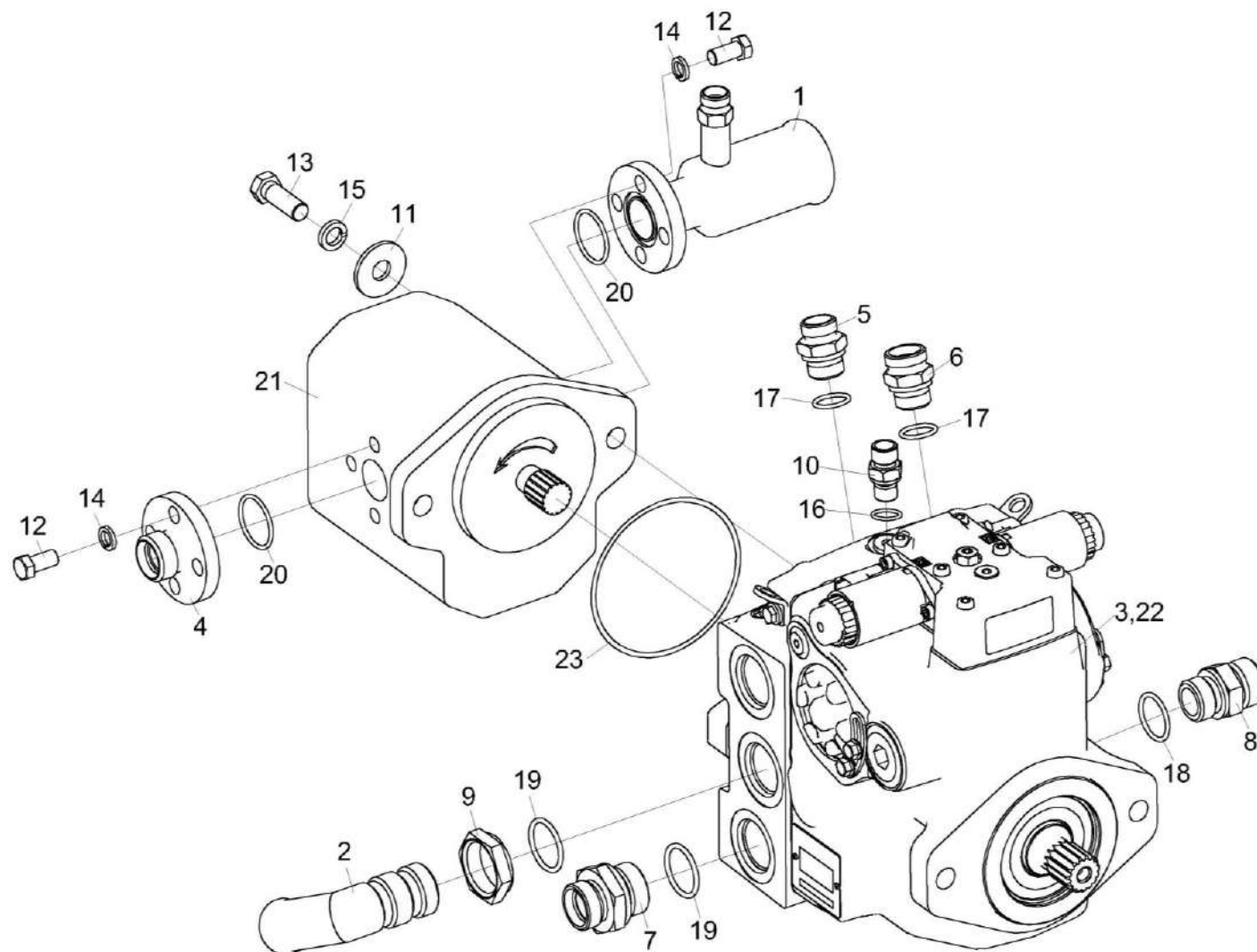
Рисунок 235 – Гидронасос двухсекционный КВС-5-0614340
