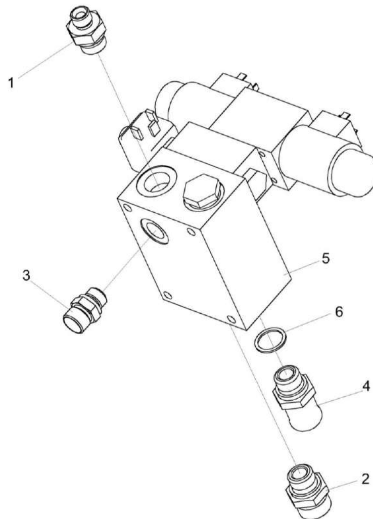
Рисунок 220 – Гидроблок навески КВС-5-0602320
