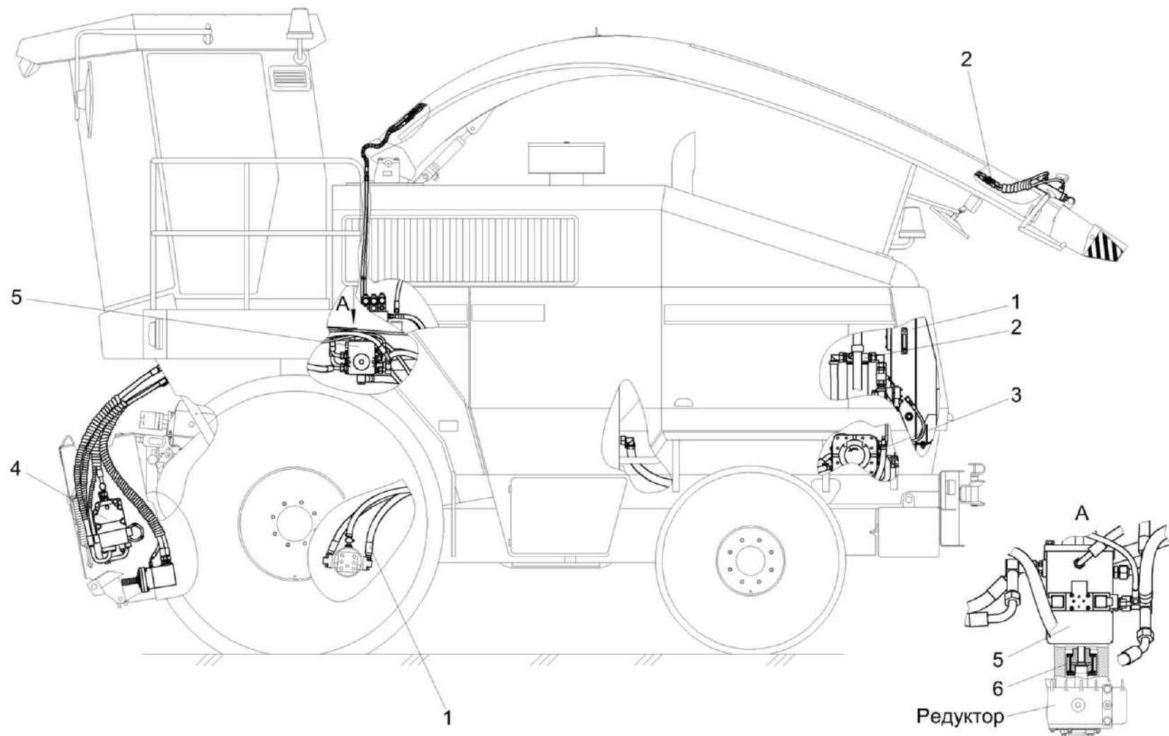
Рисунок 203 – Гидросистема КВС-80-5-0600000, КВС-80-5-0600000-01 и КВС-80-5-0600000-02
