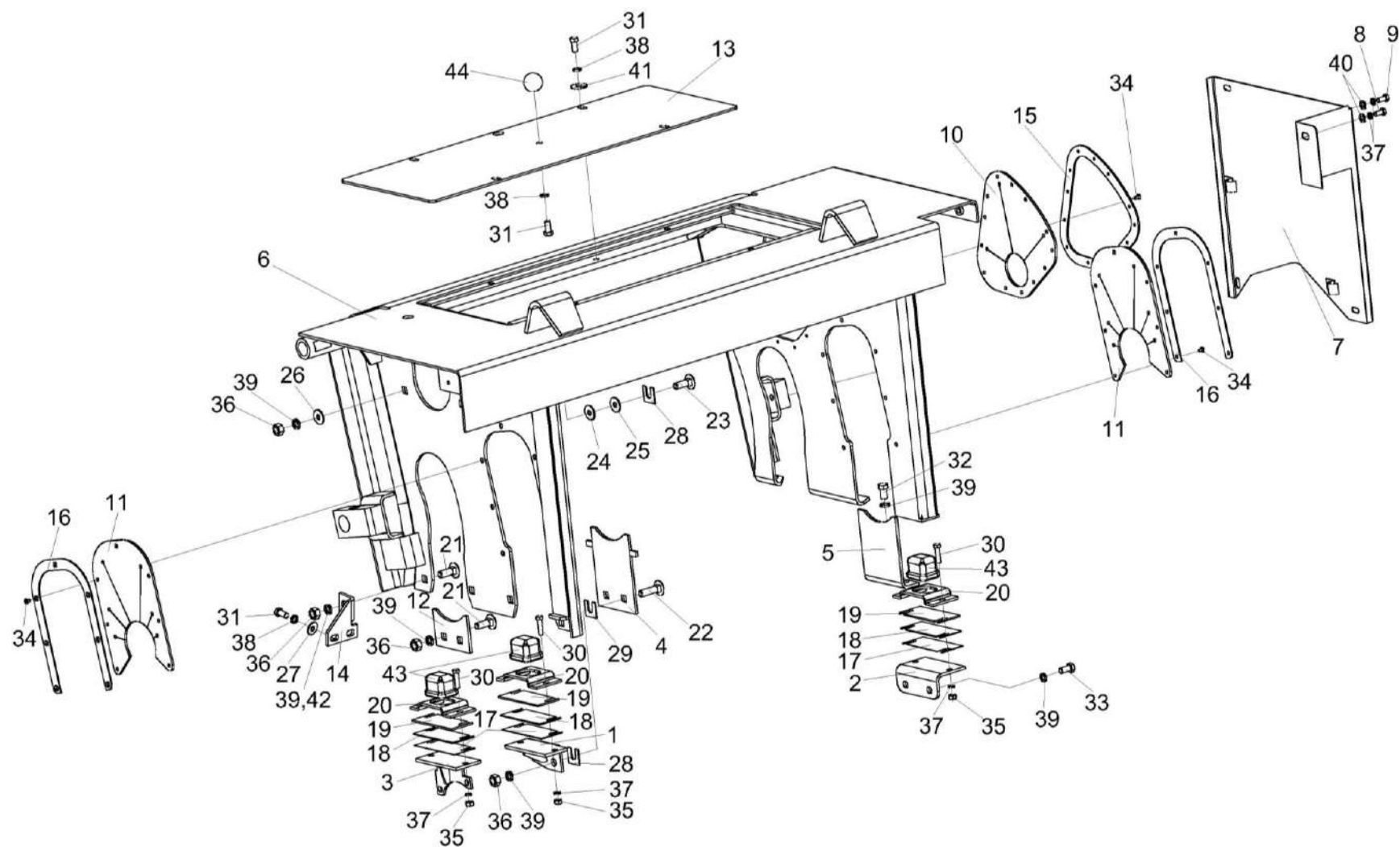
Рисунок 61 – Установка рамы верхней КВС-8-0111300А
