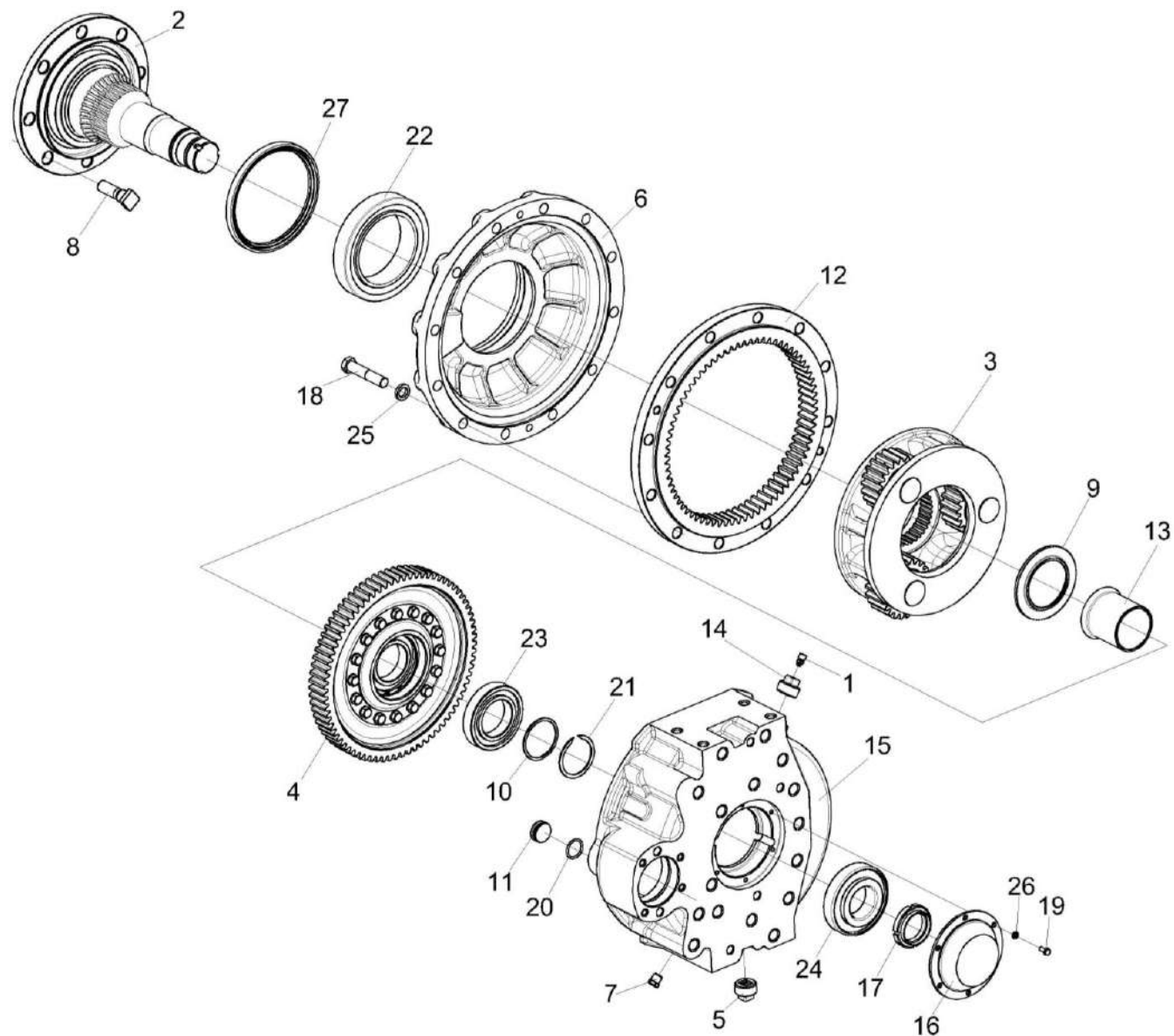
Рисунок 10 – Редуктор бортовой КЗК-400-1-0107020-01 и КЗК-400-1-0107020-02 (лист 1)
