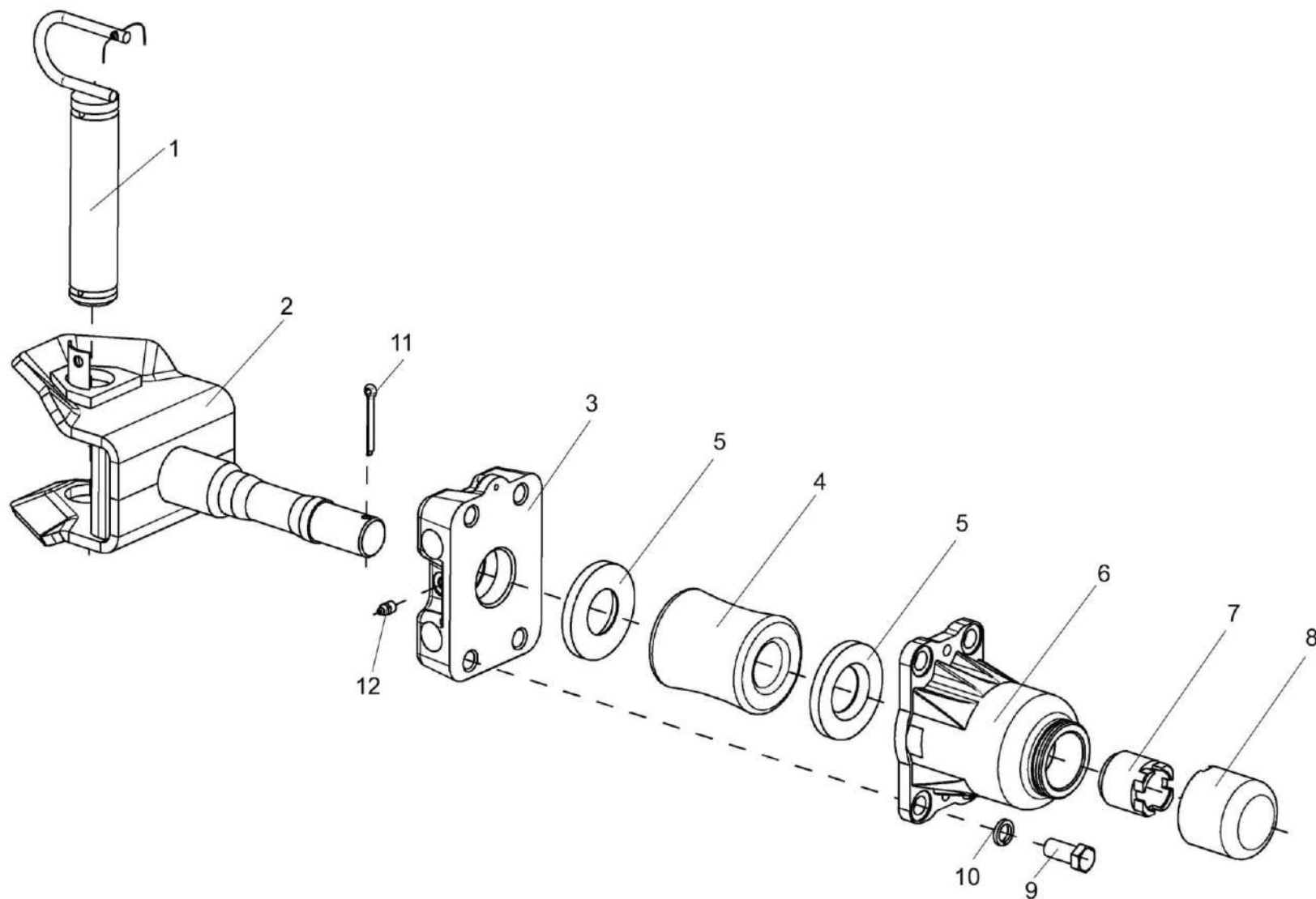
Рисунок 25 – Устройство тягово-сцепное УЭС 0003150
