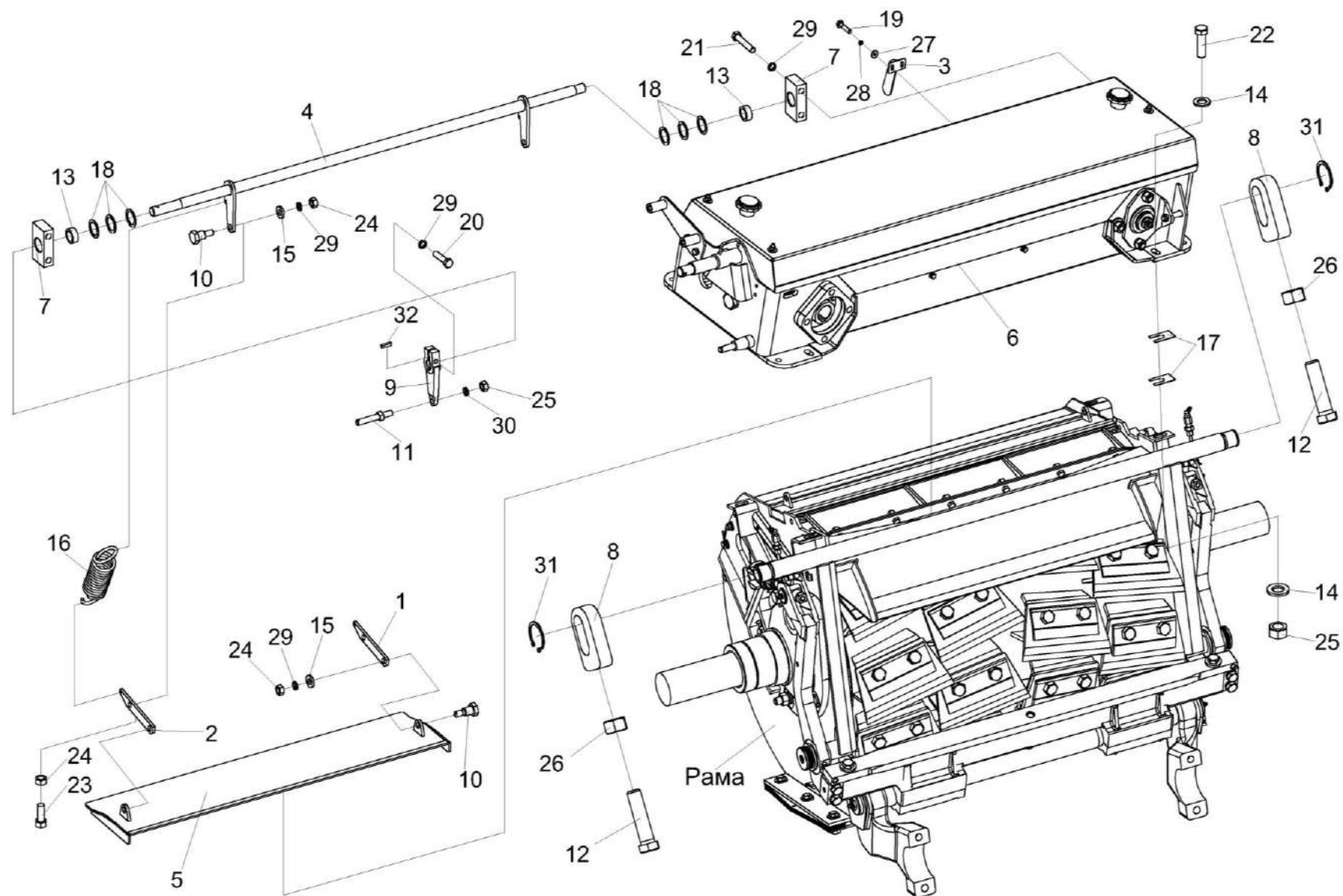
Рисунок 80 – Аппарат измельчающий КВС-8-0115000-01
