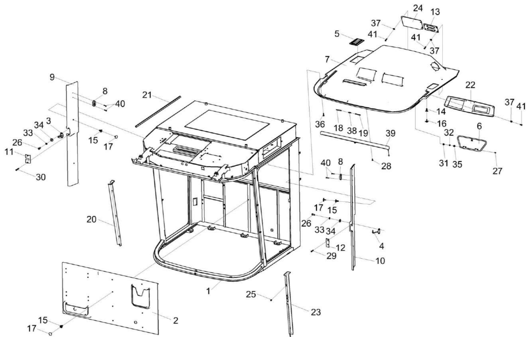
Рисунок 166 – Кабина КВС-80-8-0120010 (лист 3)
