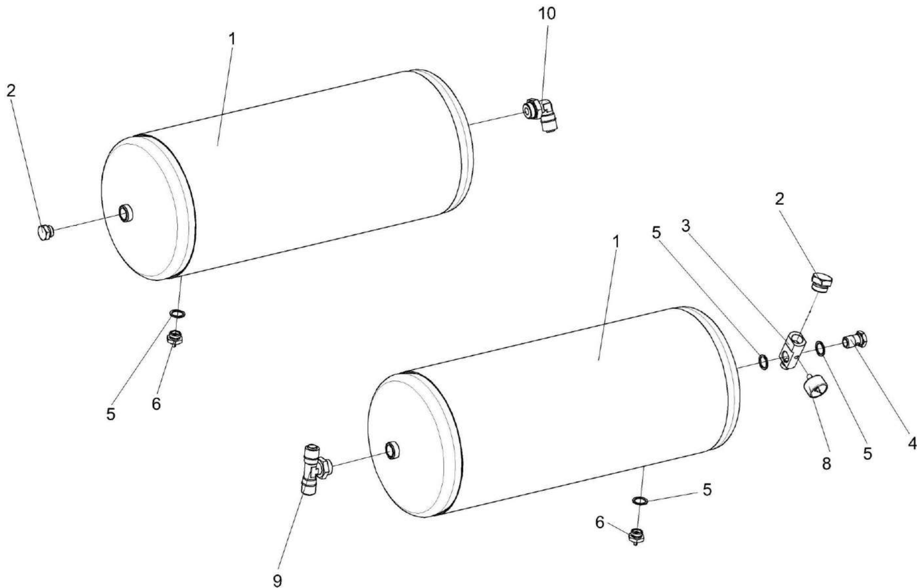
Рисунок 241 – Ресивер КВС-5-0800030 и КВС-5-0800050
