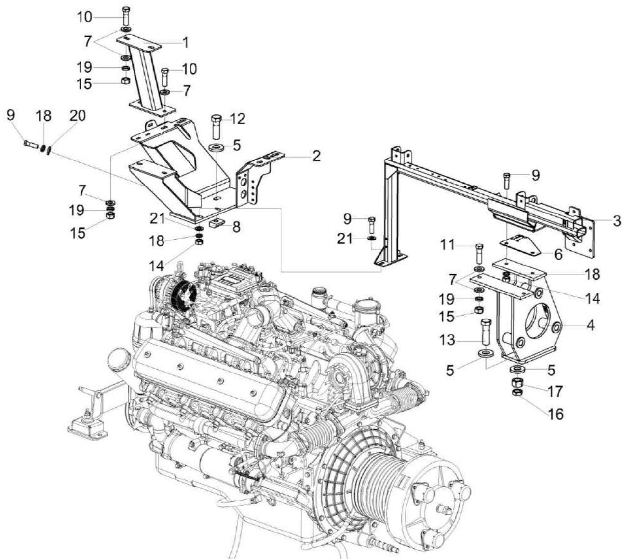
Рисунок 31 – Установка двигателя КВС-80-7-0150000 (лист 4)
