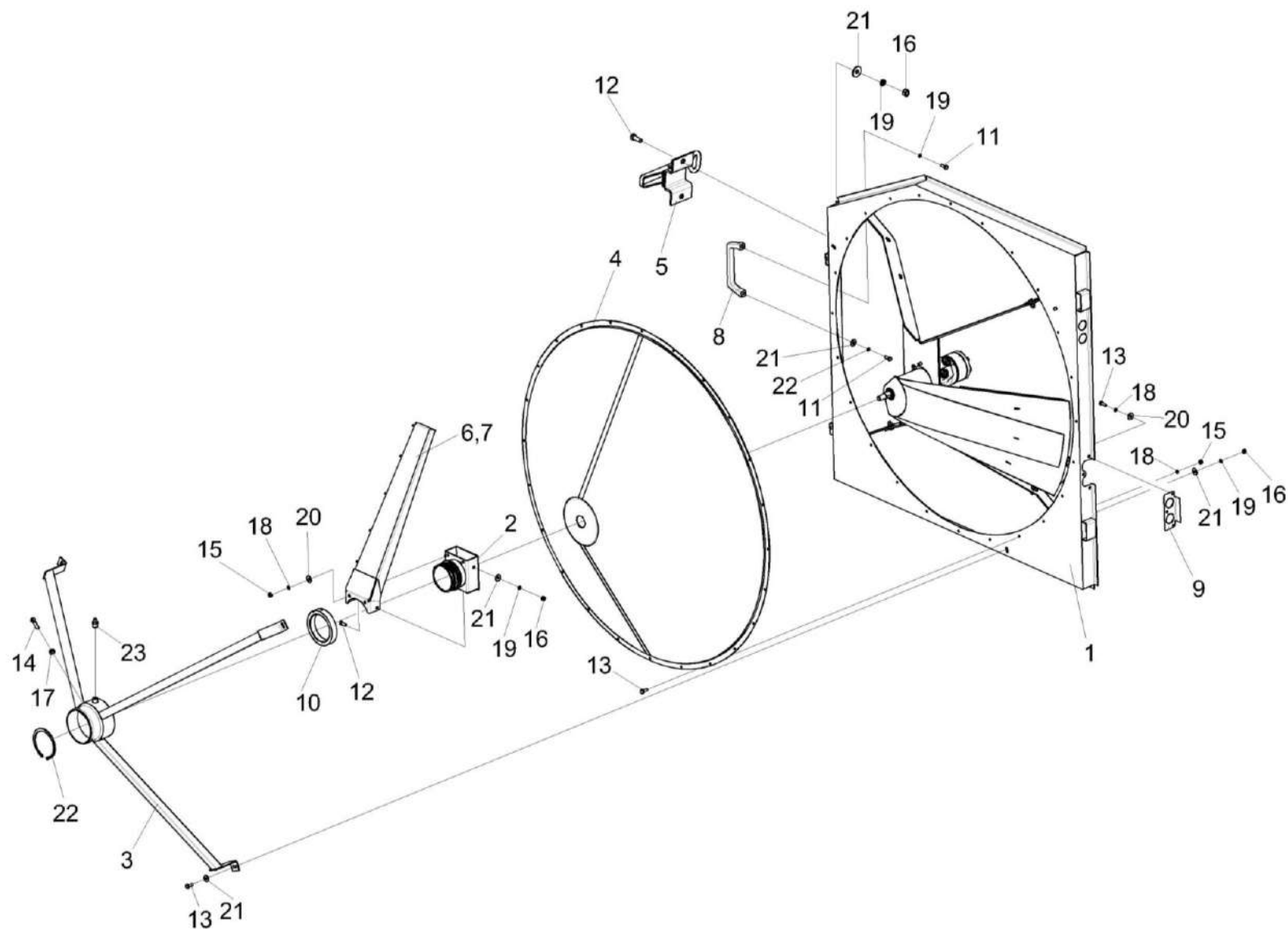
Рисунок 46 – Воздухозаборник КВС-5-0155000А (лист 1)
