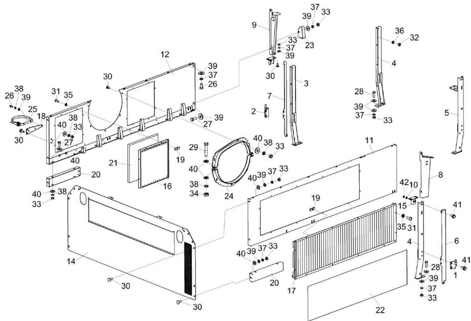
Рисунок 185 – Установка крыши КВС-80-8-0162000-01 (лист 1)
