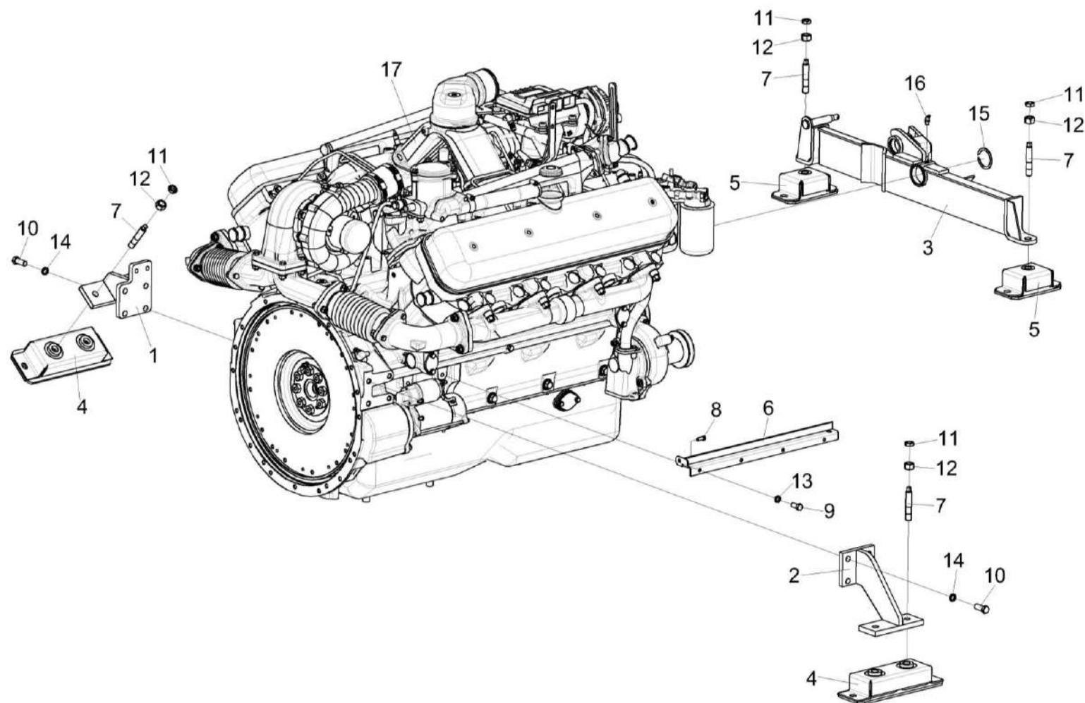
Рисунок 34 – Двигатель КВС-80-7-0150010 (лист 3)
