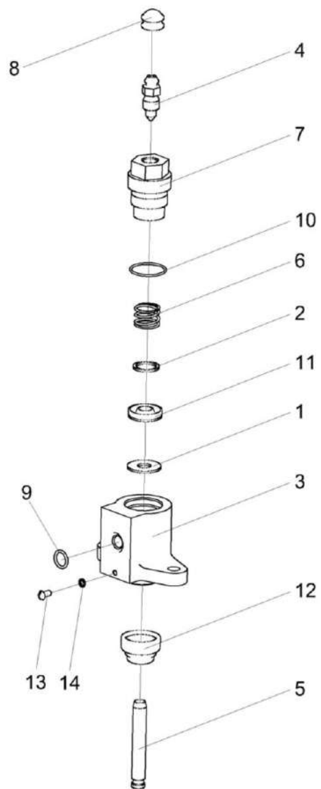
Рисунок 20 – Гидроцилиндр КЗК-12-0107200-01
