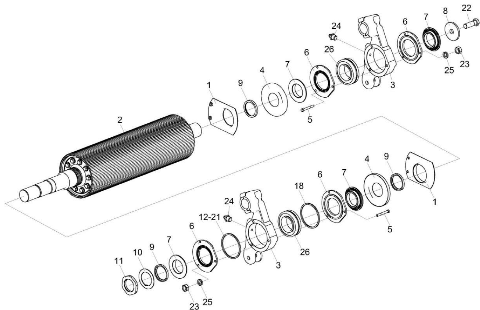
Рисунок 117 – Валец нижний КВС-80-8-0148210
