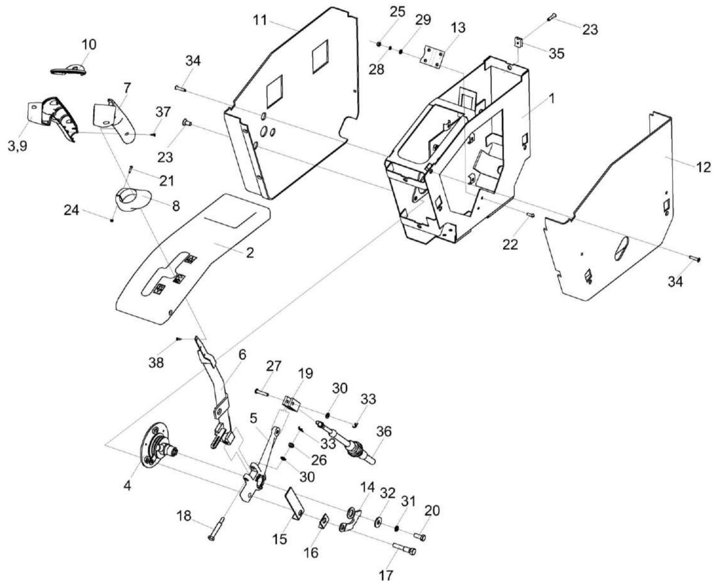
Рисунок 143 – Пульт управления КВС-80-8-0119890
