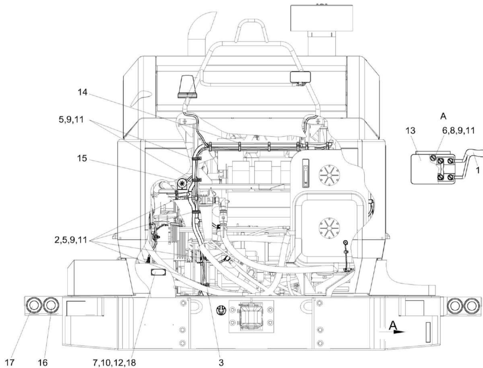
Рисунок 248 – Установка электрооборудования КВС-80-7-0721000 (лист 3)
