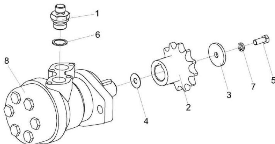
Рисунок 88 – Гидромотор заточного устройства КВС-2-0116680-01
