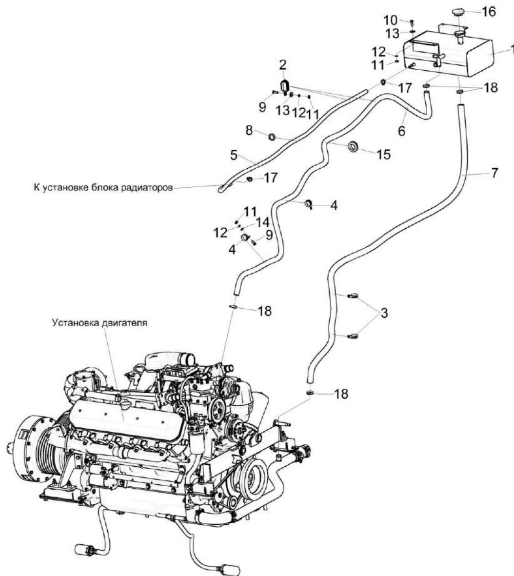
Рисунок 49 – Установка бачка расширительного КВС-7-0154000
