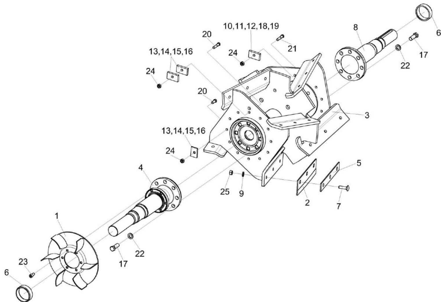
Рисунок 130 – Вал ускорителя выброса КВС-1-0142910А
