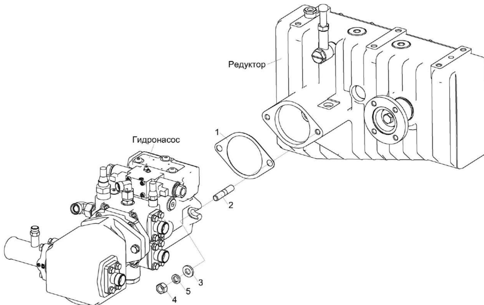
Рисунок 97 – Установка гидронасоса КВС-80-8-0138000
