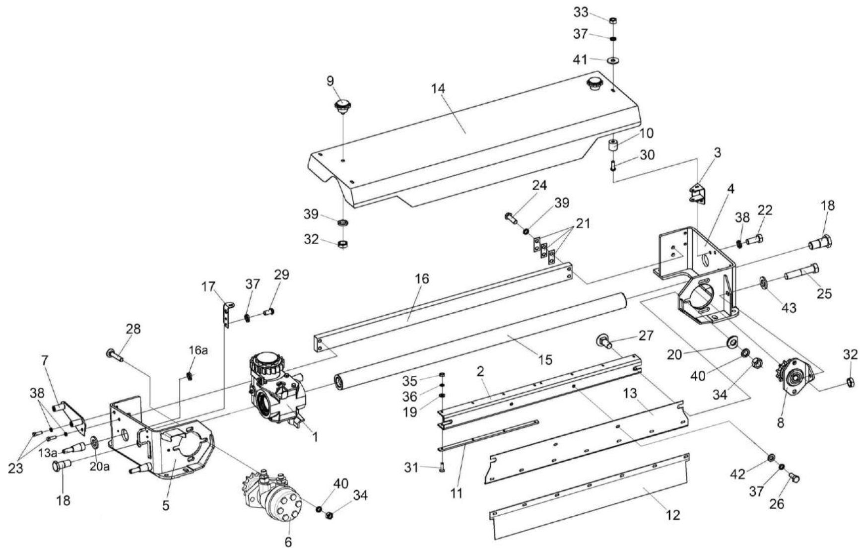
Рисунок 84 – Устройство заточное КВС-2-0116600А
