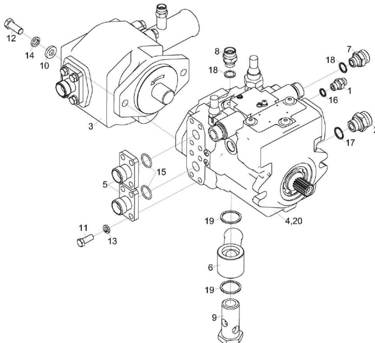
Рисунок 236 – Гидронасос двухсекционный КВС-5-0624340
