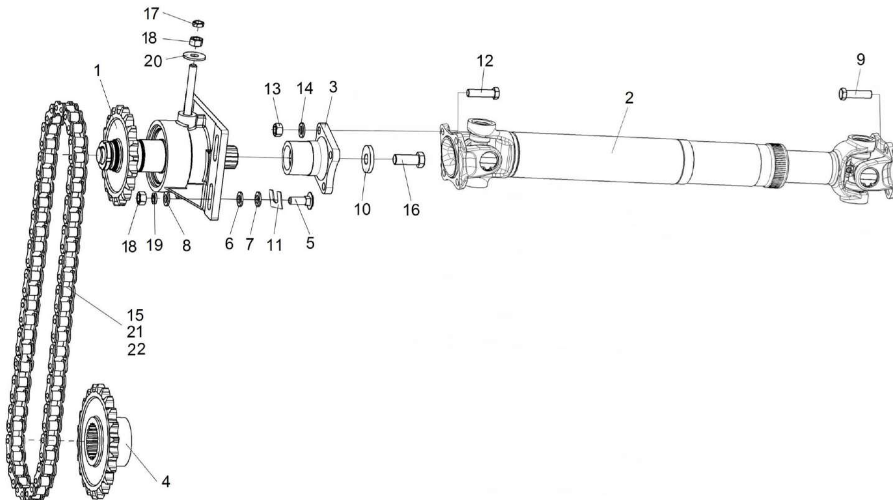
Рисунок 62 – Установка вала карданного КВС-1-0119000-01
