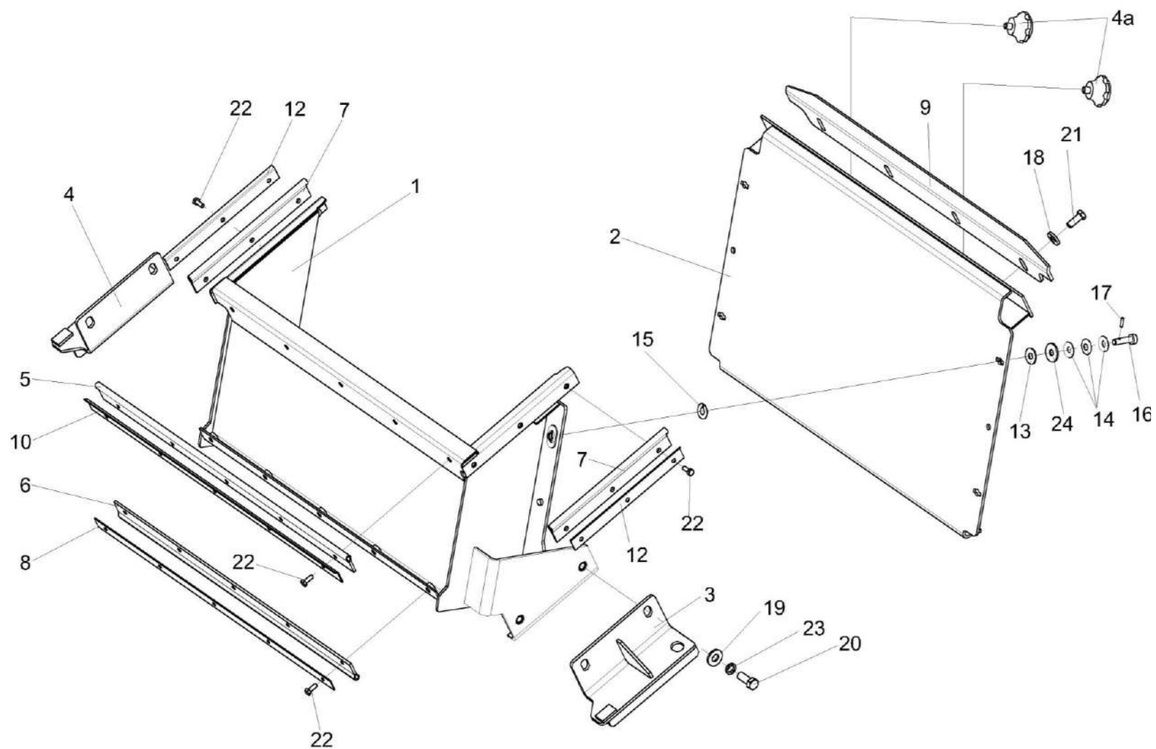
Рисунок 134 – Проставка КВС-1-0147500
