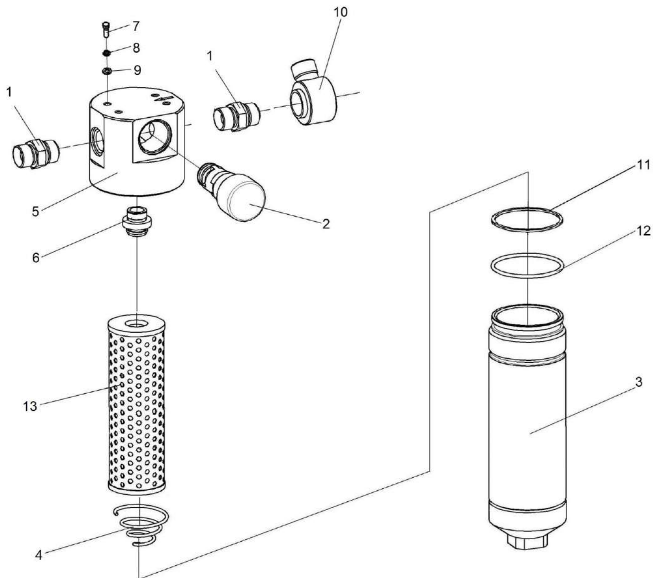
Рисунок 213 – Фильтр напорный КВС-5-0602360
