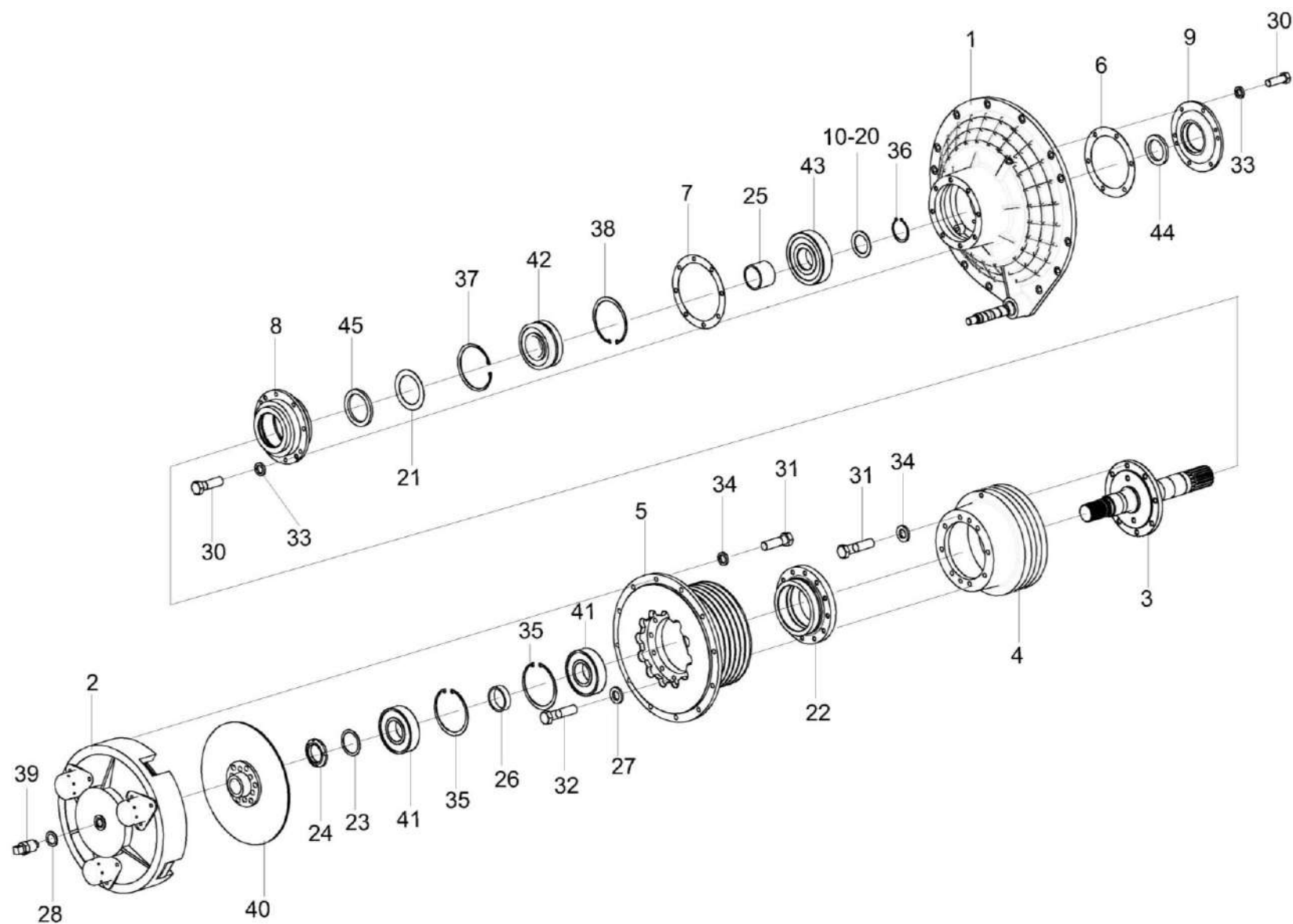
Рисунок 36 – Главный привод КВС-7-0151000
