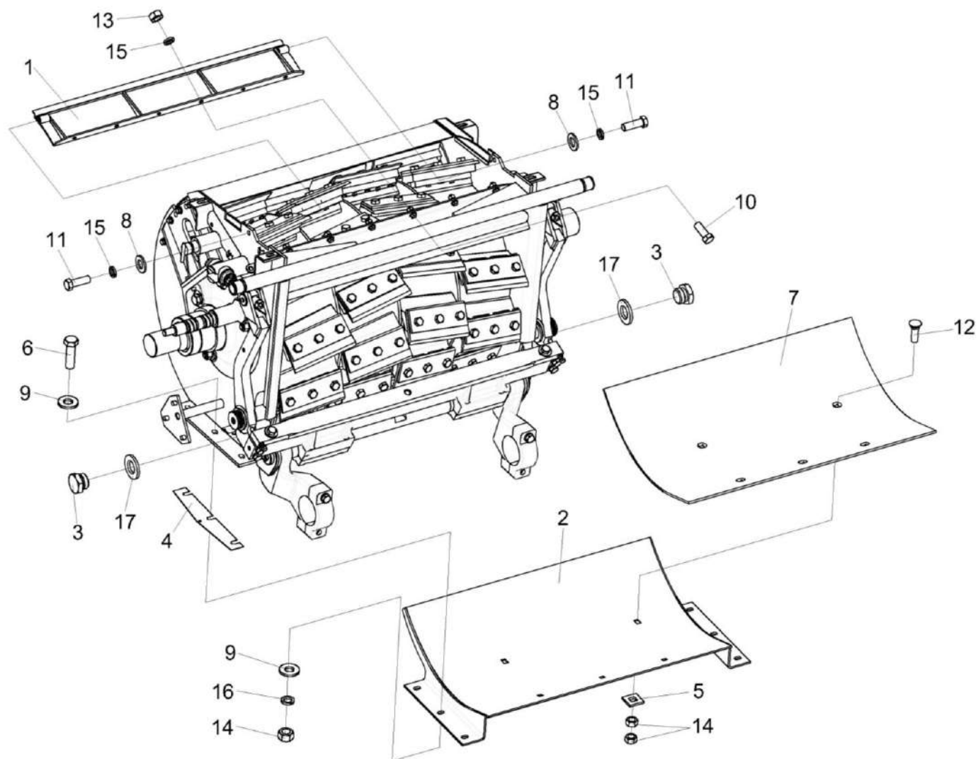
Рисунок 81 – Установка поддона КВС-2-0115050
