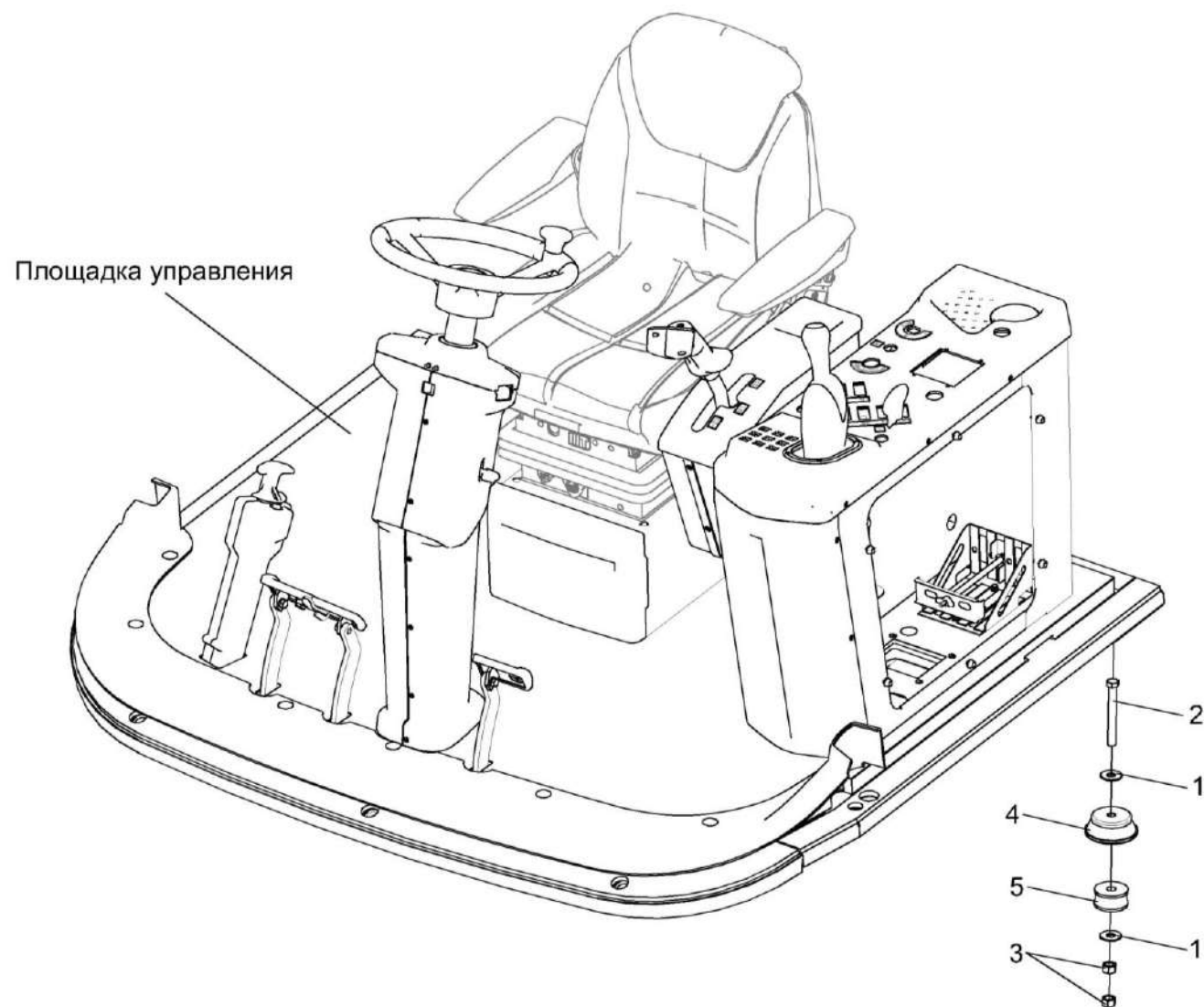
Рисунок 139 – Установка площадки управления КВС-80-8-0119200
