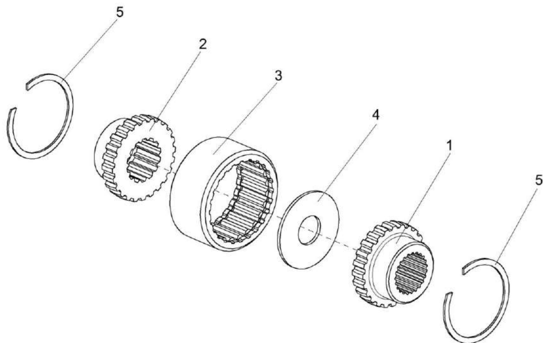
Рисунок 74 – Муфта КГС 0100120
