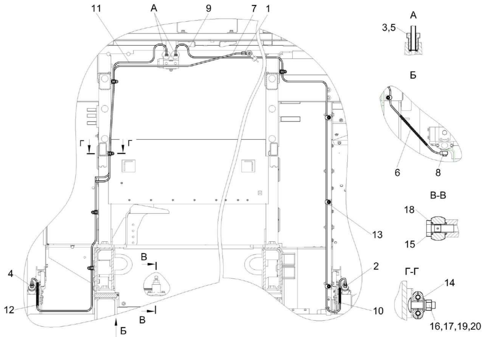
Рисунок 159 – Установка трубопроводов КВС-80-8-0119630
