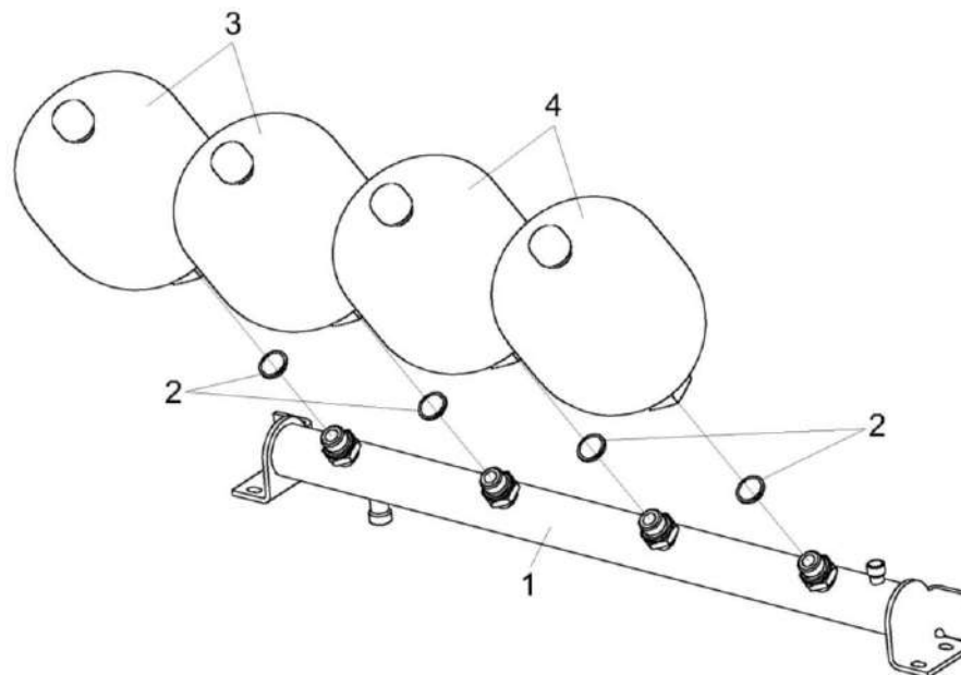
Рисунок 216 – Блок пневмогидроаккумуляторов КВС-8-0602830
