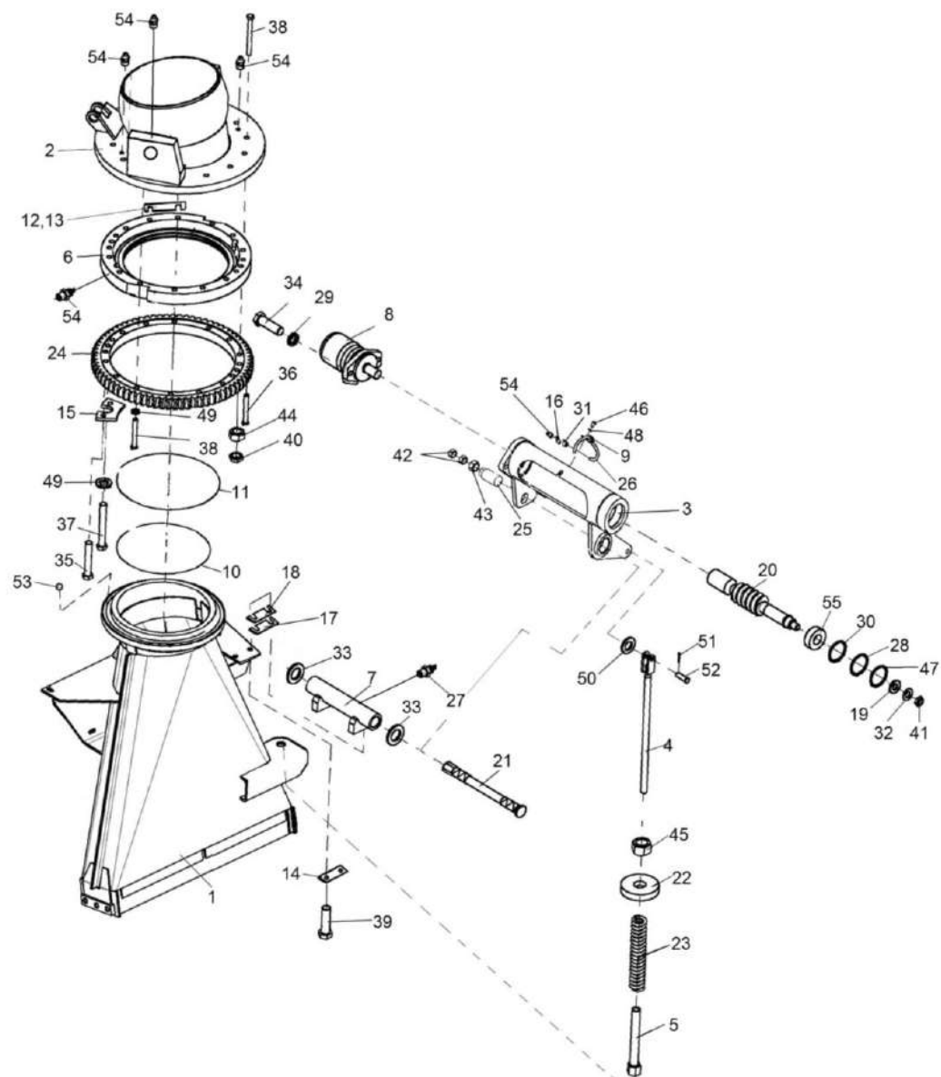
Рисунок 132 – Основание силосопровода и механизм поворота КВС-1-0143500
