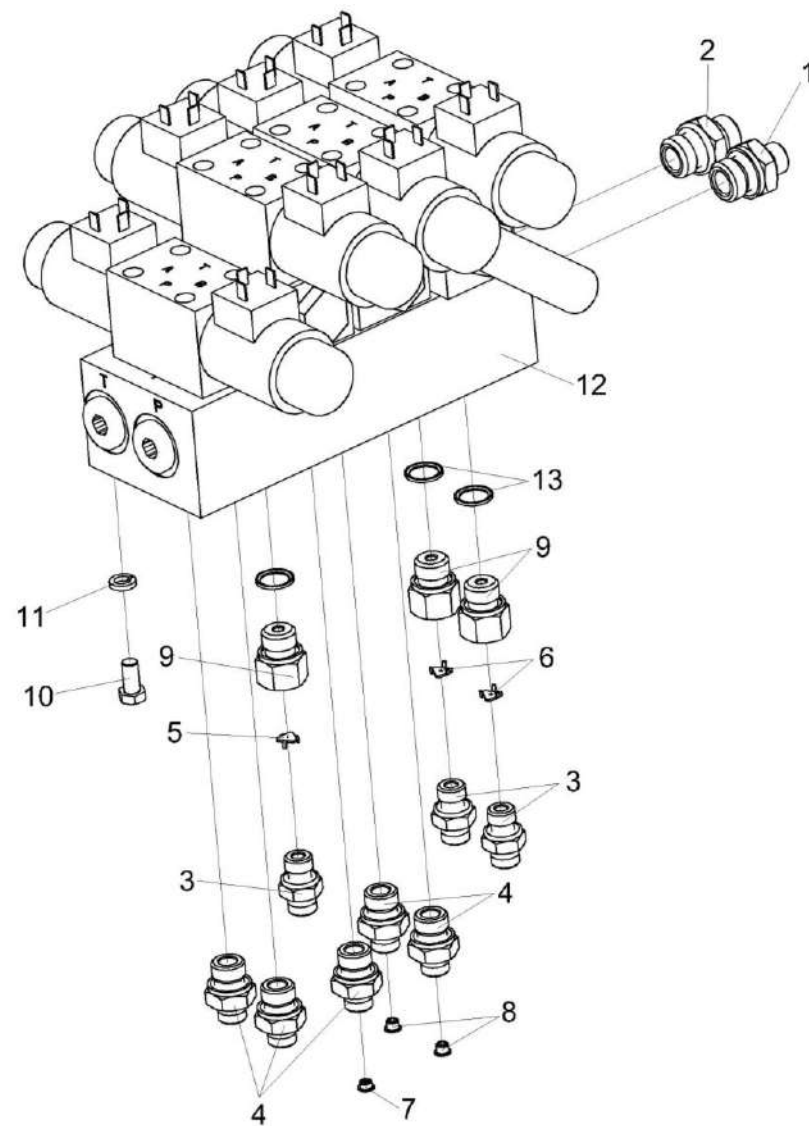
Рисунок 218 – Гидроблок КВС-8-0602310
