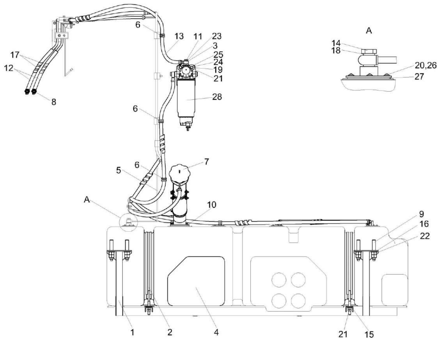
Рисунок 200 – Установка топливного оборудования КВС-7-0103700 (лист 1)
