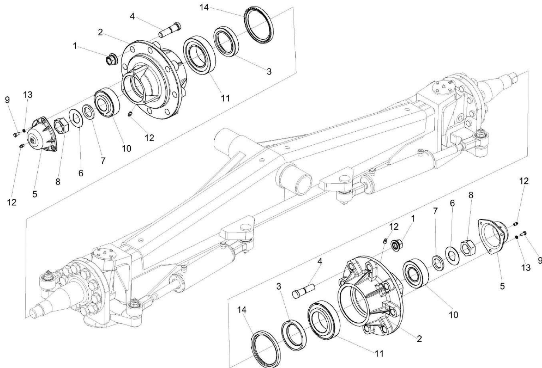
Рисунок 22 – Мост управляемых колес КВС-2-0109000 (установка ступиц)
