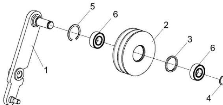
Рисунок 41 – Рычаг КВС-7-0150120
