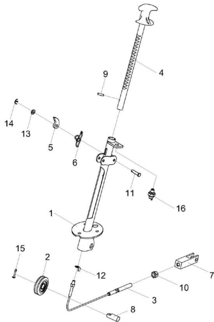
Рисунок 150 – Колонка привода КВС-80-8-0119750
