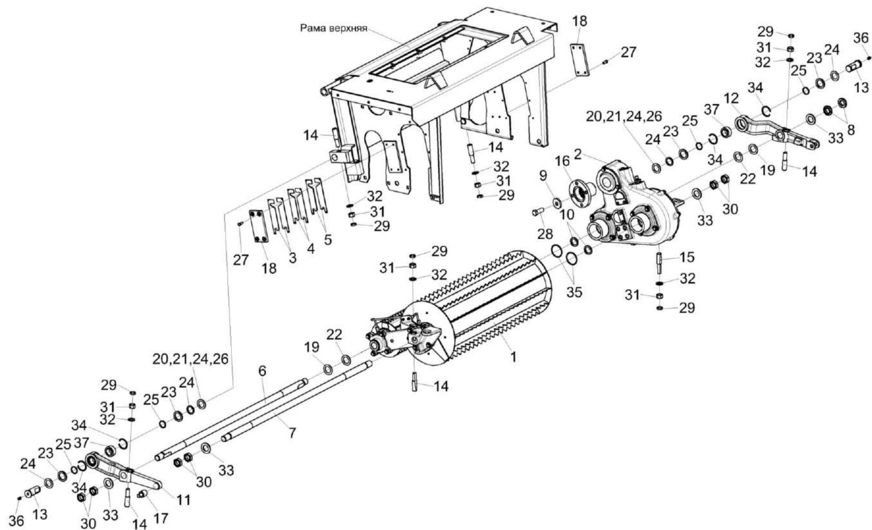
Рисунок 76 – Установка вальцев КВС-8-0111010
