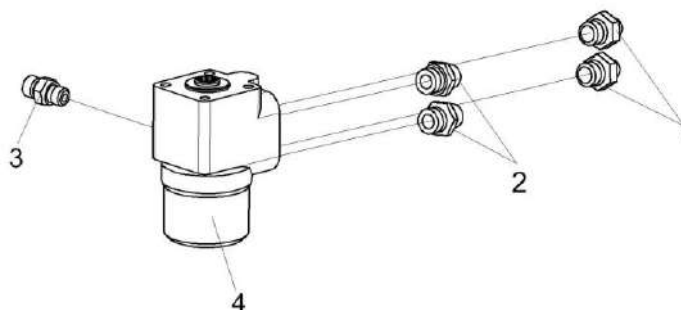
Рисунок 223 – Установка насоса-дозатора КВС-1-0602990
