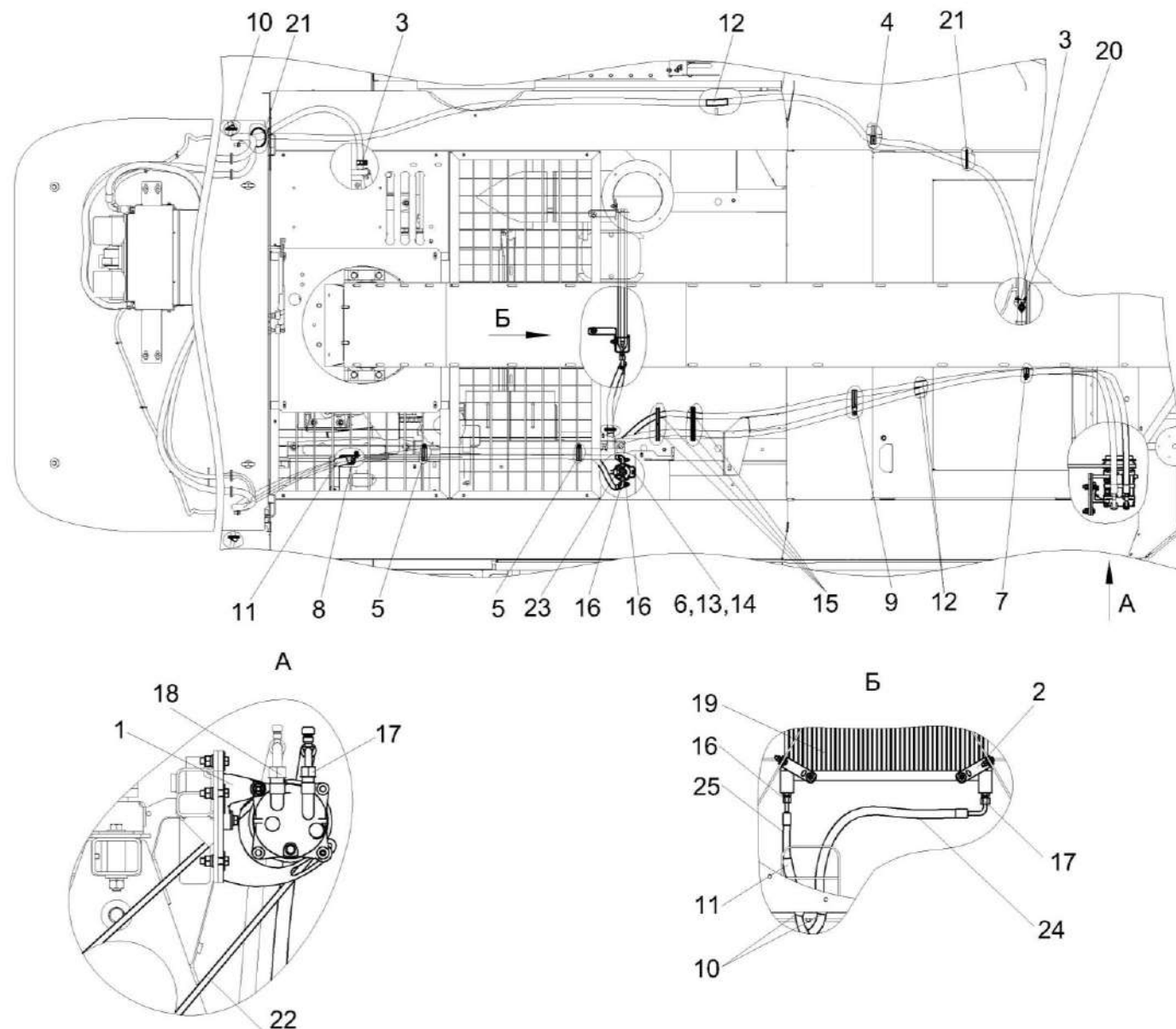
Рисунок 174 – Установка оборудования кондиционера КВС-80-7-0121010 и КВС-80-7-0121010-01
