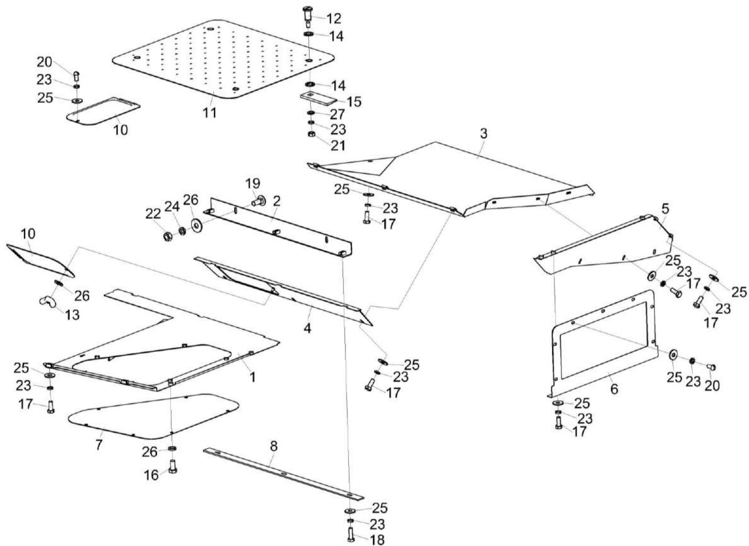
Рисунок 194 – Установка ограждений КВС-80-8-0100100 (лист 3)
