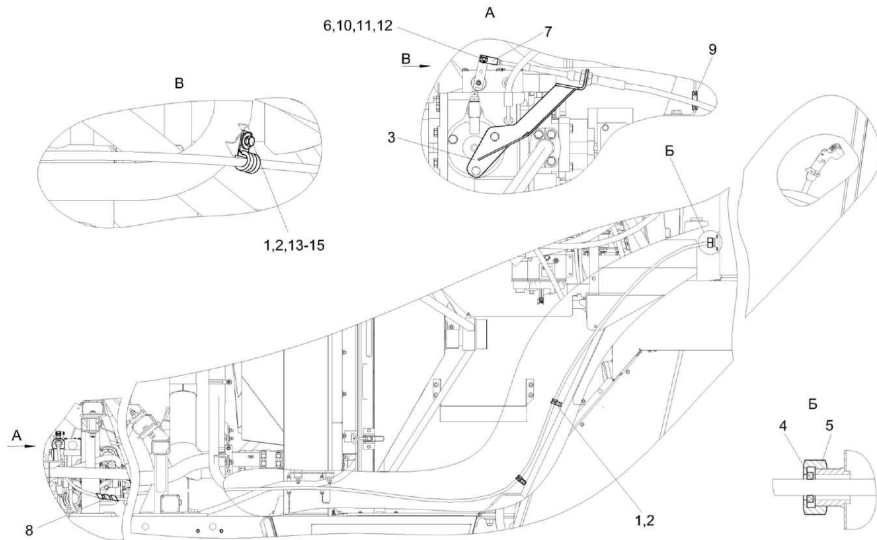
Рисунок 158 – Установка троса ГСТ КВС-80-8-0119620-01
