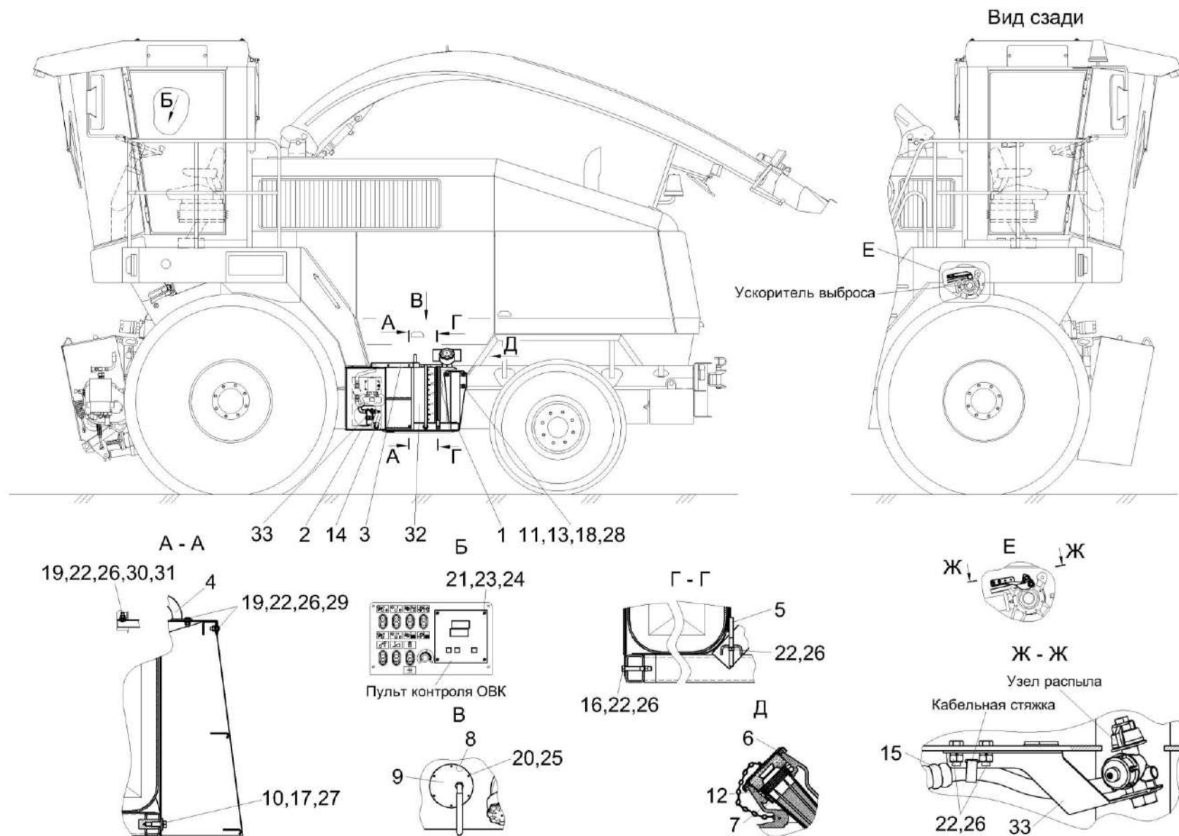
Рисунок 258 – Установка ОВК КВС-2-0900000А-01
