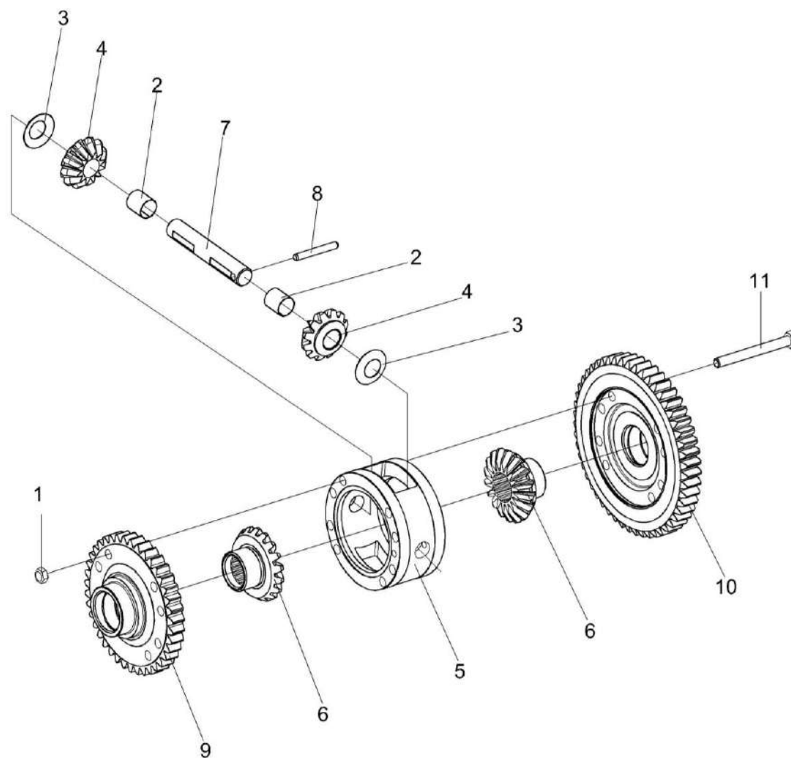
Рисунок 18 – Дифференциал КЗК-8-0107540
