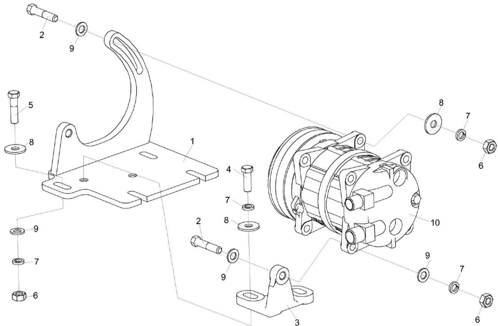
Рисунок 175 – Установка компрессора КВС-8-0121120 и КВС-8-0121120-01
