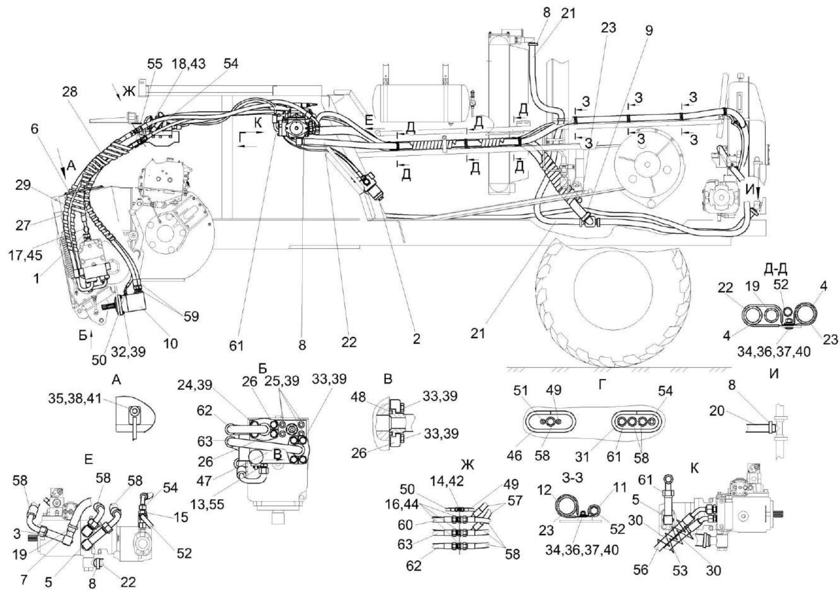
Рисунок 225 – Гидросистема привода питающего аппарата и адаптеров КВС-5-0604000 (лист 1)
