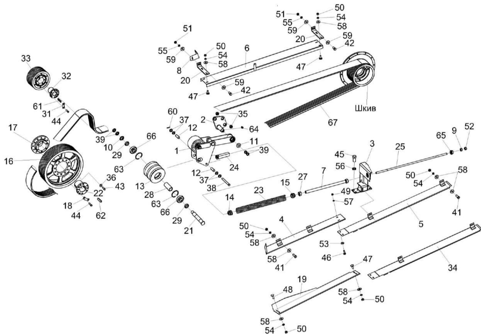
Рисунок 98 – Привод измельчающего барабана КВС-5-0130500-01
