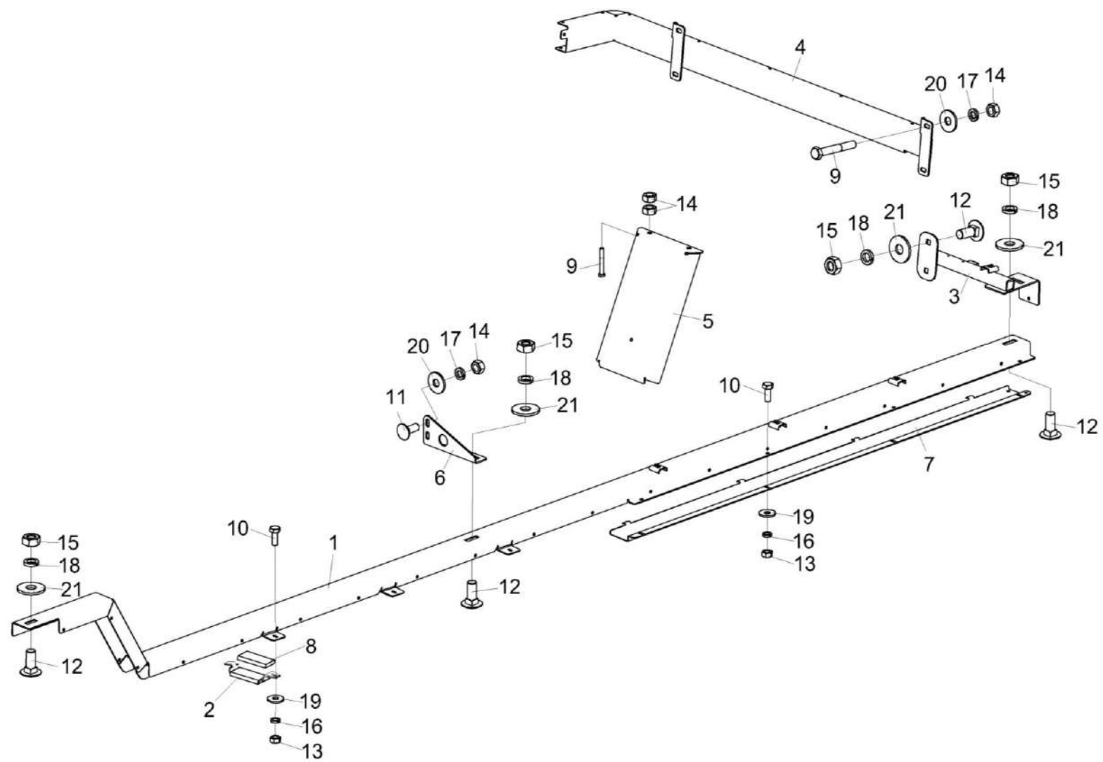
Рисунок 199 – Установка желобов КВС-80-5-0100200
