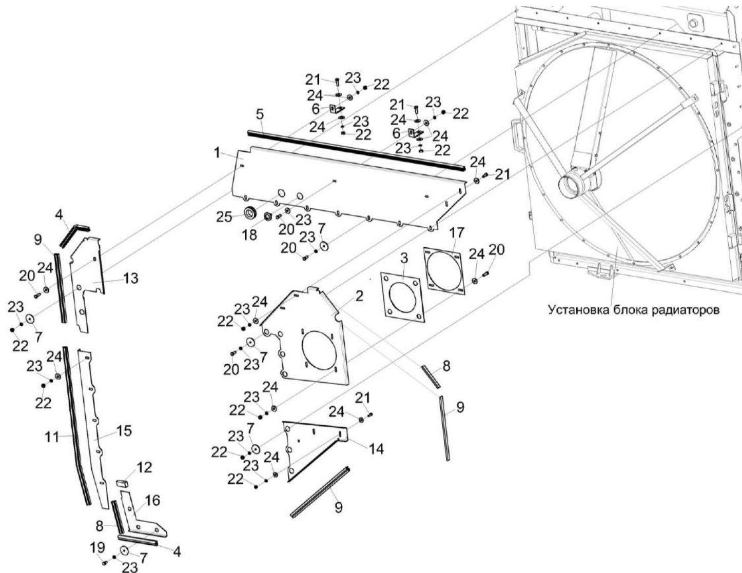
Рисунок 50 – Установка щитов КВС-80-7-0156000
