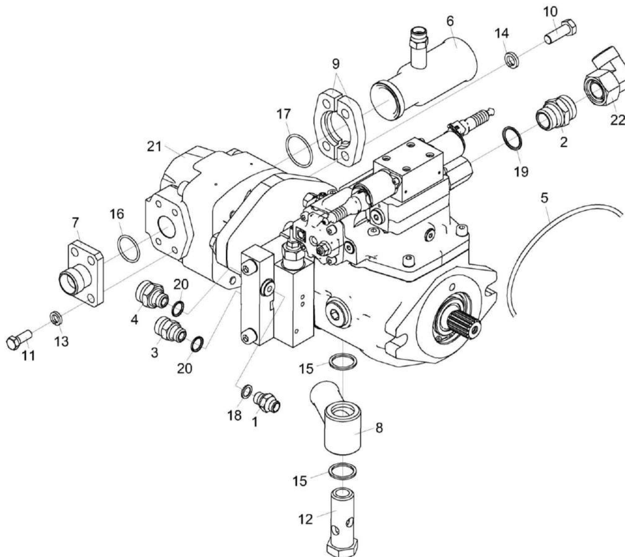
Рисунок 234 – Гидронасос двухсекционный КВС-5-0604330
