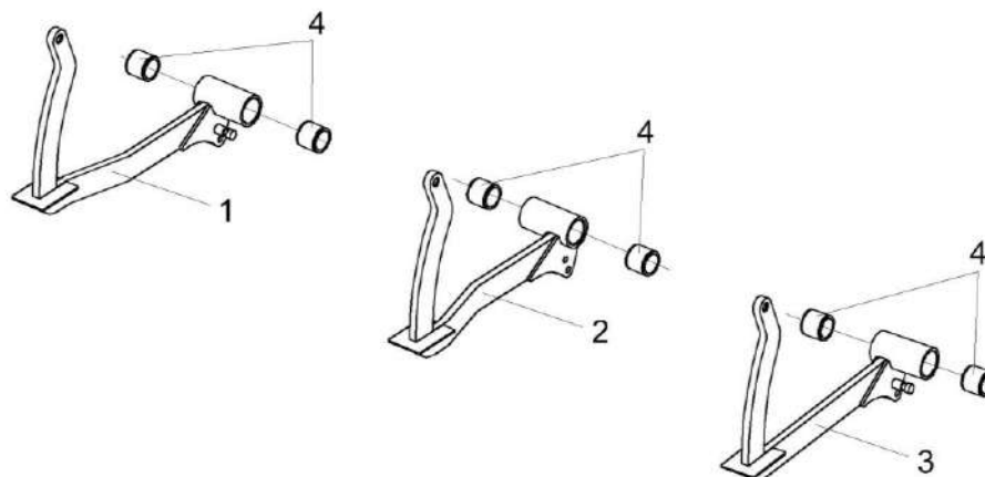
Рисунок 145 – Рычаги КВС-80-8-0119440, КВС-80-8-0119440-01 и КВС-80-8-0119440-02
