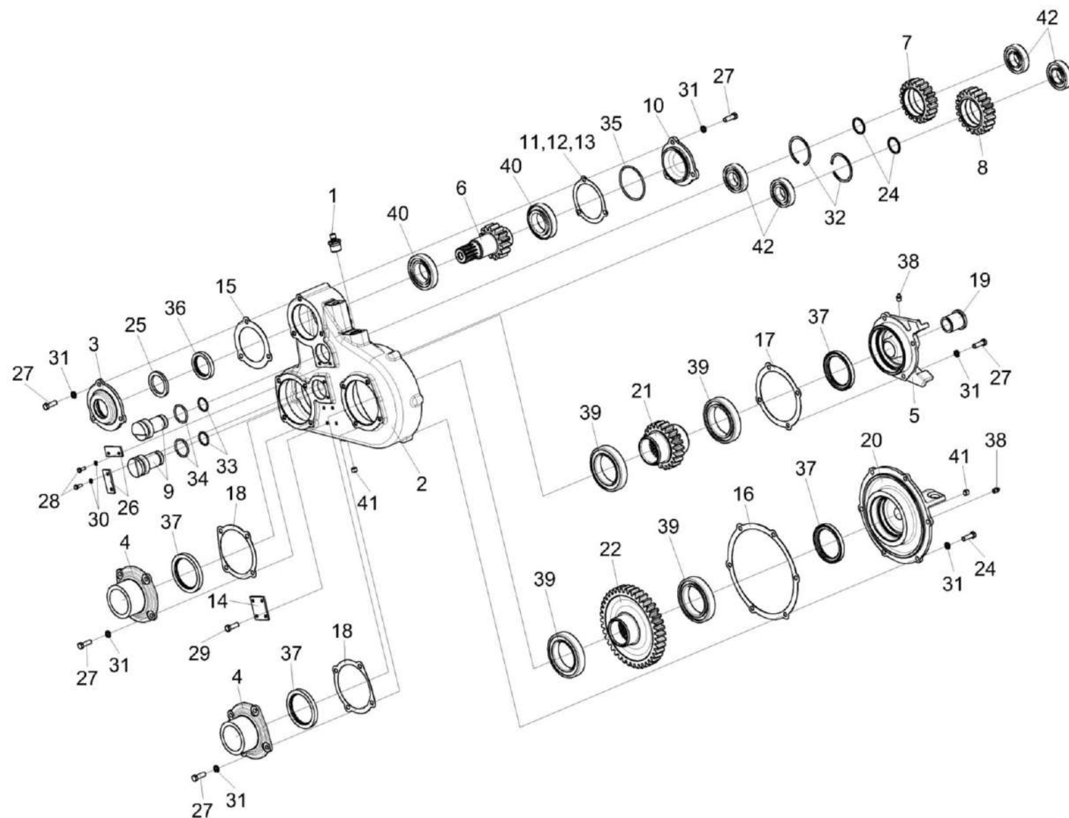
Рисунок 79 – Редуктор верхних вальцев КВС-2-0112000Б
