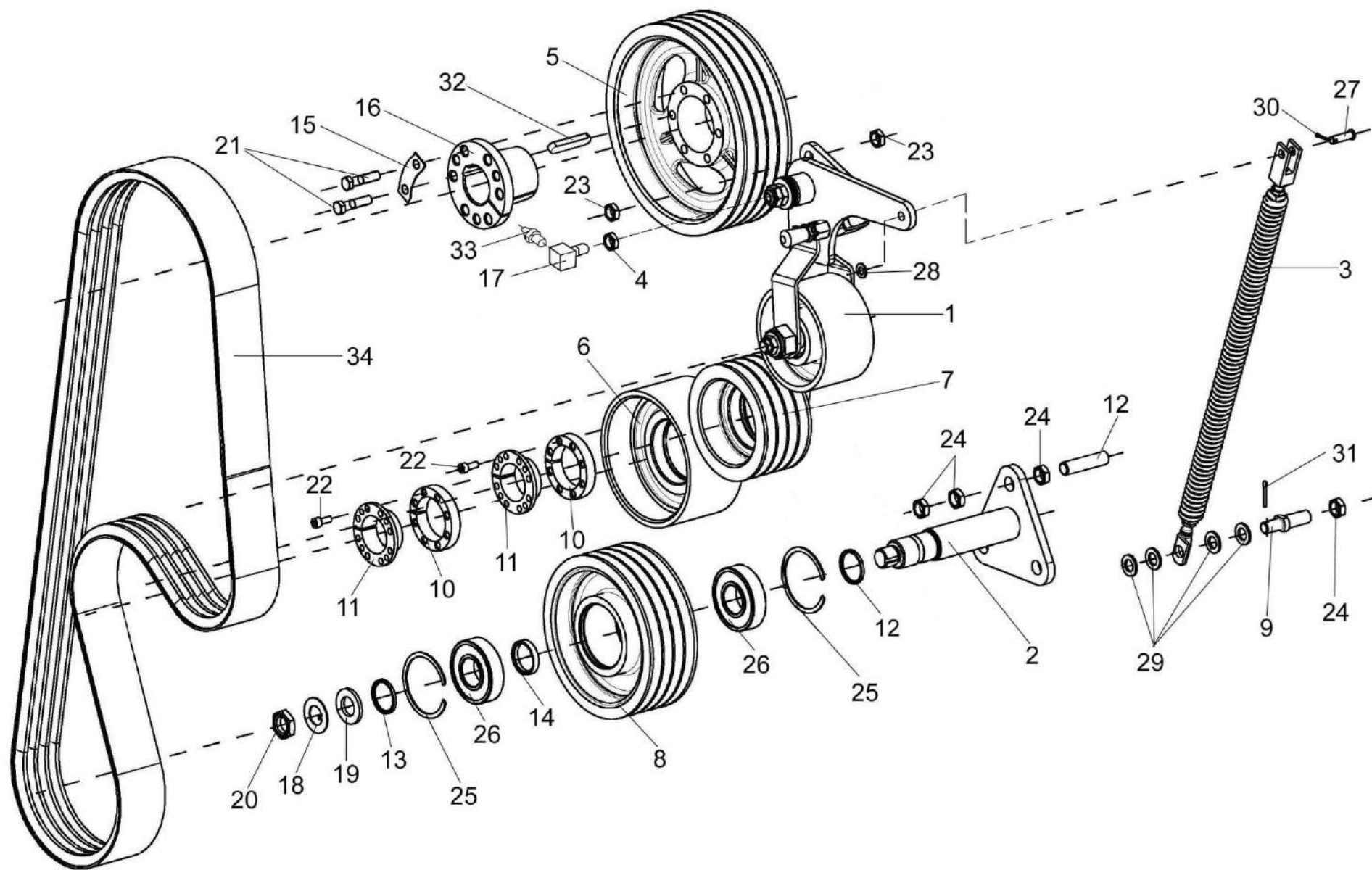
Рисунок 103 – Привод доизмельчающего устройства КВС-80-8-0132000
