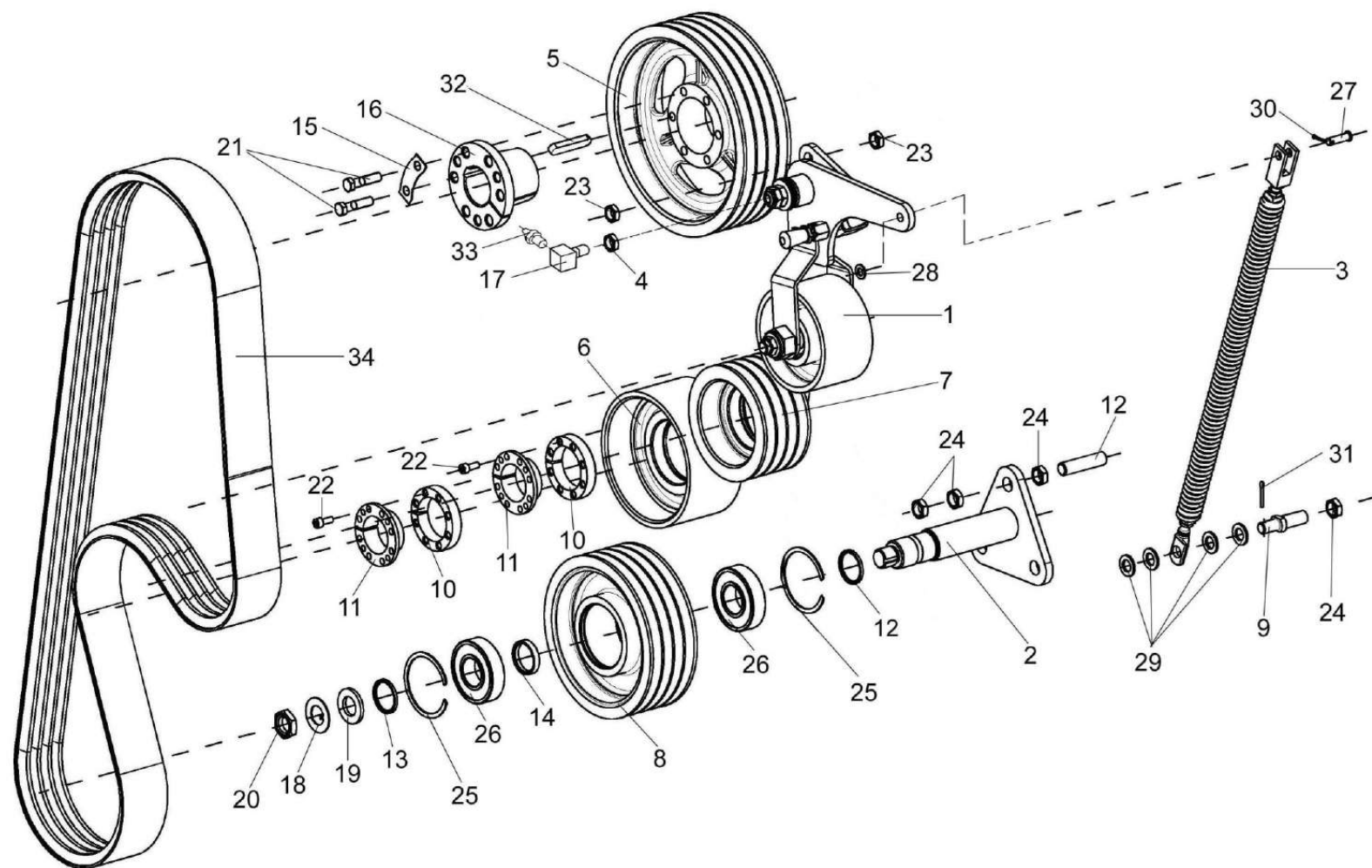
Рисунок 101 – Привод доизмельчающего устройства КВС-1-0132100
