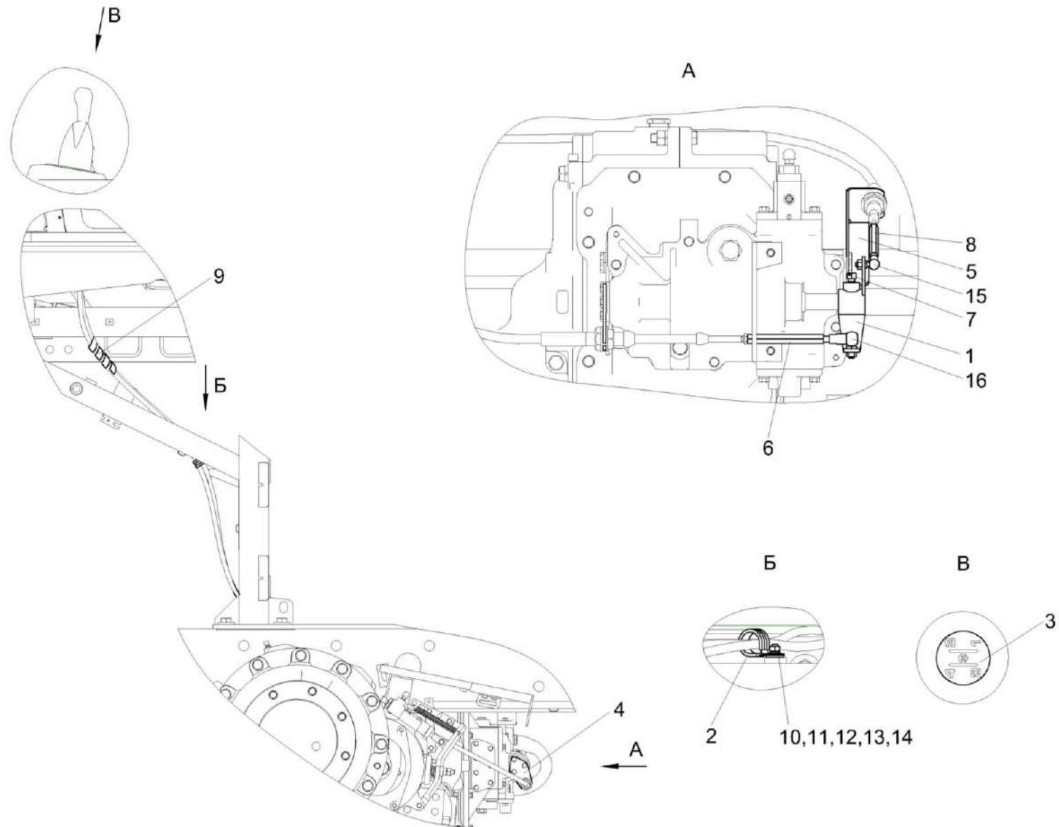
Рисунок 160 – Установка механизма переключения передач КВС-80-8-0119650
