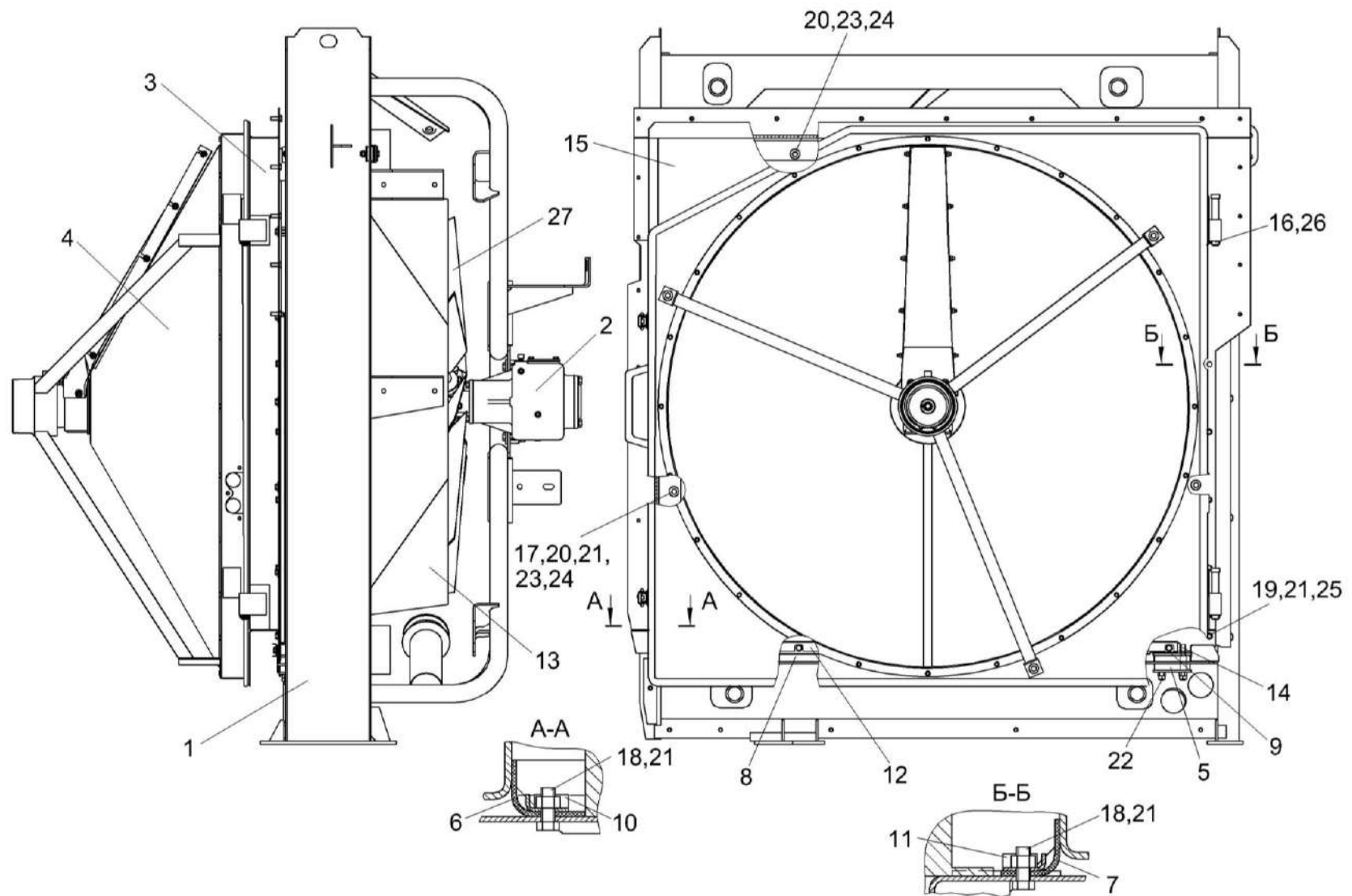
Рисунок 42 – Установка блока радиаторов КВС-7-0152000 (лист 1)
