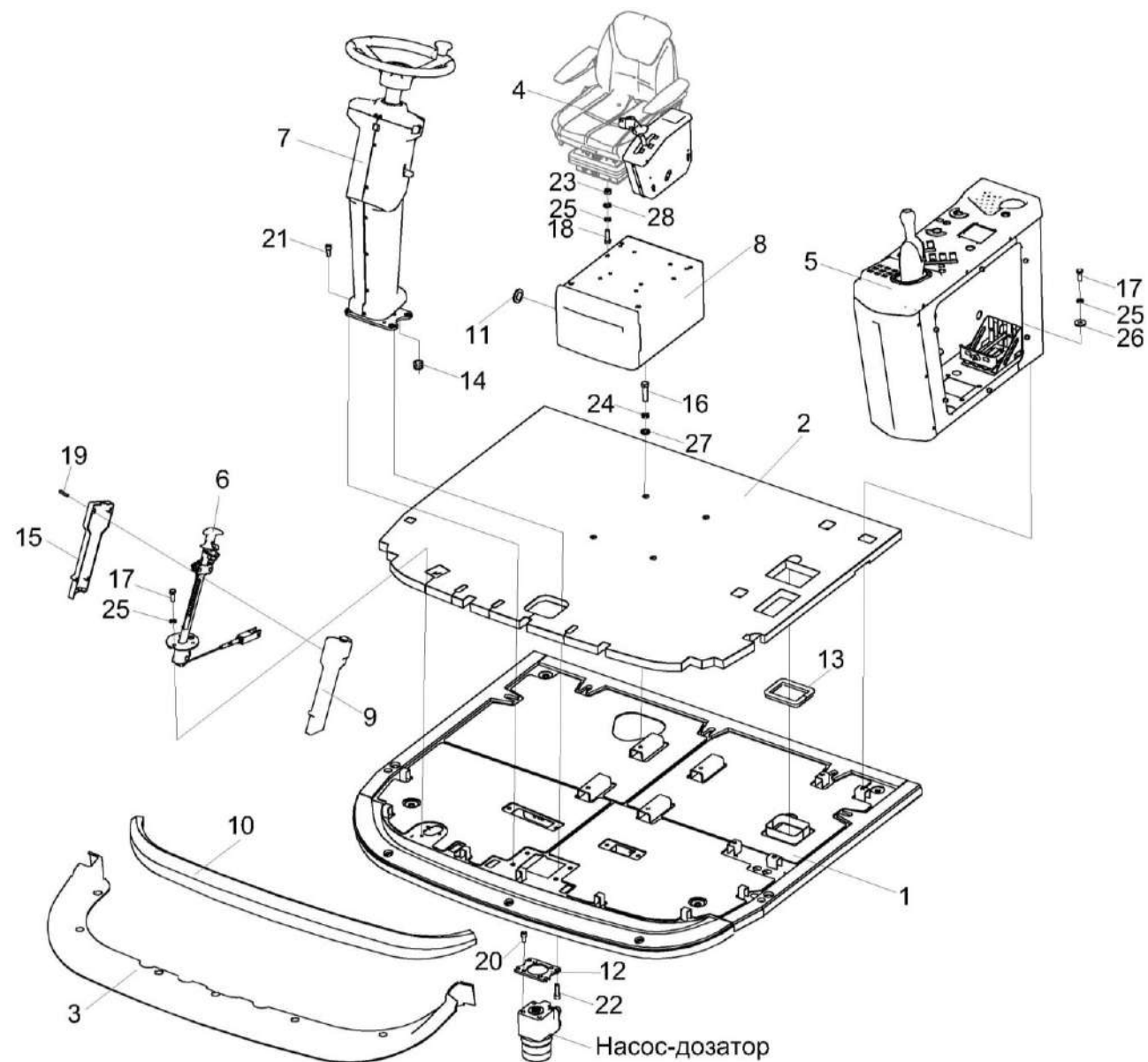
Рисунок 140 – Площадка управления КВС-80-8-0119000 (лист 1)
