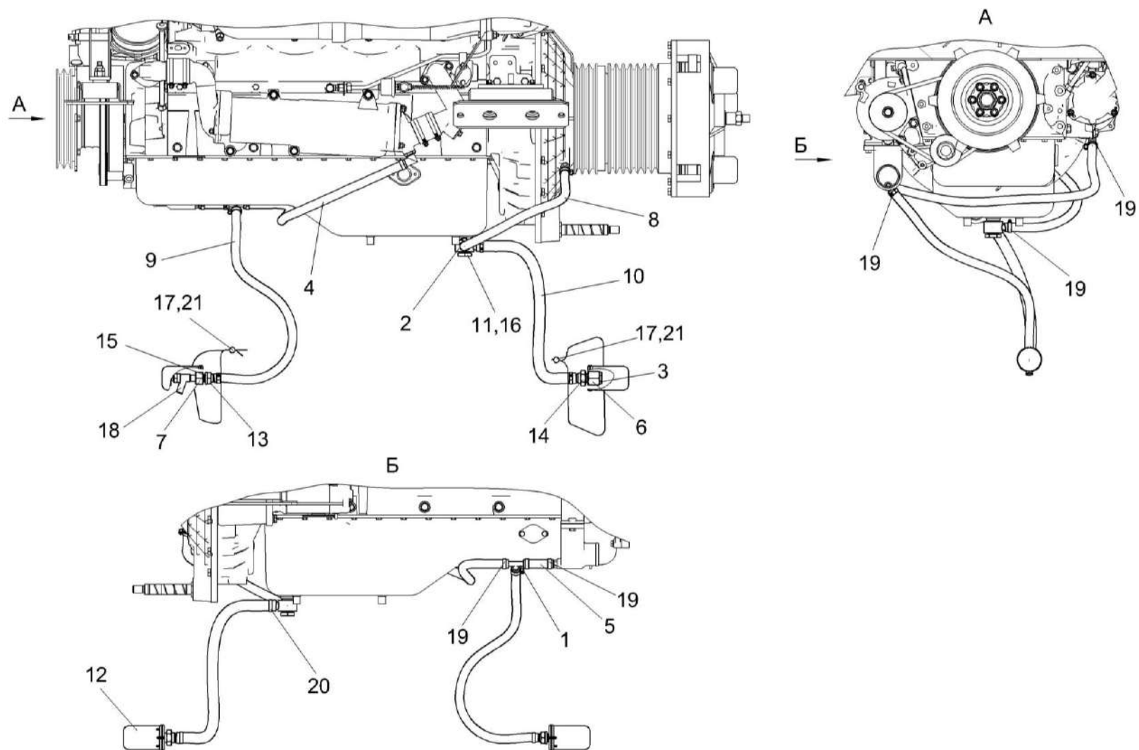
Рисунок 35 – Установка сливных рукавов КВС-7-0150260
