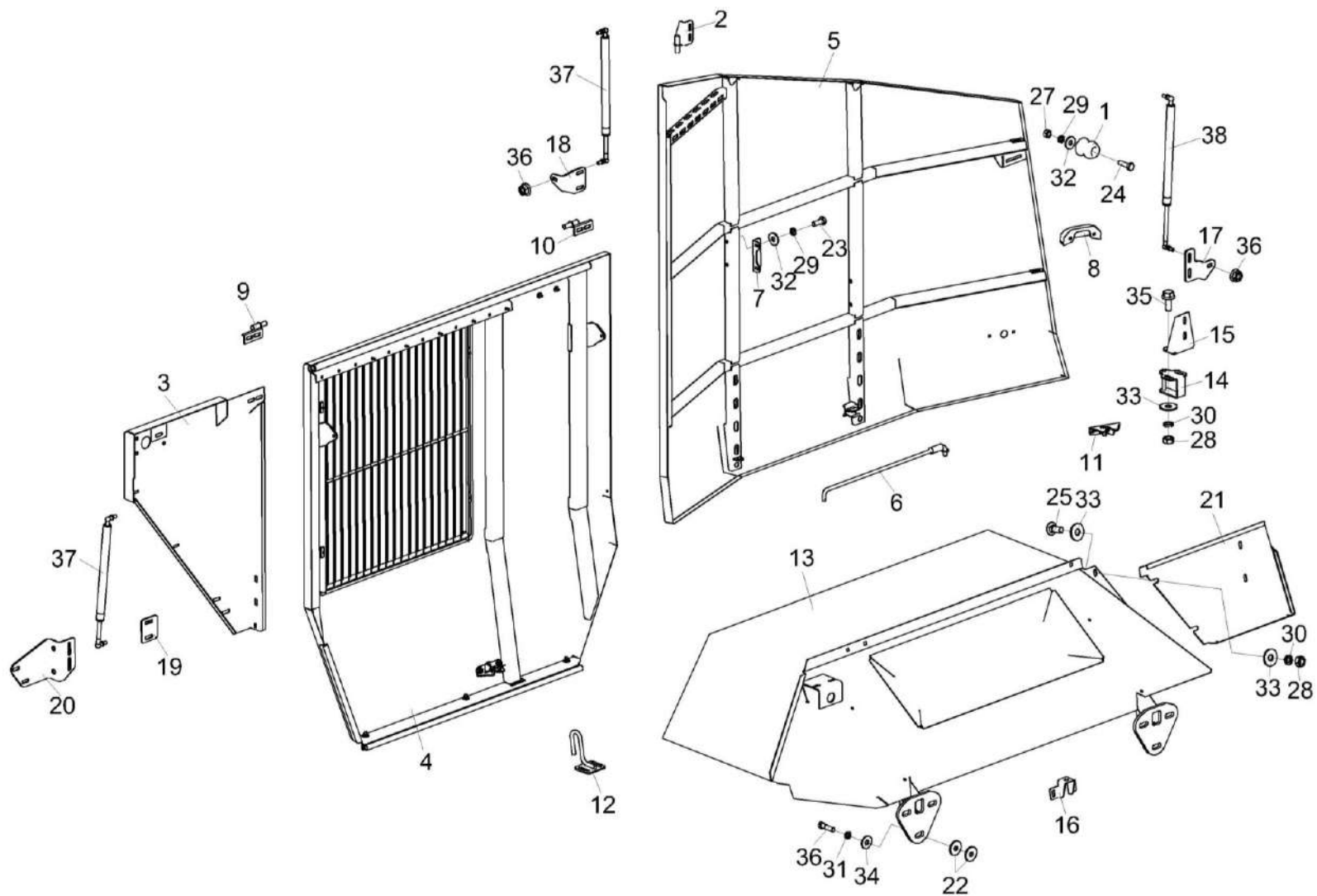
Рисунок 182 – Установка капотов КВС-80-8-0160000-01 (лист 3)
