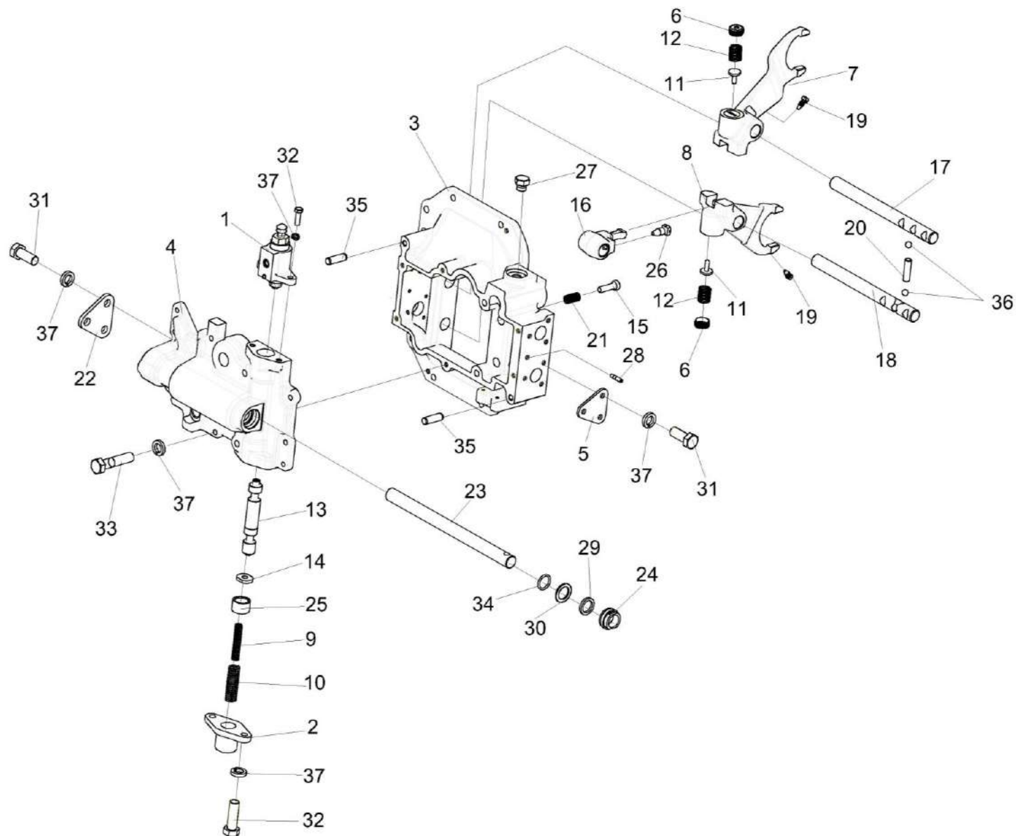
Рисунок 19 – Механизм переключения диапазонов КЗК-8-0107560-01
