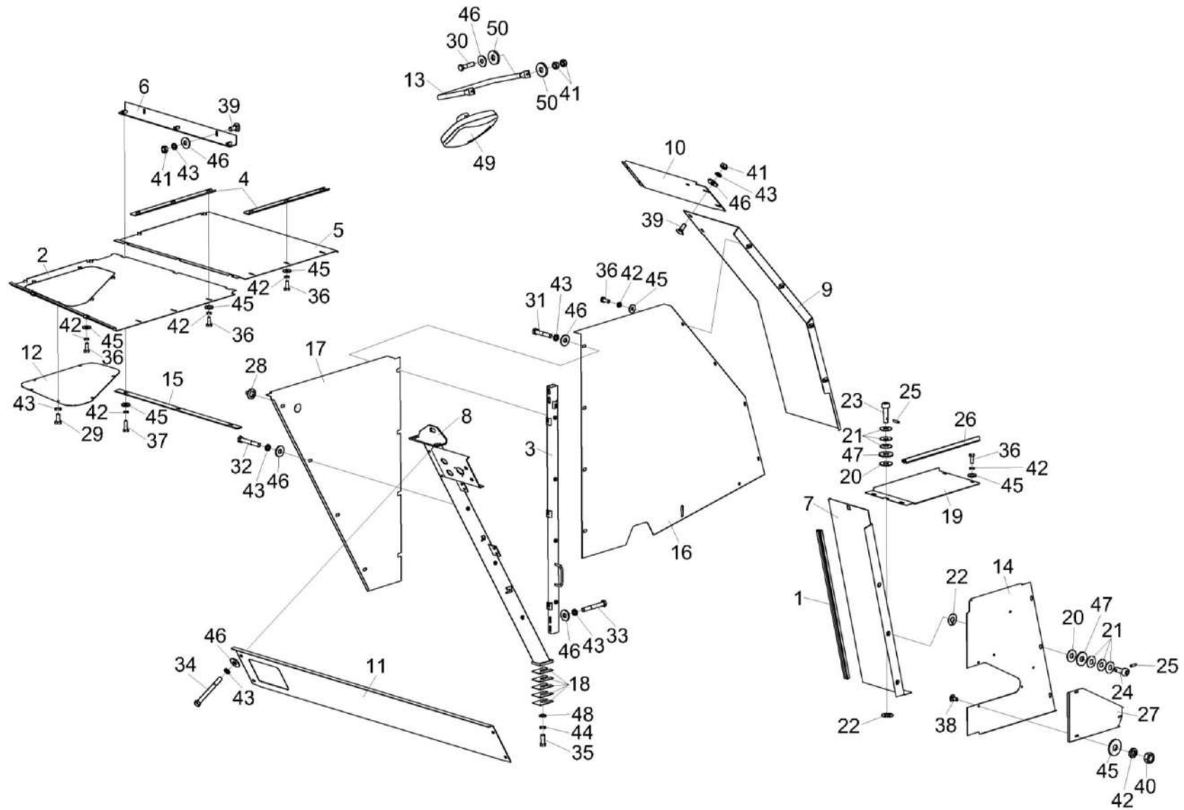
Рисунок 192 – Установка ограждений КВС-80-8-0100100 (лист 1)
