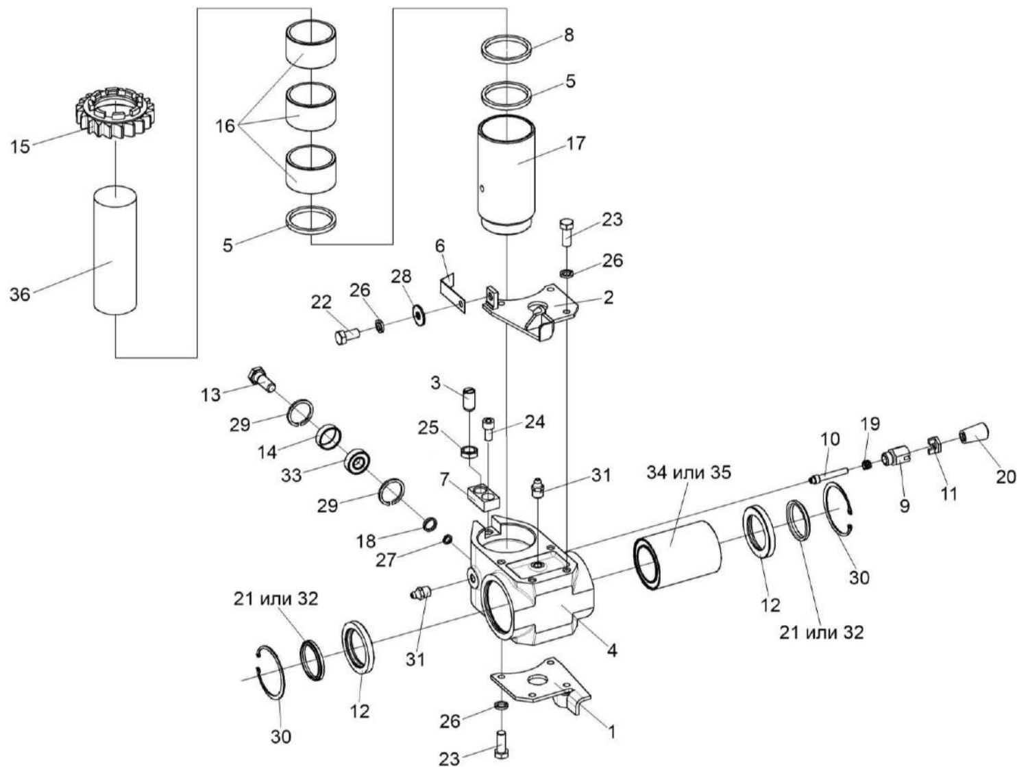
Рисунок 85 – Установка каретки КВС-2-0116650
