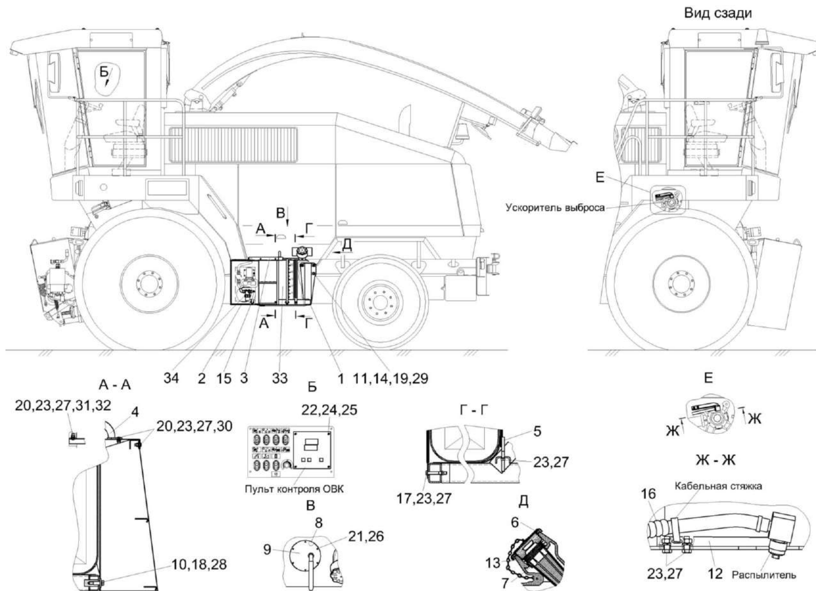
Рисунок 257 – Установка ОВК КВС-2-0900000А
