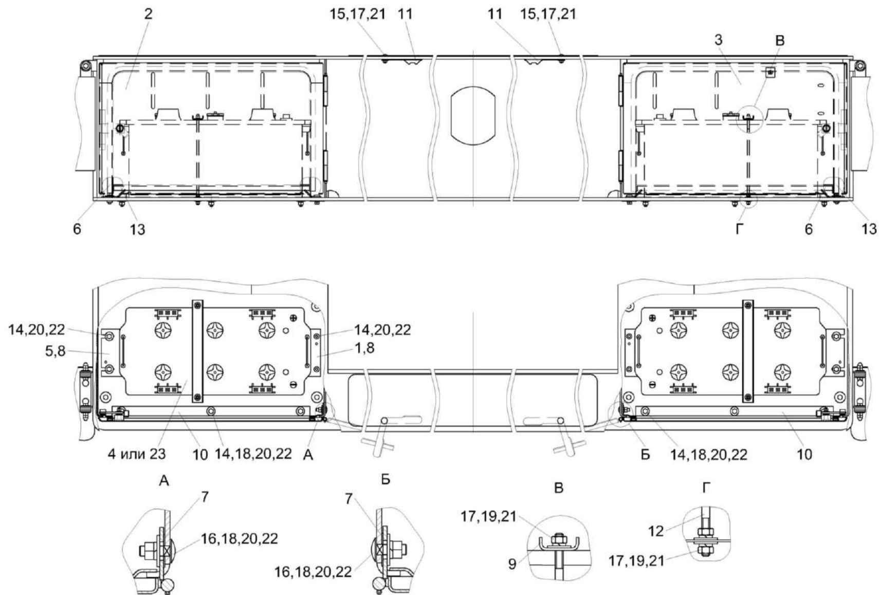
Рисунок 250 – Установка аккумуляторов КВС-2-0101040
