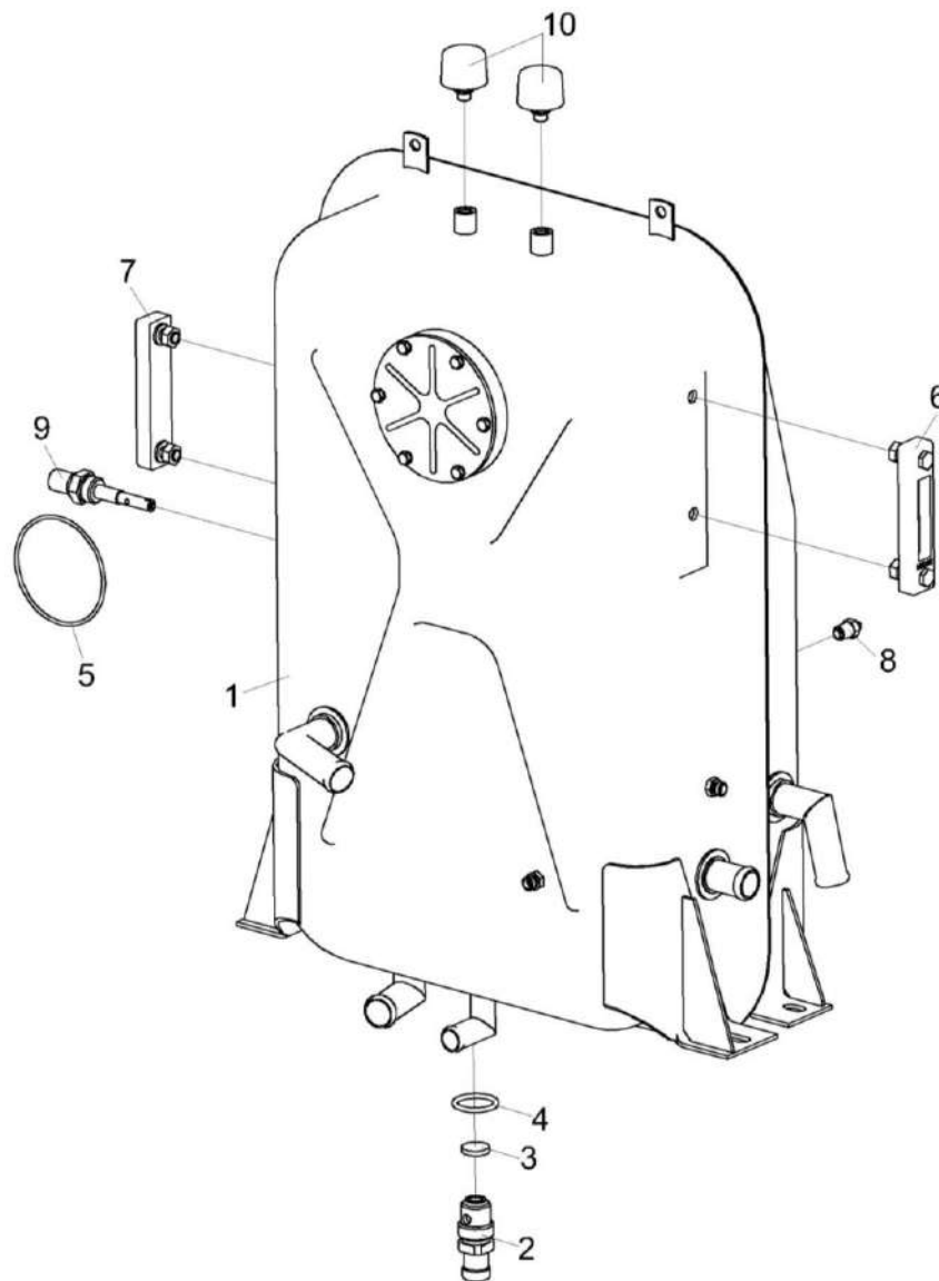
Рисунок 206 – Бак масляный КВС-2-0601310В
