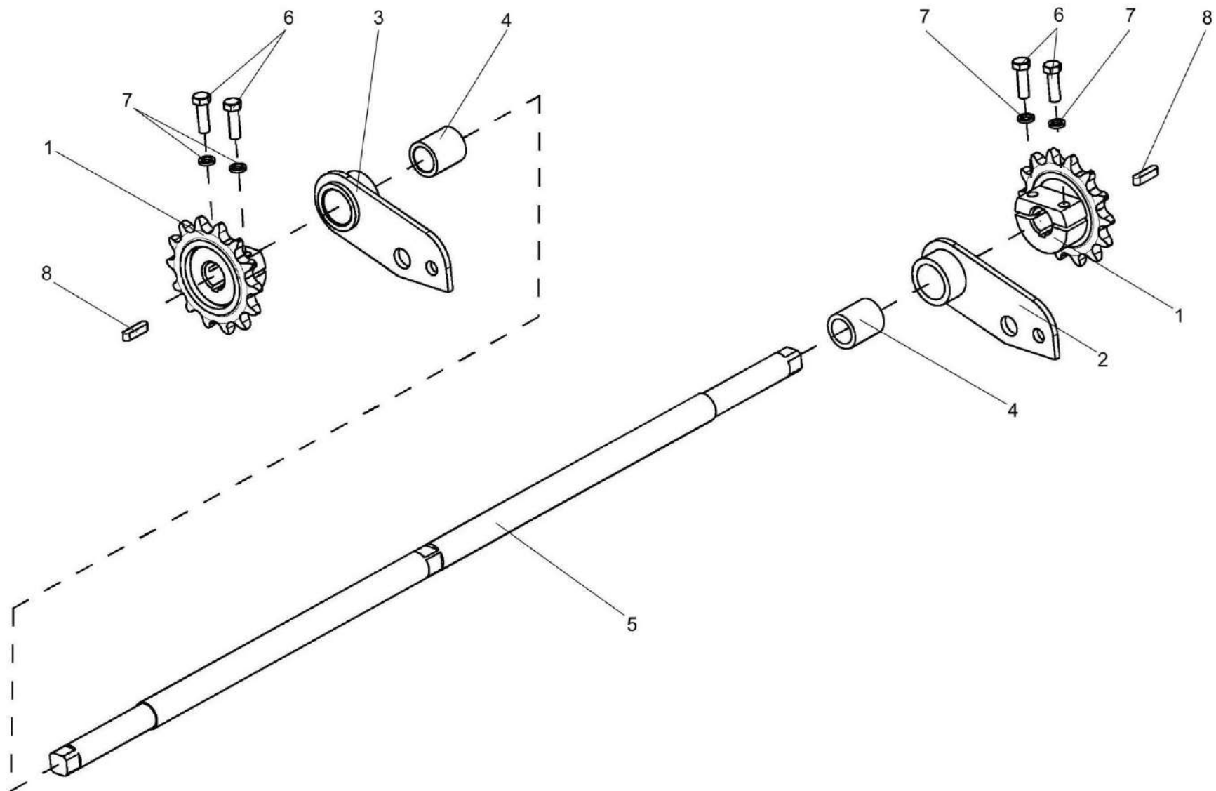
Рисунок 122 – Механизм перемещения КВС-1-0148170
