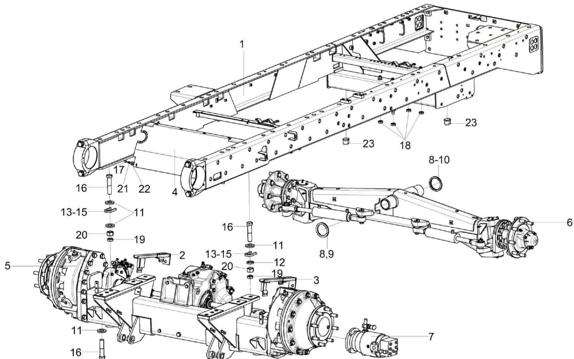
Рисунок 5 – Шасси КВС-80-8-0101000 (лист 1)
