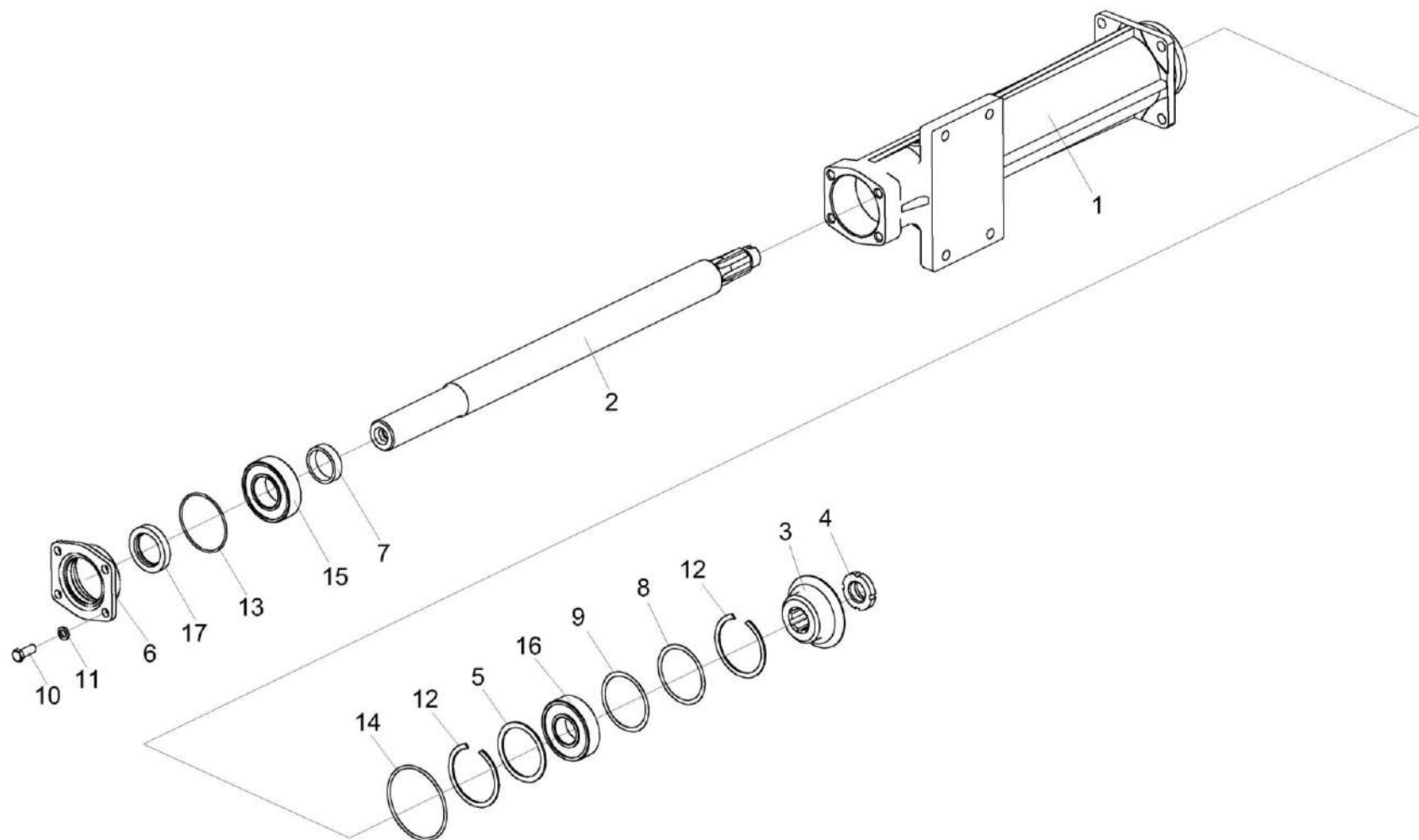
Рисунок 45 – Стакан КВС-1-0135120
