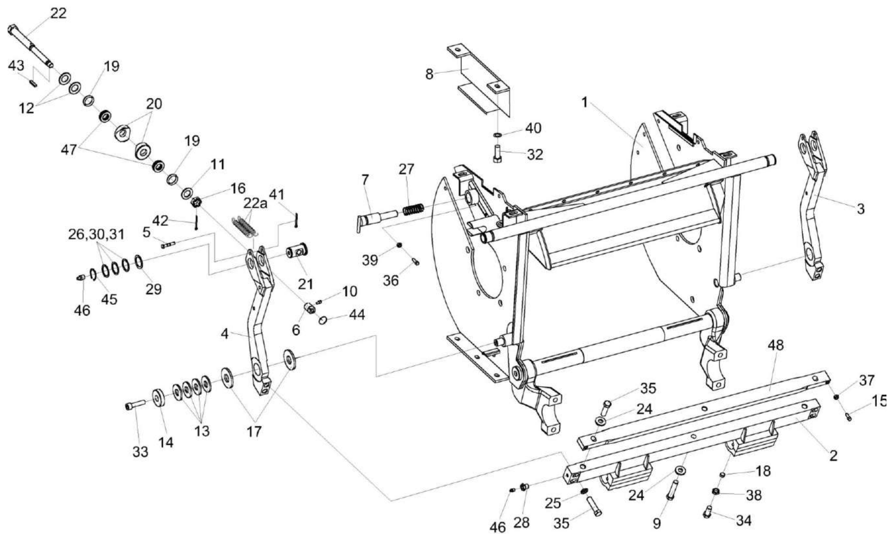
Рисунок 83 – Установка рычага КВС-8-0117120 и КВС-8-0117120-01
