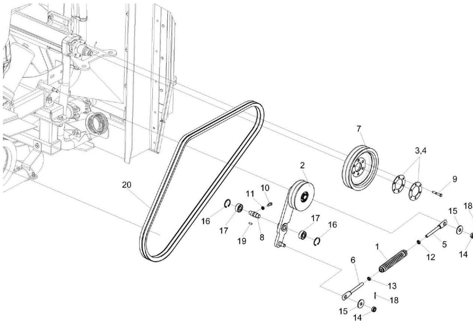
Рисунок 40 – Установка привода вентилятора КВС-7-0150800
