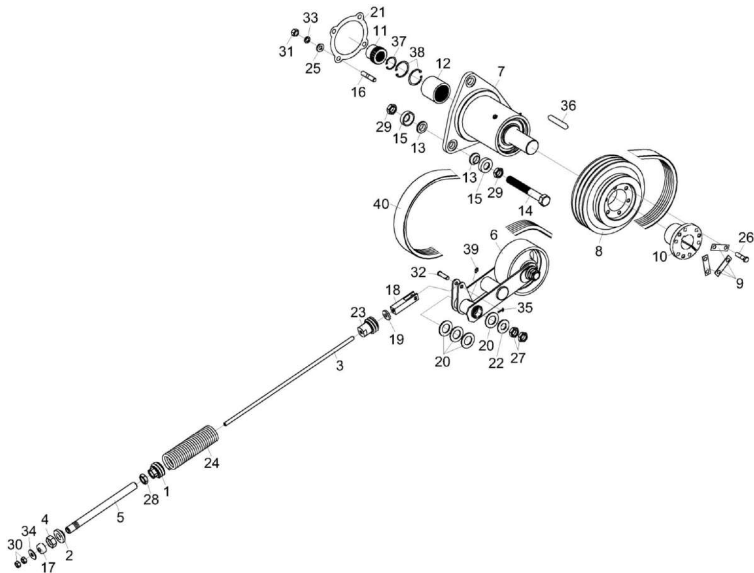
Рисунок 55 – Привод гидростата КВС-80-5-0133000
