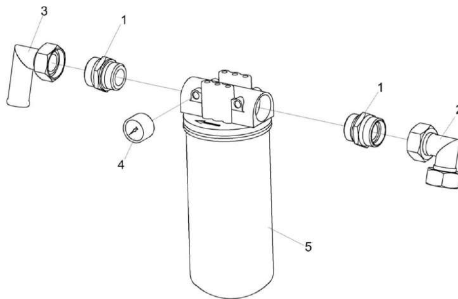
Рисунок 207 – Фильтр всасывающий КВС-2-0601090Б
