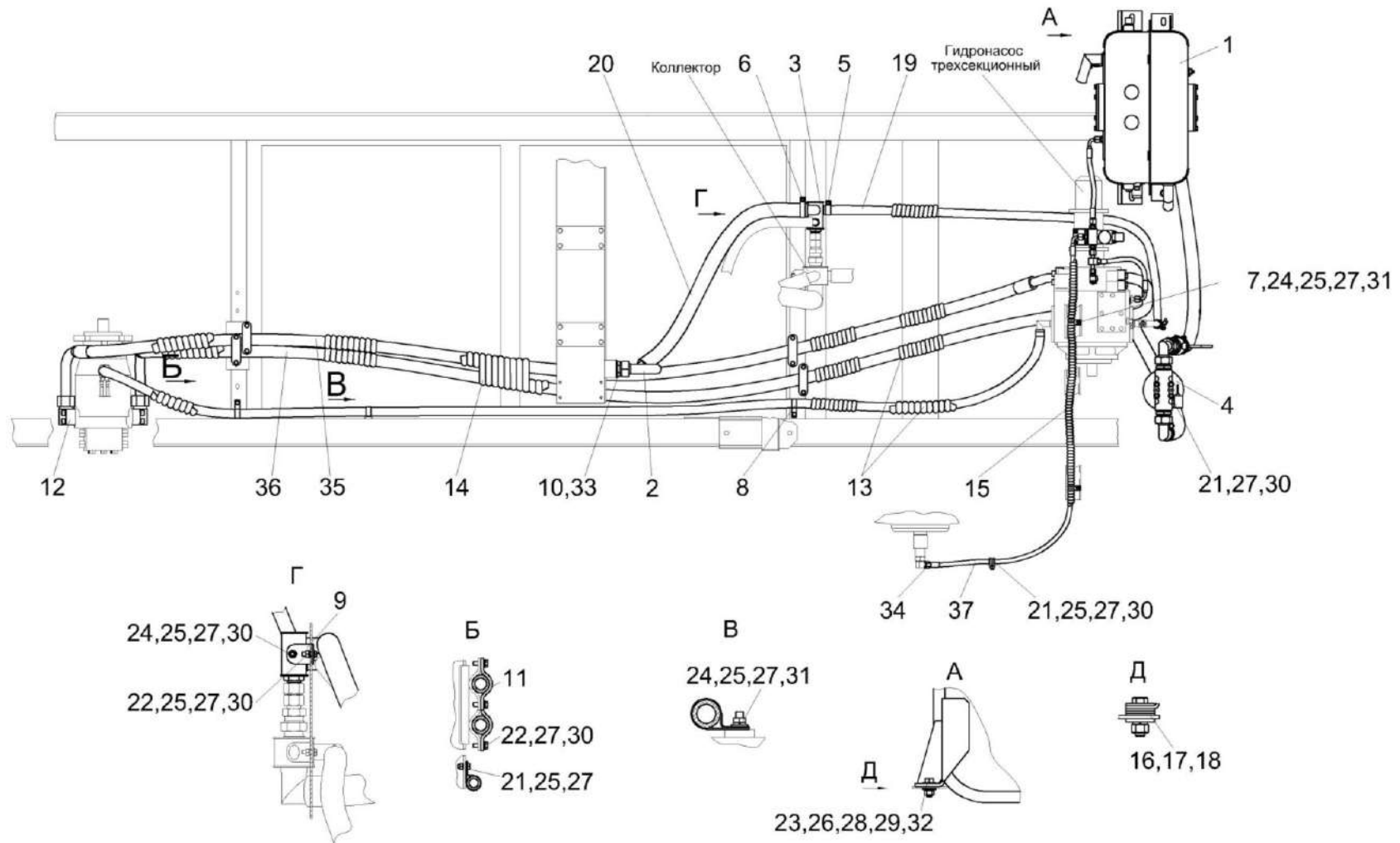
Рисунок 205 – Гидросистема привода ходовой части КВС-2-0601000В (лист 2)
