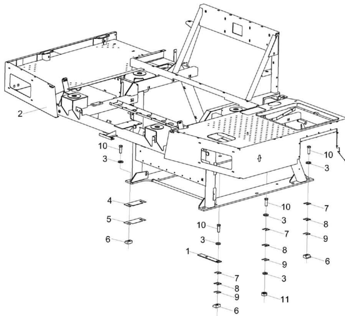
Рисунок 161 – Установка площадки входа КВС-80-8-0124000
