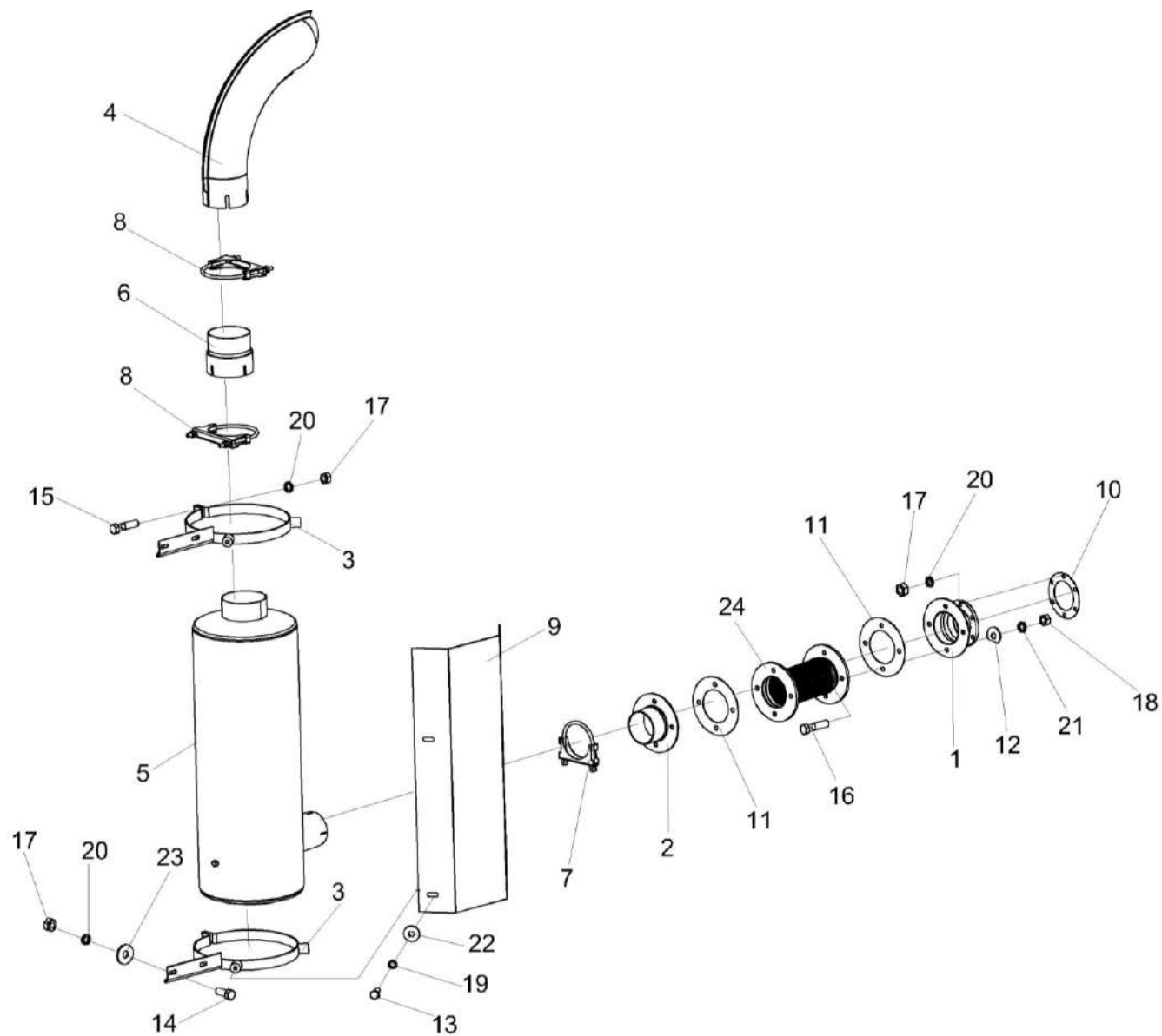
Рисунок 51 – Установка глушителя КВС-7-0157000
