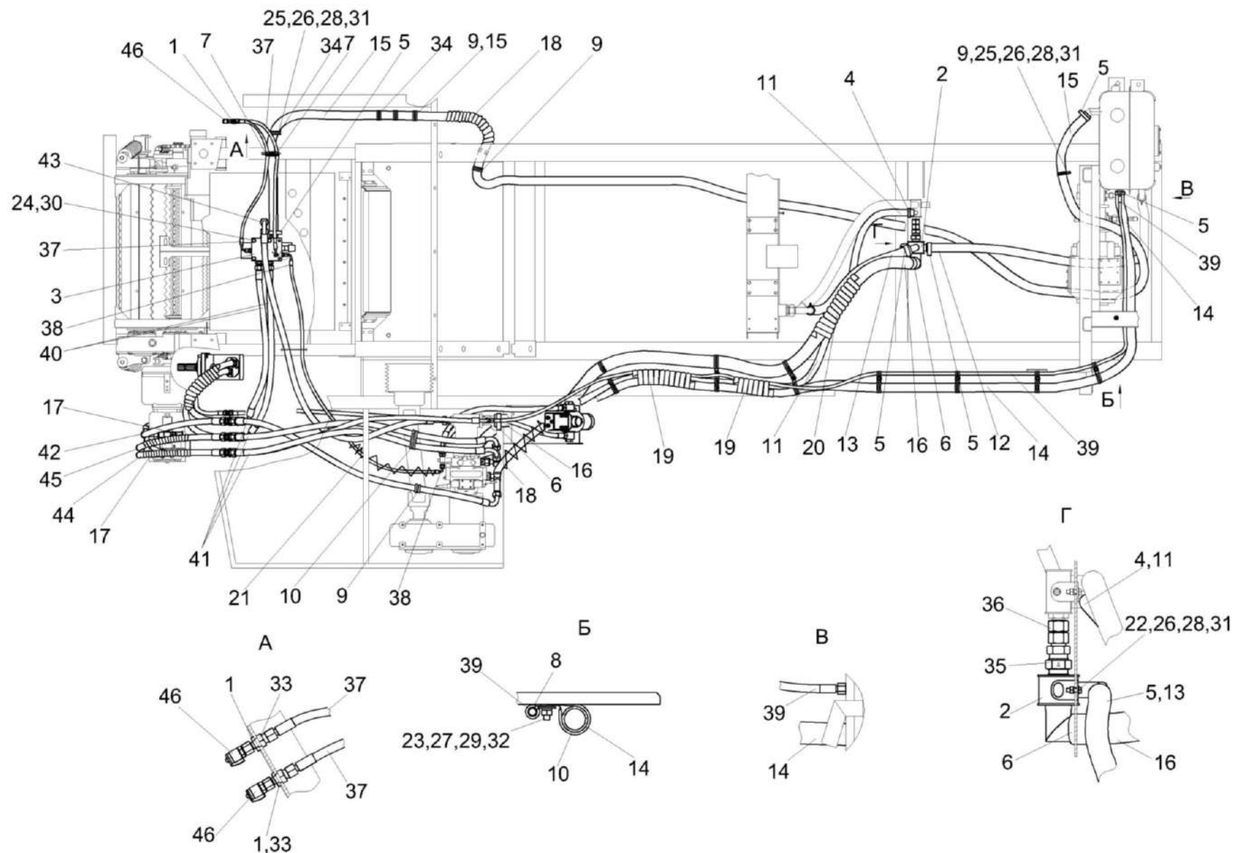
Рисунок 226 – Гидросистема привода питающего аппарата и адаптеров КВС-5-0604000 (лист 2)
