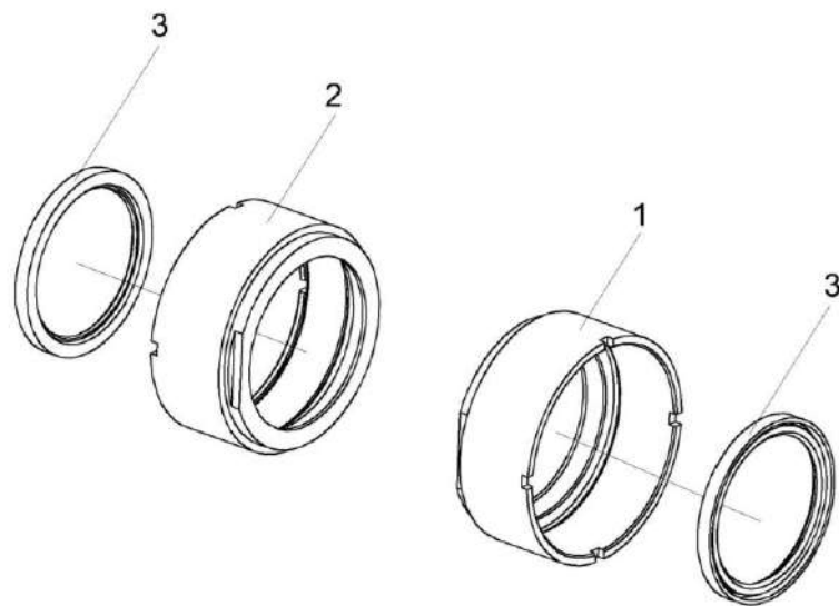
Рисунок 91 – Стакан КВС-1-0100120 и КВС-1-0100120-01
