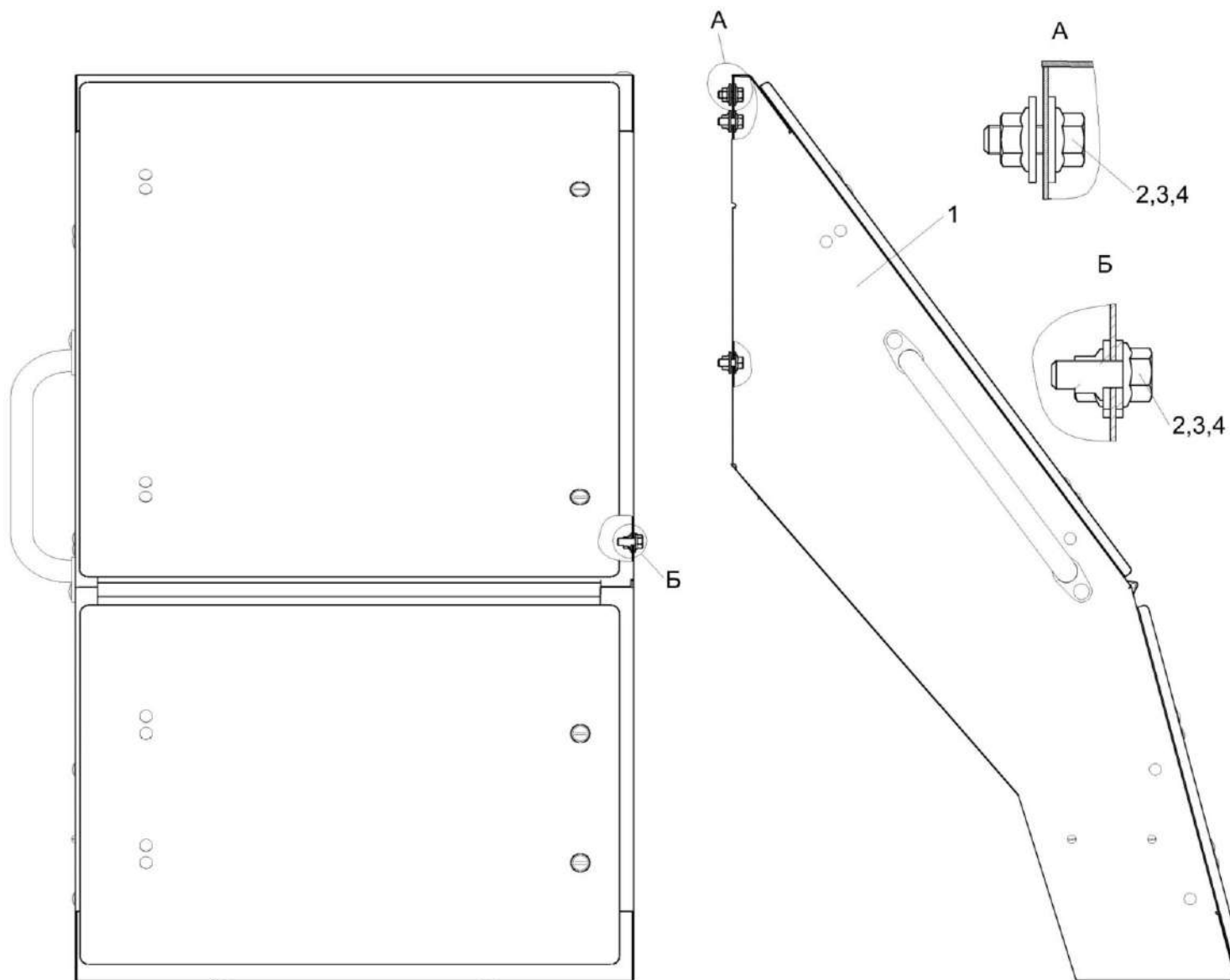
Рисунок 253 – Установка электрошкафа КВС-80-8-0702000
