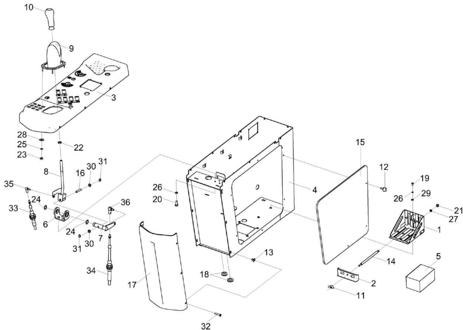
Рисунок 146 – Пульт управления КВС-80-8-0119500
