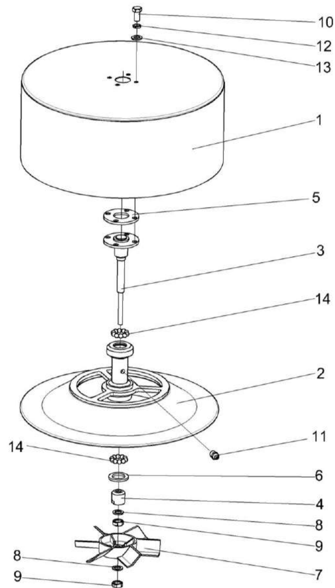
Рисунок 54 – Воздухозаборник вращающийся КВС-1-0153000А
