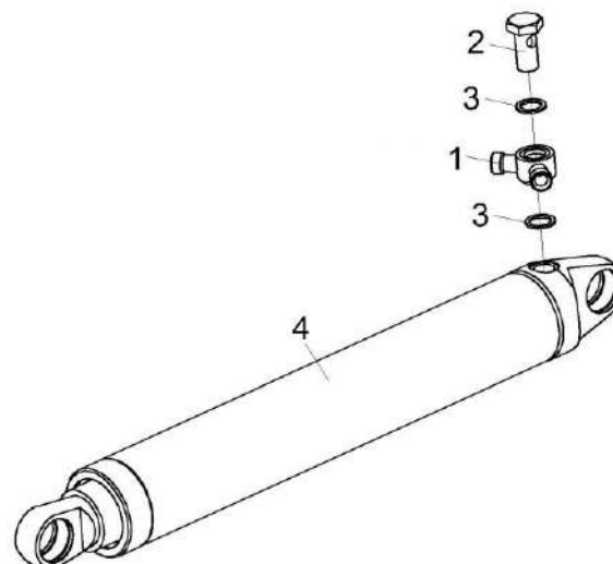
Рисунок 215 – Гидроцилиндр КВС-8-0602500 и КВС-8-0602500-01
