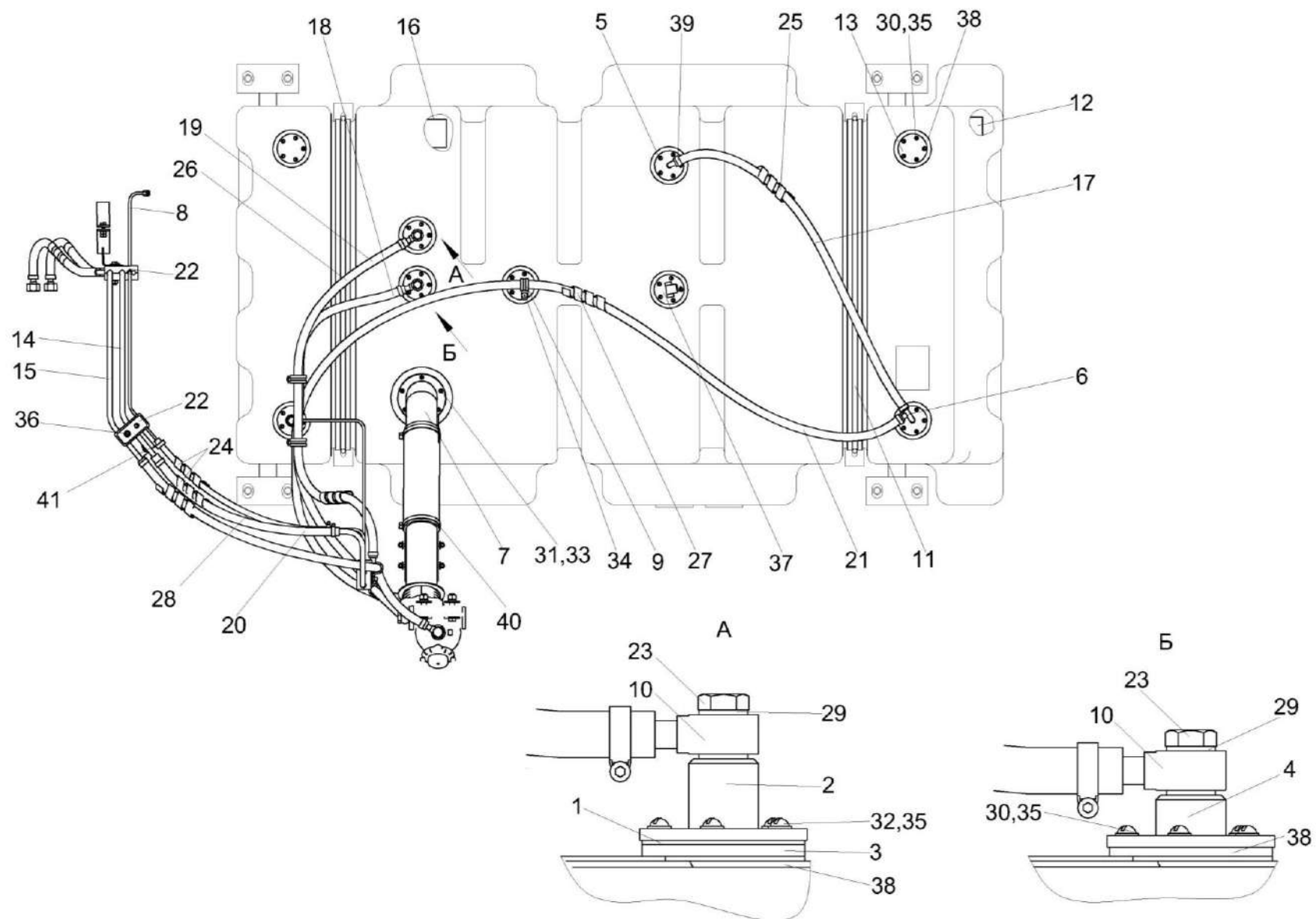
Рисунок 201 – Установка топливного оборудования КВС-7-0103700 (лист 2)
