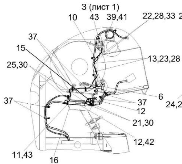
Рисунок 247 – Установка электрооборудования КВС-80-7-0721000 (лист 2)
