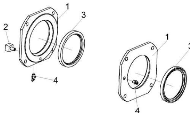
Рисунок 92 – Крышка КВС-1-0100130 и КВС-1-0100130-01
