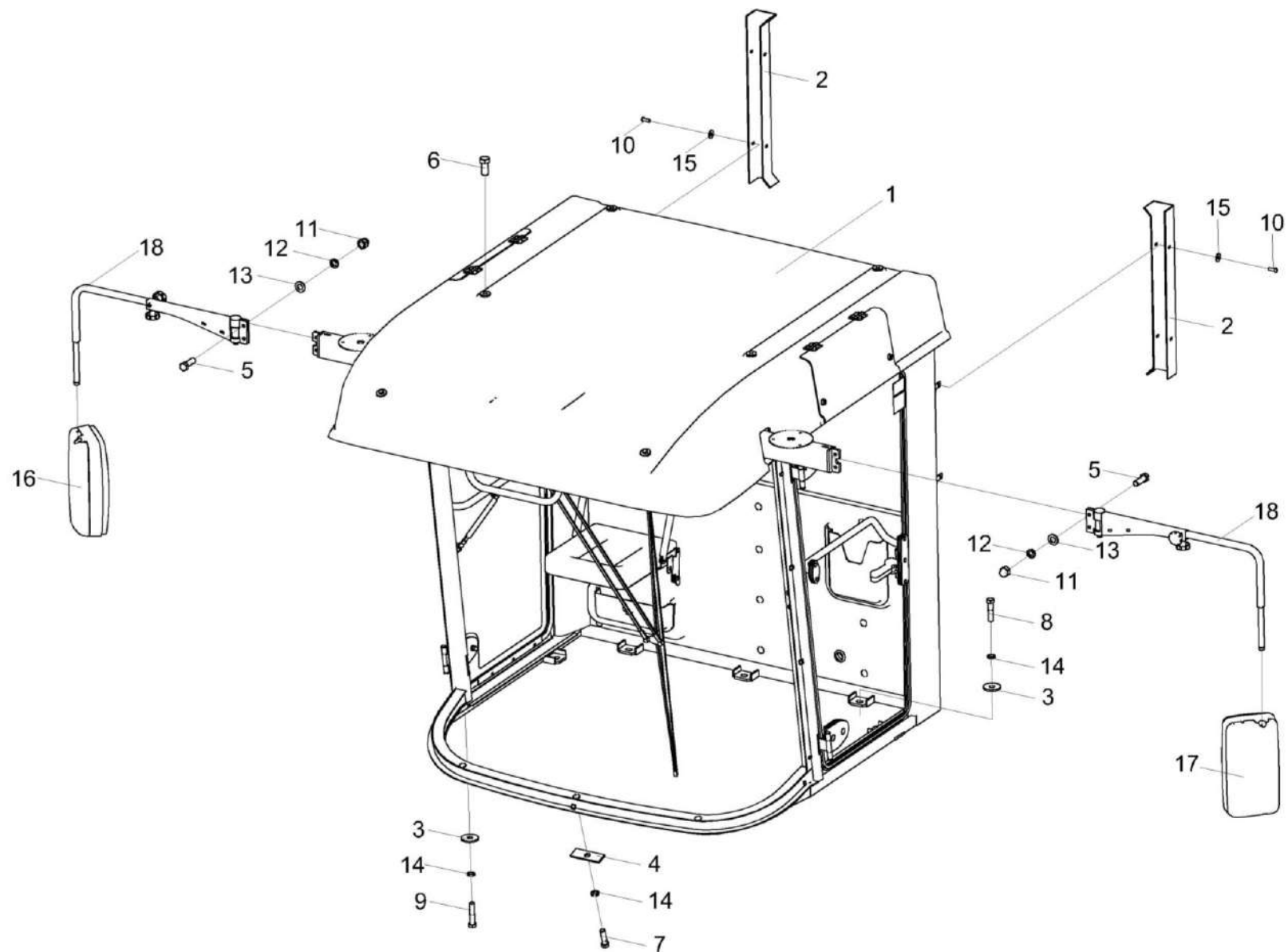
Рисунок 163 – Установка кабины КВС-80-8-0120000
