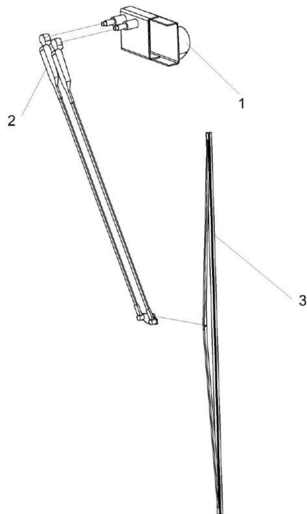
Рисунок 169 – Установка стеклоочистителя КЗК-12-0120810
