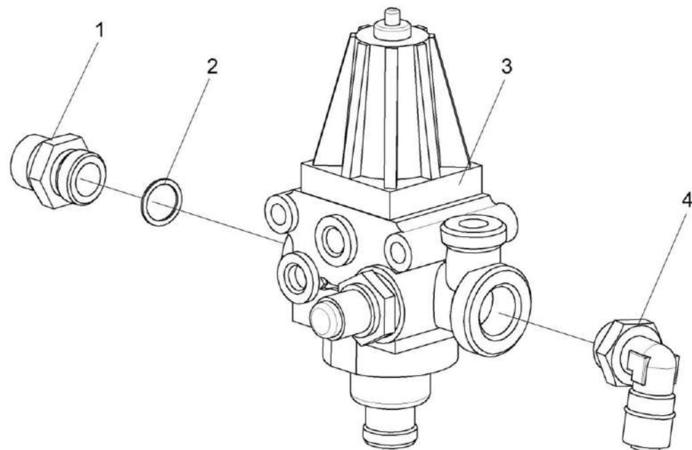
Рисунок 242 – Регулятор давления КВС-5-0800190
