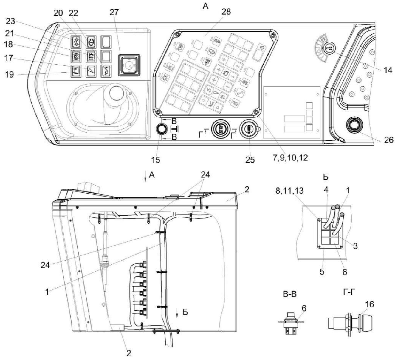
Рисунок 147 – Установка электрооборудования пульта управления КВС-80-7-0725000А
