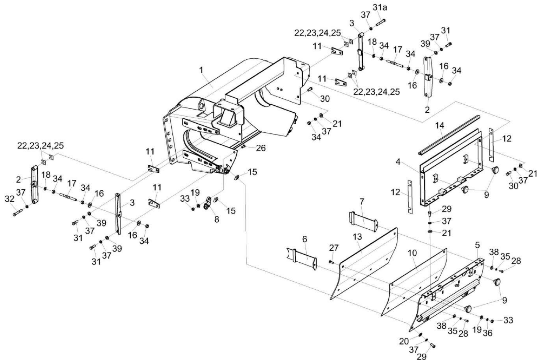
Рисунок 127 – Ускоритель выброса КВС-2-0142000 (лист 1)
