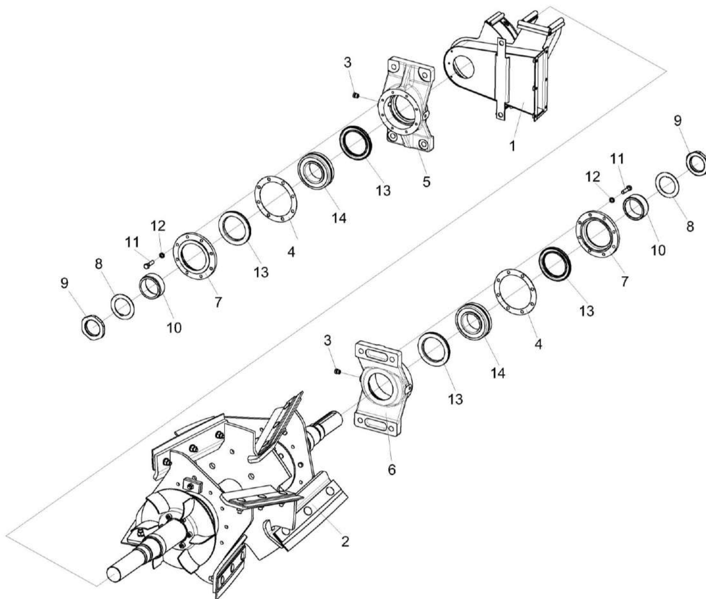
Рисунок 129 – Вал ускорителя выброса КВС-2-0142100
