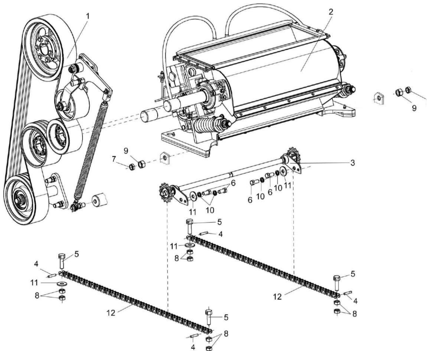
Рисунок 100 – Устройство доизмельчающее КВС-80-8-0148000
