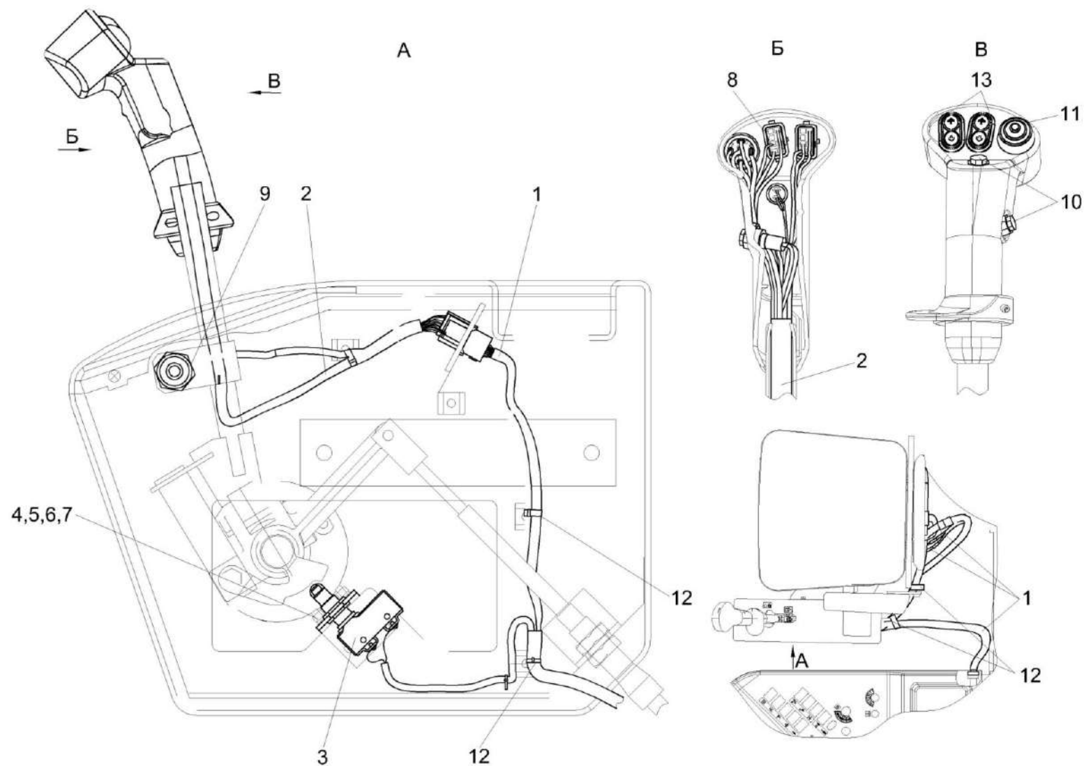
Рисунок 144 – Установка электрооборудования блока управления КВС-80-8-0727000
