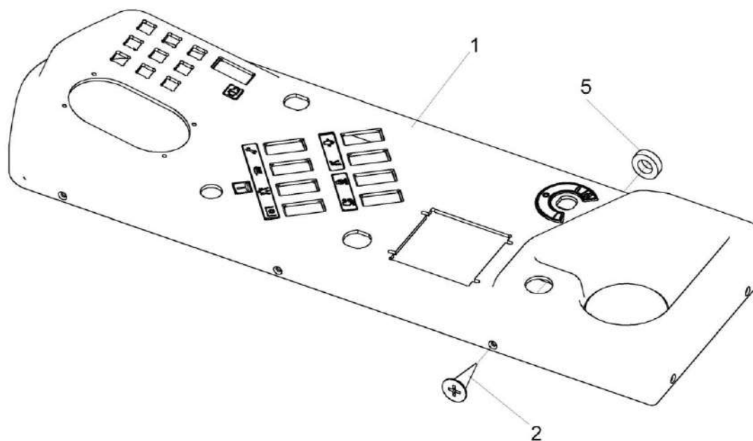
Рисунок 148 – Установка панели КВС-80-8-0119490А
