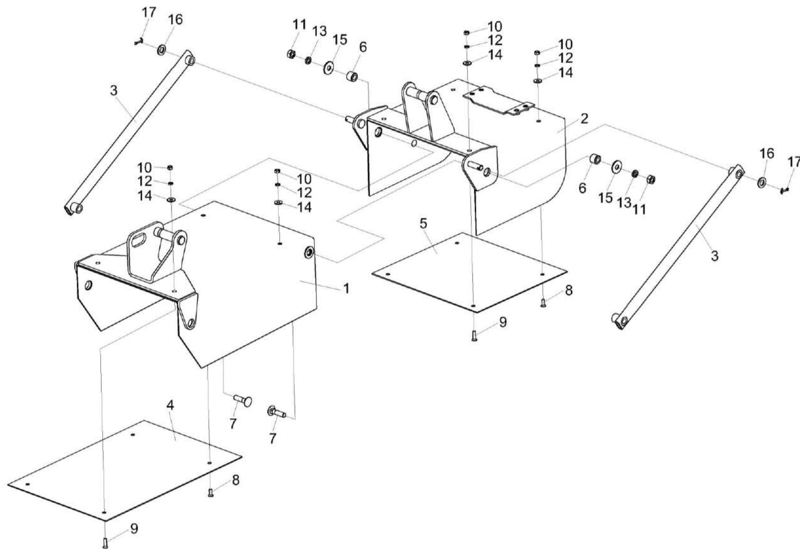
Рисунок 137 – Козырек КВС-2-0144310А
