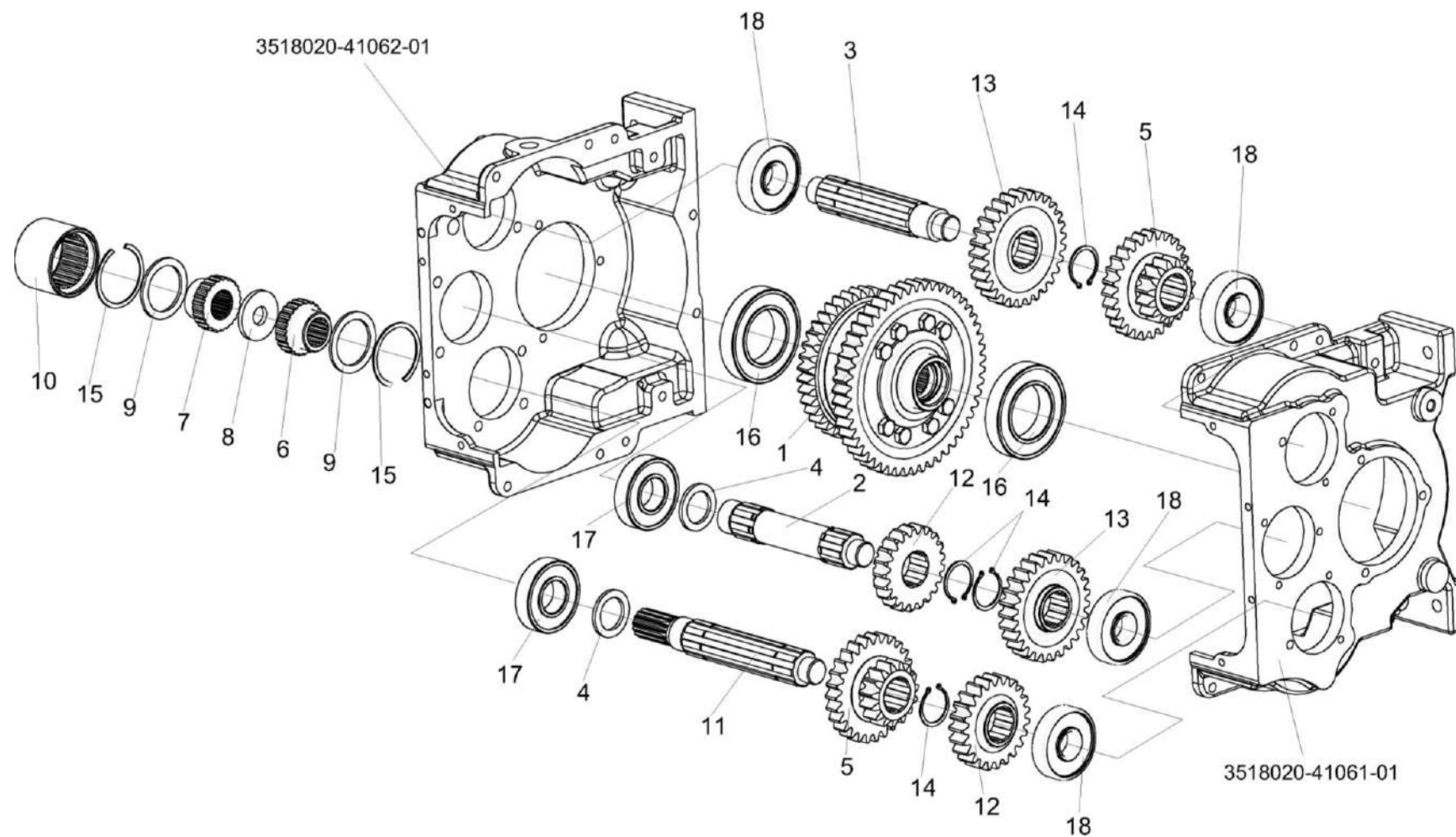
Рисунок 17 – Коробка диапазонов КВС-2-0107230 (валы и шестерни)
