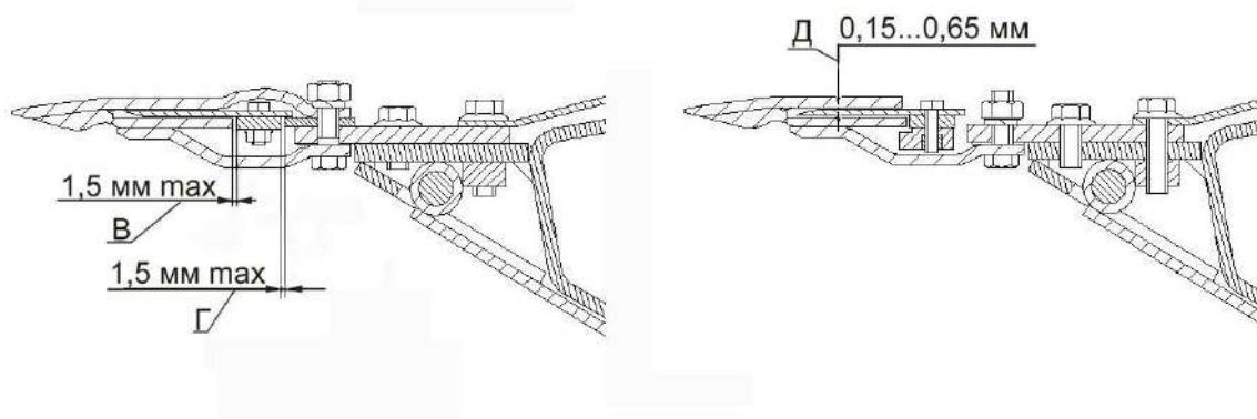
Рисунок 2.9 – Режущий аппарата жатки
