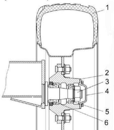
Рисунок 2.11 - Регулировка подшипников
