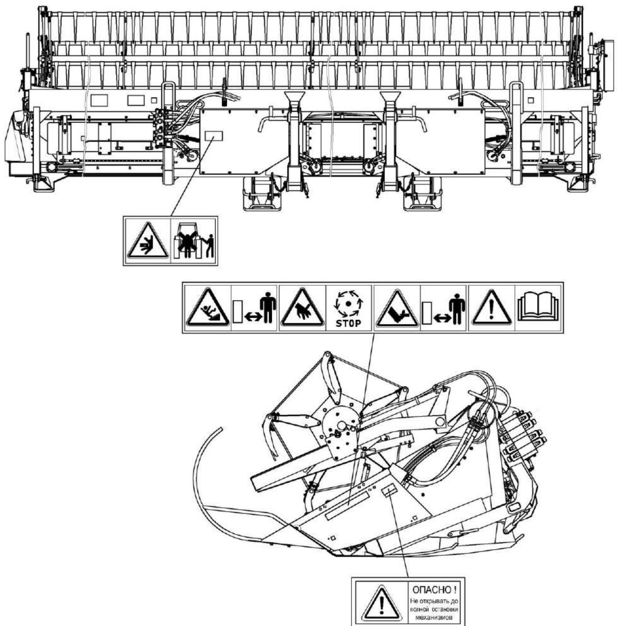
Знаки безопасности (пиктограммы) на жатке валковой
