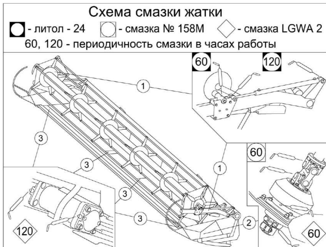
Рисунок 3.1 – Схема смазки жатки
