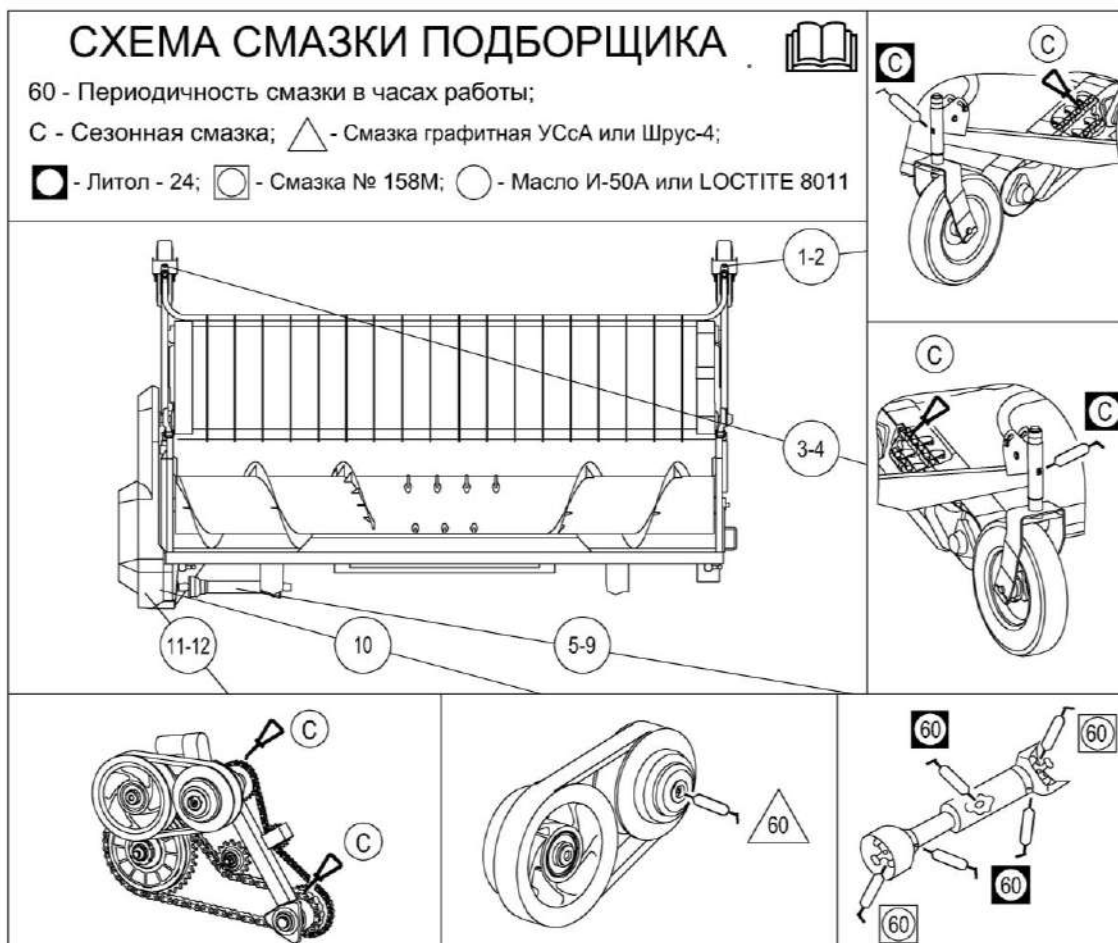
Рисунок 3.1 – Схема смазки
