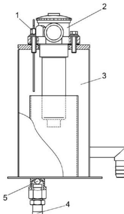
Рисунок 1.4 – Масляный бак
