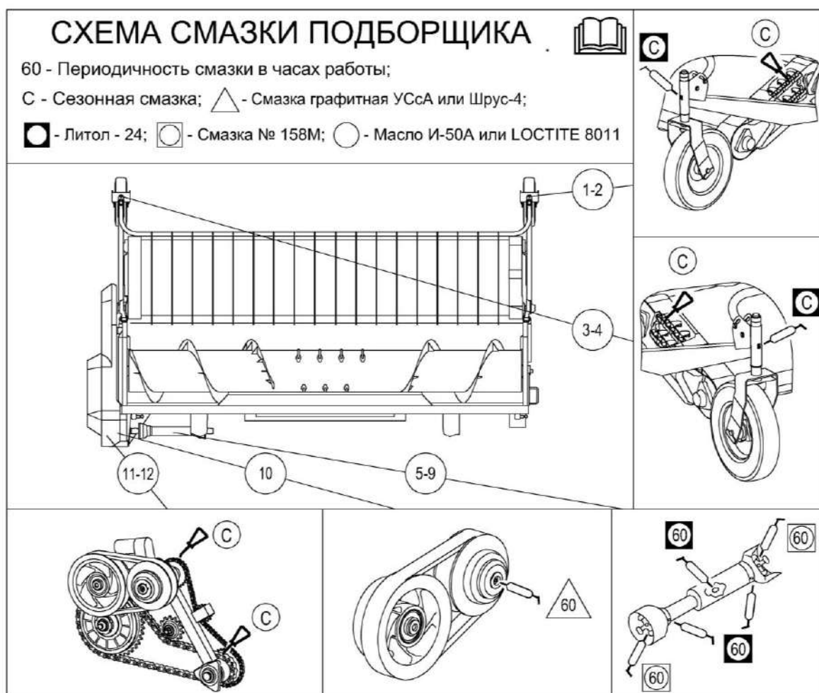
Рисунок 3.1 – Схема смазки
