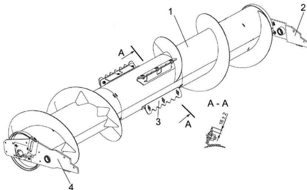
Рисунок 1.5 – Шнек
