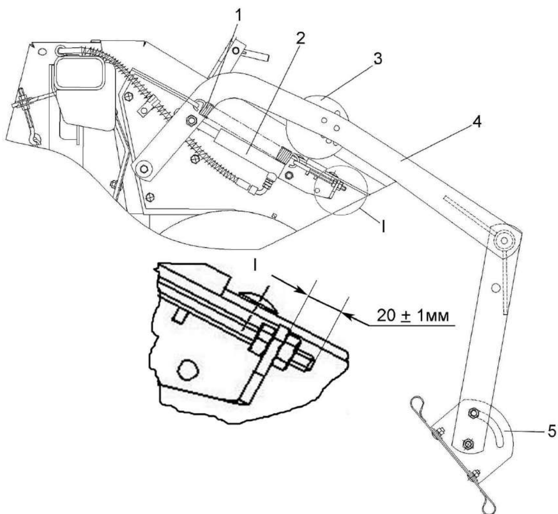
Рисунок 1.6 – Устройство прижимное
