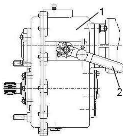
Рисунок 2.1 - Коробка передач
