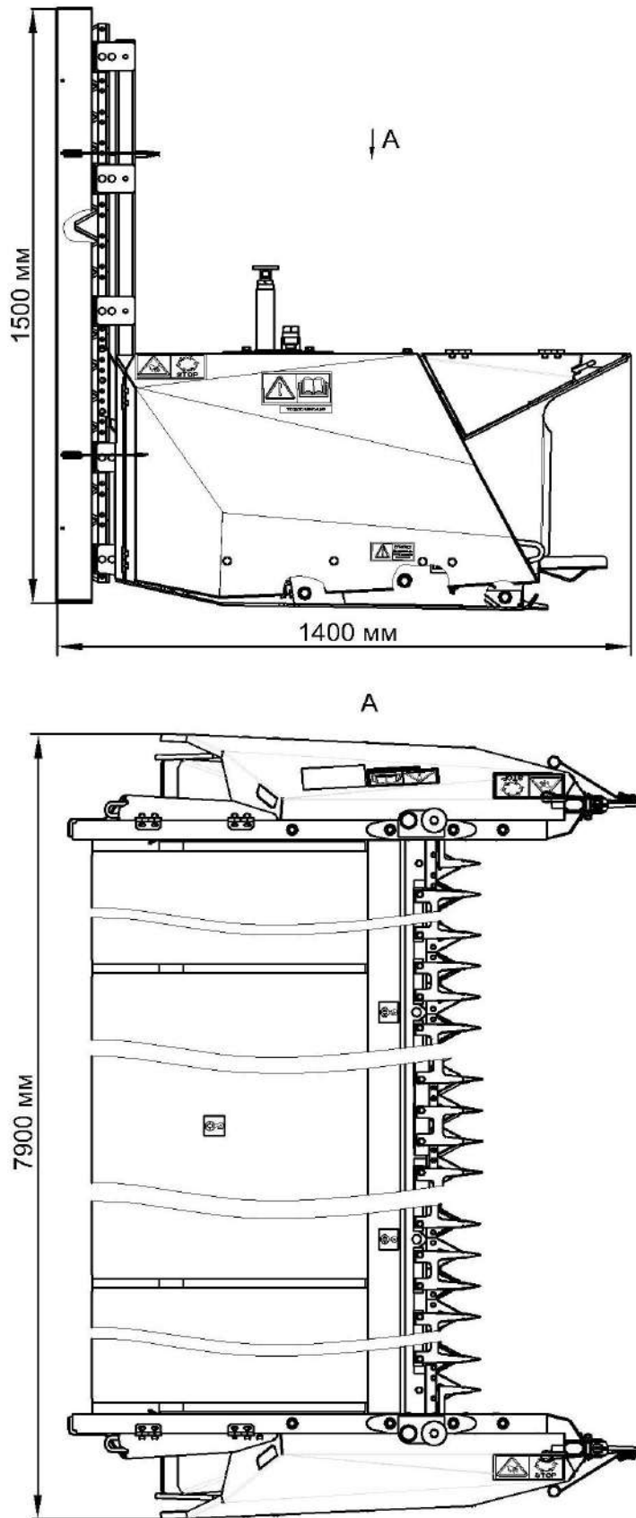
Рисунок 1.1 – Габаритные размеры
