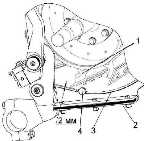
Рисунок 2.13 - Измельчающий аппарат
