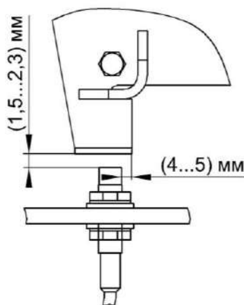
Рисунок 2.12 – Установка датчика положения бруска абразивного
