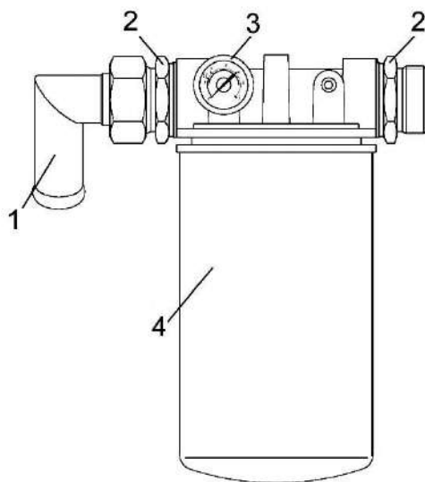
1 - угольник; 2 - штуцеры; 3 - манометр; 4 – фильтр
