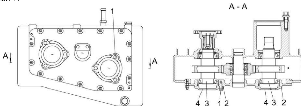
1 – болты; 2 – прокладки; 3 – вал-шестерня; 4 – крышка
