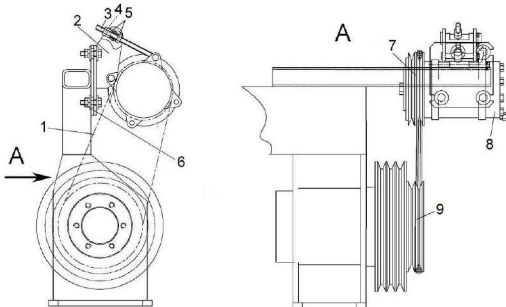
Рисунок 2.19 – Регулировка привода компрессора кондиционера
