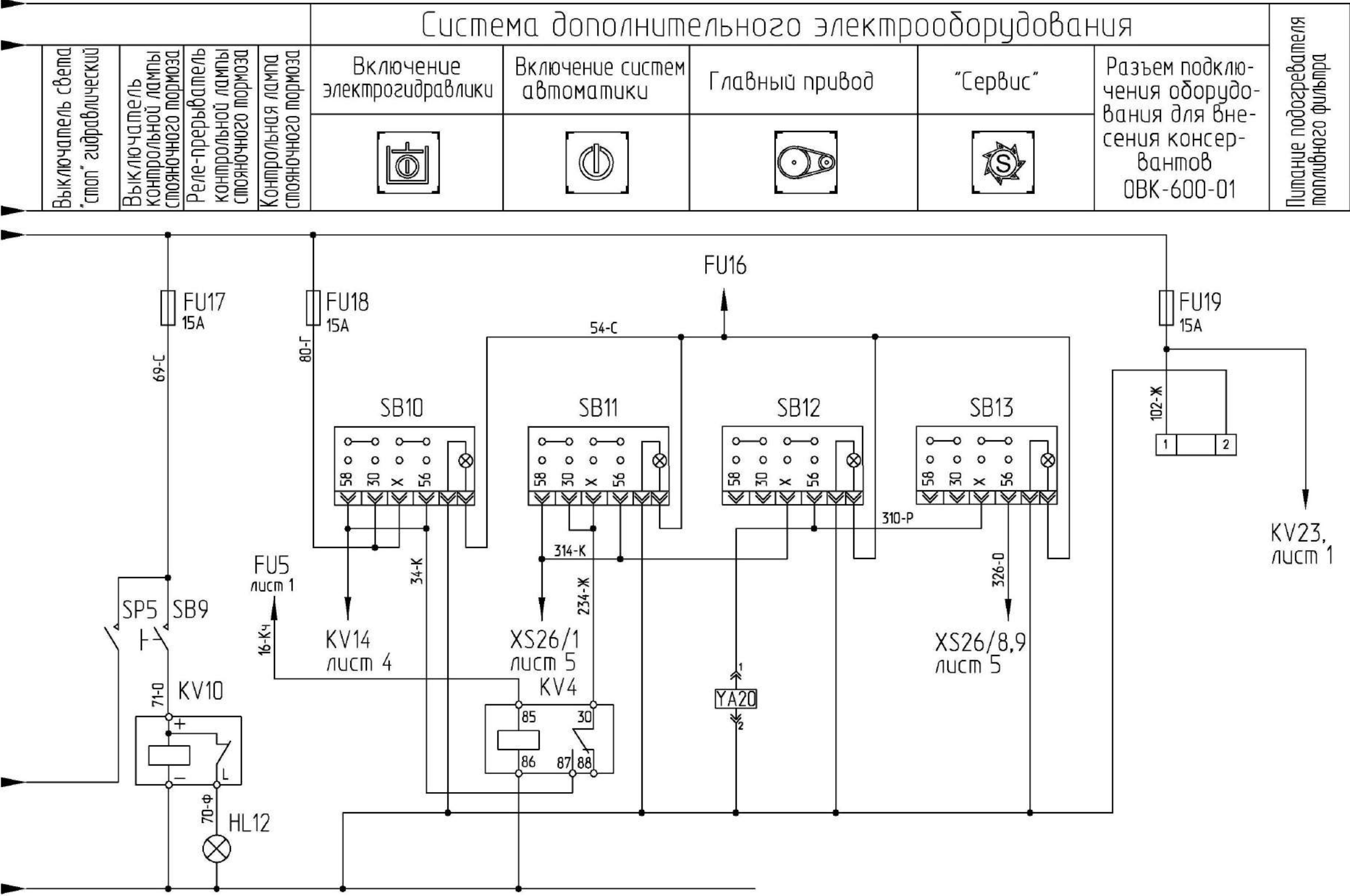
Рисунок Б.2 – Схема электрическая принципиальная комплекса (лист 2)
