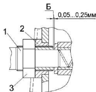
Рисунок 2.26 – Основание силосопровода
