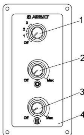
Рисунок 1.41 – Панель управления климатической установкой
