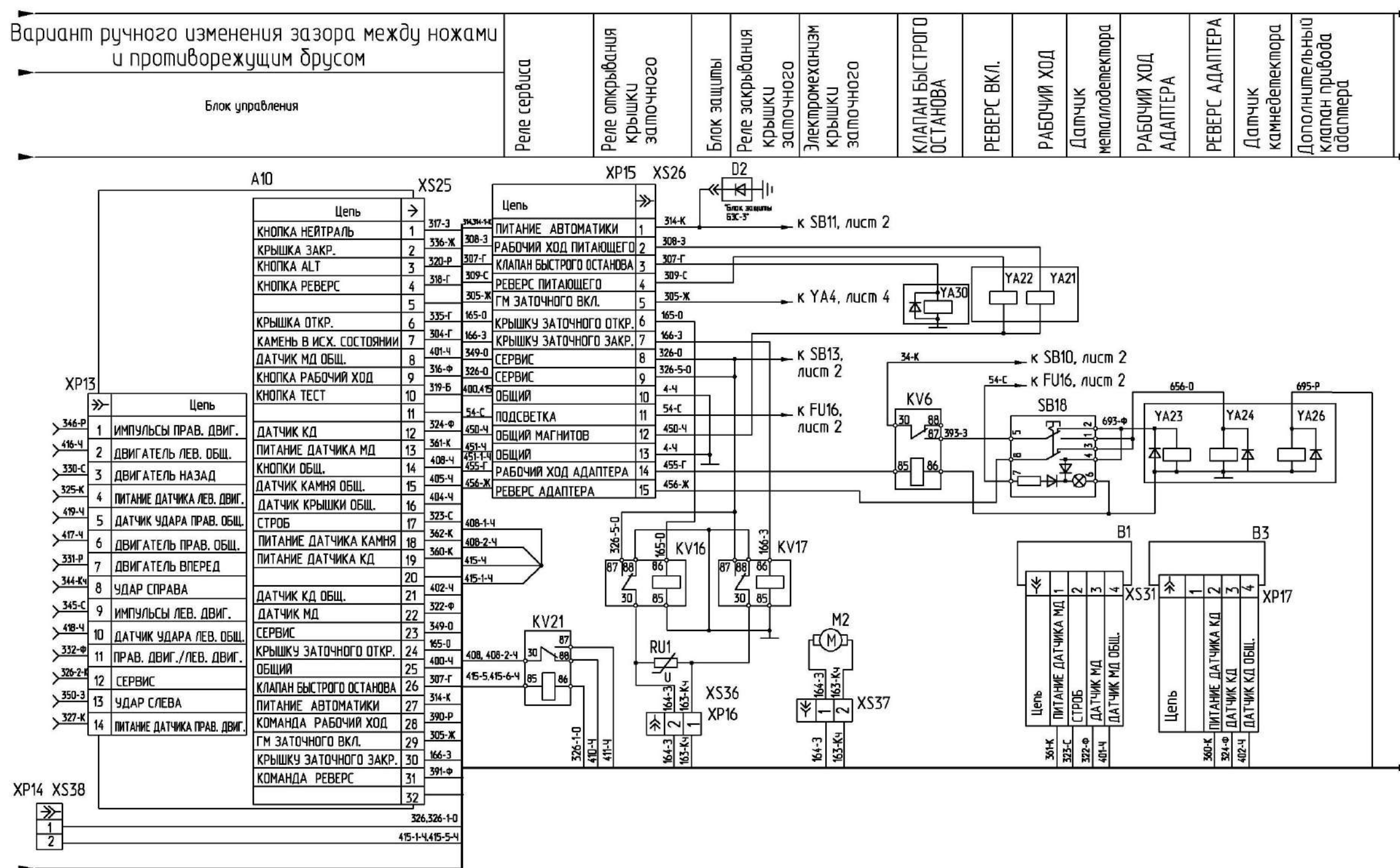
Рисунок Б.5 – Схема электрическая принципиальная комплекса (лист 2)
