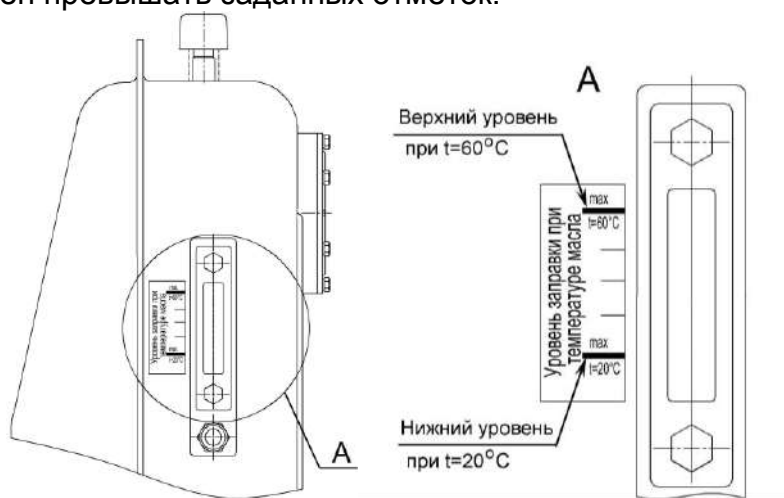
Рисунок 2.5 – Заправка гидросистем
