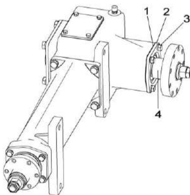
1 – набор прокладок; 2 – крышка; 3 – болты; 4 – вал
