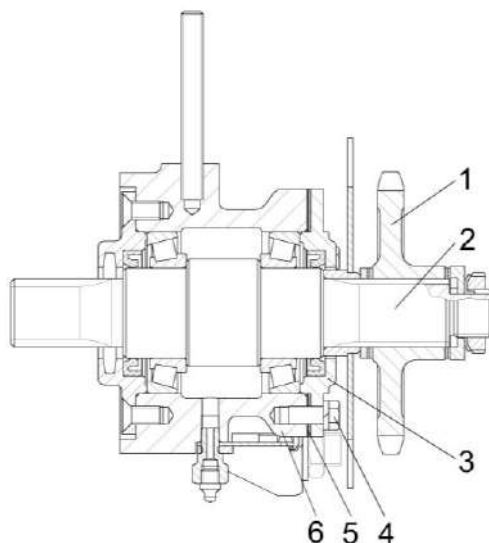
1 – звездочка; 2 – вал; 3 – крышка; 4 – болты; 5 – прокладки; 6 – корпус
