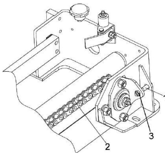
Рисунок 2.20 – Устройство заточное
