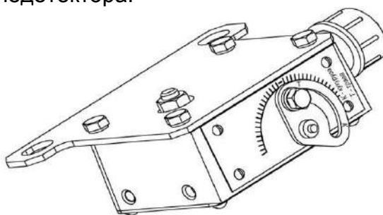
Рисунок 2.6 – Датчик камнедетектора
