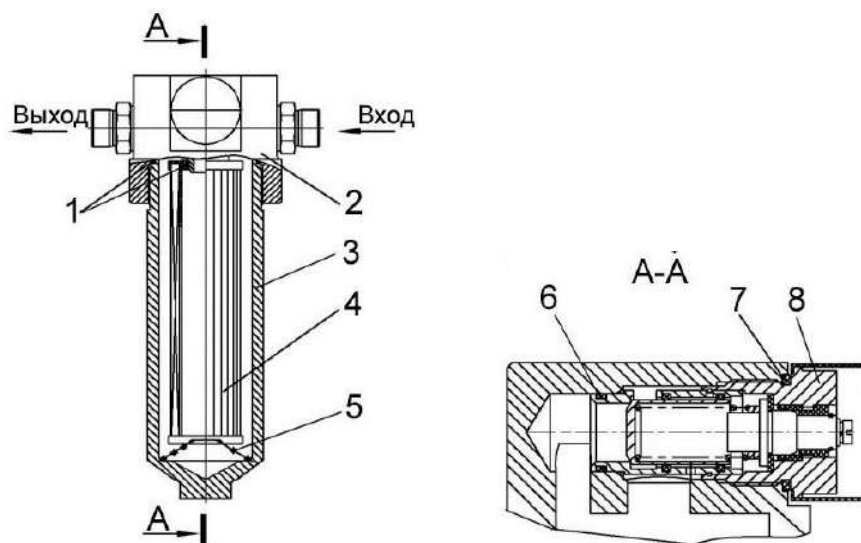
1,6,7, - кольца уплотнительные; 2 – головка фильтра; 3 – стакан; 4 - фильтроэлемент; 5 – пружина; 8 – клапан - сигнализатор
