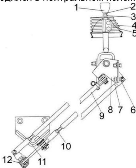
Рисунок 2.23 – Механизм переключения передач
