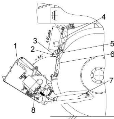
Рисунок 2.10 – Отвод питающего аппарата от измельчающего
