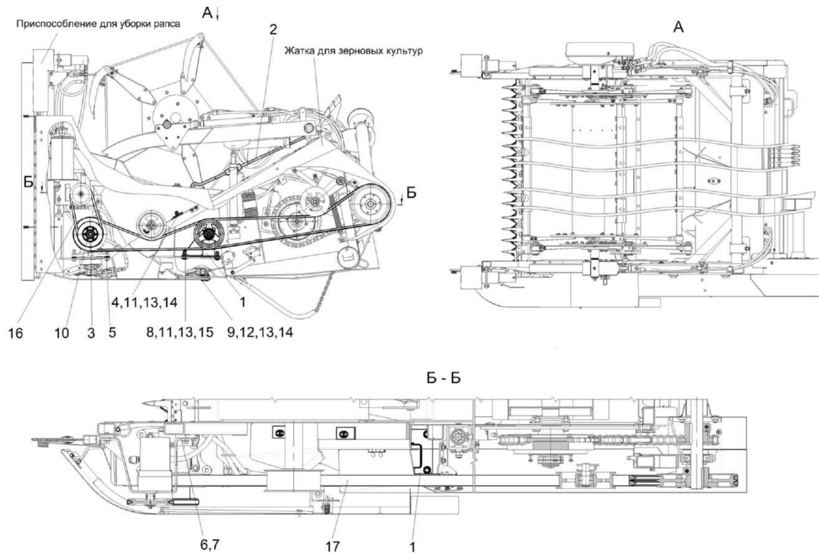
Рисунок 19 – Комплект монтажных частей КЗК-1492-1540700 (лист 1)
