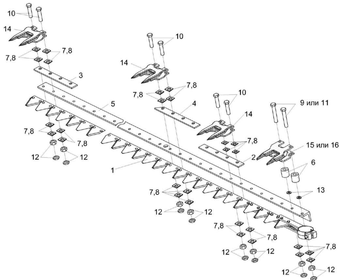
Рисунок 4 – Аппарат режущий КЗК-1492-1547000
