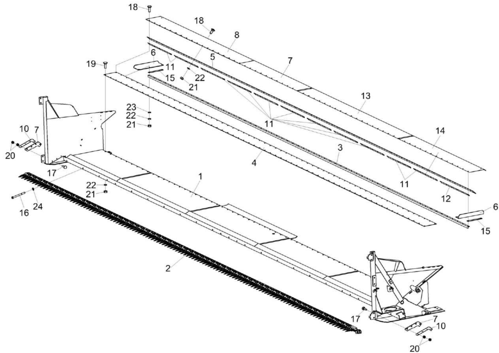
Рисунок 2 – Приспособление для уборки рапса КЗК-1492-1540000 (лист 2)
