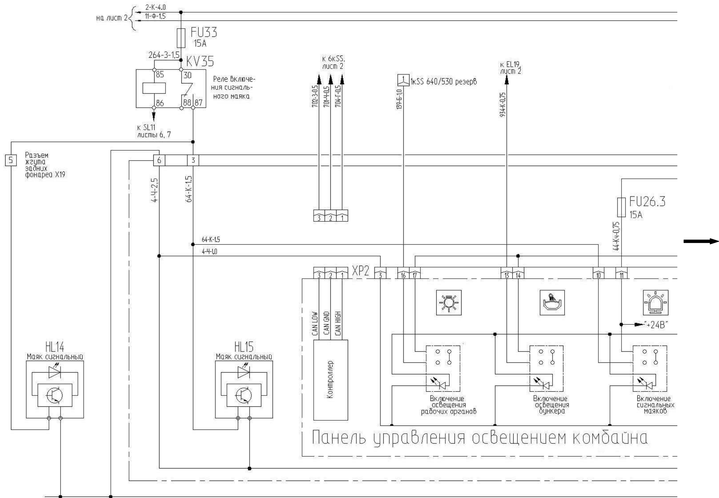
Рисунок Б.3 – Схема электрическая принципиальная комбайна (лист 3.1)
