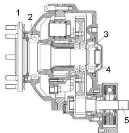
Рисунок 2.19 – Редуктор бортовой
