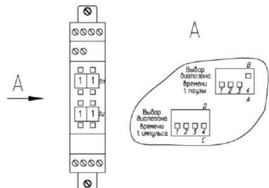
Рисунок 1.30 – Реле времени
