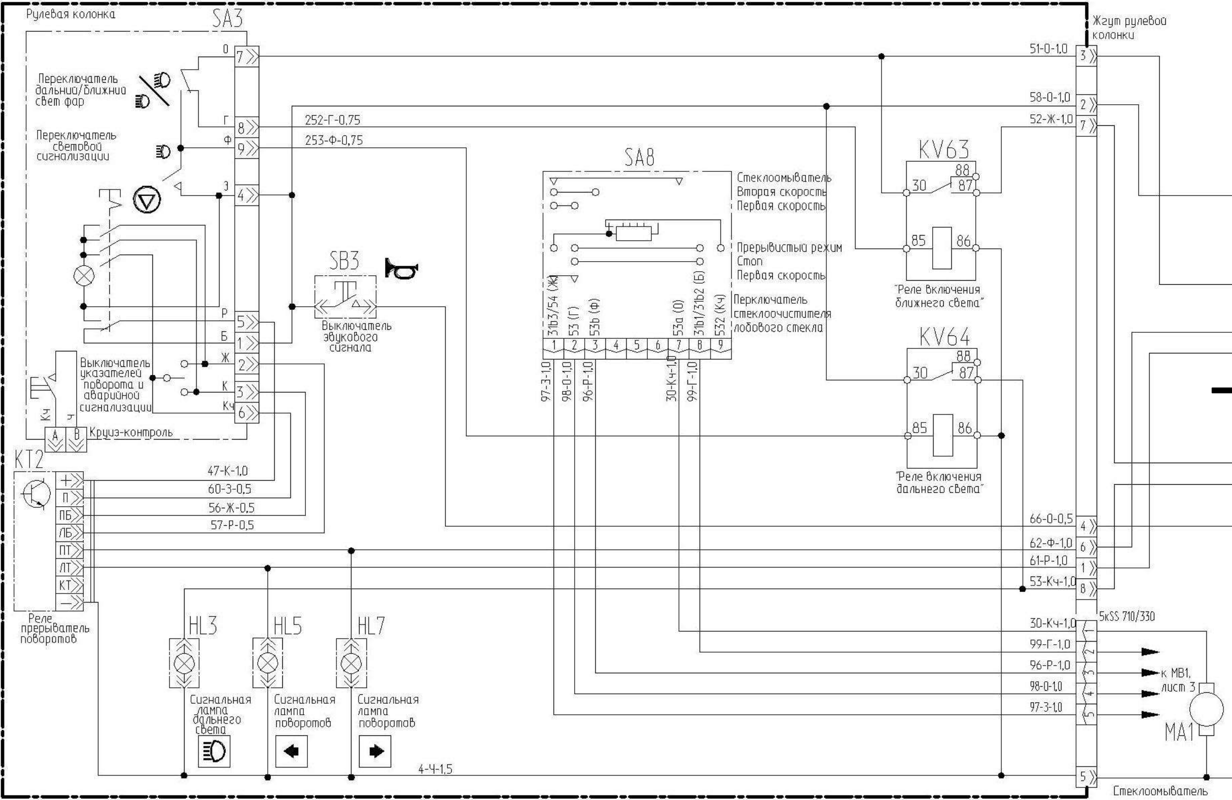
Рисунок Б.2 – Схема электрическая принципиальная комбайна (лист 2.1)
