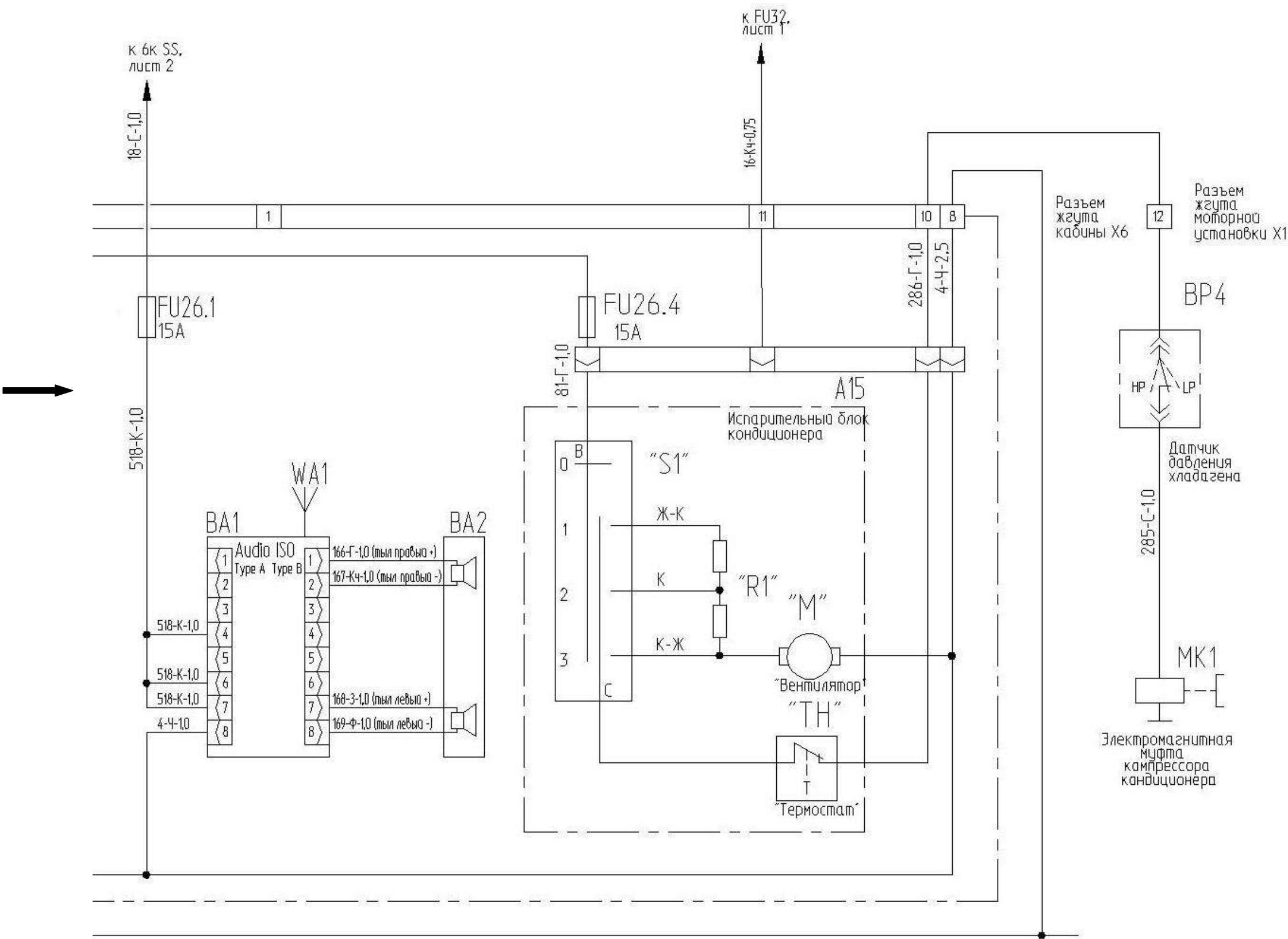
Рисунок Б.3 – Схема электрическая принципиальная комбайна (лист 3.4)
