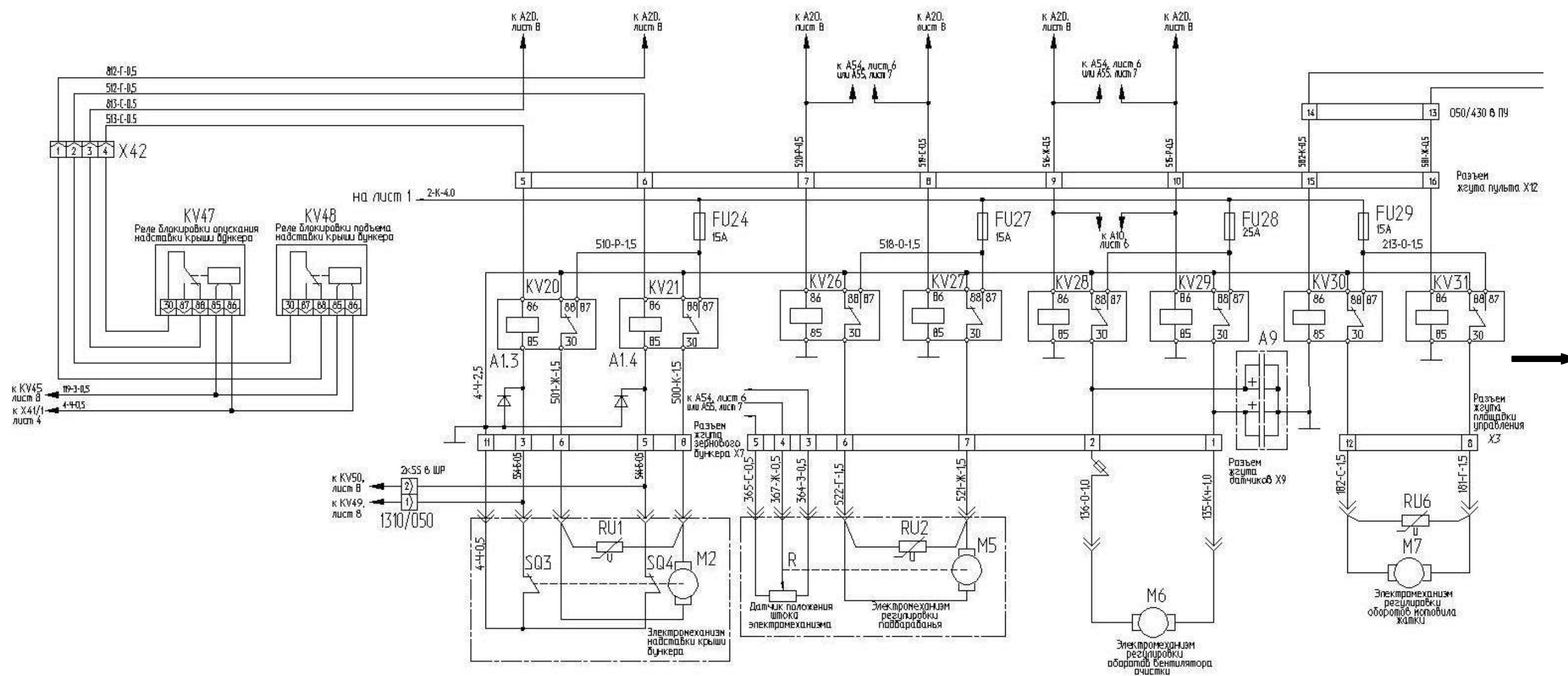
Рисунок Б.5 – Схема электрическая принципиальная комбайна (лист 5.1)
