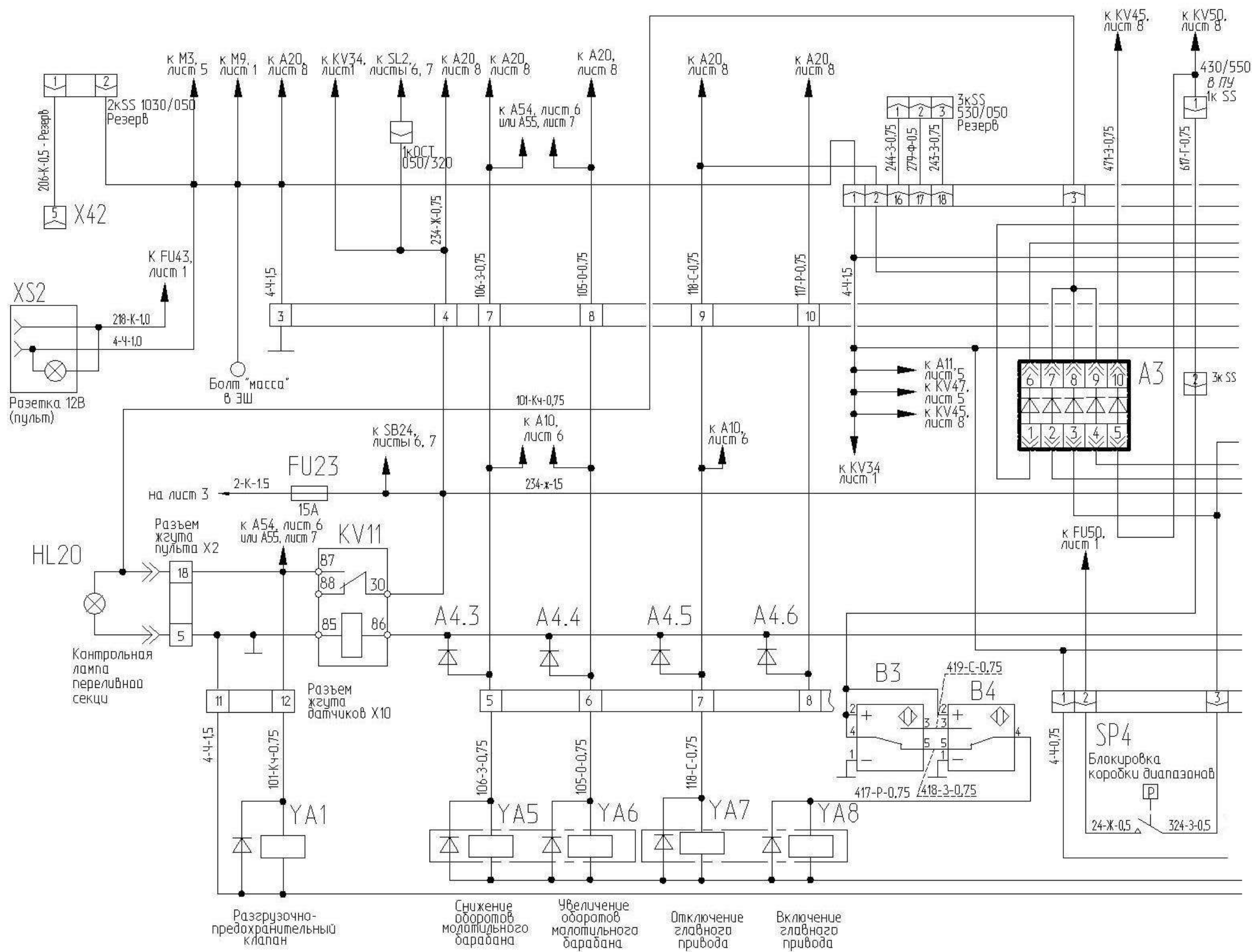
Рисунок Б.4 – Схема электрическая принципиальная комбайна (лист 4.1)
