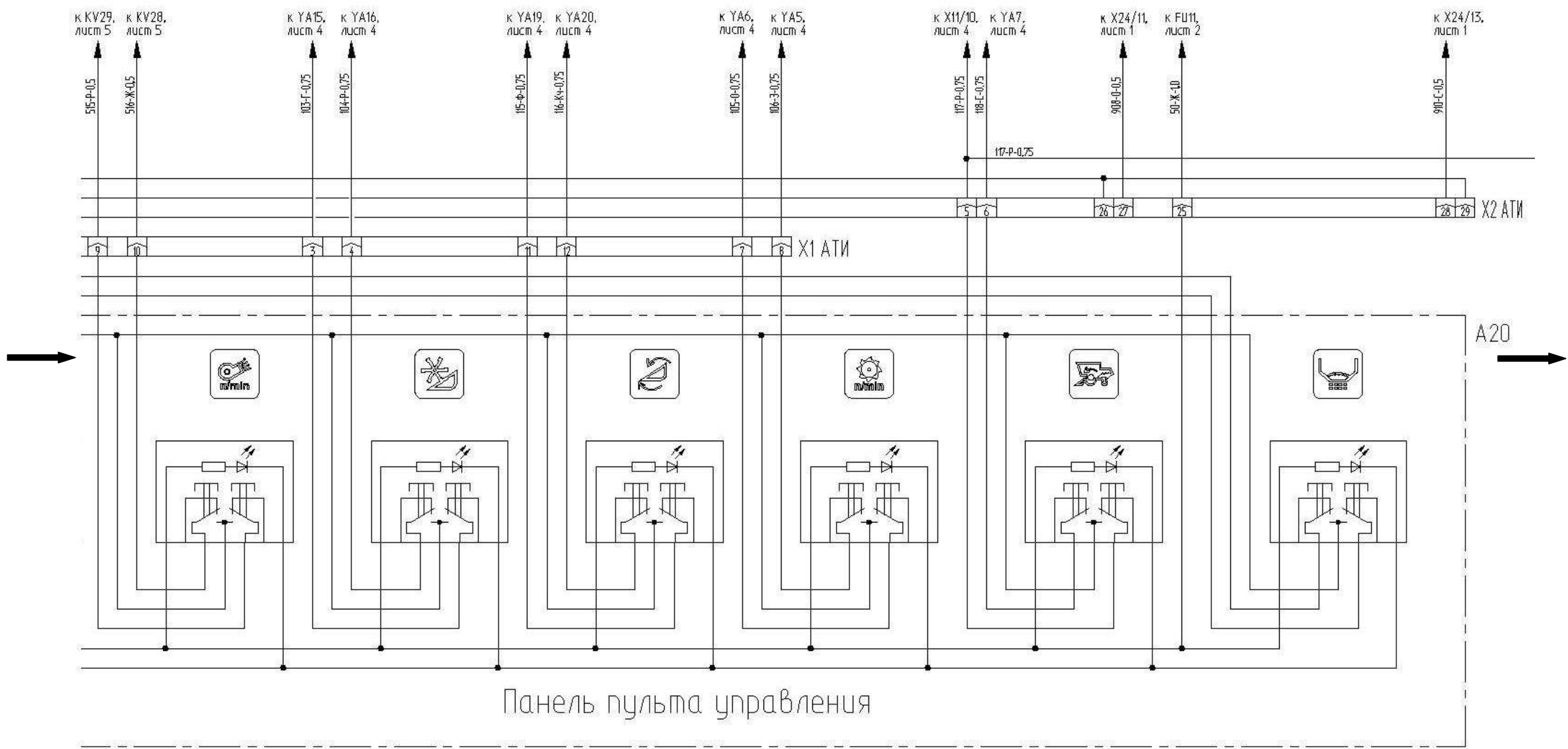
Рисунок Б.8 – Схема электрическая принципиальная комбайна (лист 8.2)
