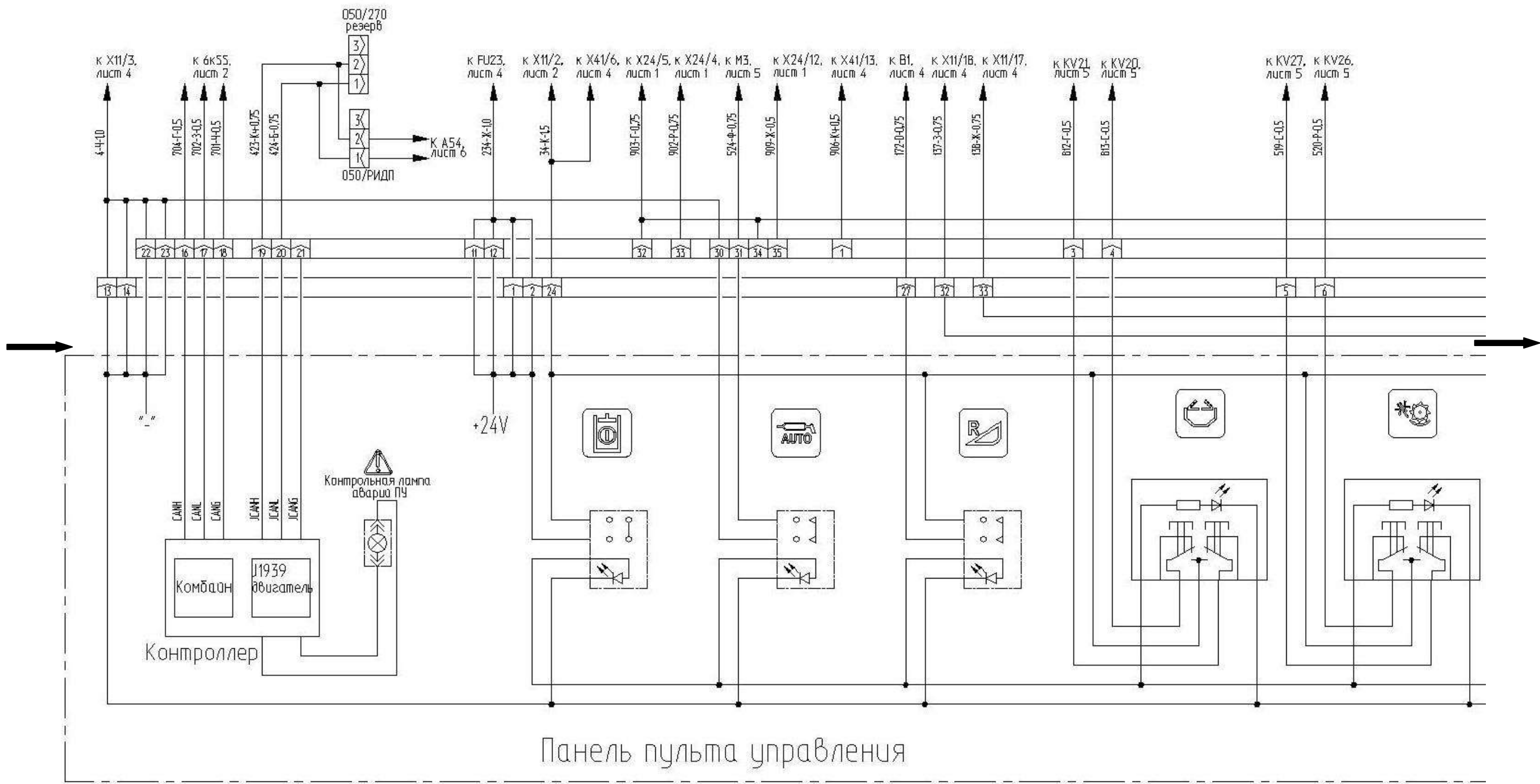
Рисунок Б.8 – Схема электрическая принципиальная комбайна (лист 8.1)
