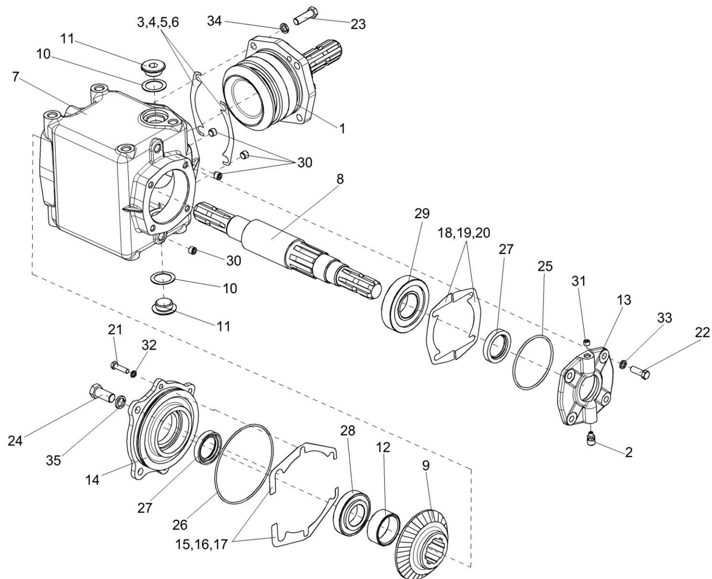
Рисунок 37 – Редуктор КПР 9303100
