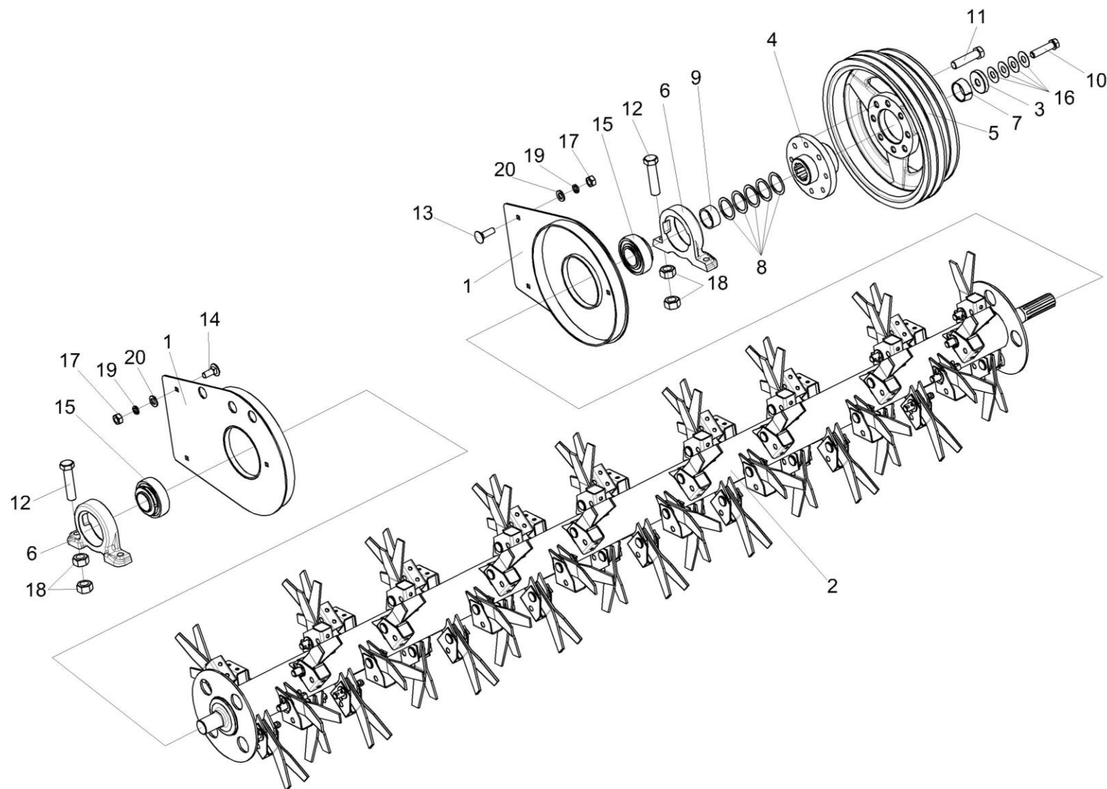
Рисунок 22 – Привод устройства бильного (правой секции) (изображено) Рисунок 23 – Привод устройства бильного (левой секции) (зеркальное отражение)
