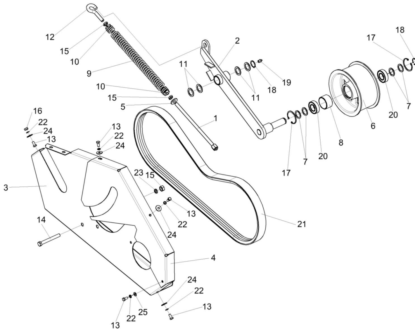
Рисунок 28 – Установка устройства натяжного КПР 9206000А (правой секции) (изображено)
