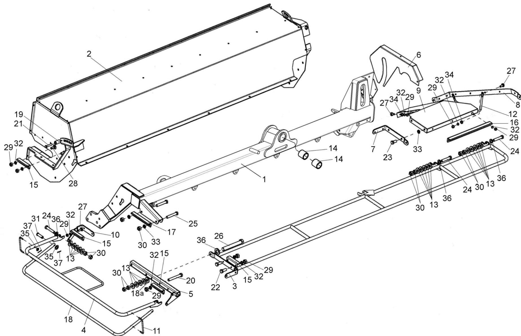
Рисунок 18 – Рама КПР-1-9201000А. Каркас КПР-1-9205000А (правой секции) (изображено)
