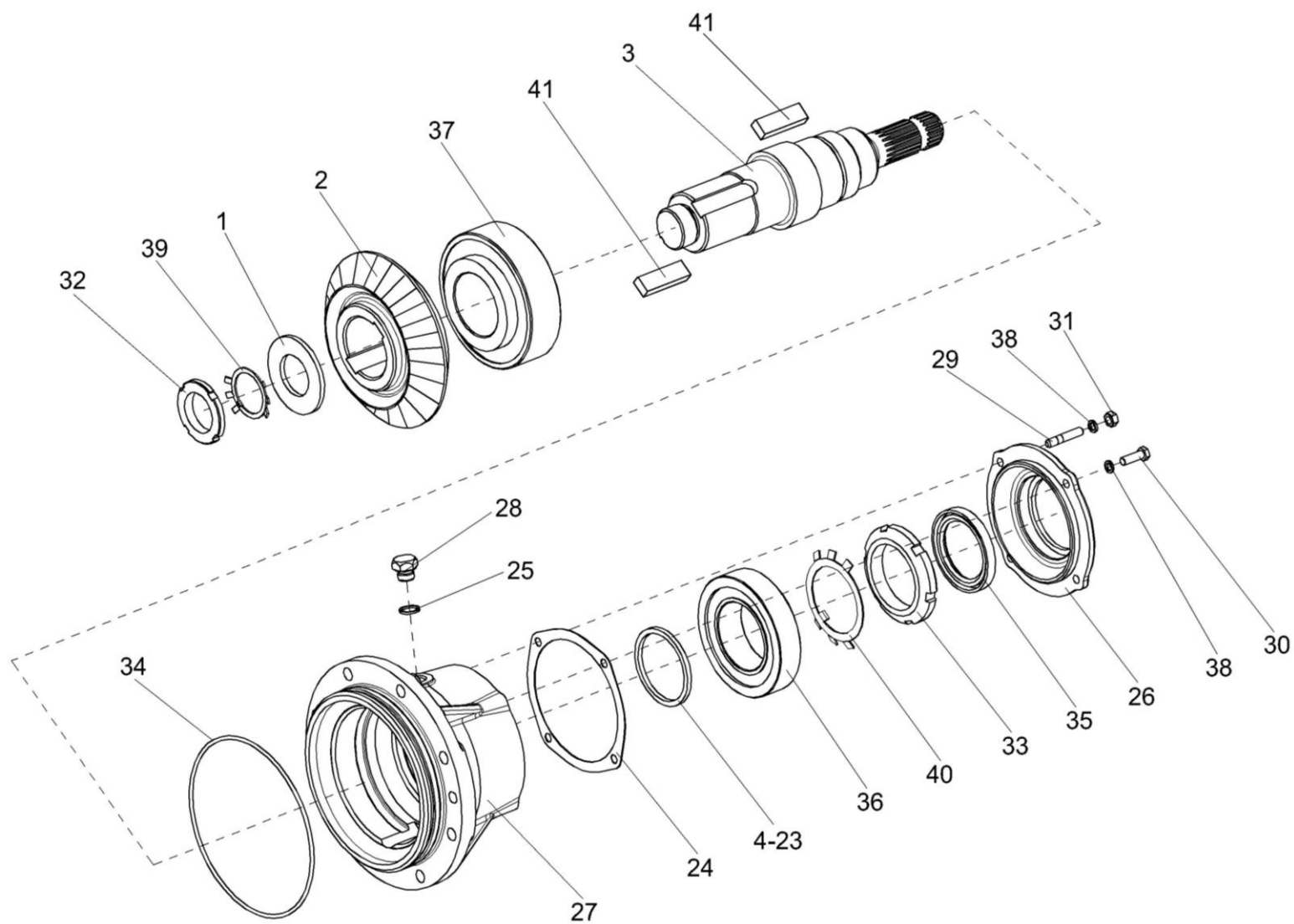
Рисунок 13 – Стакан КПР 9103050
