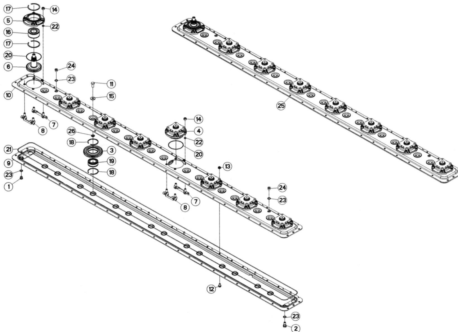
Рисунок А.4 – Резущий брус правый
