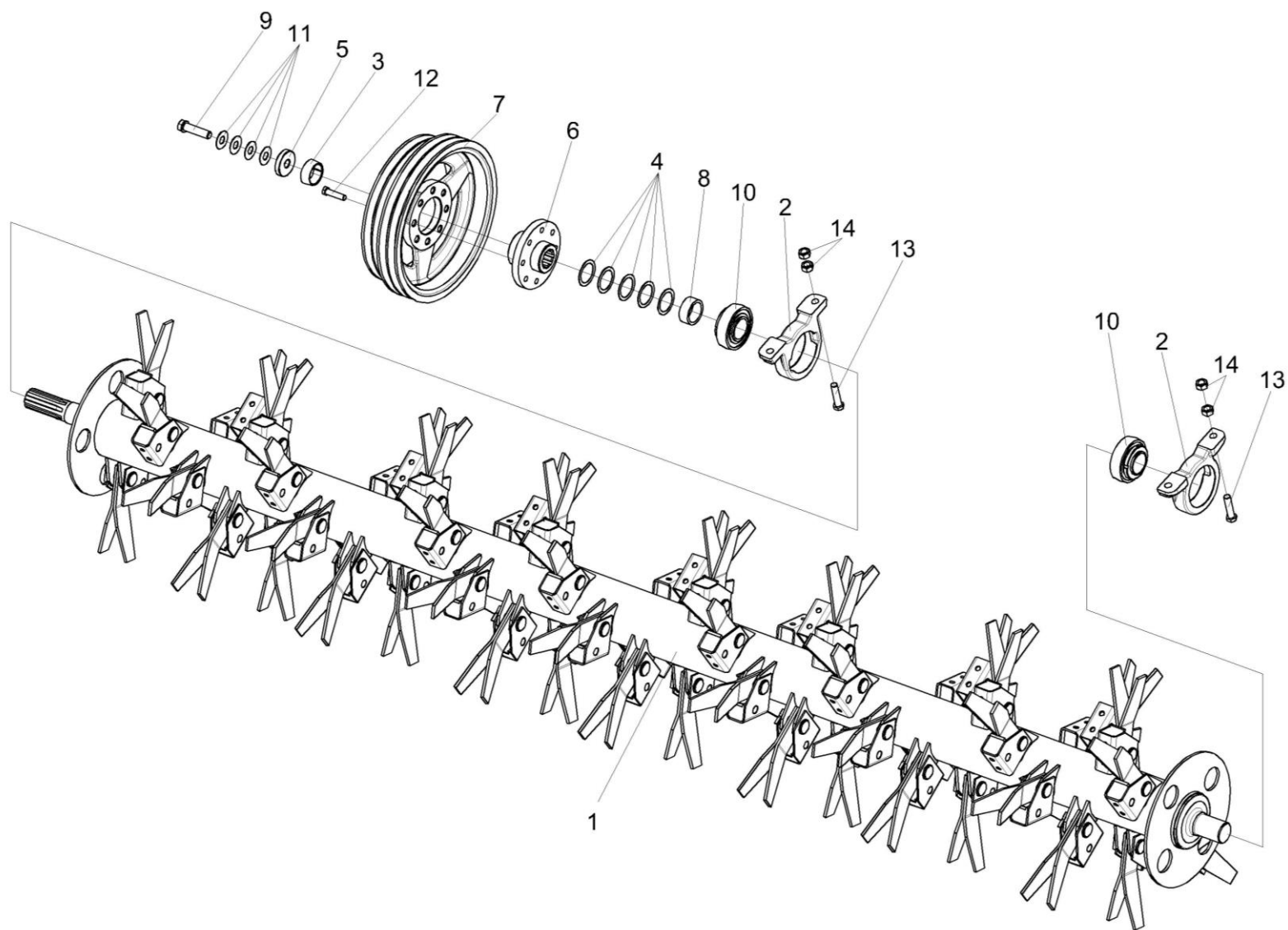
Рисунок 39 – Установка устройства бильного КПР 9202000Б-02 центральной секции
