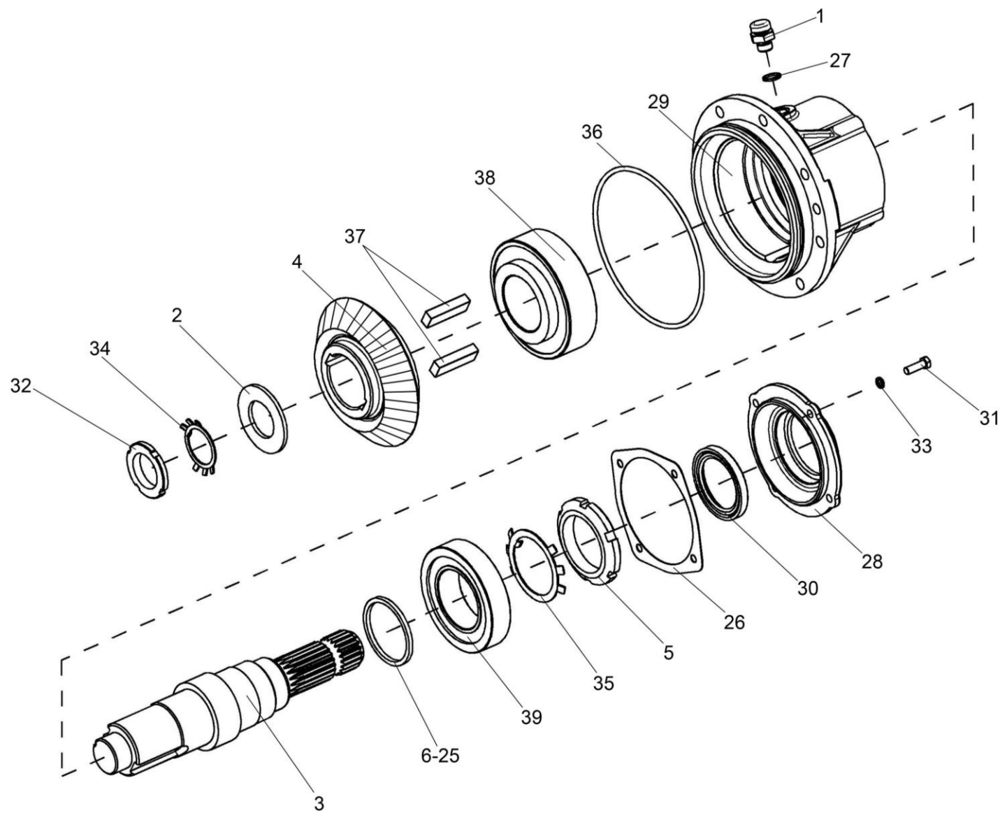
Рисунок 12 – Стакан КПР 9103010
