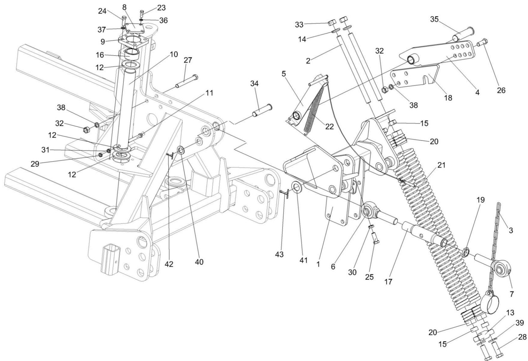
Рисунок 3 – Вывешивание центральной секции
