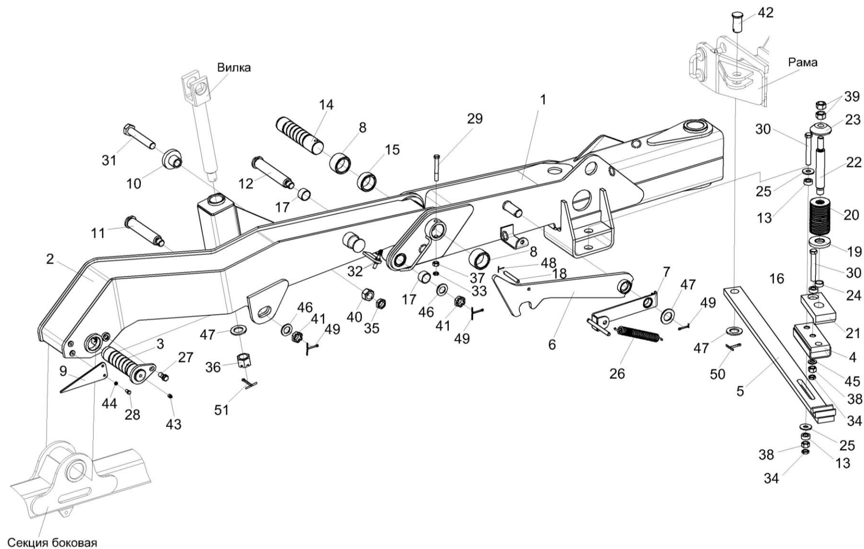
Рисунок 7 – Навеска боковой секции (правой) (изображено)
