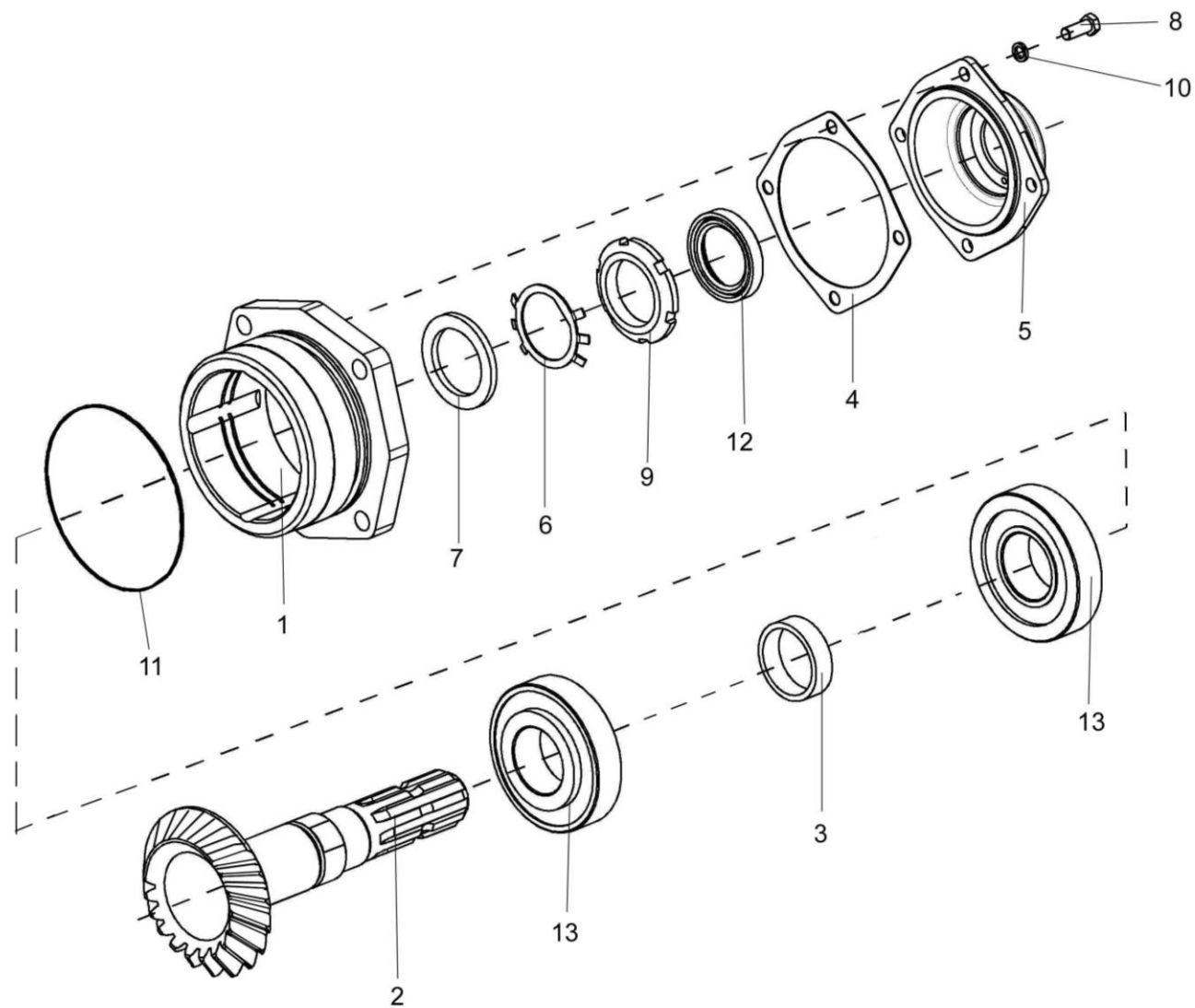
Рисунок 38 – Стакан КПР 9303010
