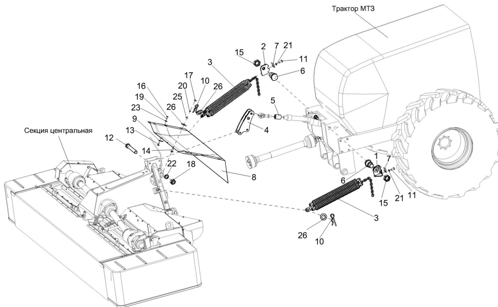
Рисунок 48 – Установка комплекта монтажных частей (для навески центральной секции на трактор)
