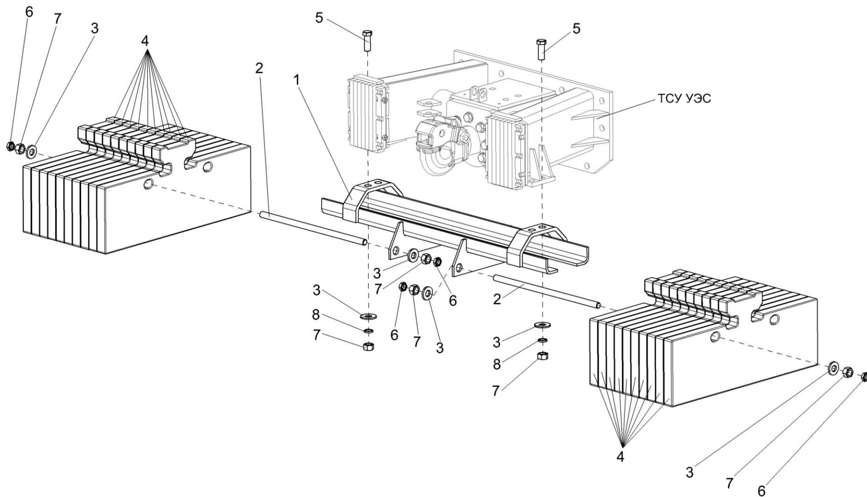
Рисунок 51 – Установка комплекта монтажных частей (установка противовесов на УЭС)
