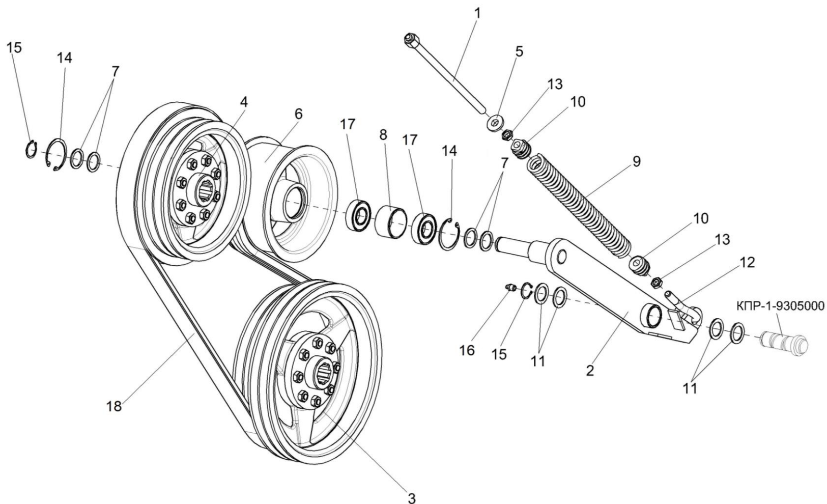
Рисунок 42 – Устройство натяжное центральной секции КПР 9206000А-01
