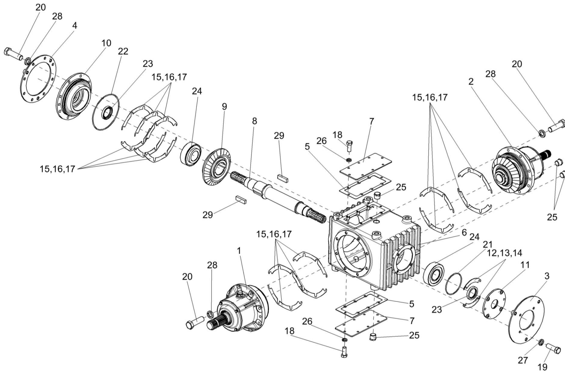
Рисунок 11 – Редуктор КПР 9103100
