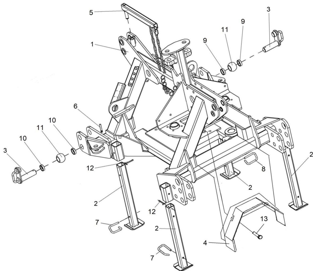
Рисунок 2 – Установка рамы КПР 9101000А
