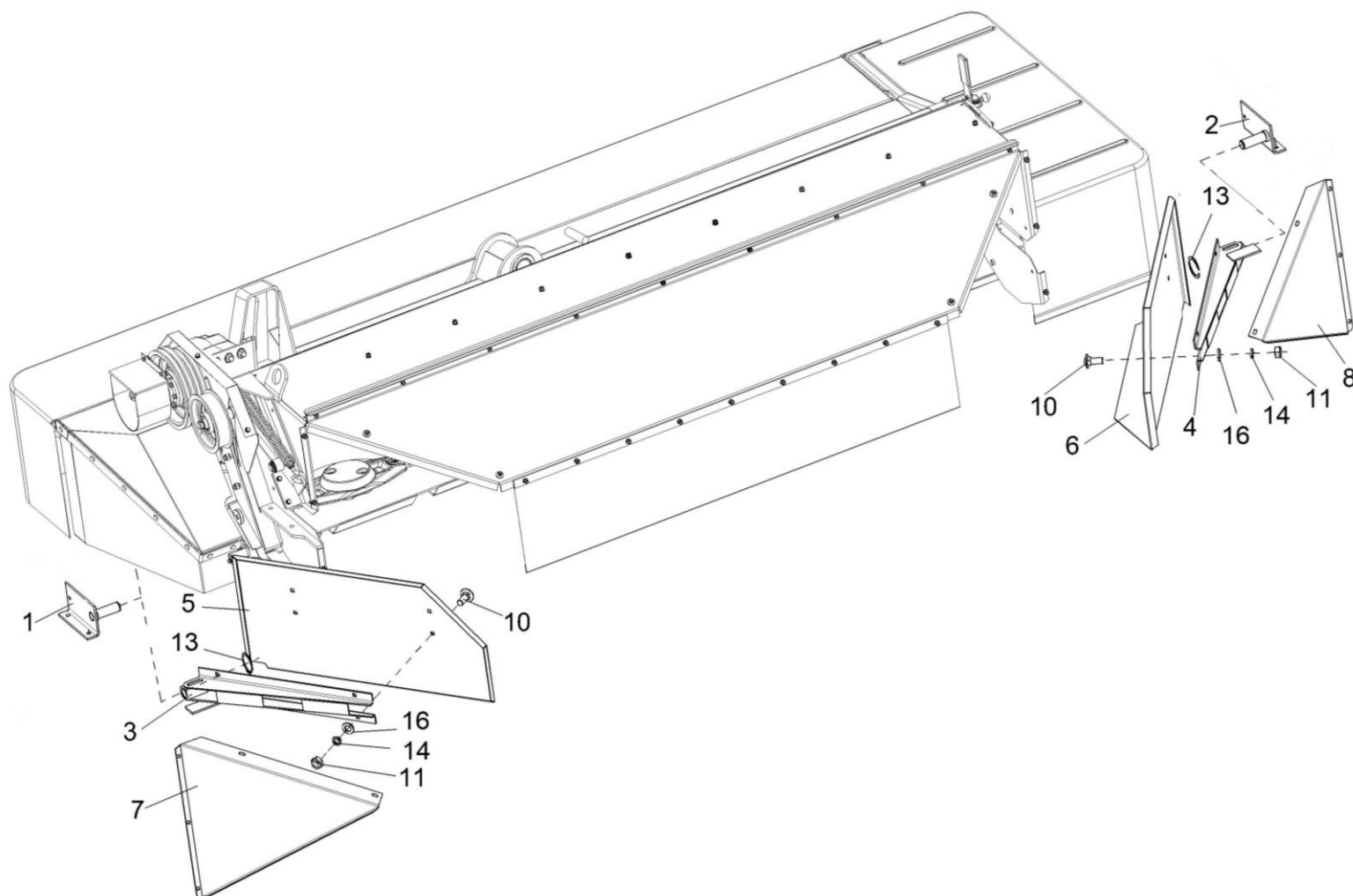
Рисунок 45 – Установка сменных щитков (секция боковая правая) (изображено)
