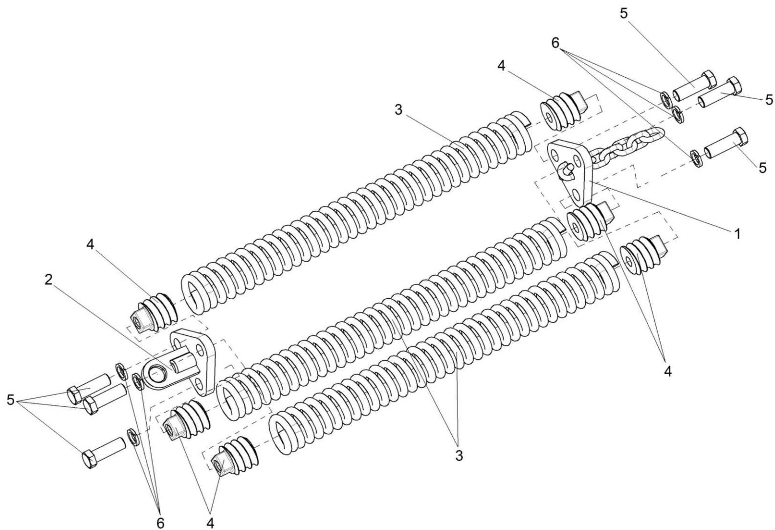
Рисунок 50 – Подвеска КПР-1-9340000А
