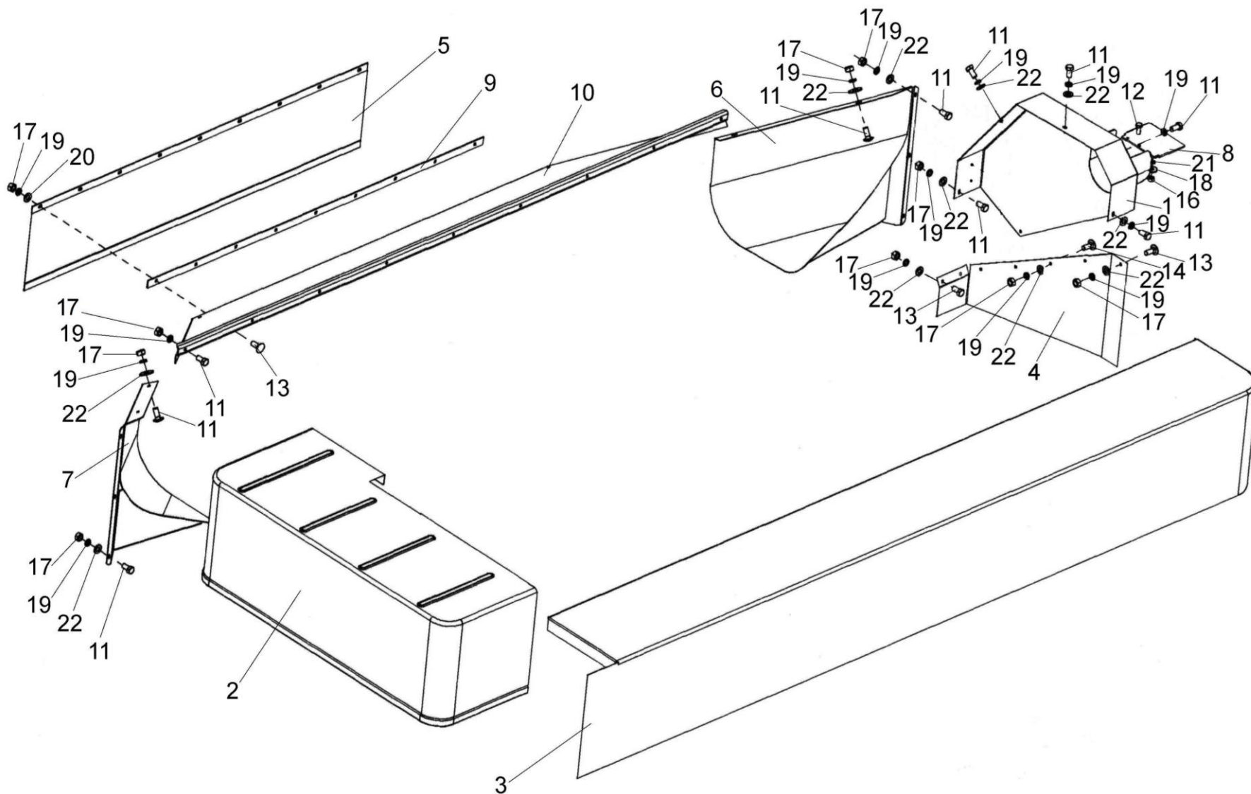
Рисунок 16 – Ограждения и полога боковой секции (правой) (изображено)
