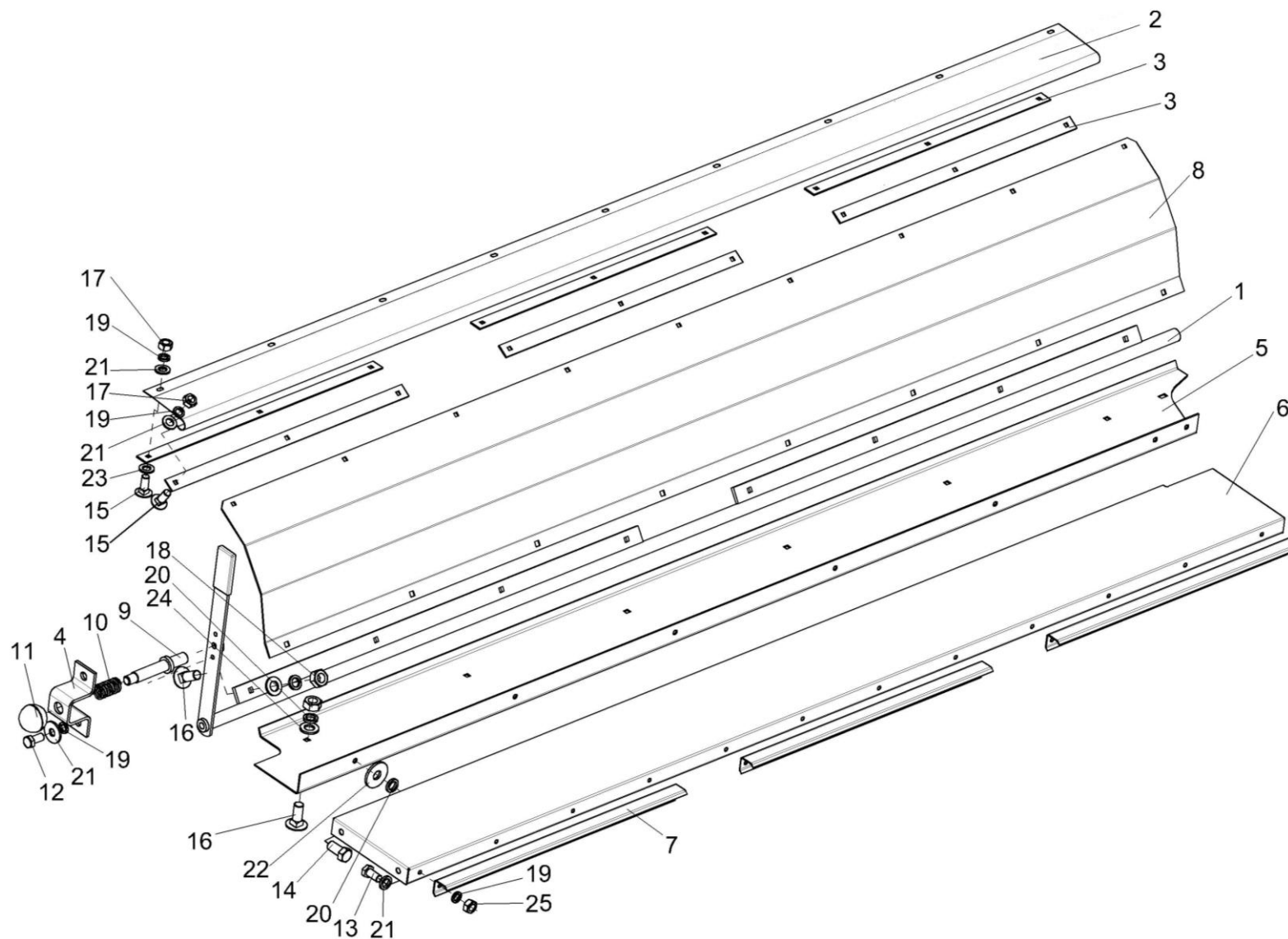
Рисунок 20 – Дека КПР-1-9200416 и рычаг КПР-1-9210000 (правой секции) (изображено)
