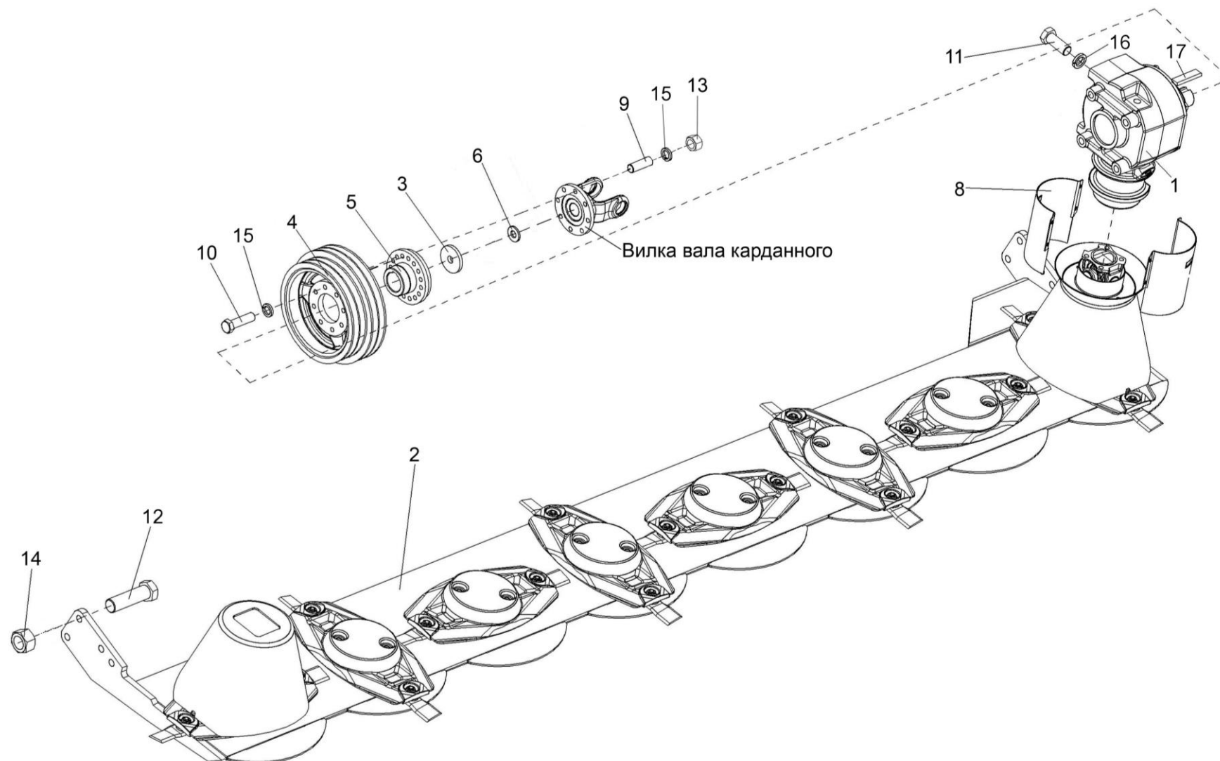
Рисунок 26 – Привод режущего аппарата (правой секции) (изображено)
