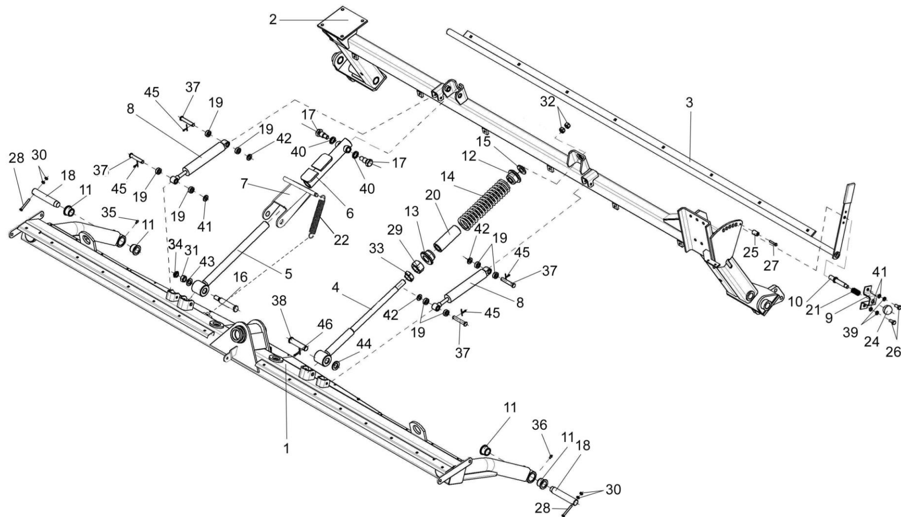
Рисунок 32 – Установка коромысла КПР-1-9304000 и рамы КПР-1-9308000
