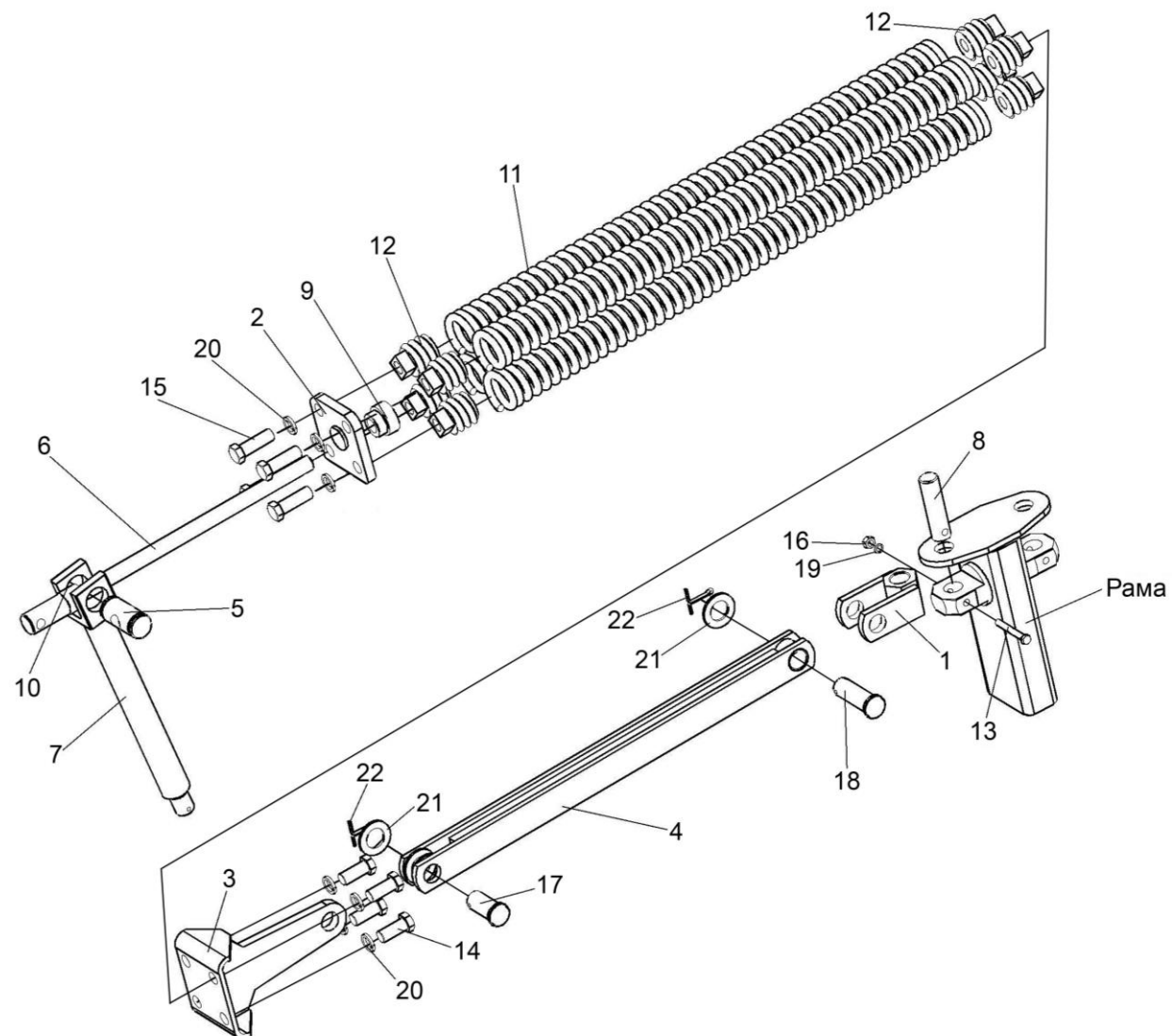
Рисунок 5 – Вывешивание боковой секции (правой) (изображено)
