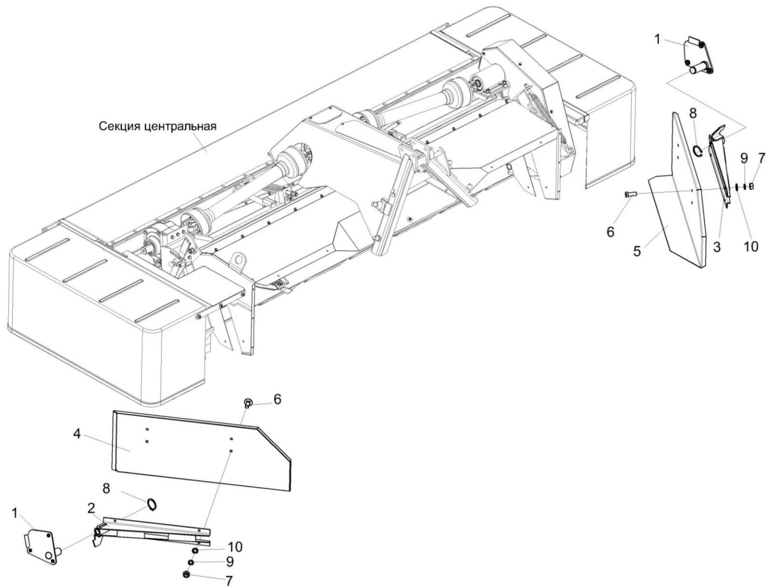
Рисунок 47 – Установка сменных щитков (секция центральная)
