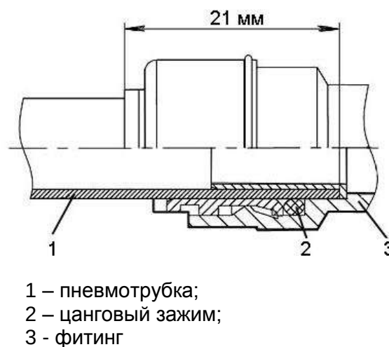
Рисунок 3.8 – Фитинг «цангового» типа
