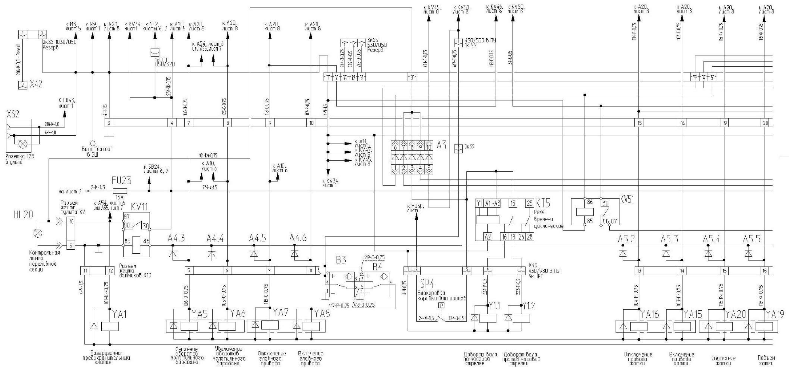
Рисунок Б.4 – Схема электрическая принципиальная комбайна (лист 4.1)
