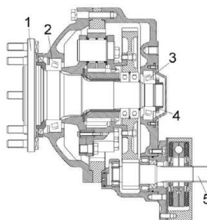
Рисунок 2.18 – Редуктор бортовой
