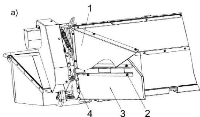
а) боковая секция;
