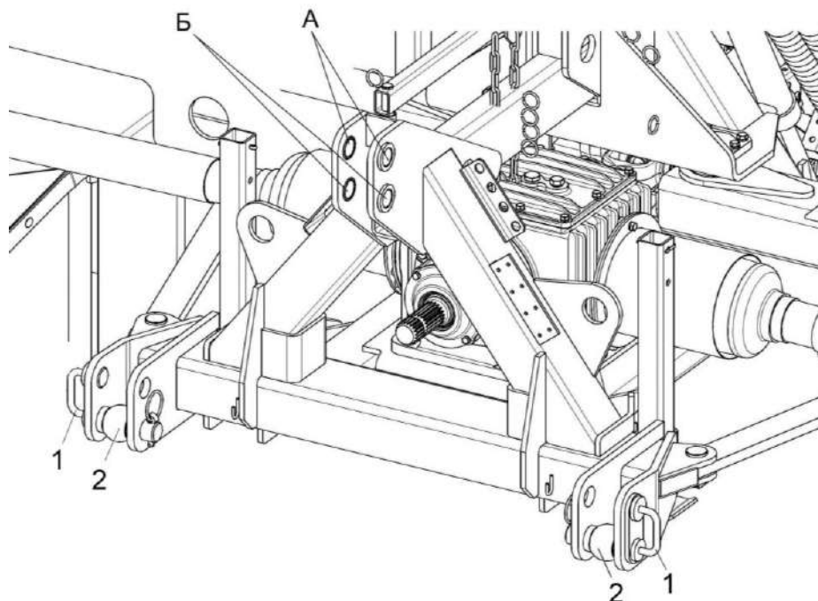
1 – фиксаторы; 2 – шаровые опоры
