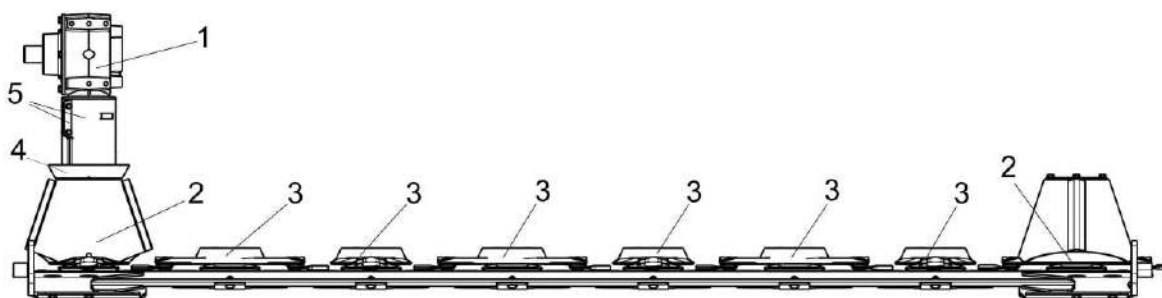
1 – конический редуктор; 2 – диски с конусом; 3 – плоские диски; 4 – конусная крышка; 5 – щитки
