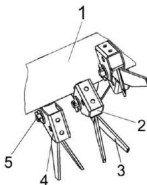
1 – вал; 2 – демпфер; 3 – бич; 4 – корпус; 5 – ось со шплинтом
