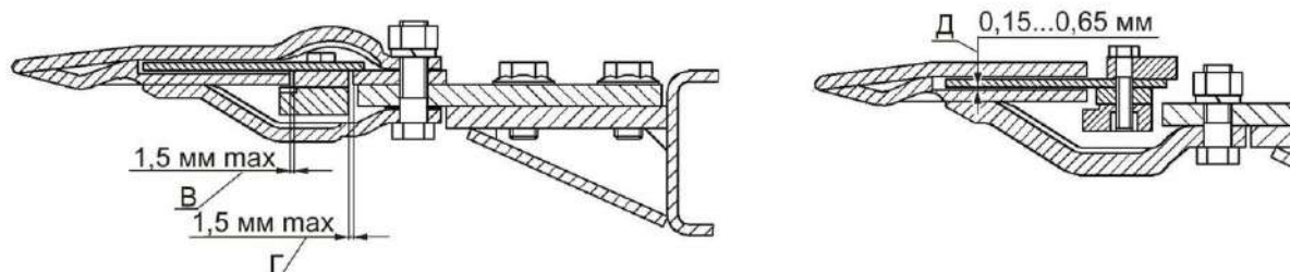
Рисунок 2.12 – Режущий аппарата
