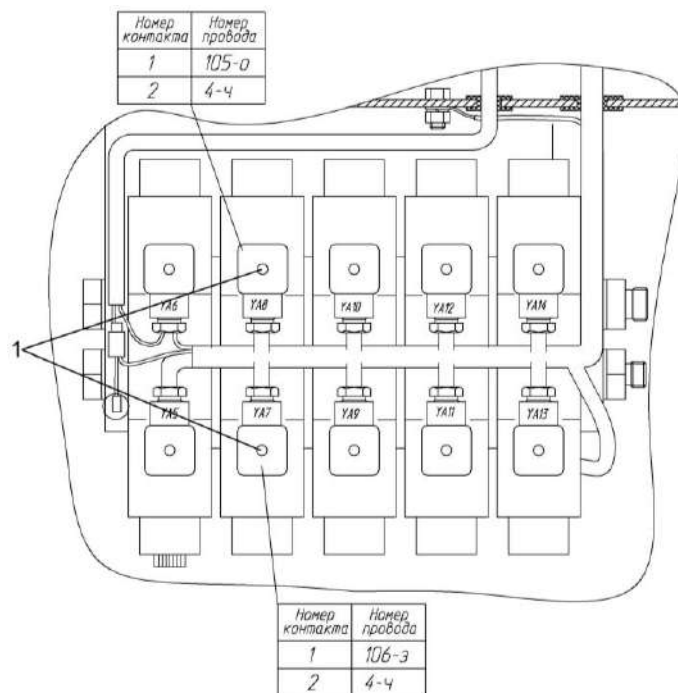
Рисунок 2.5 – Гидроблок
