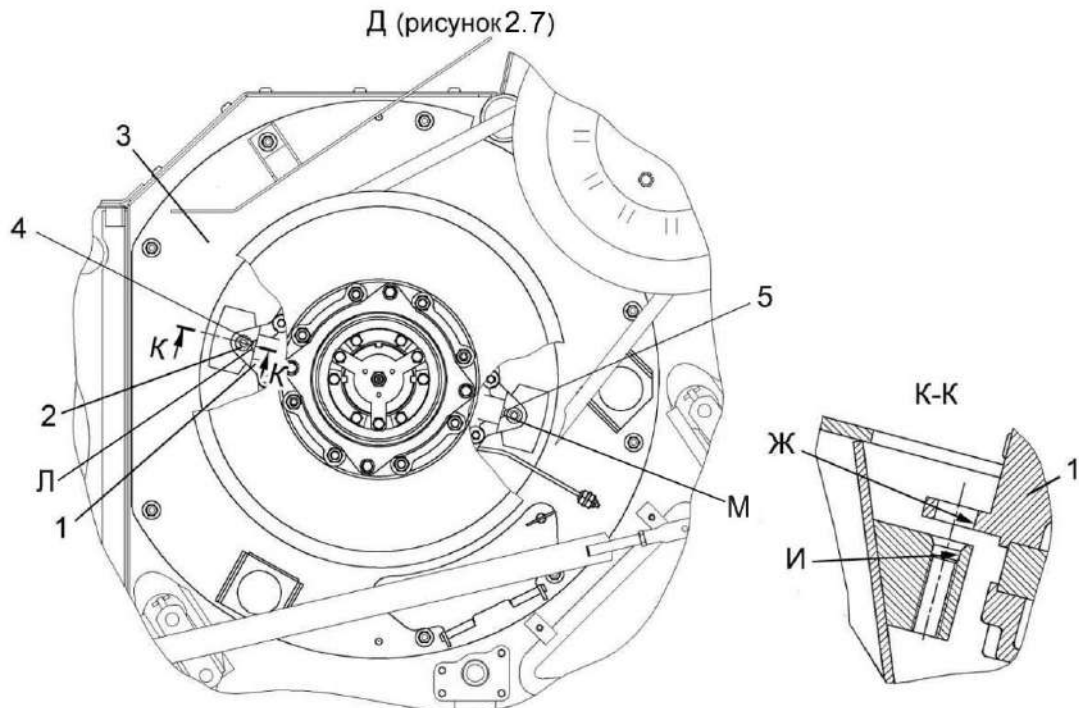
Рисунок 2.9 – Разблокировка понижающего редуктора
