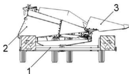
Рисунок 1.10 – Жатка, установленная на тележке
