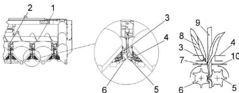
Рисунок 1.11 – Схема технологического процесса работы комбайна с комплектом
