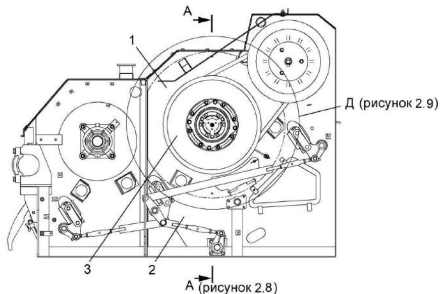
Рисунок 2.7 – Аппарат молотильный
