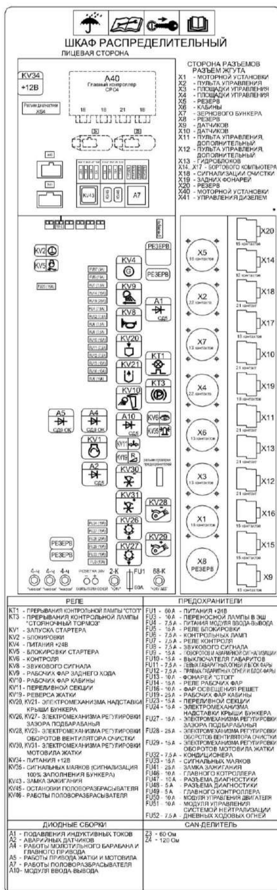
Рисунок 1.24 – Шкаф электрический
