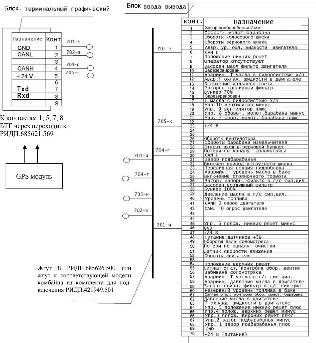
Рисунок 1.79 – Схема подключения БТГ, БВВ и GPS модуля комбайна
