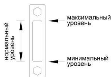
Рисунок 2.7 - Маслоуказатель
