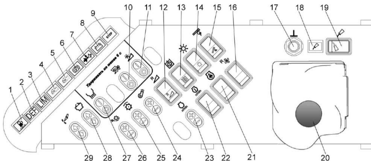
Рисунок 1.27 – Пульт управления комбайна
