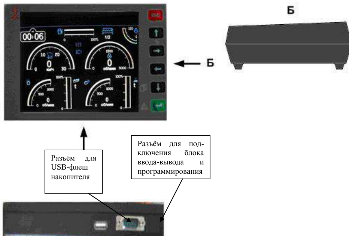
Рисунок 1.33 – Внешний вид лицевой панели БТГ
