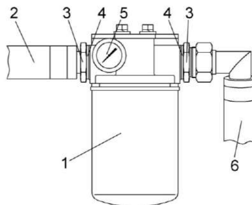
Рисунок 1.20 – Гидросистема привода ходовой части
