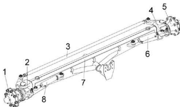
Рисунок 1.9 – Шасси
