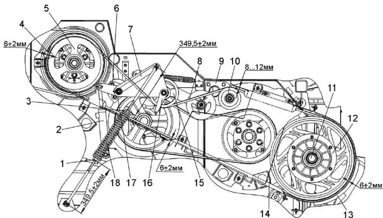
1, 3, 6 – гайки; 2 – гидроцилиндр; 4, 13, 14 – щитки; 5, 12 – шкивы; 7 – рычаг; 8 – ремень; 9, 17 – опоры; 10, 15 – ролики; 11 – вал; 16 – кронштейн; 18 – пружина;
