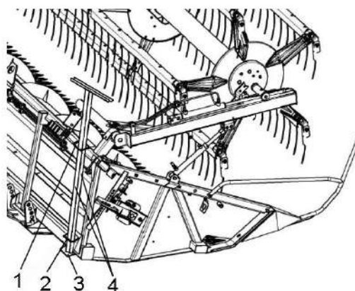
1- верхняя скоба; 2 - нижняя скоба; 3 - площадка; 4 - швабры
