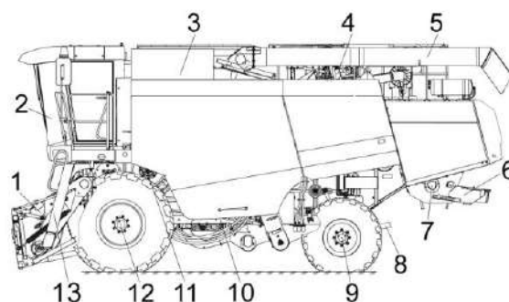
1 – наклонная камера; 2 – кабина; 3 – бункер зерновой; 4 – установка двигателя; 5 – шнек выгрузной; 6 – дефлектор; 7 – соломоизмельчитель; 8 – половоразбрасыватель; 9 – мост управляемых колес; 10 – очистка; 11 – молотильный аппарат; 12 – мост ведущих колес; 13 – трап
