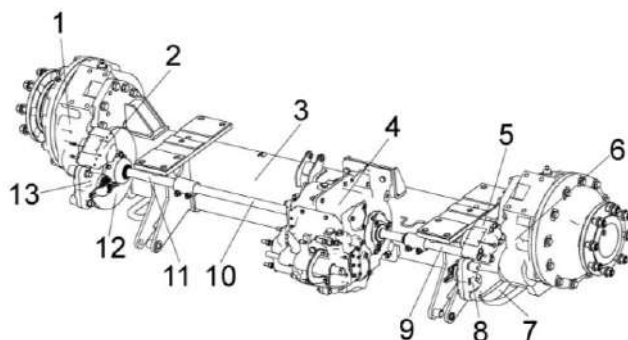
Рисунок 1.10 – Мост управляемых колес.
