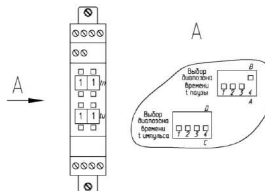
Рисунок 1.35 – Реле времени
