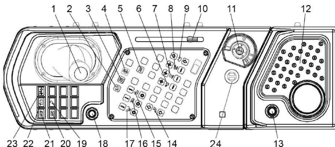
Рисунок 1.36 – Пульт управления комбайна
