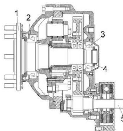
Рисунок 2.20 – Редуктор бортовой
