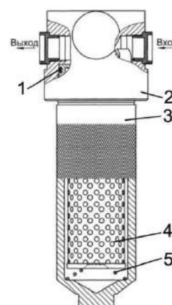
Рисунок 3.10 – Сливной фильтроэлемент, демонтируемый при помощи ключа фильтра
