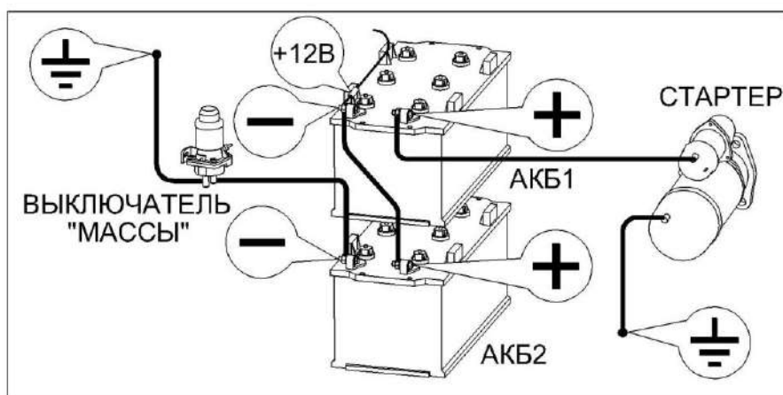
Рисунок 2.4 - Подключение аккумуляторных батарей
