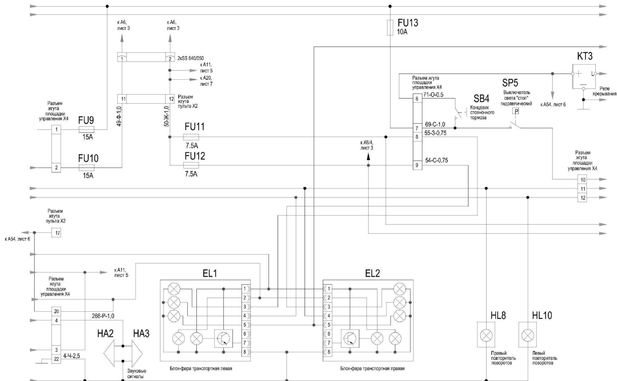
Рисунок Б.2 – Схема электрическая принципиальная комбайна (лист 2.2)
