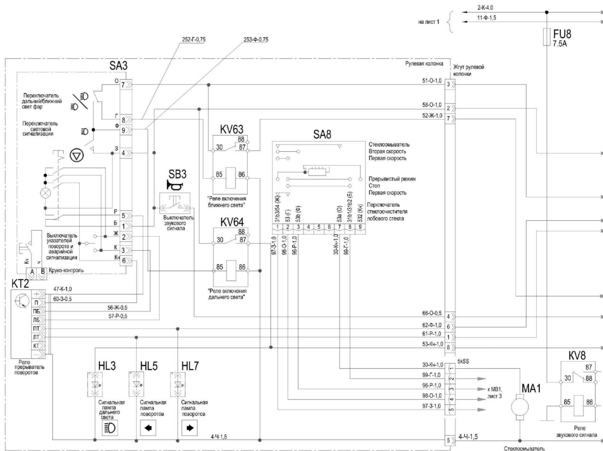
Рисунок Б.2 – Схема электрическая принципиальная комбайна (лист 2.1)
