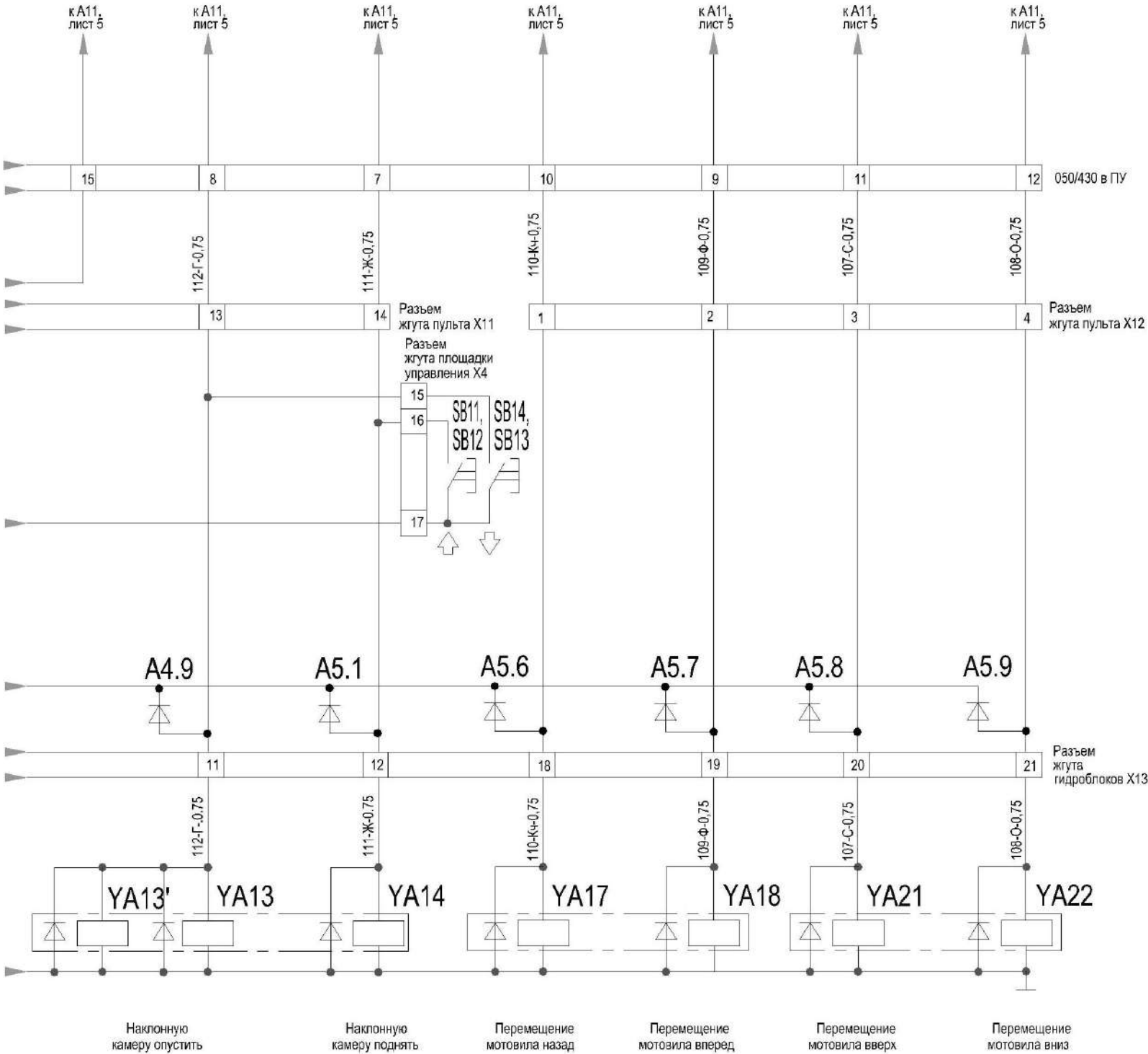
Рисунок Б.4 – Схема электрическая принципиальная комбайна (лист 4.3)
