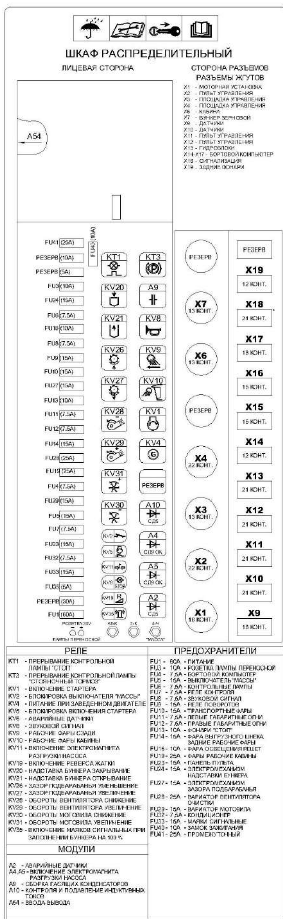
Рисунок 1.25 – Схема соединений шкафа распределительного
