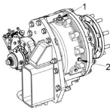
1 – отверстие для заправки; 2 – контрольное отверстие
