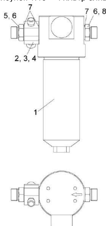
Рисунок 1.19 – Фильтр сливной
