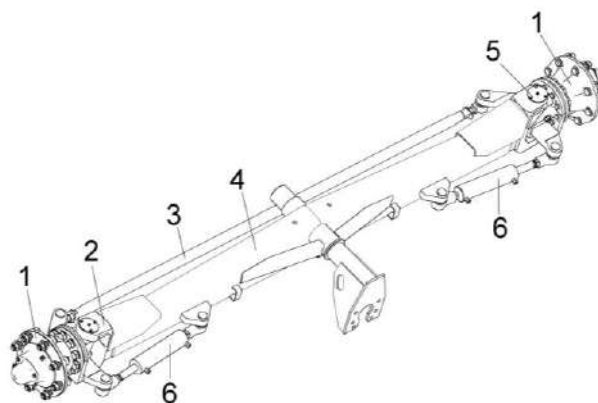
Рисунок 1.8 – Шасси
