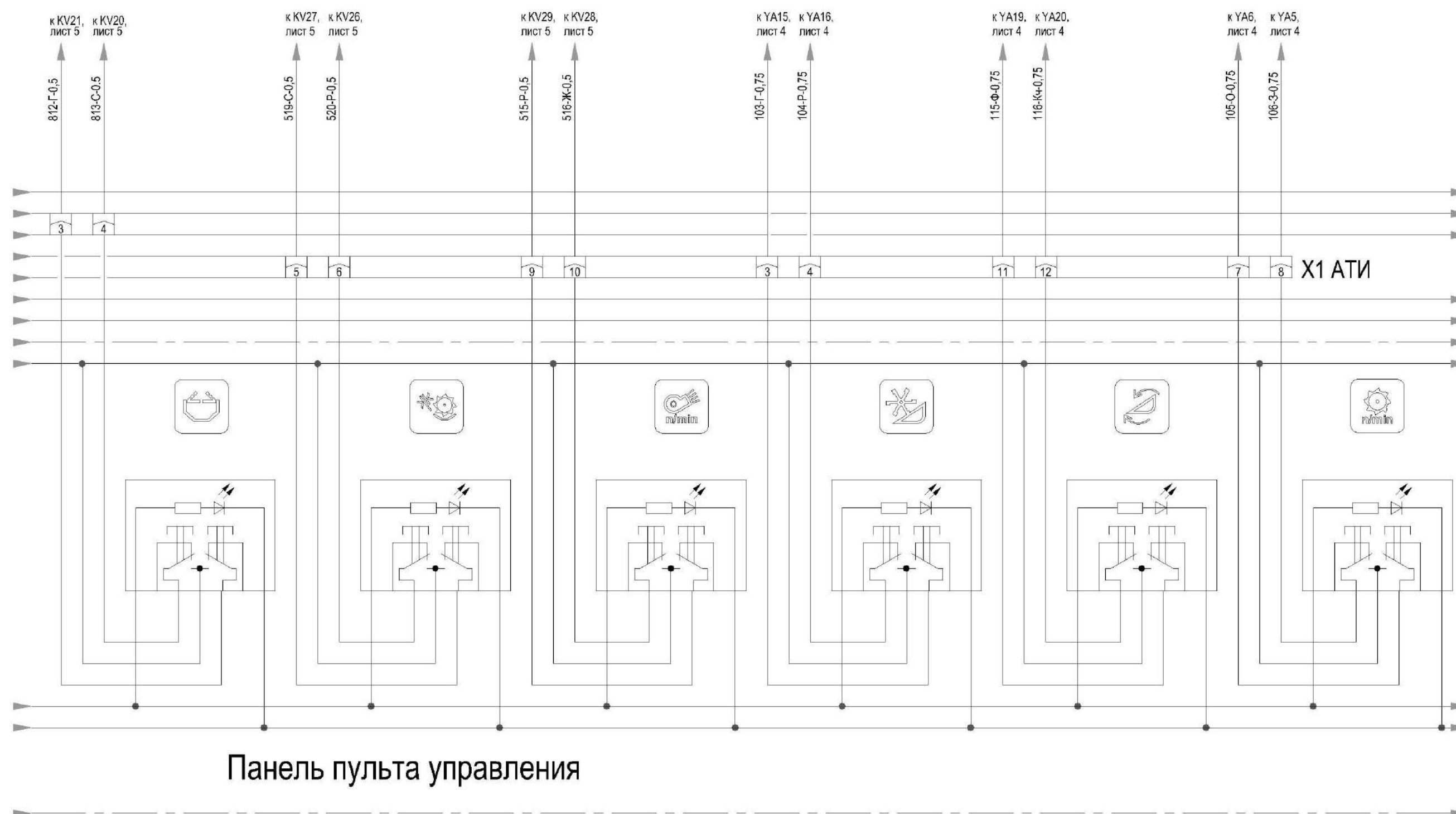
Рисунок Б.7 – Схема электрическая принципиальная комбайна (лист 7.2)
