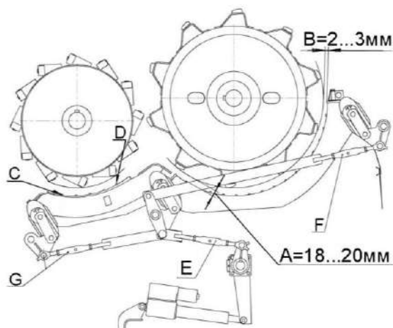
Рисунок 2.12 - Схема молотильного аппарата
