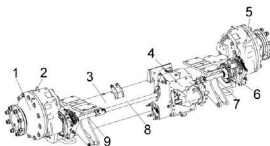
Рисунок 1.9 - Мост управляемых колес.
