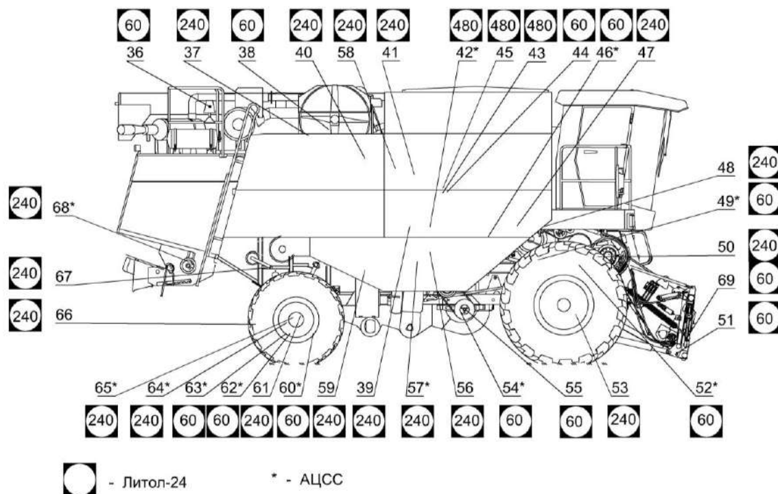
Рисунок 3.2 – Смазка комбайна АЦСС (вид справа)
