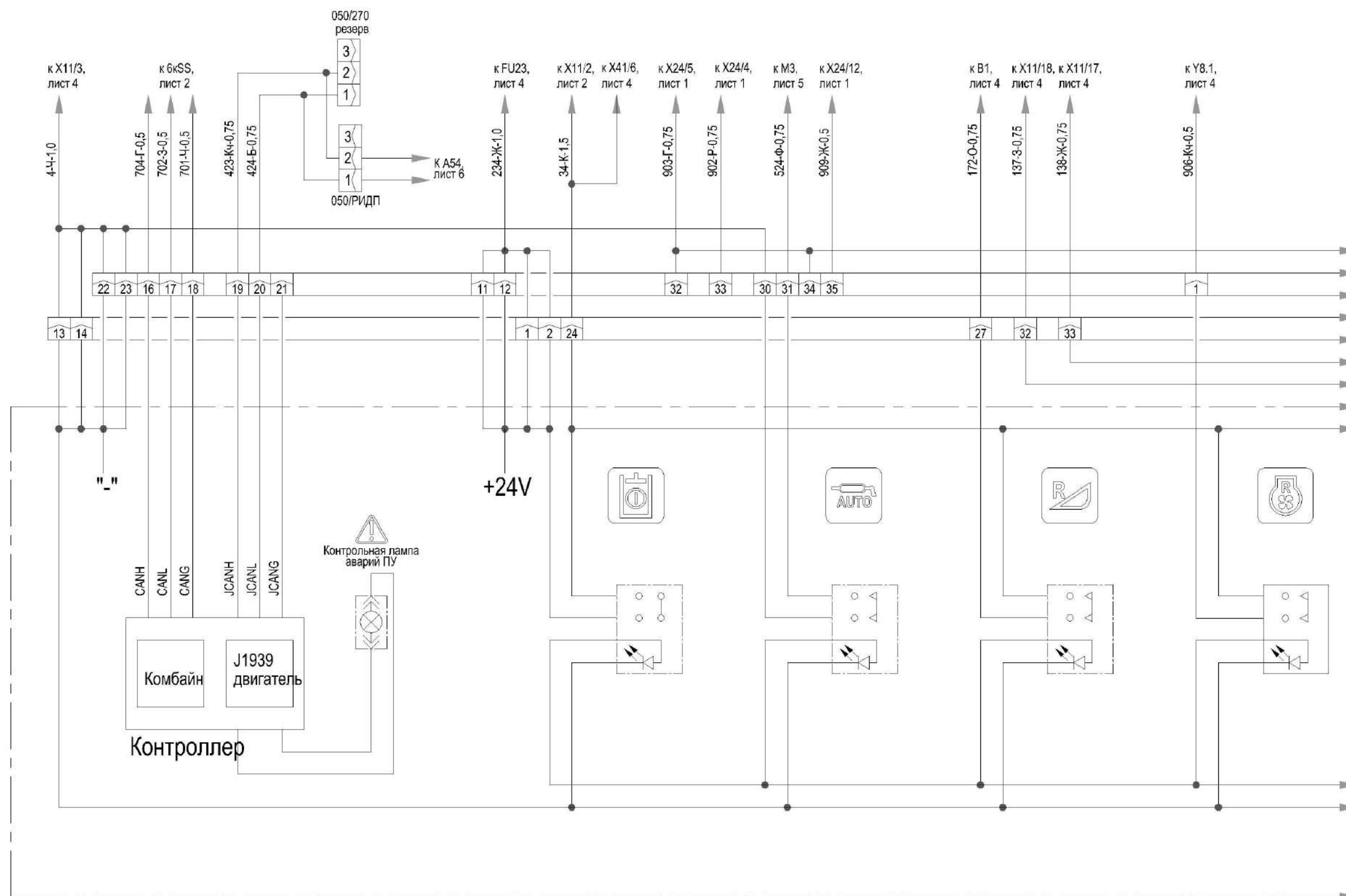
Рисунок Б.7 – Схема электрическая принципиальная комбайна (лист 7.1)
