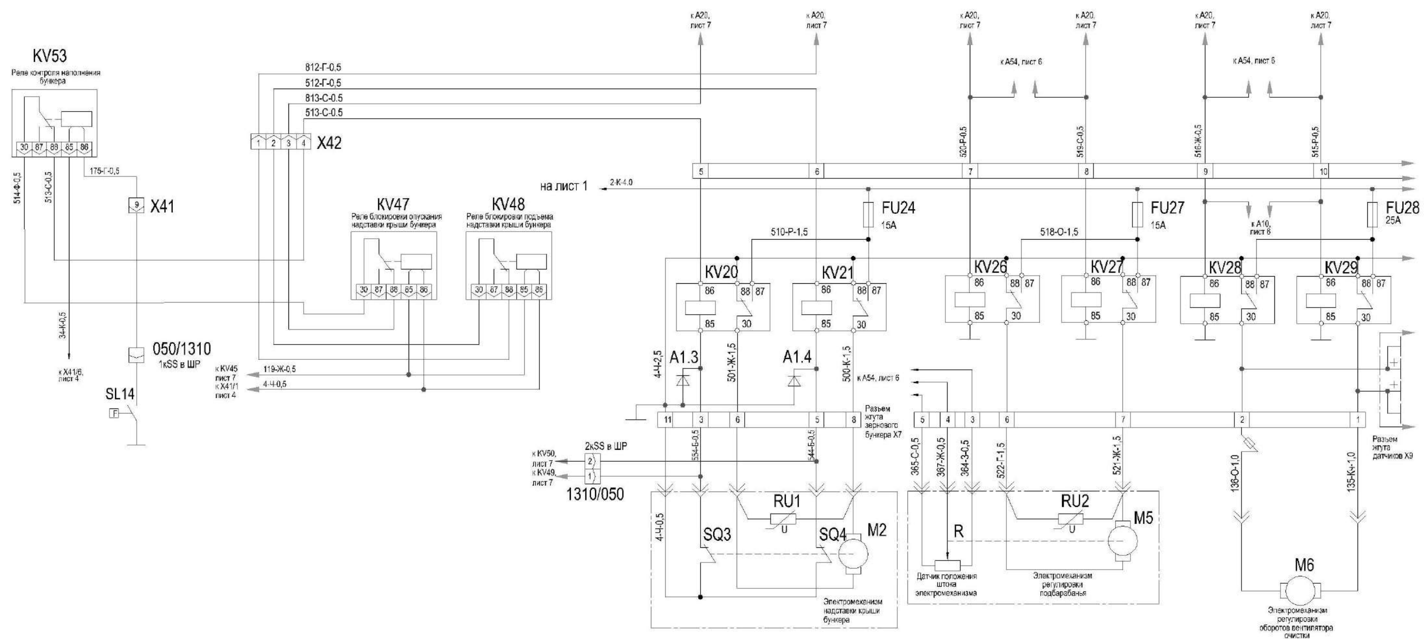
Рисунок Б.5 – Схема электрическая принципиальная комбайна (лист 5.1)
