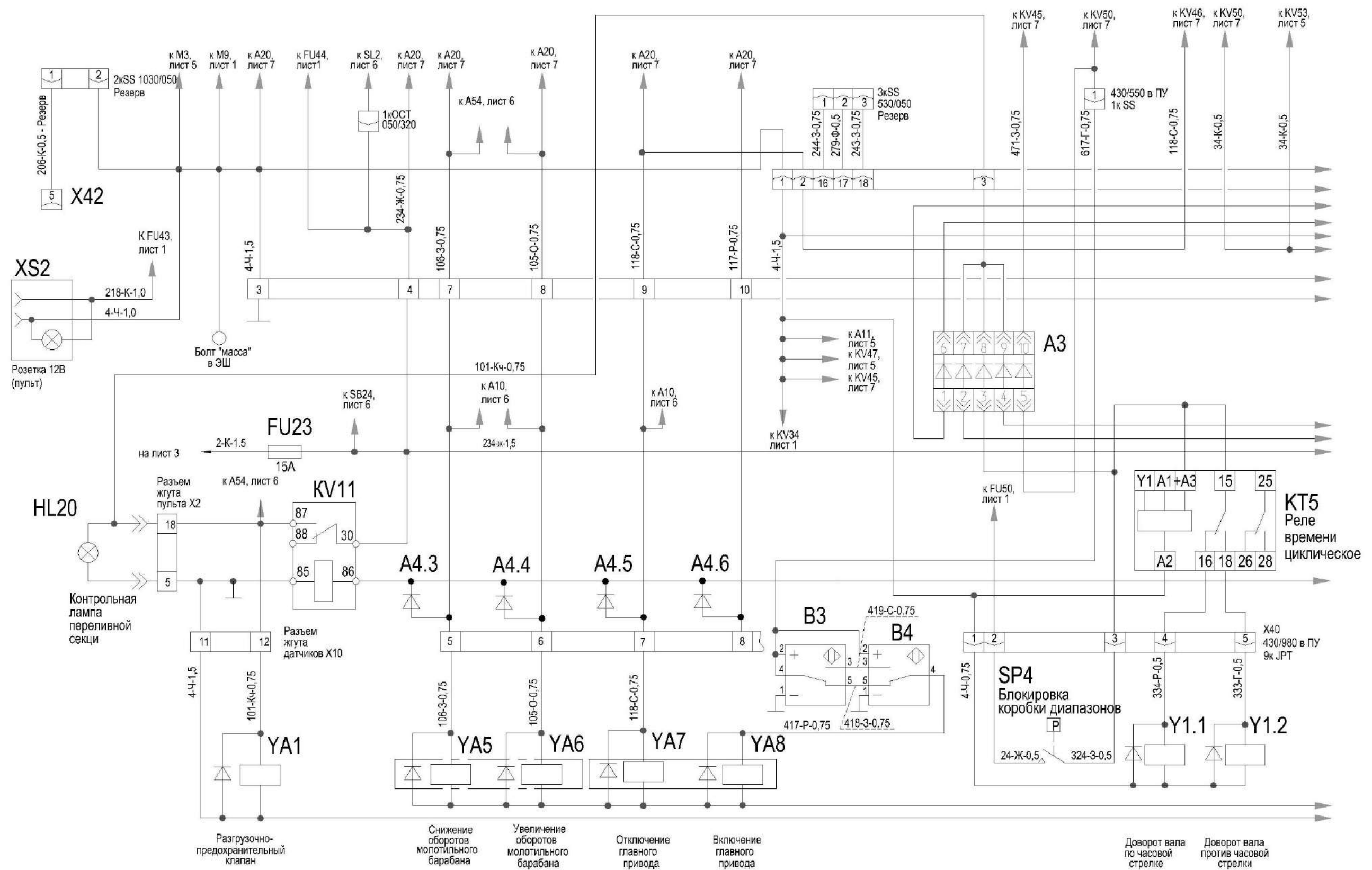
Рисунок Б.4 – Схема электрическая принципиальная комбайна (лист 4.1)
