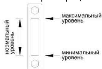
Рисунок 2.7 - Маслоуказатель
