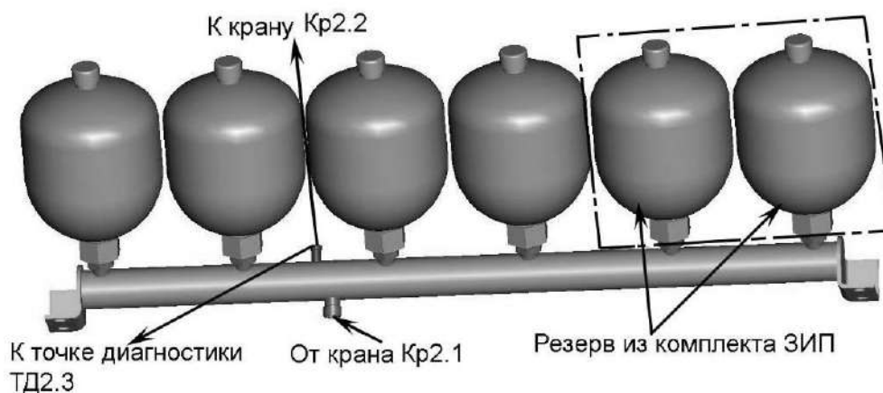
Рисунок 1.32 – Блок пневмогидроаккумуляторов
