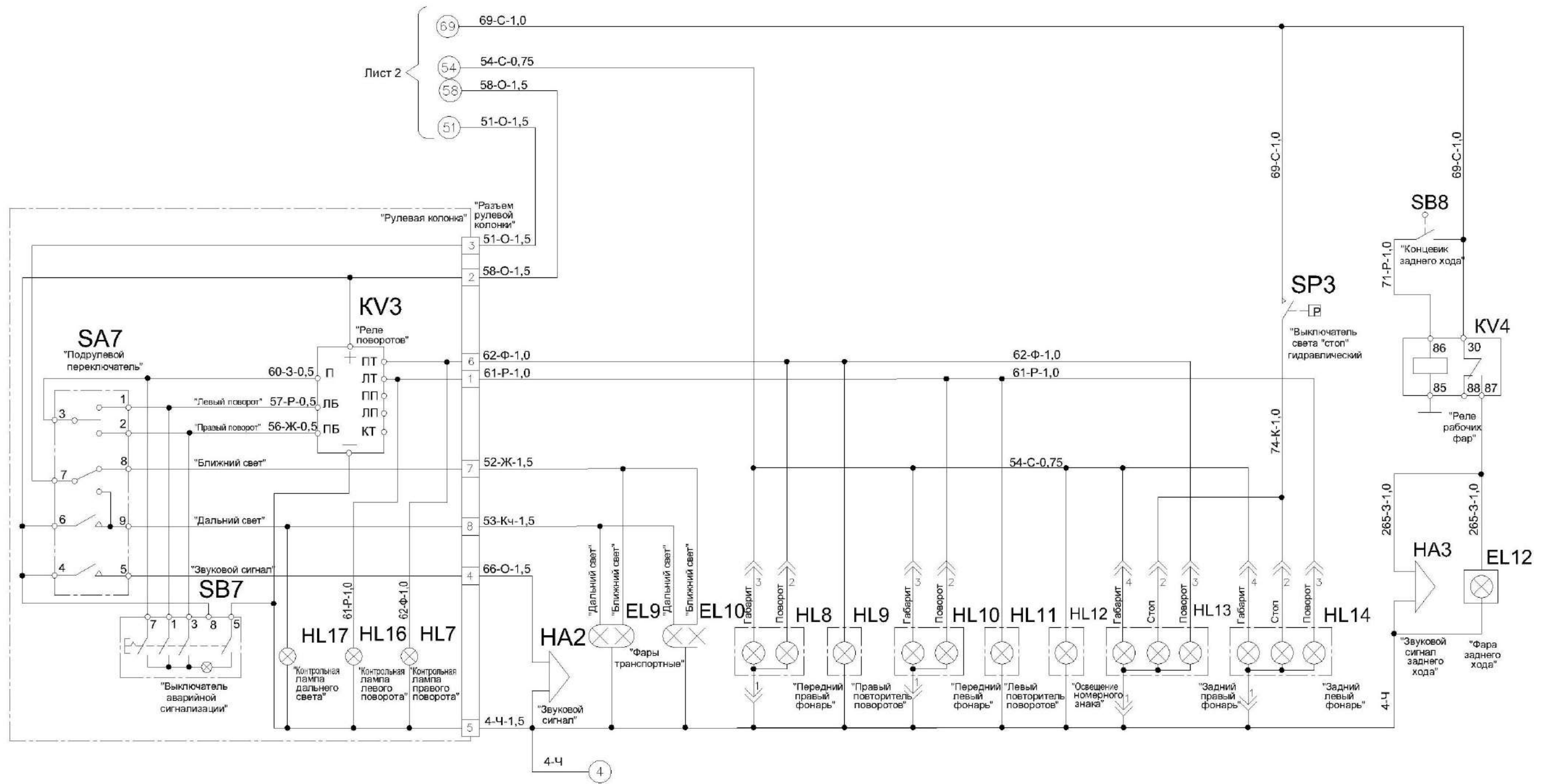
Рисунок Б.3 – Схема электрическая принципиальная комбайна (лист 3)
