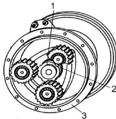
Рисунок 2.33 – Редуктор бортовой
