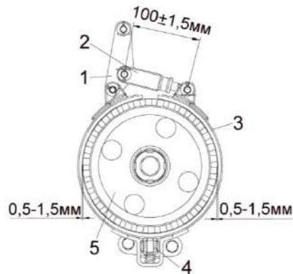
Рисунок 2.30 – Регулировка стояночного тормоза
