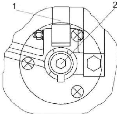
Рисунок 2.27 – Регулировка усилия
