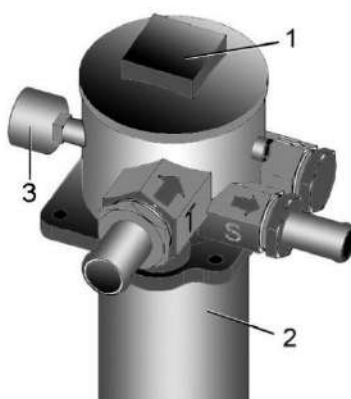
Рисунок 3.5 – Фильтр тонкой очистки
