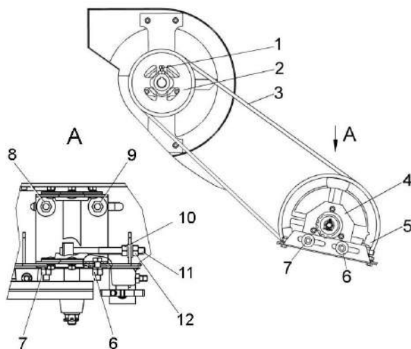
Рисунок 2.8 – Регулировка привода вентилятора
