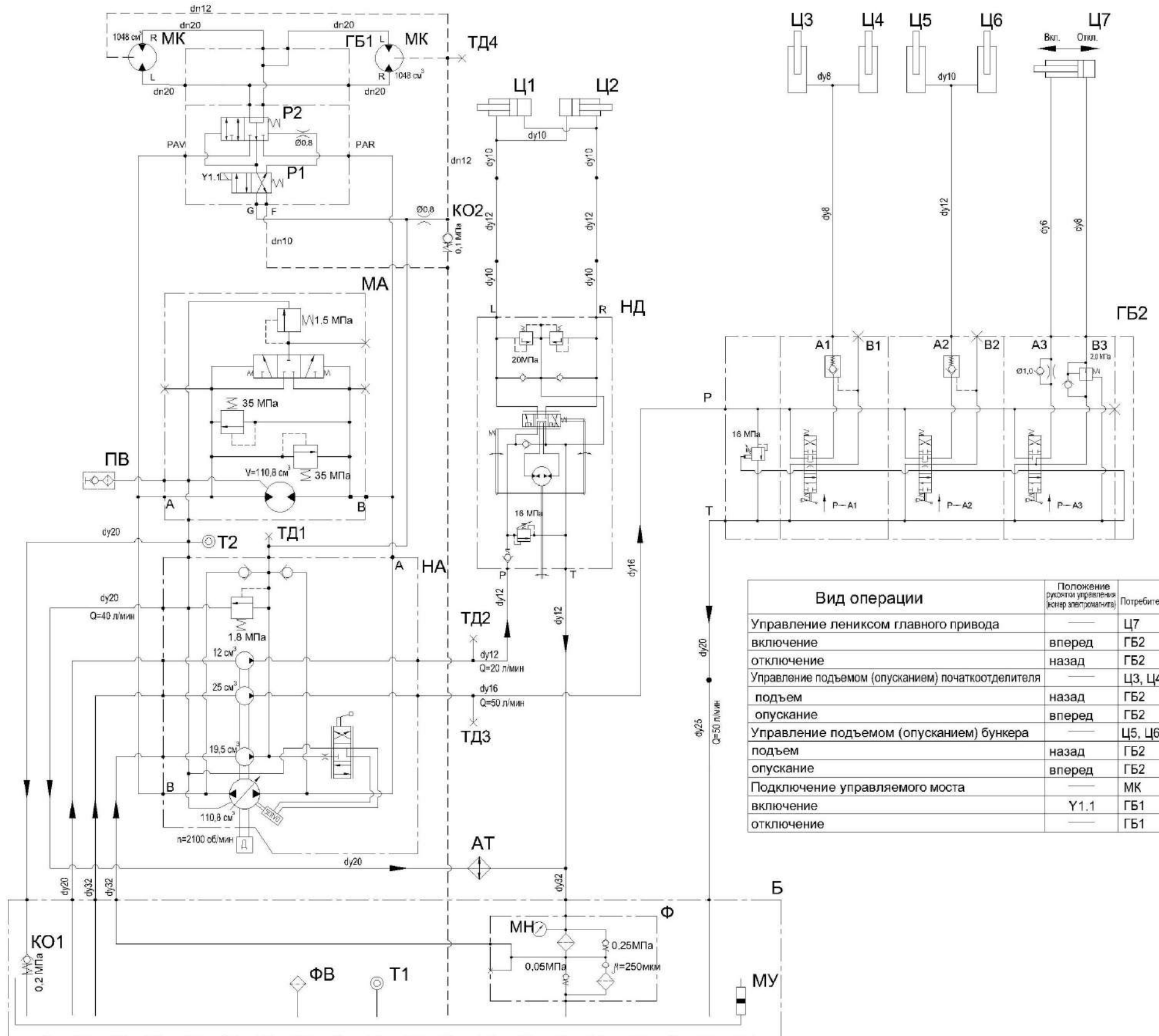
Рисунок А.1 – Схема гидравлическая принципиальная комбайна
