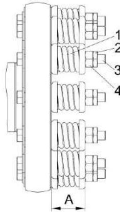
Рисунок 2.35 – Прокрутка предохранительных муфт
