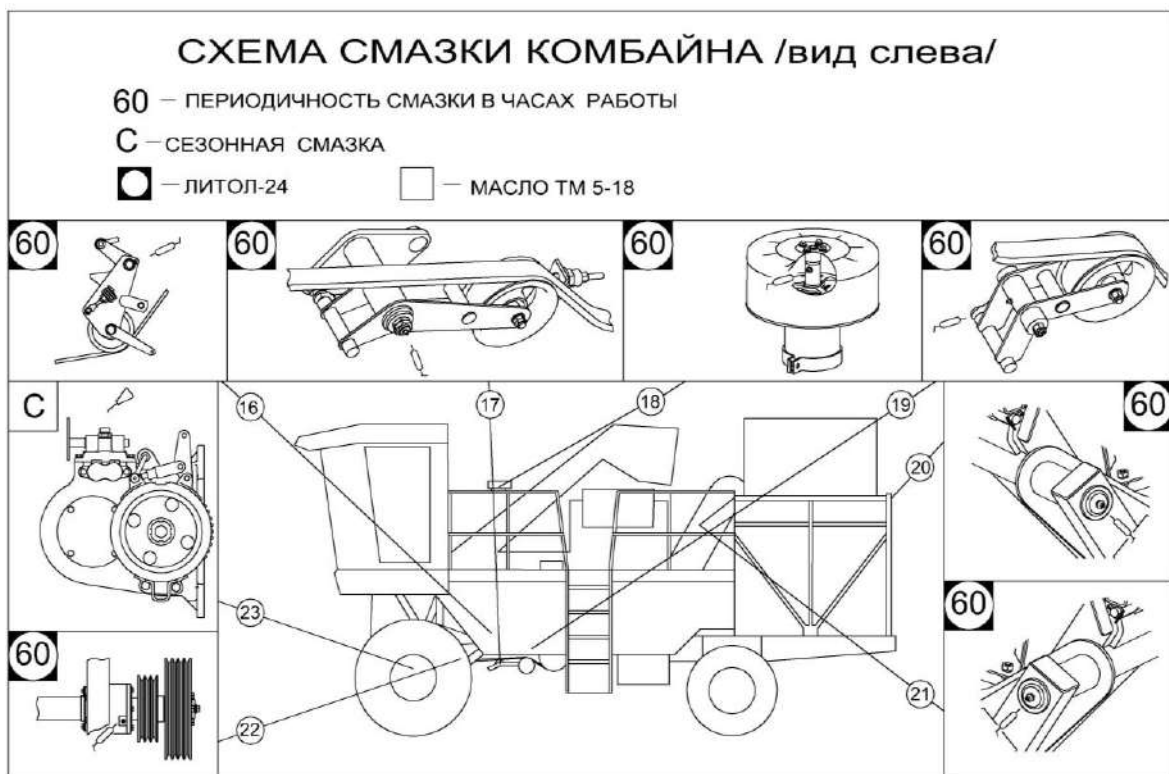
Рисунок 3.2 – Схема смазки комбайна (вид слева)
