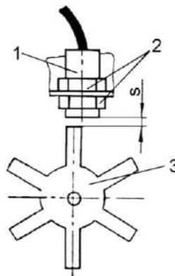
Рисунок 2.34 – Регулировка зазора между датчиком и лучами звездочек
