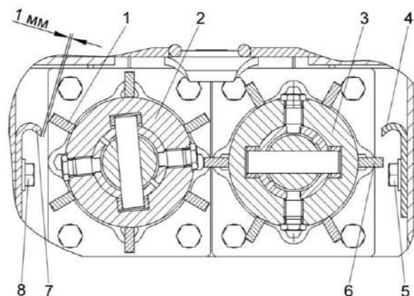
Рисунок 2. 24 – Регулировка чистиков
