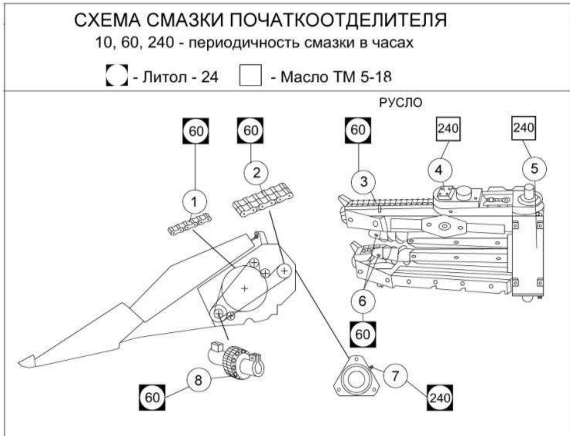
Рисунок 3.3 – Схема смазки початкоутделителя
