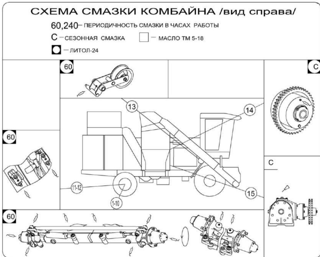
Рисунок 3.1 – Схема смазки комбайна (вид справа)
