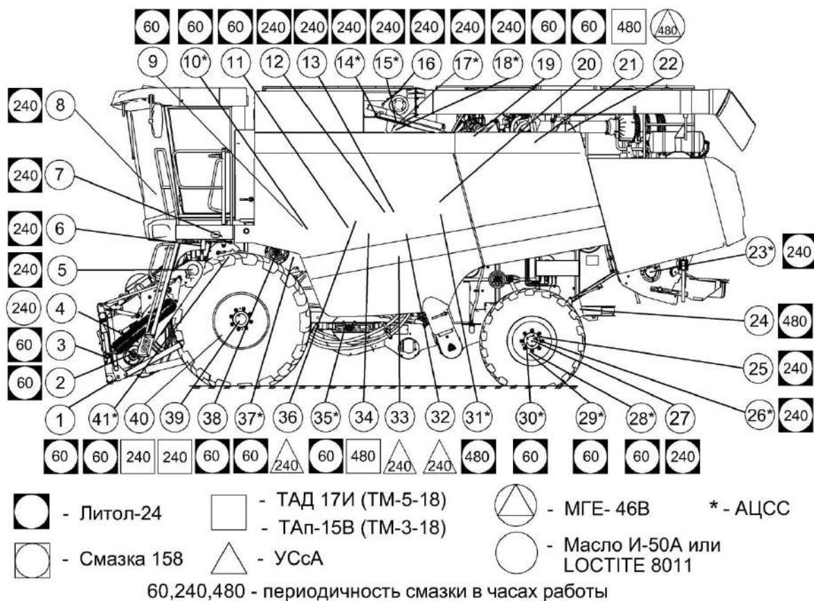
Рисунок 3.1 – Смазка комбайна (вид слева)
