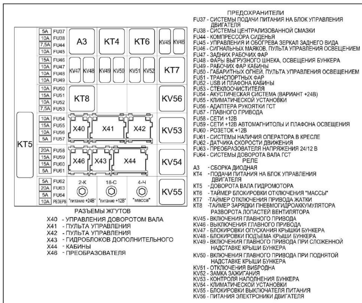
Рисунок 1.39 – Реле и предохранители пульта управления
