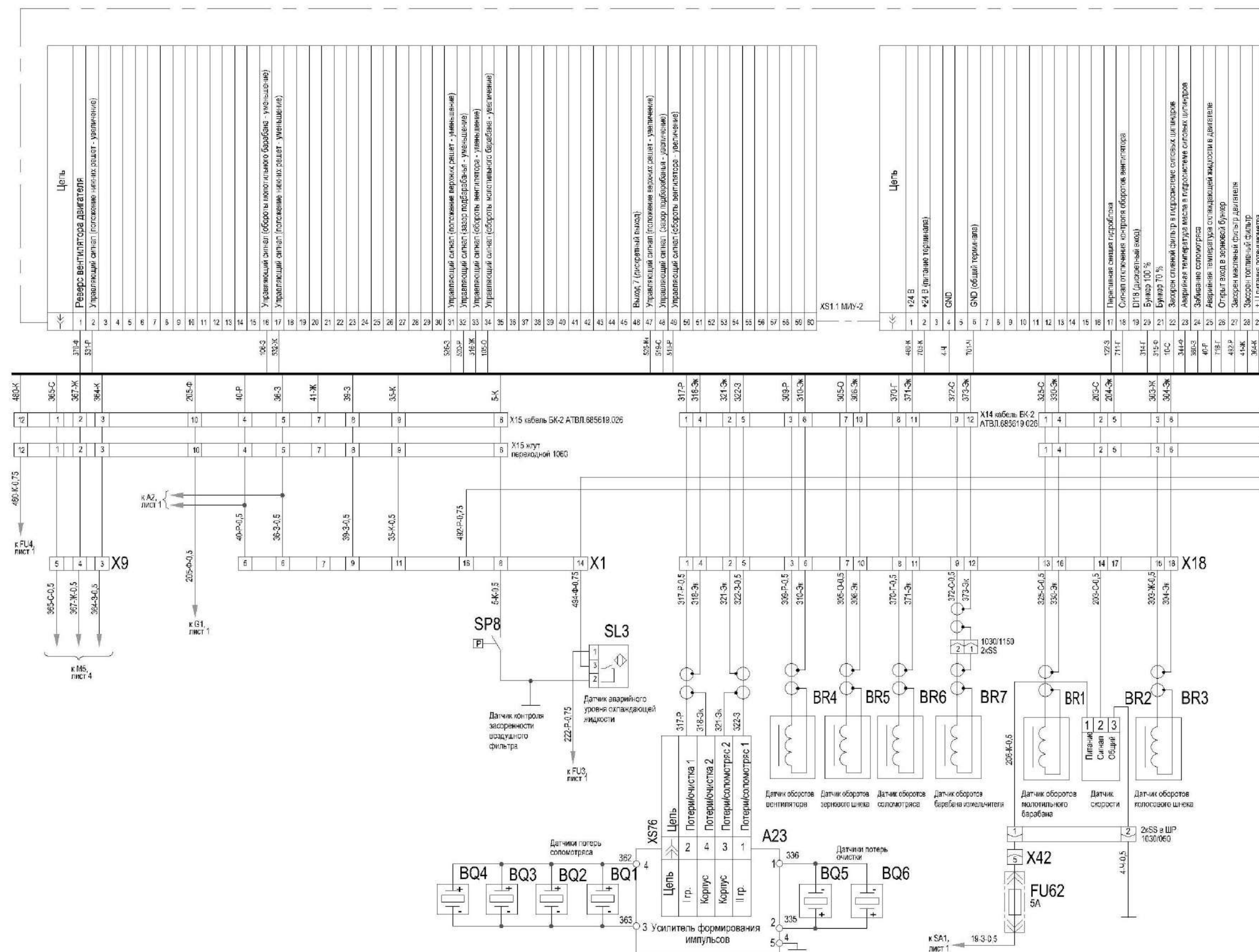
Рисунок Б.6 – Схема электрическая принципиальная комбайна (лист 6.1)
