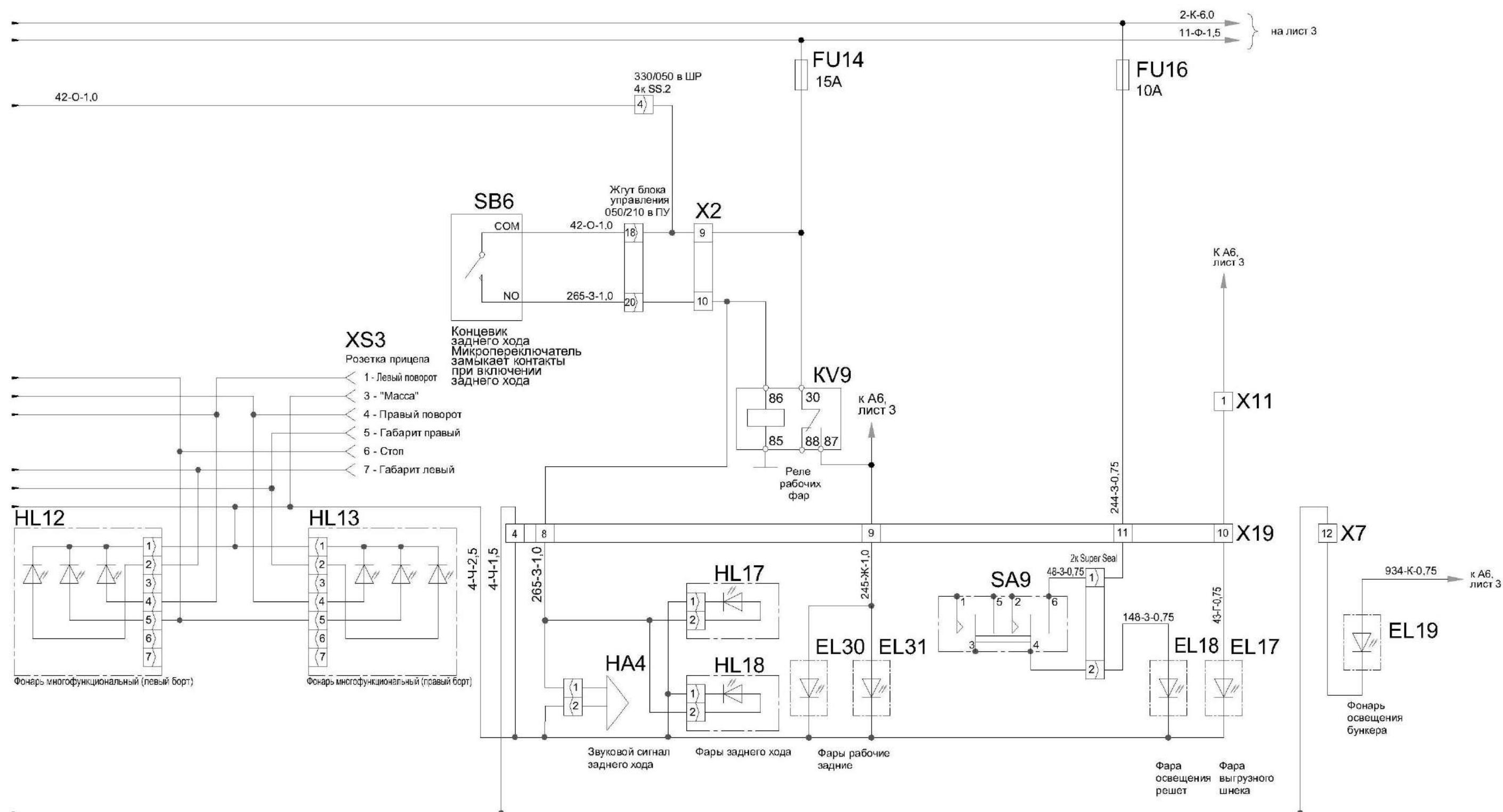
Рисунок Б.2 – Схема электрическая принципиальная комбайна (лист 2.3)
