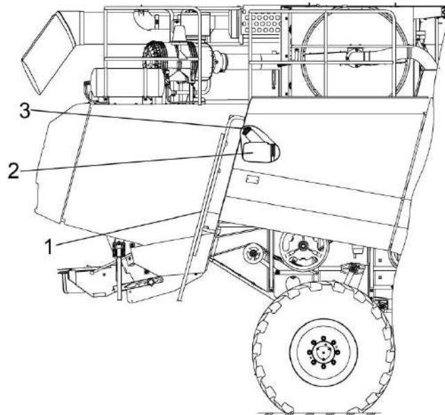
Рисунок 2.7 – Заправка топливного бака
