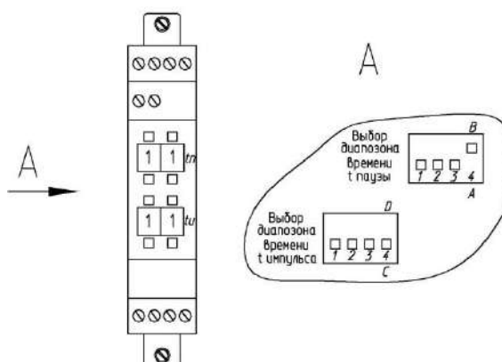
Рисунок 1.36 – Реле времени
