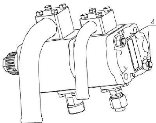
Рисунок 4.1 – Демонтаж гидронасоса
