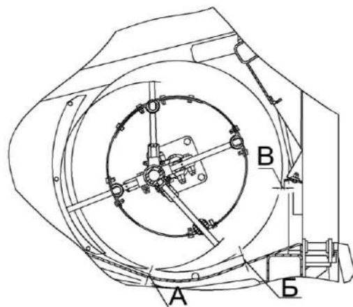
А – зазор между витками шнека и днищем жатки; Б – зазор между пальцами шнека и днищем жатки В – зазор между витками шнека и чистиками
