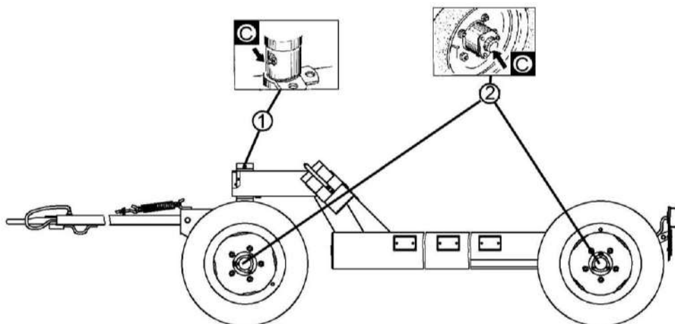
Рисунок 3.5 – Схема смазки транспортной тележки
