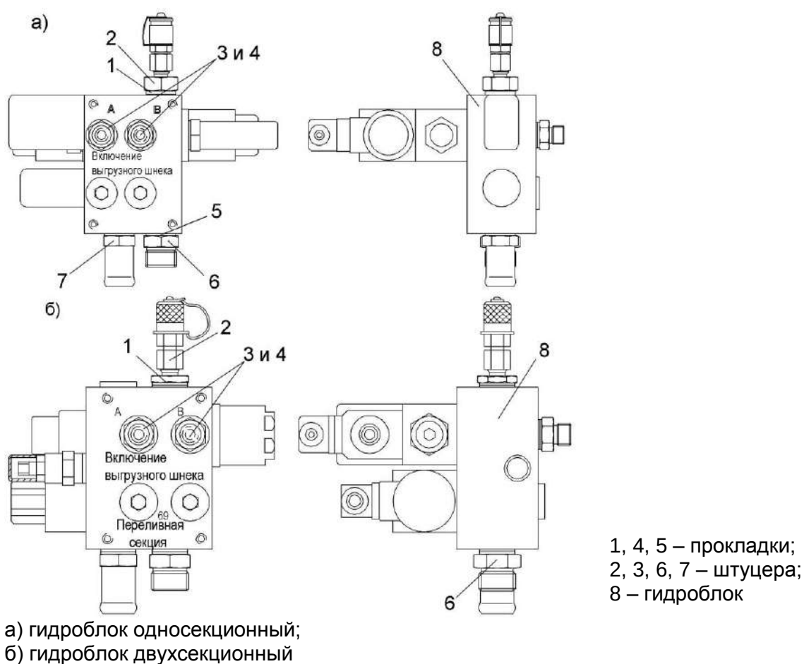
Рисунок 1.23 – Гидроблоки
