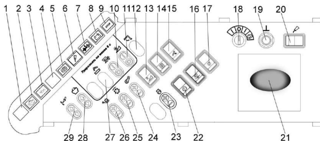
Рисунок 1.34 – Пульт управления комбайна с двигателем DTA
