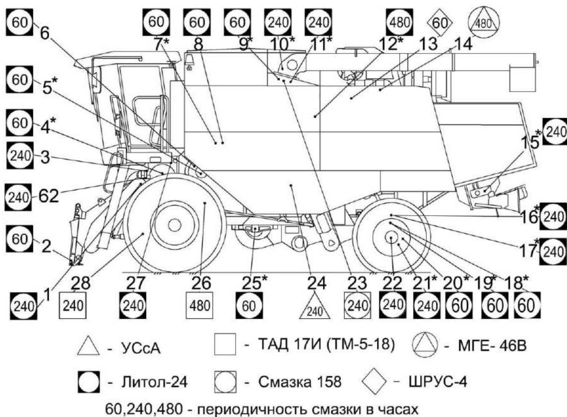
Рисунок 3.2 – Смазка молотилки (вид слева)
