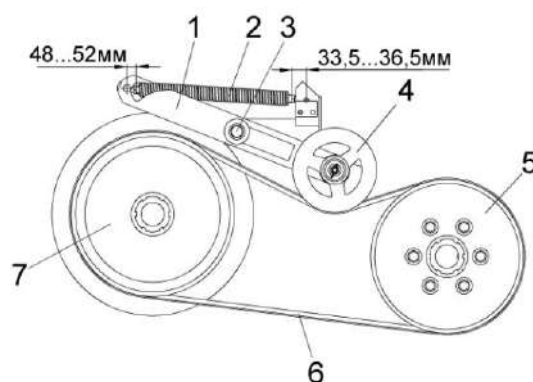
Рисунок 2.35 – Привод отбойного бitera
