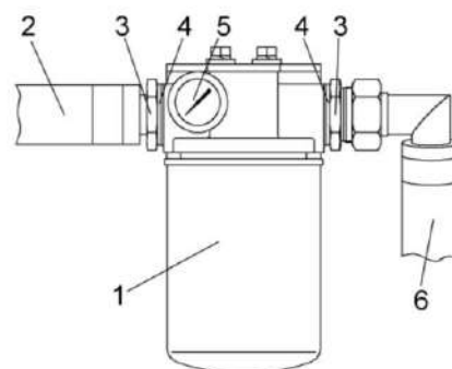
1 – фильтр; 2, 6 – рукава высокого давления; 3 – штуцера; 4 – прокладки; 5 – вакуумметр
