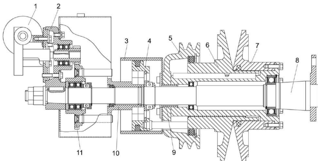
1, 2 – привод; 3 - кожух; 4 – упор; 5, 6, 7 – шкивы; 8 – ось; 9, 10 – втулки; 11 – колесо
