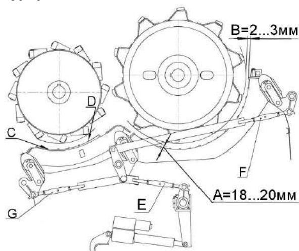
Рисунок 2.19 - Схема молотильного аппарата
