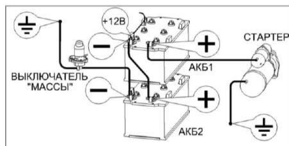
Рисунок 2.2 - Подключение аккумуляторных батарей
