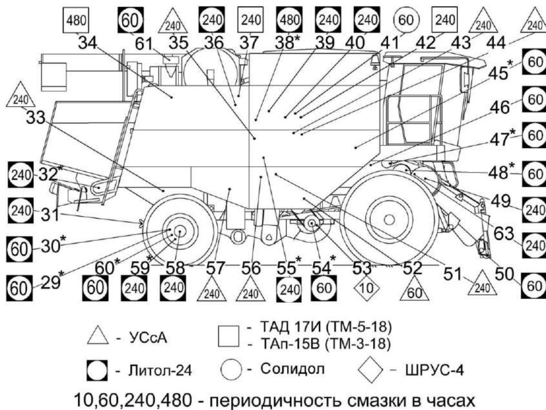
Рисунок 3.3 – Смазка молотилки (вид справа)
