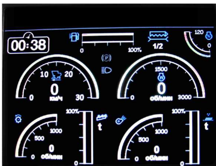
Рисунок 1.110 – Экран технологического режима уборки (комбайнирования)
