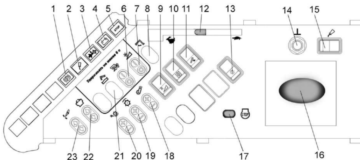
Рисунок 1.33 – Пульт управления комбайна с двигателем ЯМЗ
