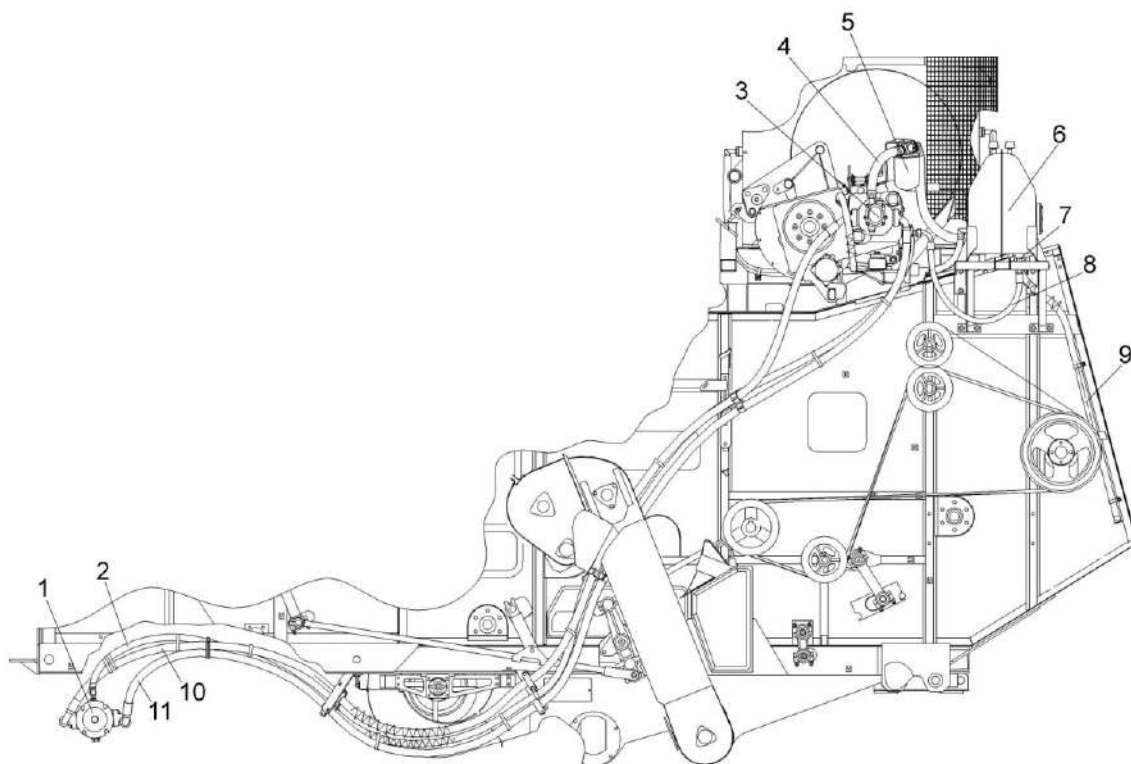
1 – гидромотор; 2, 9 – рукава; 3 – гидронасос; 4, 8, 10, 11 – рукава высокого давления; 5 – фильтр всасывающий; 6 - бак масляный; 7 - гидроклапан обратный
