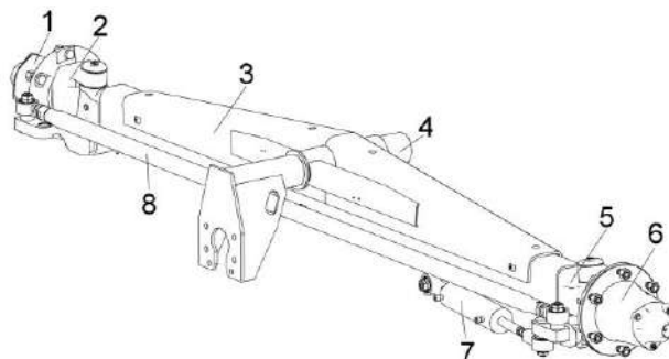
Рисунок 1.8 – Шасси
