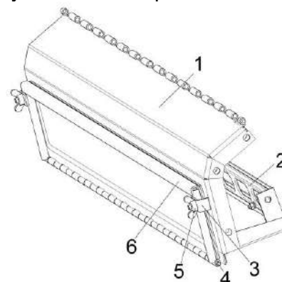
Рисунок 1.5– Аппарат молотильный
