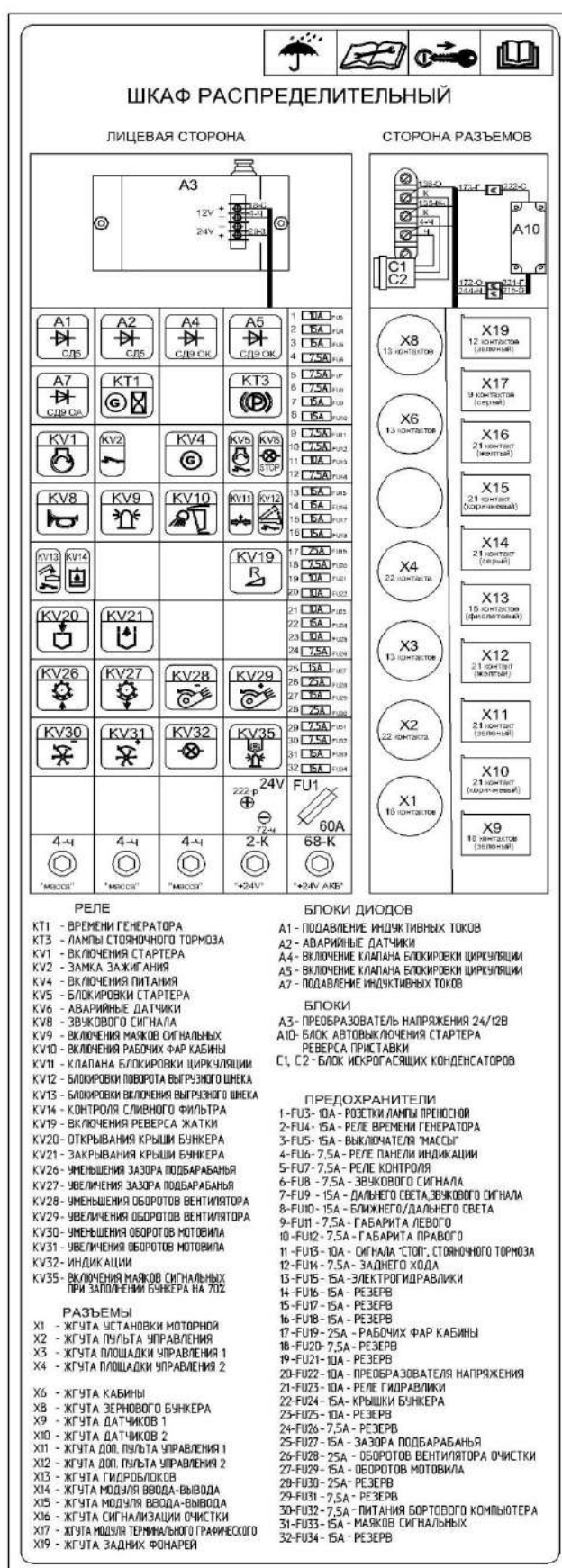
Рисунок 1.22 – Схема соединений шкафа распределительного
