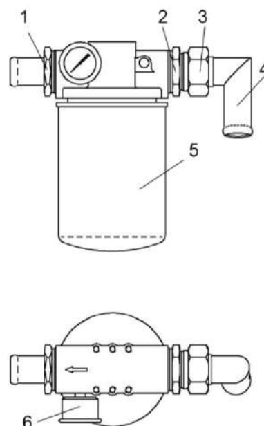
Рисунок 1.18 – Фильтр напорный
