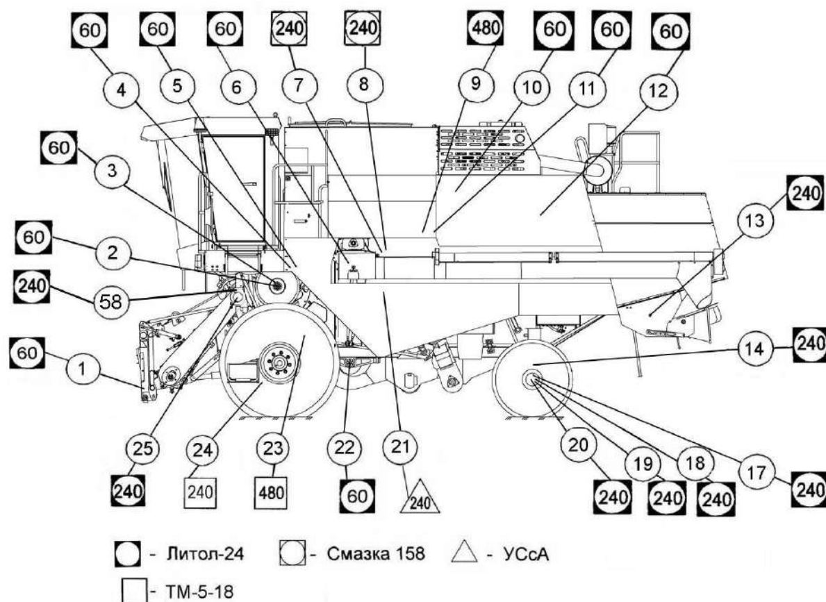
Рисунок 3.1 – Смазка комбайна (вид слева)
