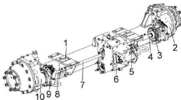
Рисунок 1.9 – Мост управляемых колес.
