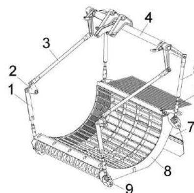
Рисунок 1.6 – Камнеуловитель
