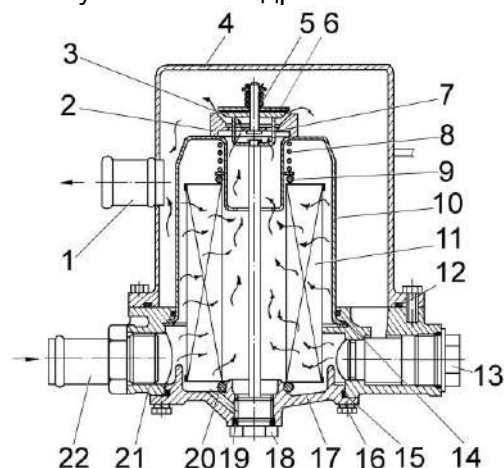
Рисунок 1.16 - Гидросистема
