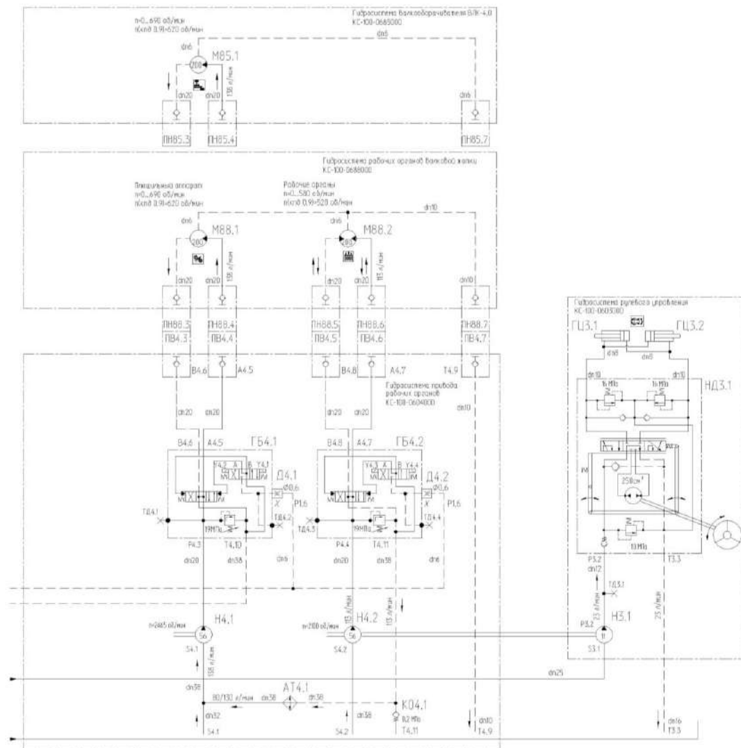
Рисунок А.1 – Схема гидравлическая принципиальная косилки самоходной КС-100 (лист 2)
