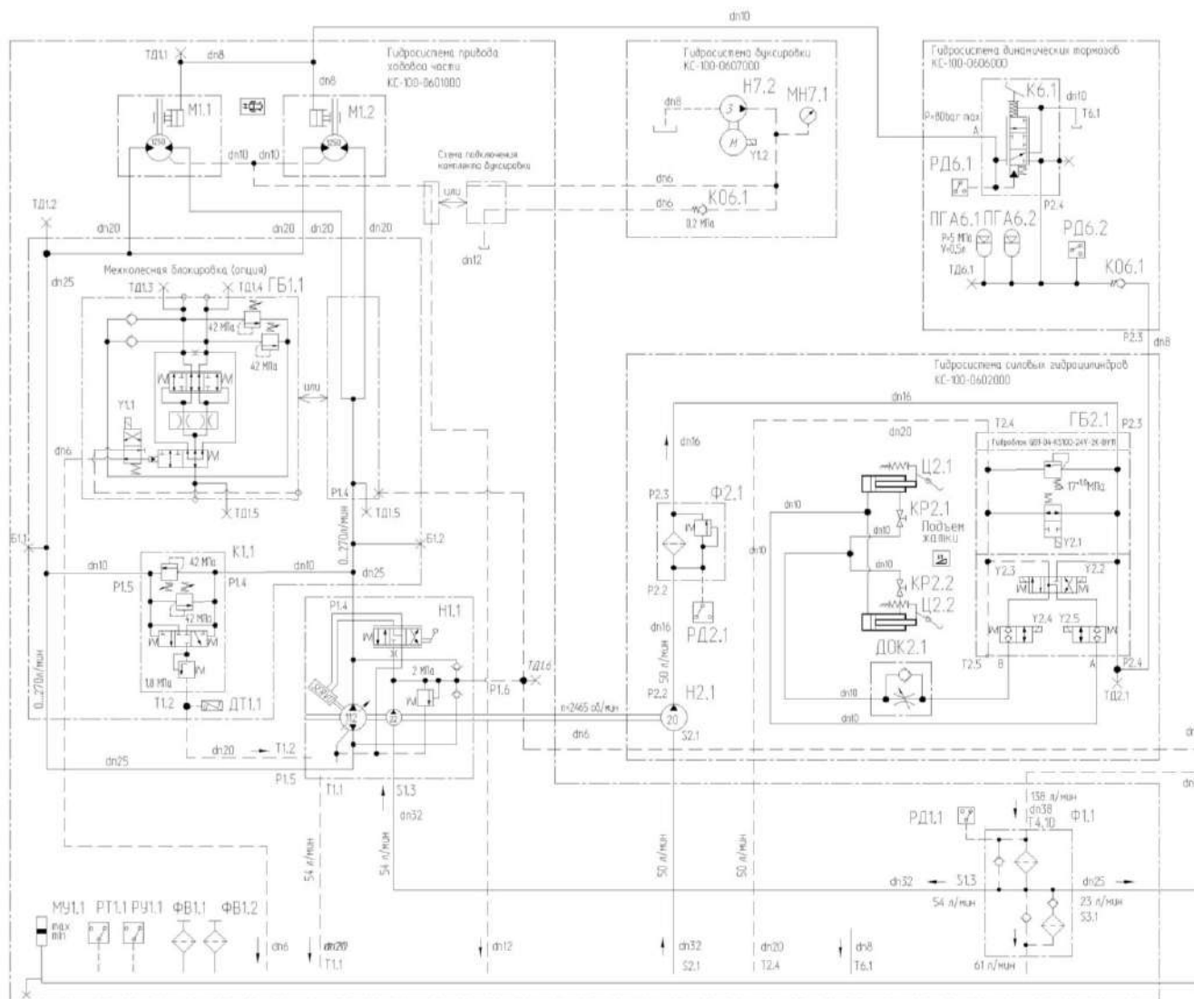
Рисунок А.1 – Схема гидравлическая принципиальная косилки самоходной КС-100 (лист 1)
