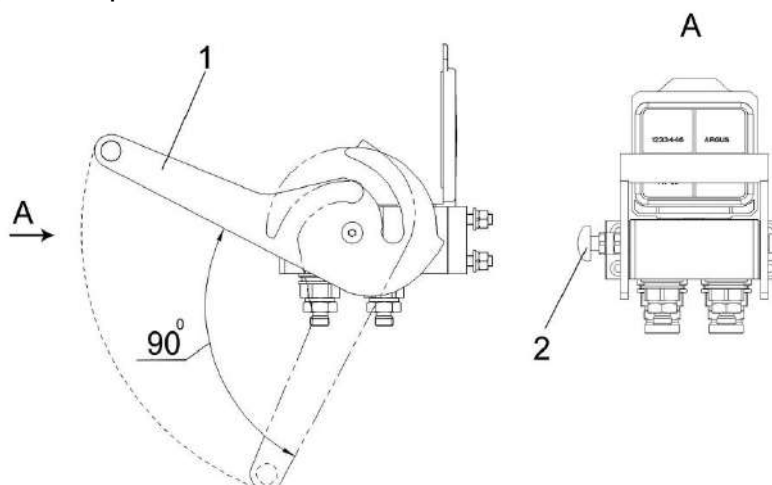
Рисунок 2.7 – Разъем многофункциональный
