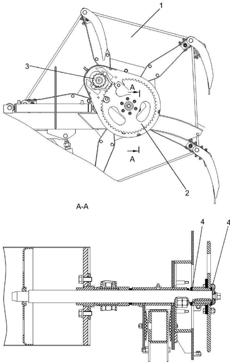
Рисунок 2.16 – Регулировка цепной передачи (жатка справа)
