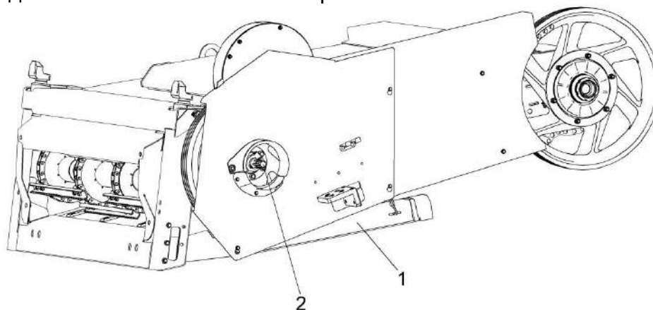
Рисунок 2.6 – Наклонная камера
