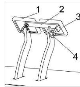
1, 3 – педали тормозные; 2 – планка; 4 – упор
