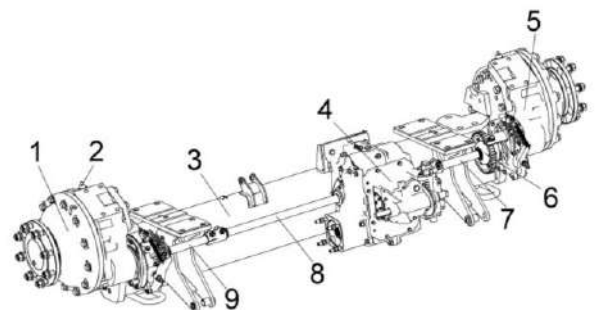
Рисунок 1.10 - Мост управляемых колес.
