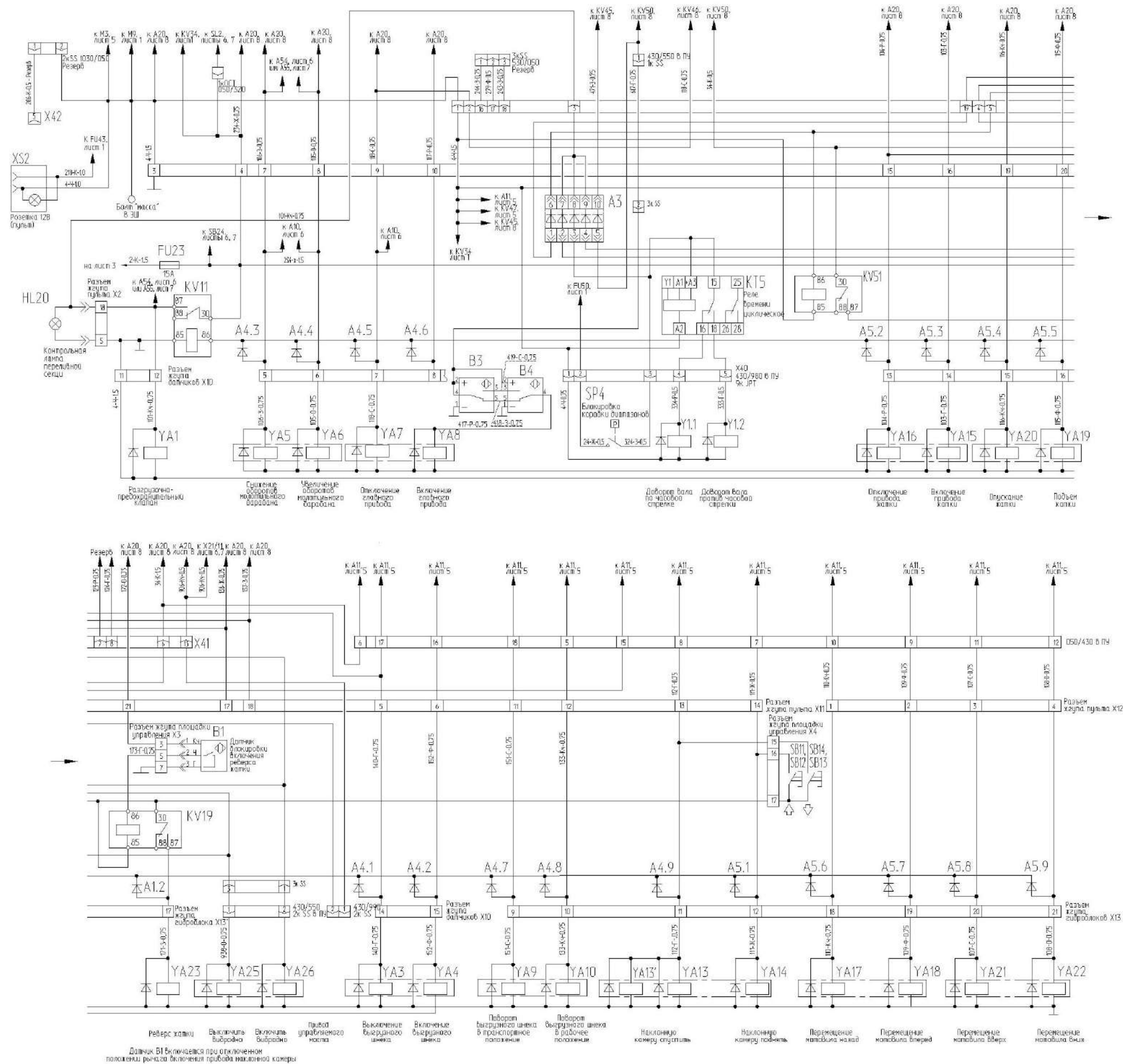
Рисунок Б.4 – Схема электрическая принципиальная комбайна (лист 4)
