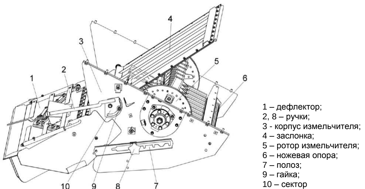
Рисунок 1.15 – Соломоизмельчитель
