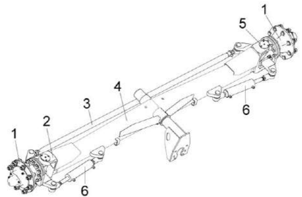
Рисунок 1.9 – Шасси
