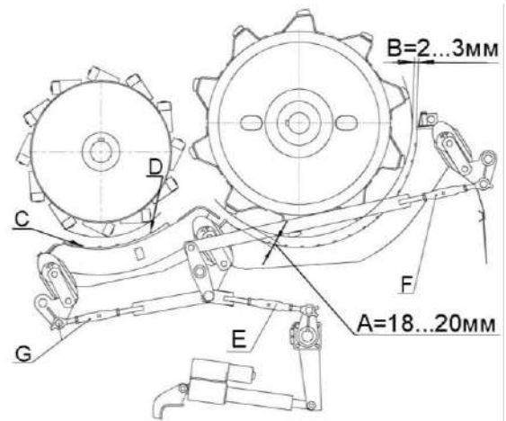
Рисунок 2.10 - Схема молотильного аппарата
