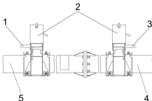
Рисунок 2.4 – Расфиксация жатки
