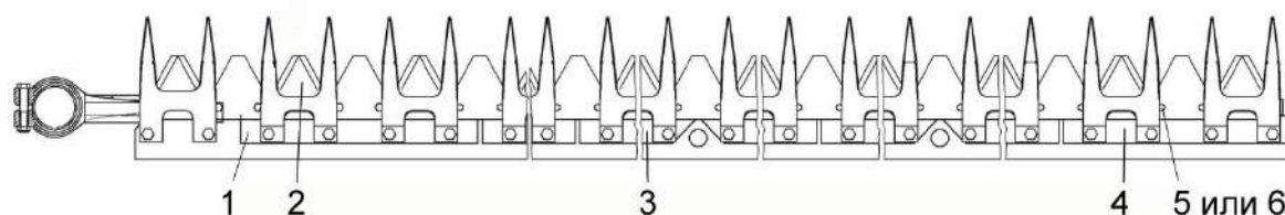
1, 3, 4 – пластины трения; 2 – сегмент; 5 – заклепка; 6 – болт
