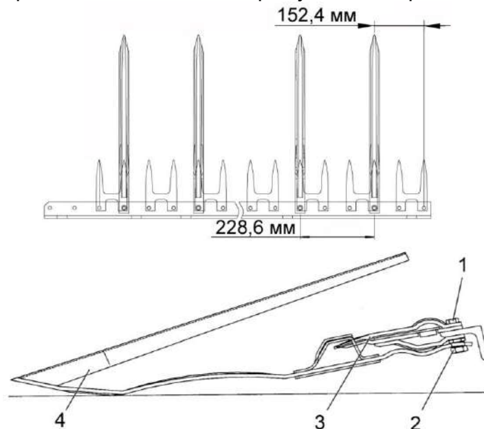
Рисунок 2.10– Установка стеблеподъемника
