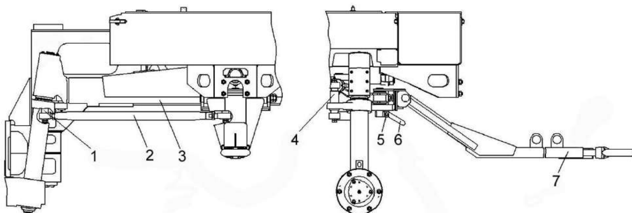
1, 4 – оси; 2 – тяга; 3 – балка моста; 5 – болт; 6 – палец; 7 - дышло
