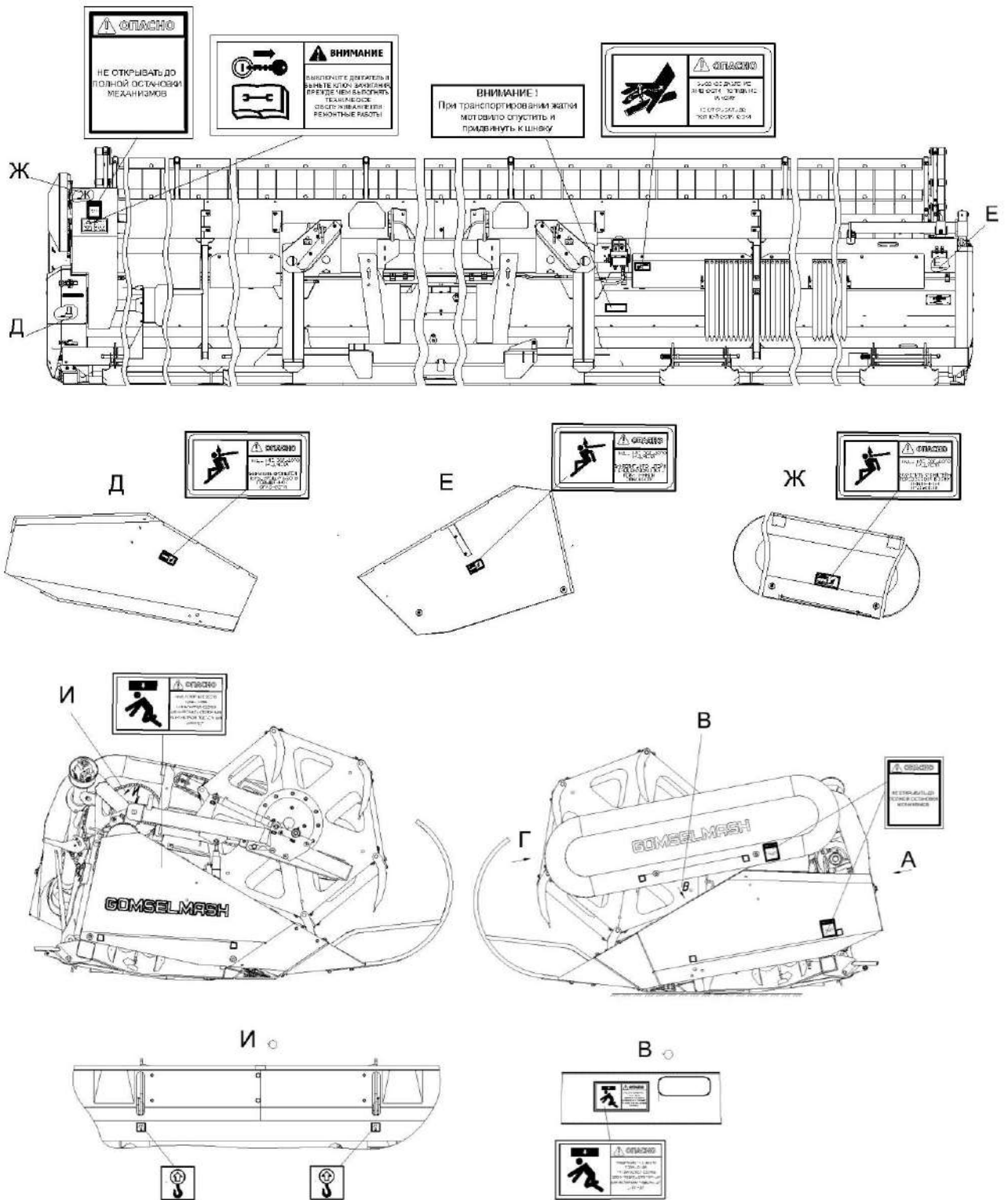
Расположение на жатке предупредительных и указательных знаков и табличек безопасности
