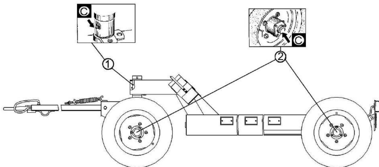
Рисунок 3.3 – Схема смазки транспортной тележки
