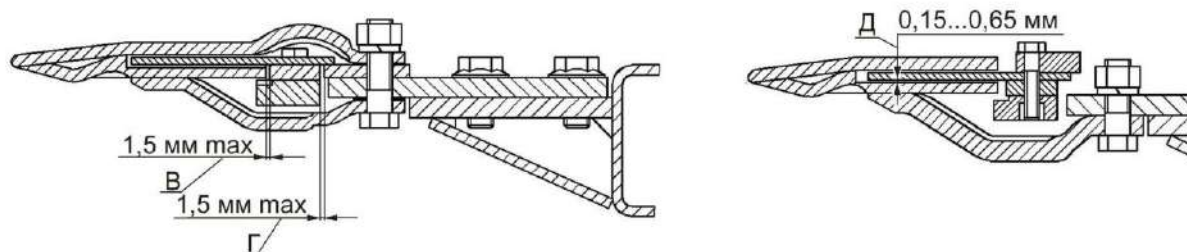
Рисунок 2.12 – Режущий аппарата
