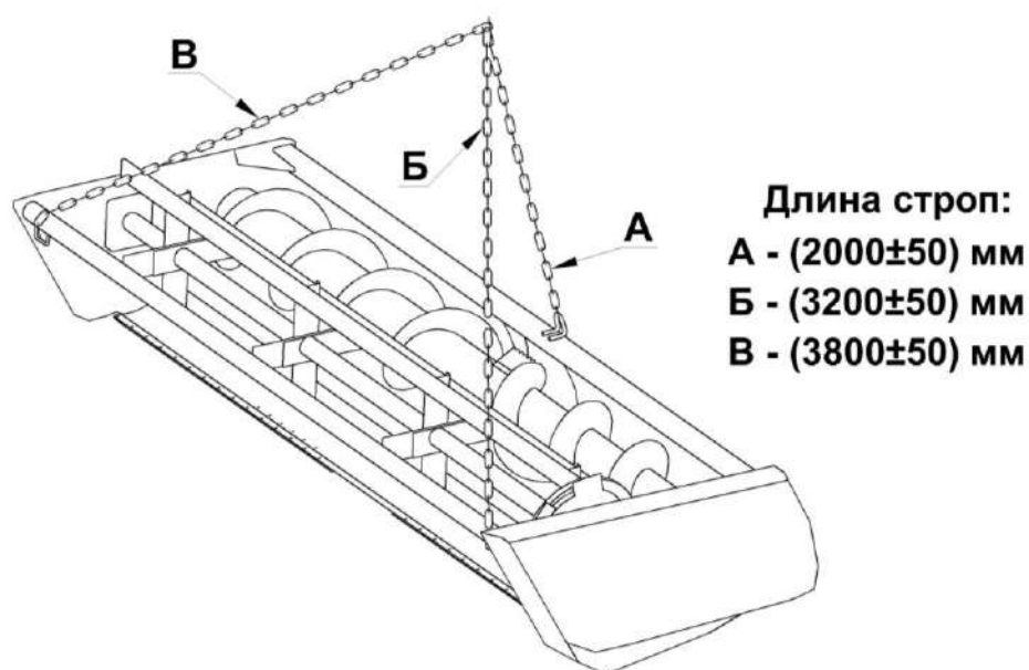
Рисунок 8.1 – Схема строповки
