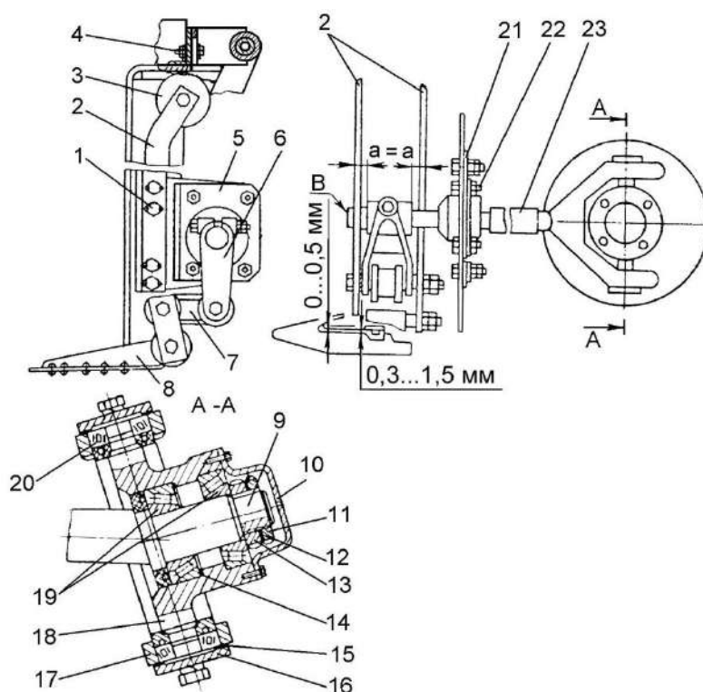
Рисунок 2.10 – Регулирование режущего аппарата и его привода
