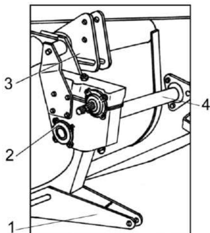
1 – ловители нижние; 2 – редуктор контрпривода; 3 – ловители верхние; 4 – контрпривод
