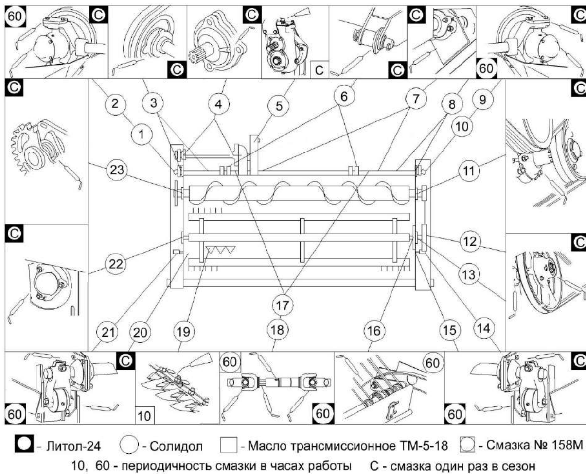
Рисунок 3.1 – Схема смазки жатки для трав
