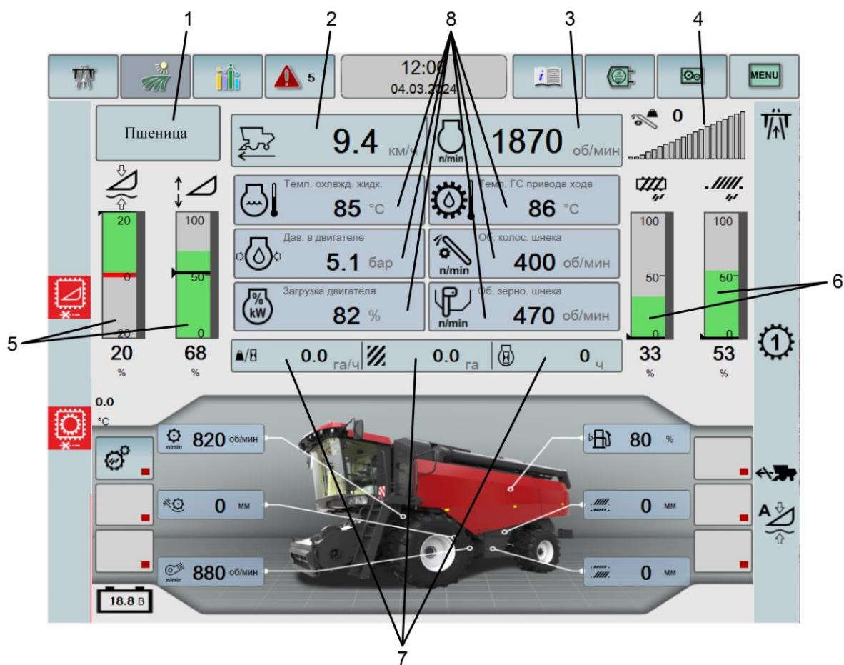
Рисунок Ж.4 – Экран терминала в режиме «Поле»
