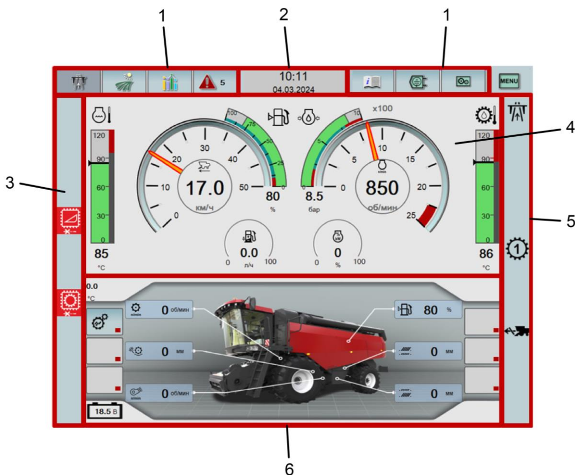
Рисунок Ж.2 – Экран терминала
