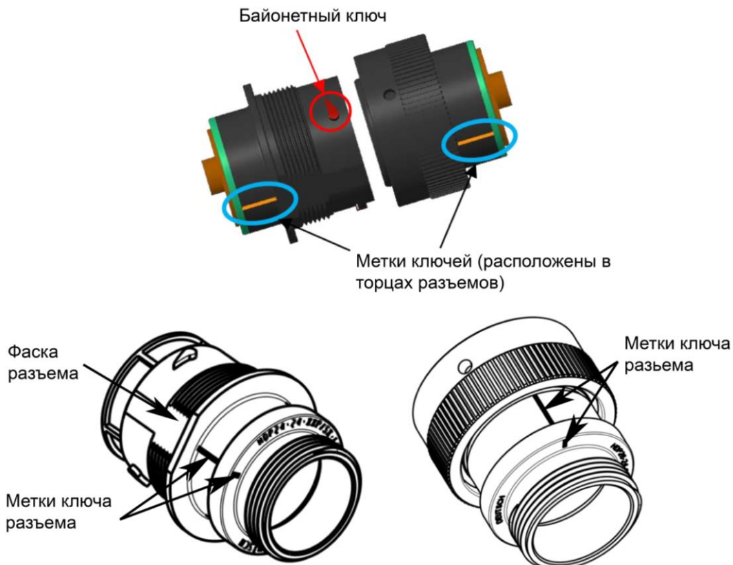
Рисунок 2.9 – Совмещение по ключам
