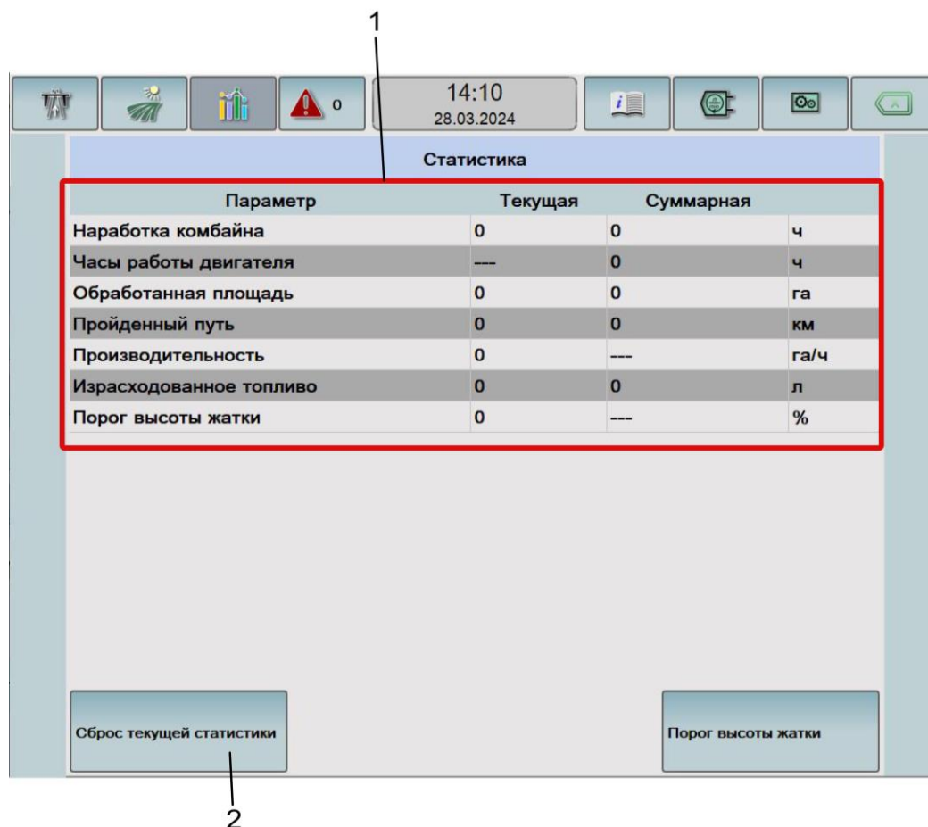
Рисунок Ж.22 – Экран «Статистика»
