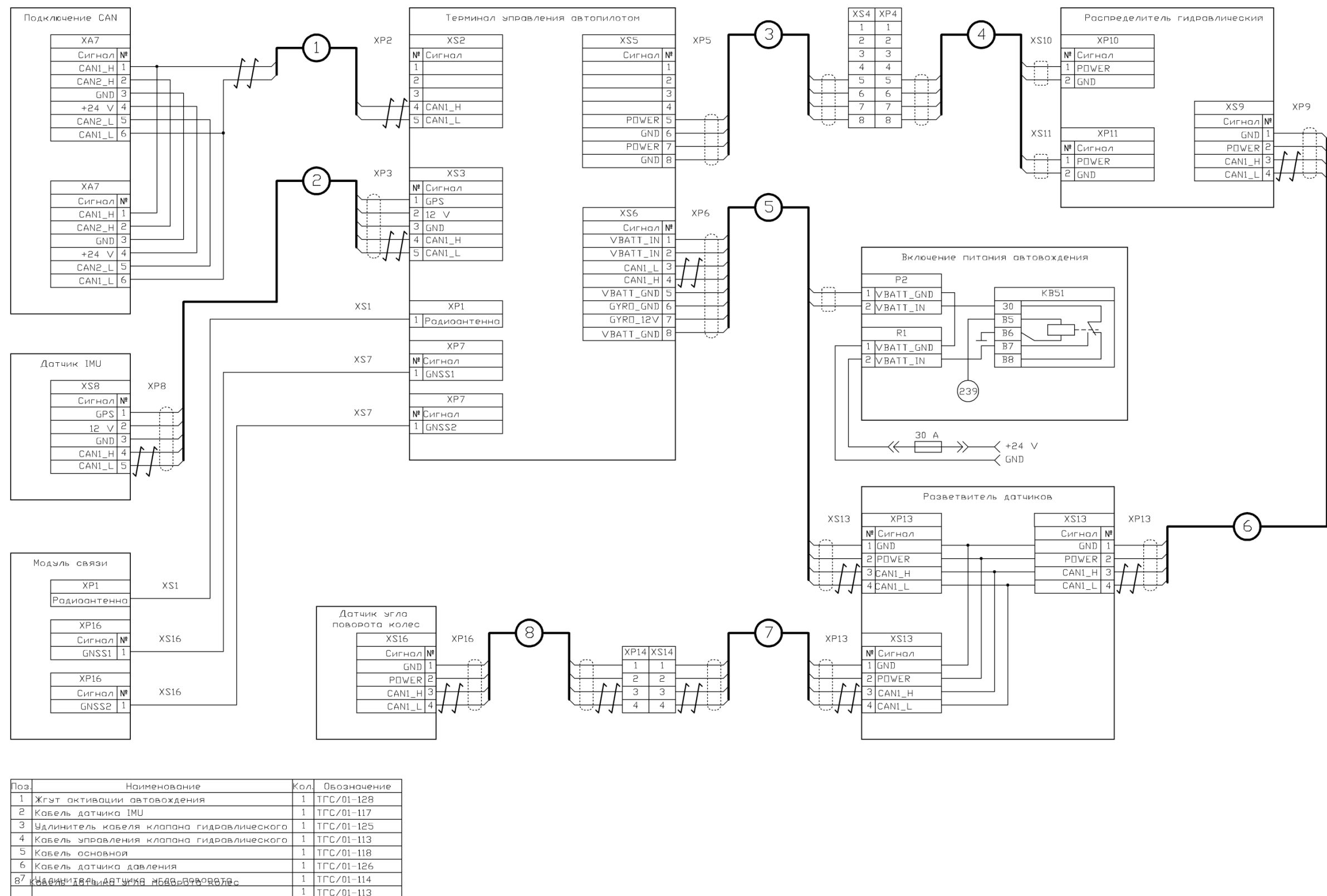
Рисунок Б.18 – Схема электрическая принципиальная комбайна
