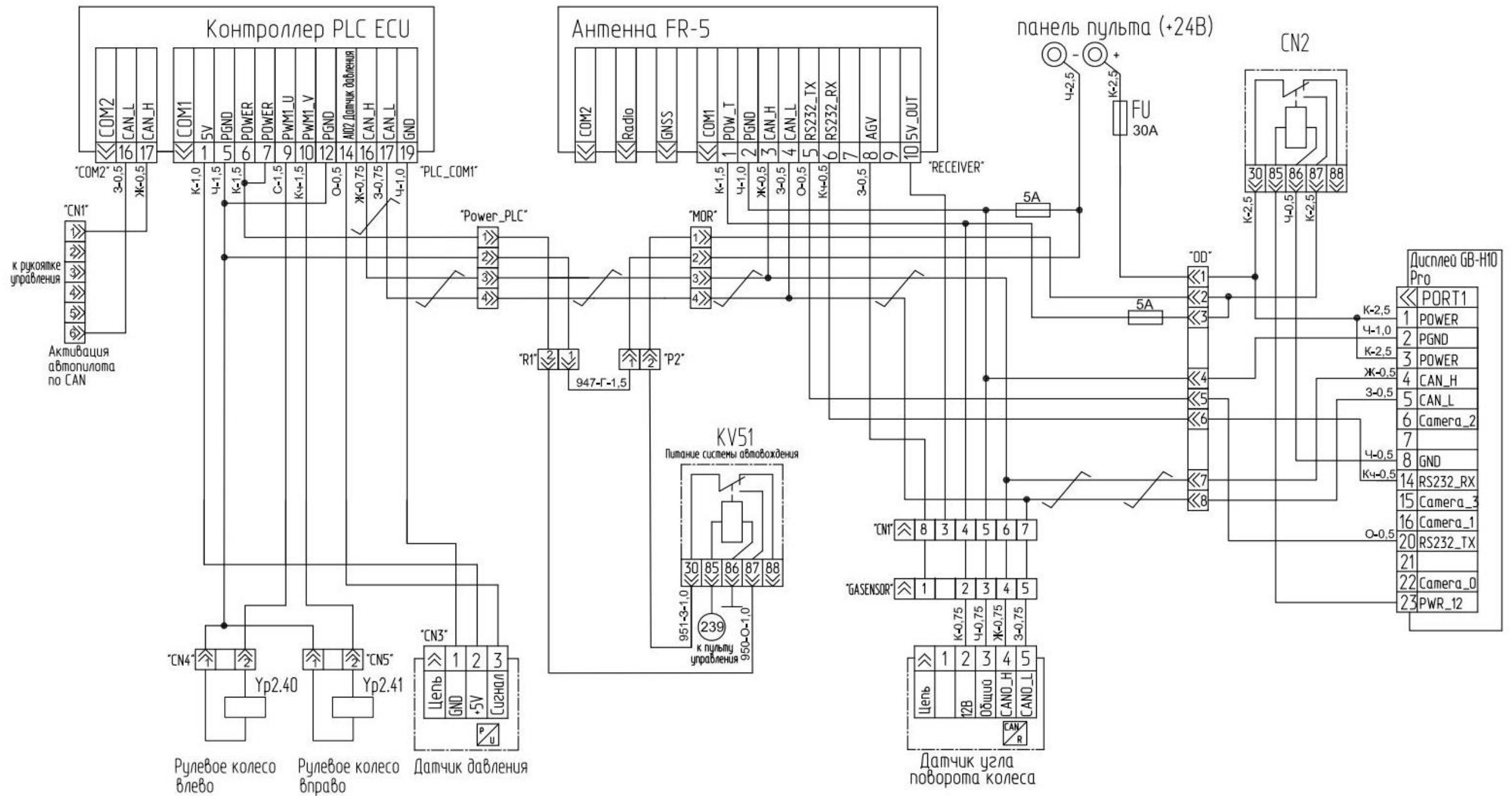
Рисунок Б.17 – Схема электрическая принципиальная комбайна
