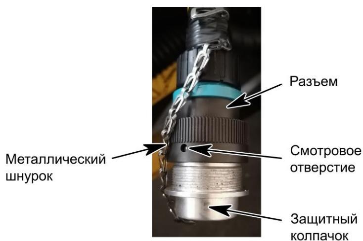
Рисунок 2.13 – Соединение защитного колпачка
