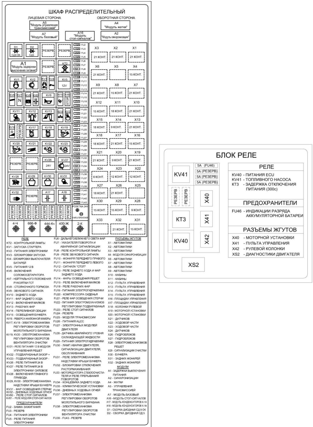
Рисунок 1.24 – Схема соединений шкафа распределительного и блока реле
