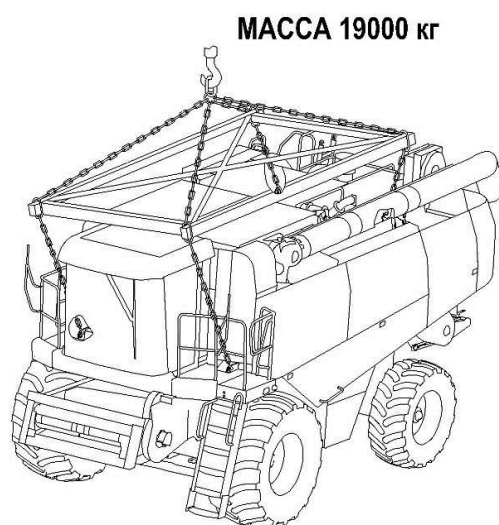
Рисунок 6.1 – Схема строповки комбайна
