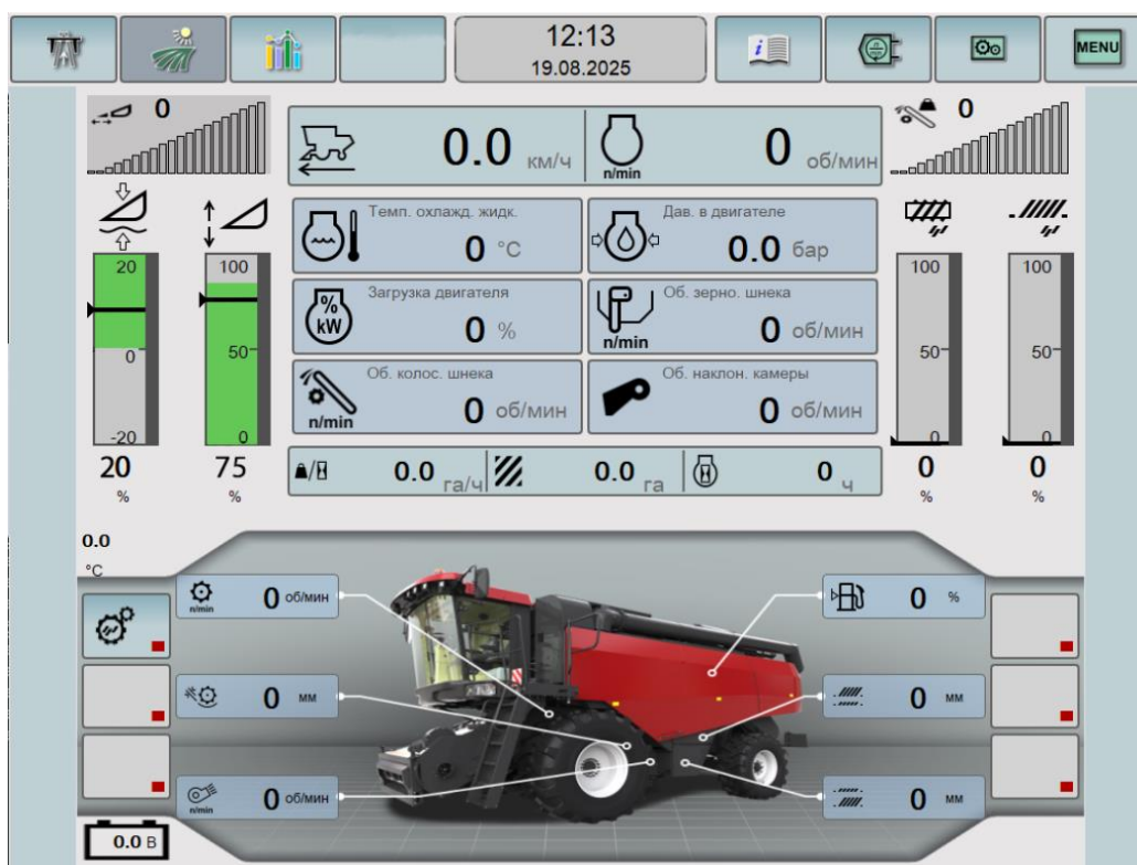
Рисунок 2.14 – Экран «ПОЛЕ»
