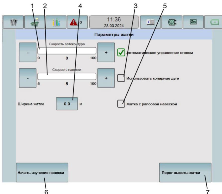
Рисунок Ж.9 – Экран «Параметры жатки»
