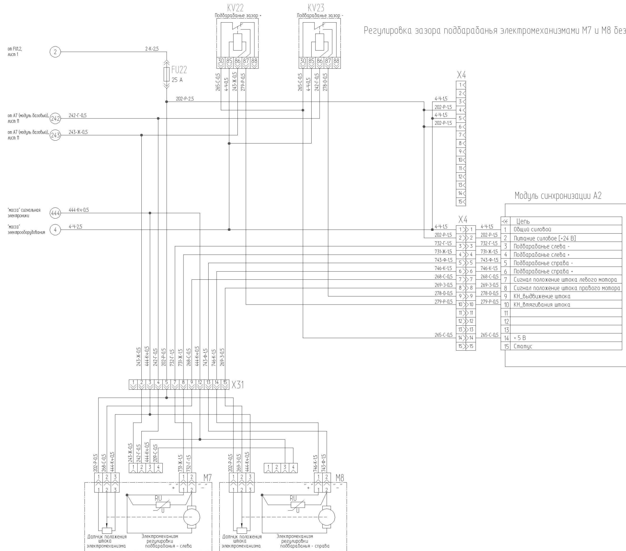
Рисунок Б.12 – Схема электрическая принципиальная комбайна
