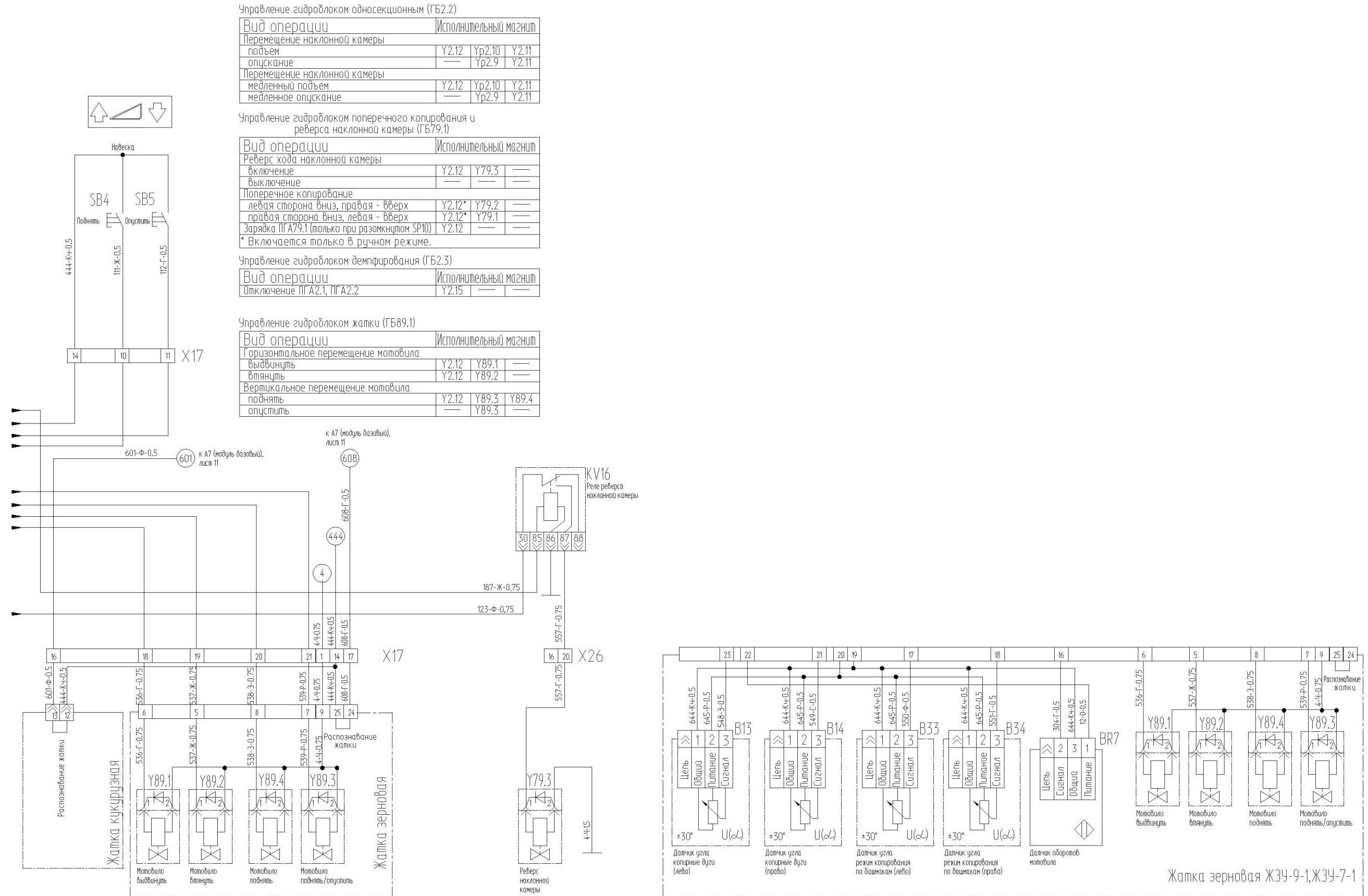
Рисунок Б.9 – Схема электрическая принципиальная комбайна (лист 2)
