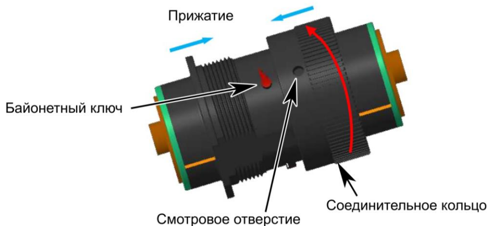
Рисунок 2.10 – Прижатие и проворот соединительного кольца
