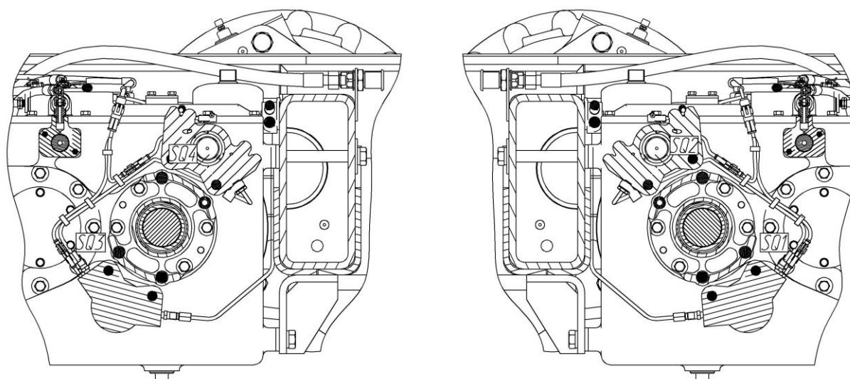
Вариант 2. Ведущий мост. Вид сбоку
