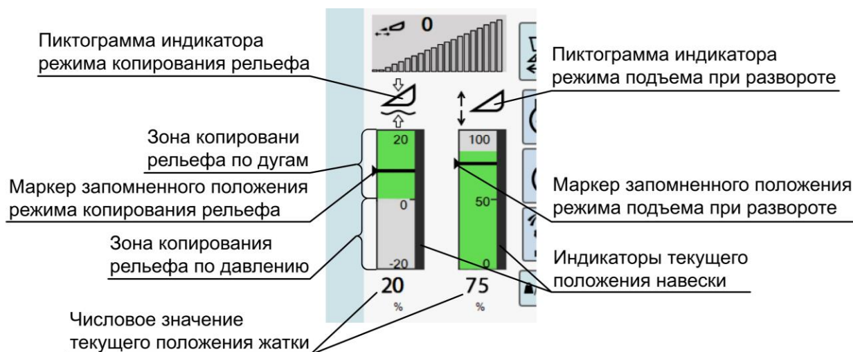
Рисунок 2.15 – Индикаторы положения навески
