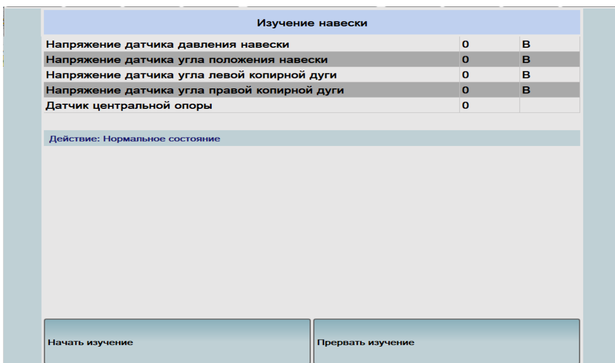
Рисунок Ж.10 – Экран «Изучение навески»
