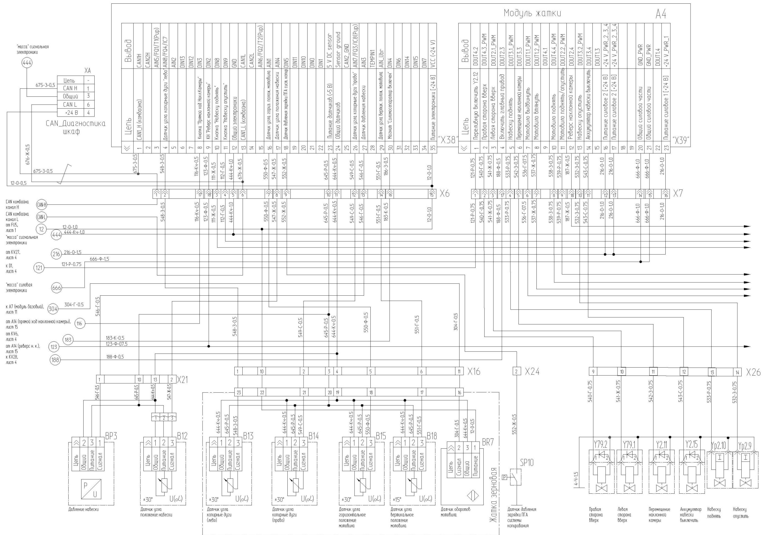
Рисунок Б.9 – Схема электрическая принципиальная комбайна (лист 1)
