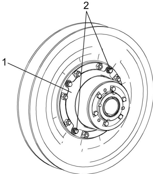
а) Вариатор
