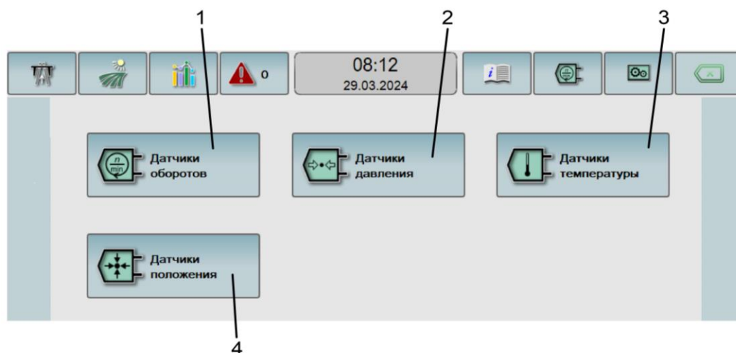
Рисунок Ж.12 – Экран «Диагностика датчиков»
