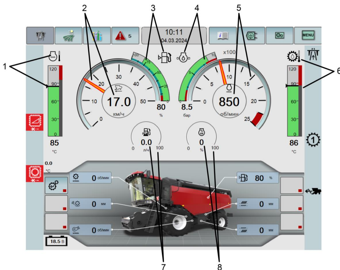
Рисунок Ж.3 – Экран терминала в режиме «Дорога»
