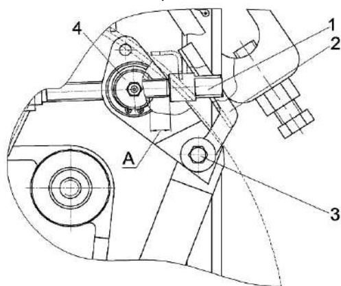
Рисунок 2.11 – Отвод питающего аппарата от измельчающего
