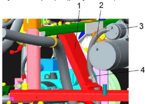
1 – щиток; 2 – жгут стартера; 3 – стартер; 4 – хомут
