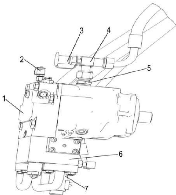
1 – гидромотор привода питающего аппарата; 2 – точка диагностики; 3 - полумуфта заправочная; 4 – тройник; 5 - шланг; 6 – гидроблок экстренного останова
