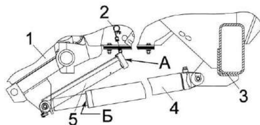
1 – питающе-измельчающий аппарат; 2 – пружина; 3 - балка моста; 4 – гидроцилиндр; 5 – упор; А и Б – опорные поверхности
