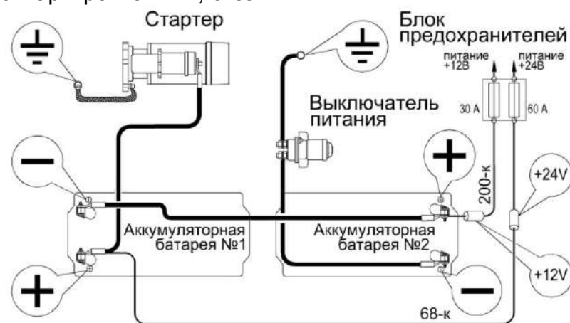
Рисунок 2.3 – Схема подключения аккумуляторных батарей
