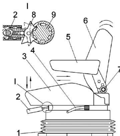
1 – чехол; 2 – рукоятка регулировки сиденья по массе оператора; 3 – подушка сиденья; 4 – рычаг фиксации продольного перемещения сиденья; 5 – подлокотник; 6 – подушка спинки; 7 – маховик регулировки спинки; 8 – собачка; 9 – винт
