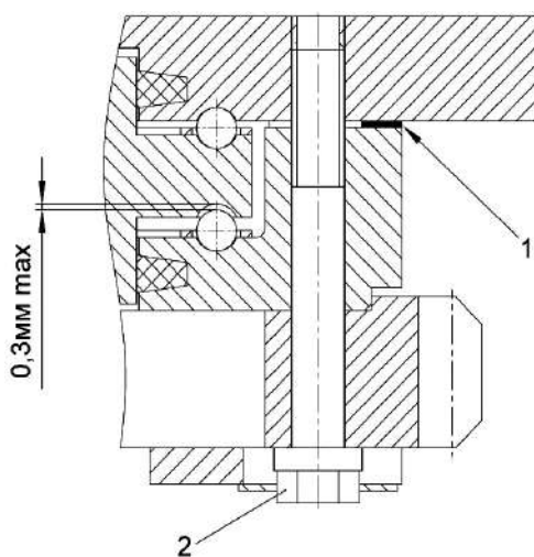
1 – прокладка; 2 – болт
