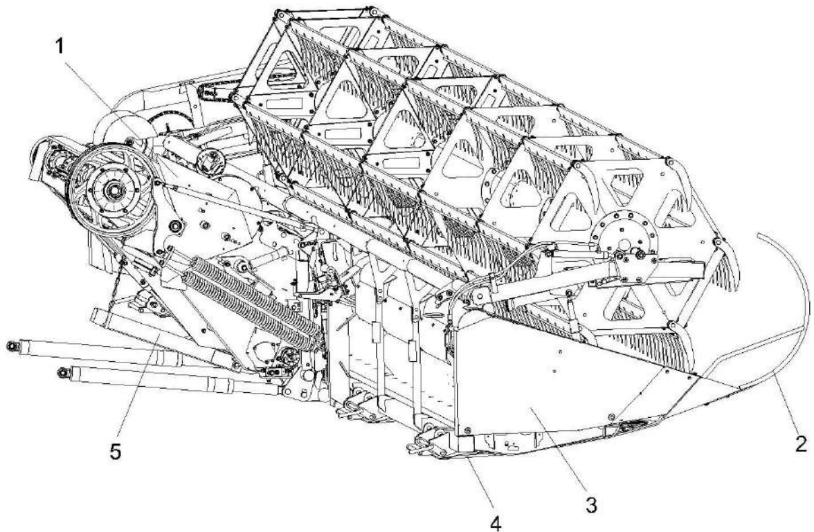
Рисунок 2.12 – Жатка, навешенная на наклонную камеру
