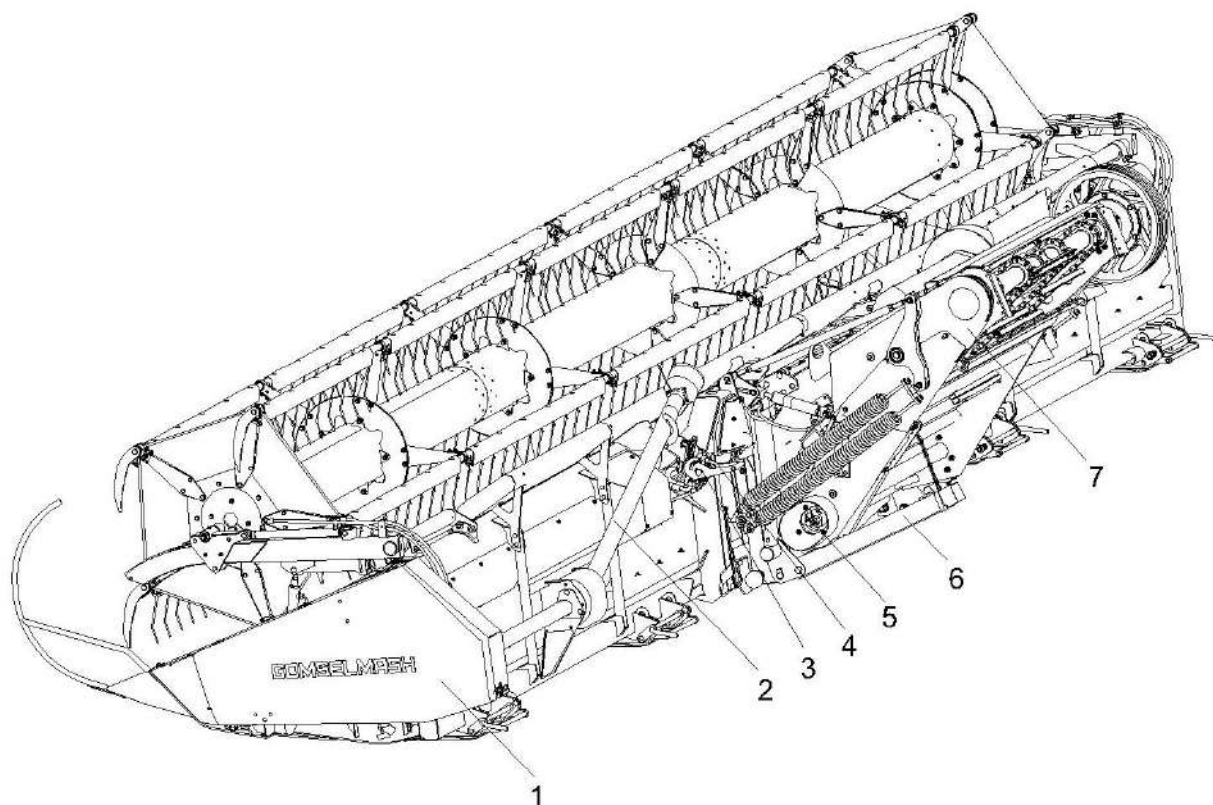
1 – жатка; 2 – вал карданный жатки; 3 – разъем многофункциональный; 4 – розетка; 5 – вал трансмиссионный наклонной камеры; 6 – упор; 7 – наклонная камера
