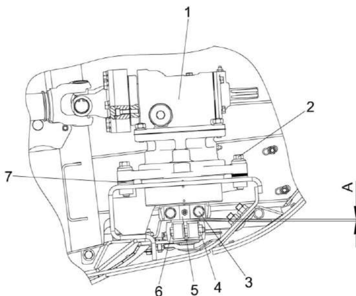
1 – редуктор; 2, 3, 6 – болты; 4 – гайка; 5 – водило; 7 – регулировочные прокладки
