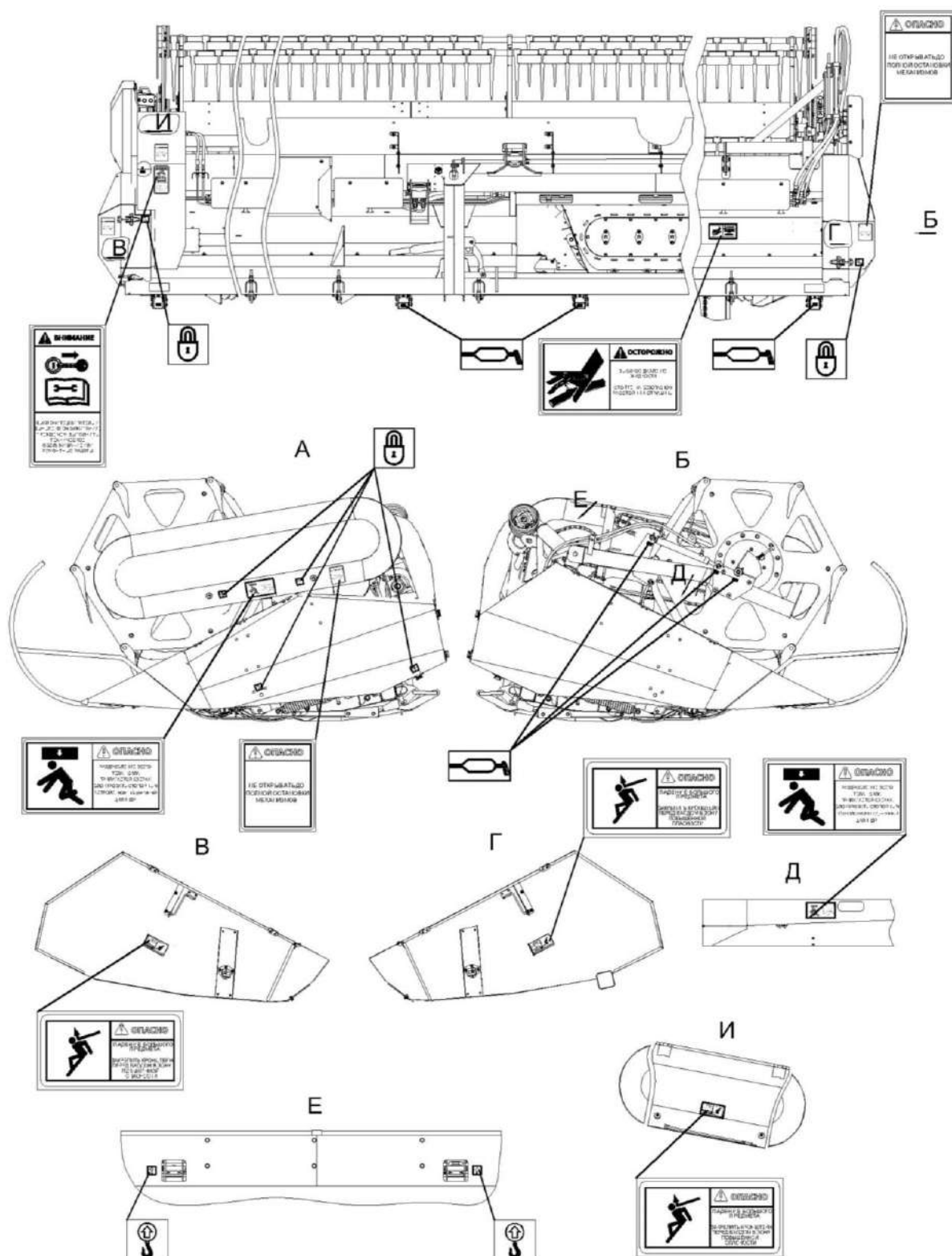
Расположение на жатке предупредительных и указательных знаков и табличек безопасности (для жаток III)
