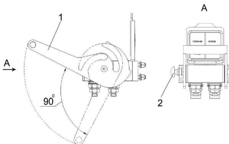
1 – рукоятка разъёма; 2 – фиксатор
