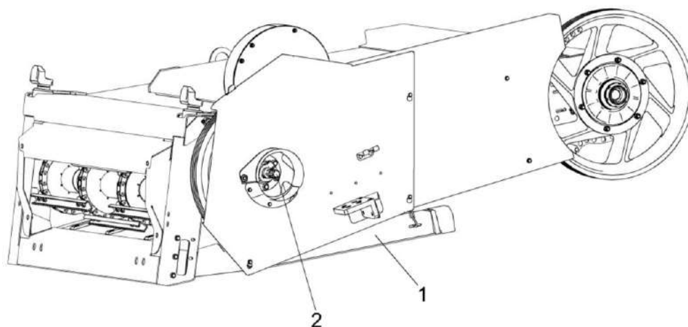
Рисунок 2.2 – Наклонная камера
