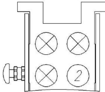
Схема подключения стационарной части разъема гидравлического многофункционального
