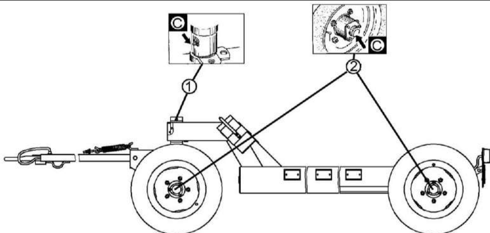
Рисунок 3.3 – Схема смазки транспортной тележки
