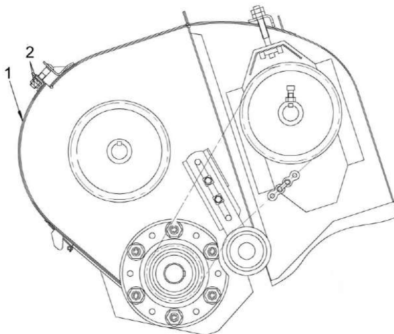
1 – крышка; 2 – гайки
