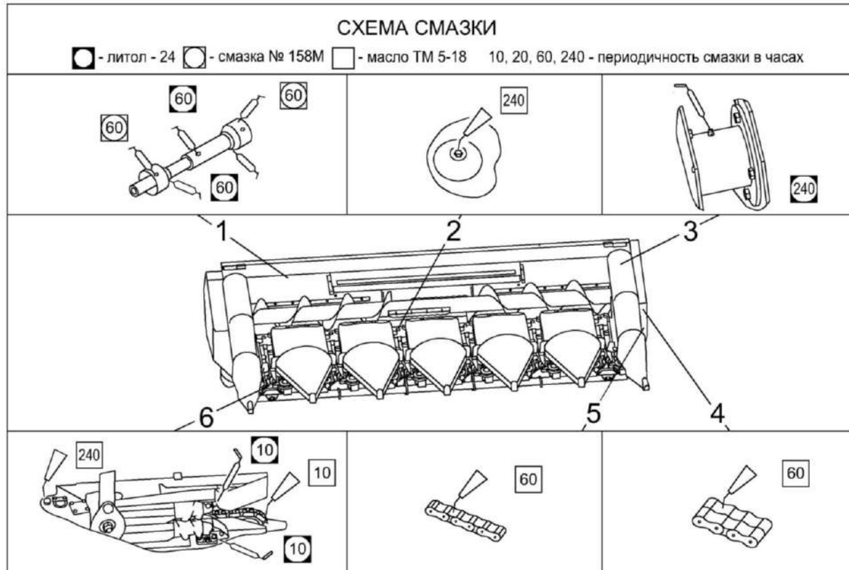
Рисунок 3.1 – Схема смазки жатки
