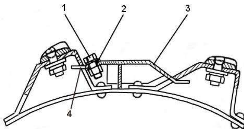
1 – болт М12х25 ( M_{кр}=90\ldots100Н\cdot м ); 2 – шайба; 3 – щиток перекрытия барабана; 4 – планка упорная
