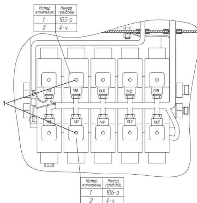
Рисунок 2.3 – Гидроблок
