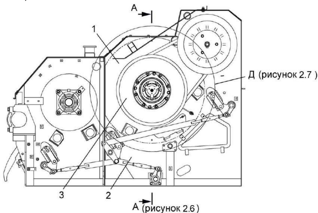
Рисунок 2.5 – Аппарат молотильный
