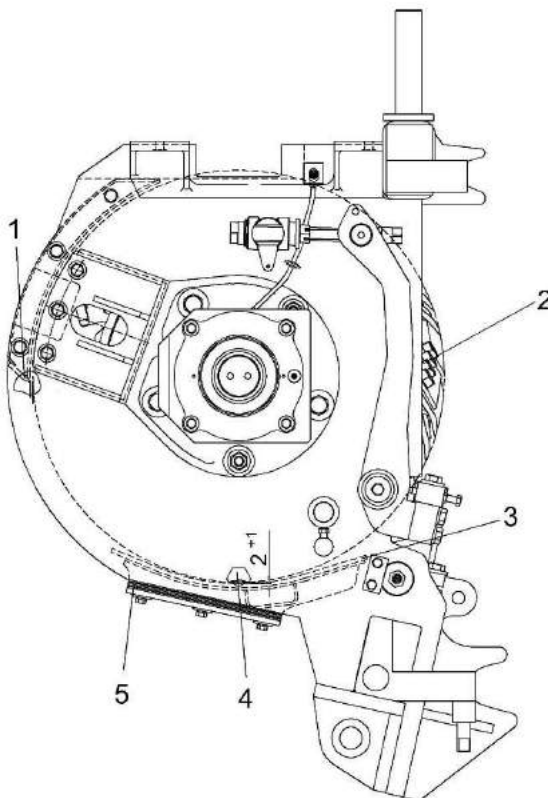
1 – отсекатель; 2 – ножи измельчающего барабана; 3 – поддон; 4 – пробка; 5– прокладки
