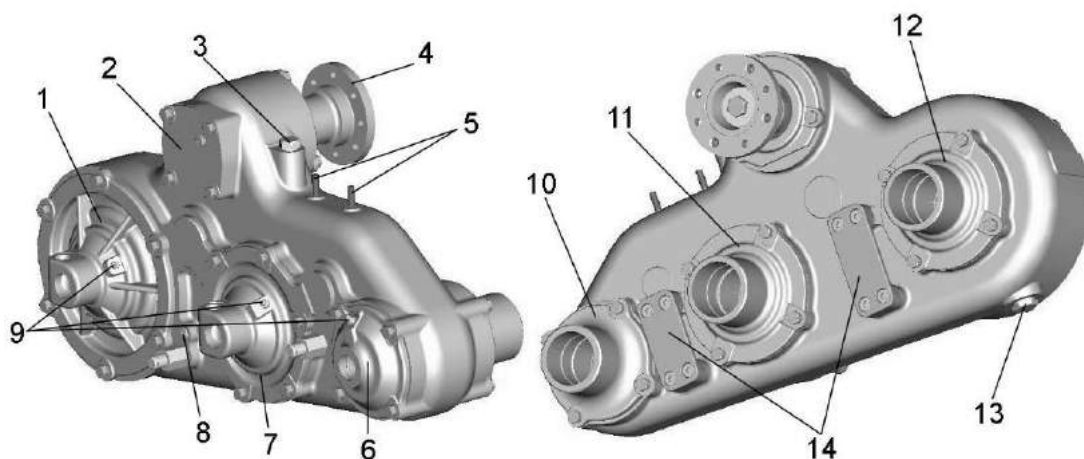
Рисунок 1.16 – Редуктор привода питающего аппарата
