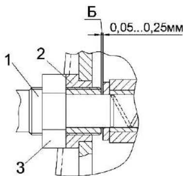
Рисунок 2.18 – Основание силосопровода
