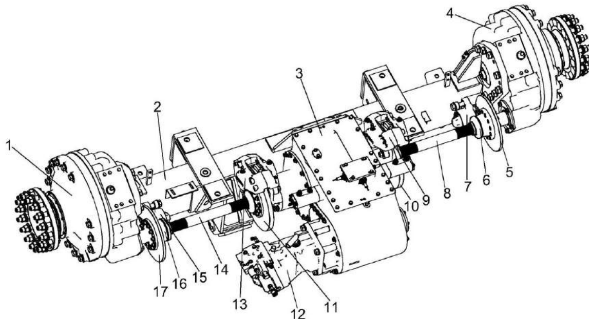
1, 4 – бортовые редуктора; 2 – балка моста; 3 – коробка передач; 5,10,11,17 – диски тормозные; 6, 16 – муфты соединительные; 7,9,13,15 – тормоза; 8,14 – полуоси; 12 - гидромотор
