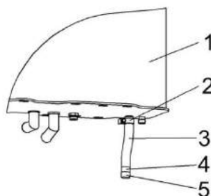
1 –бак масляный; 2,4 – хомуты; 3 – рукав; 5 – пробка
