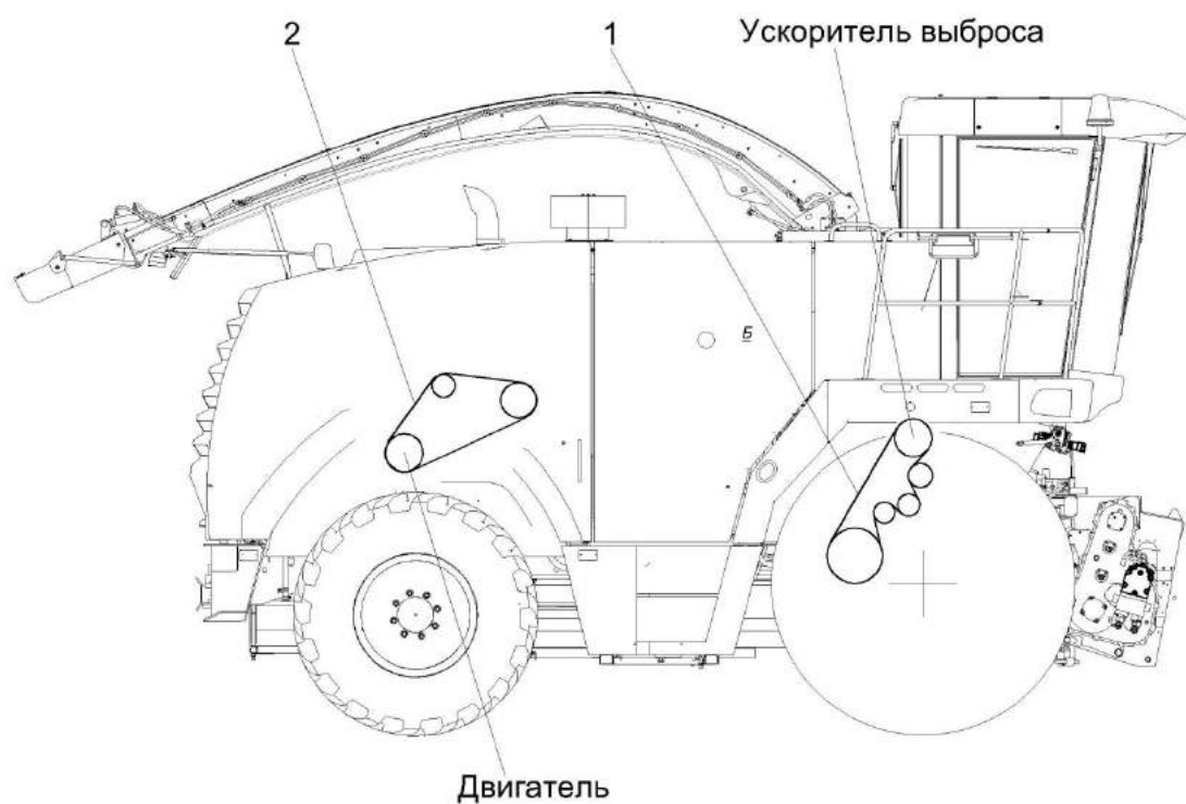
Рисунок Т.2 – Схема приводов измельчителя (вид справа)
