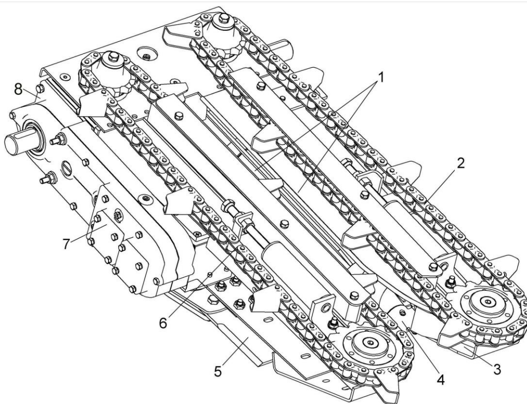
Рисунок 1.2 – Жатка
