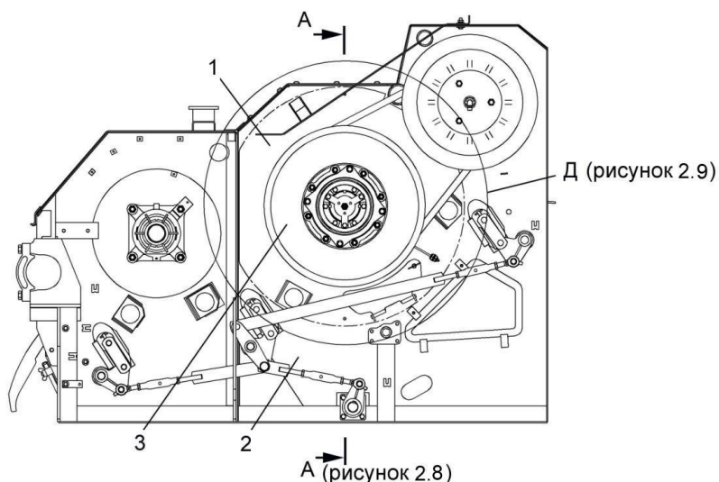
1 – фланец; 2 – аппарат молотильный; 3 – вариатор барабана
