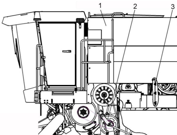
Рисунок 2.3 – Установка щитков перекрытия соломотряса
