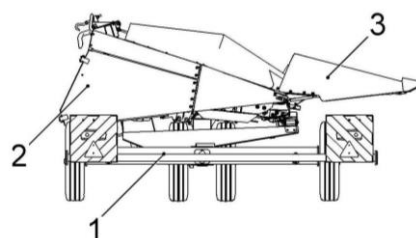
1 – тележка; 2 - жатка; 3 – делители
