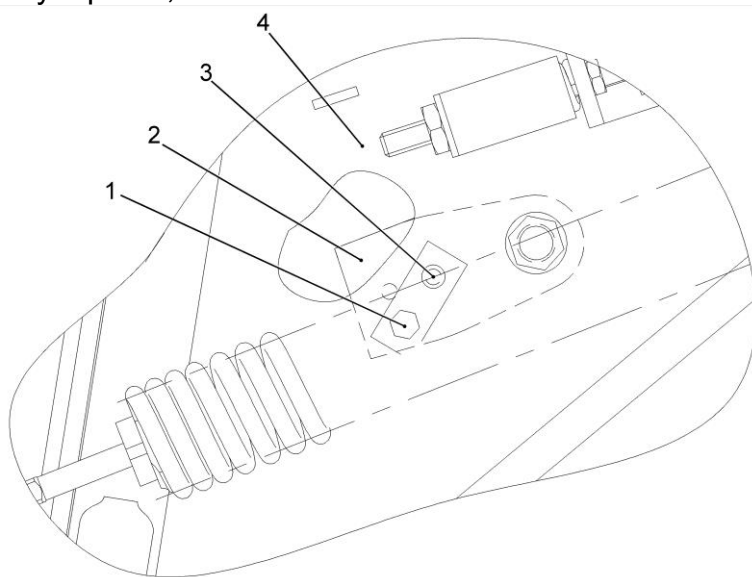
1 – болты; 2 – упоры; 3 – отверстие; 4 – наклонная камера
