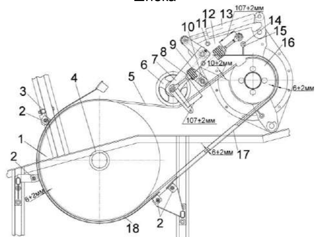
Рисунок 2.21 – Привод горизонтального шнека
