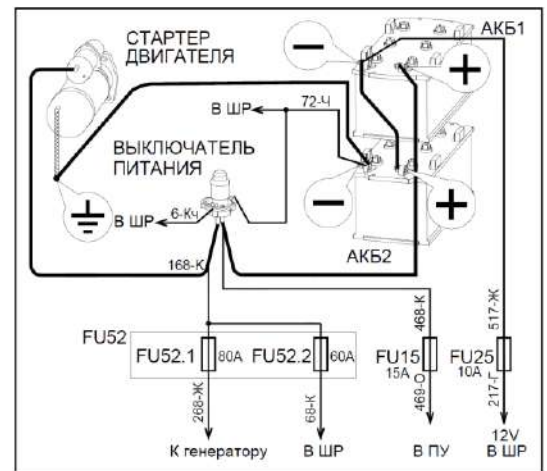
Рисунок 2.3 - Подключение аккумуляторных батарей
