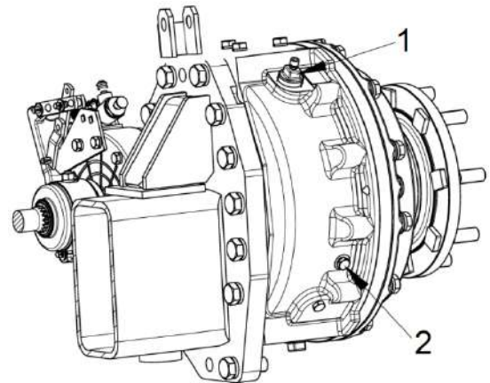
1 – отверстие для заправки; 2 – контрольное отверстие
