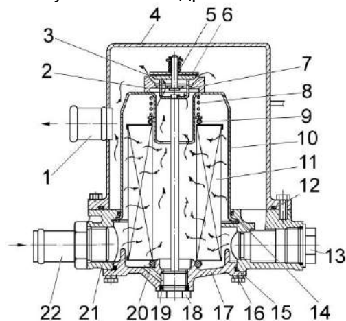
Рисунок 1.20 - Гидросистема
