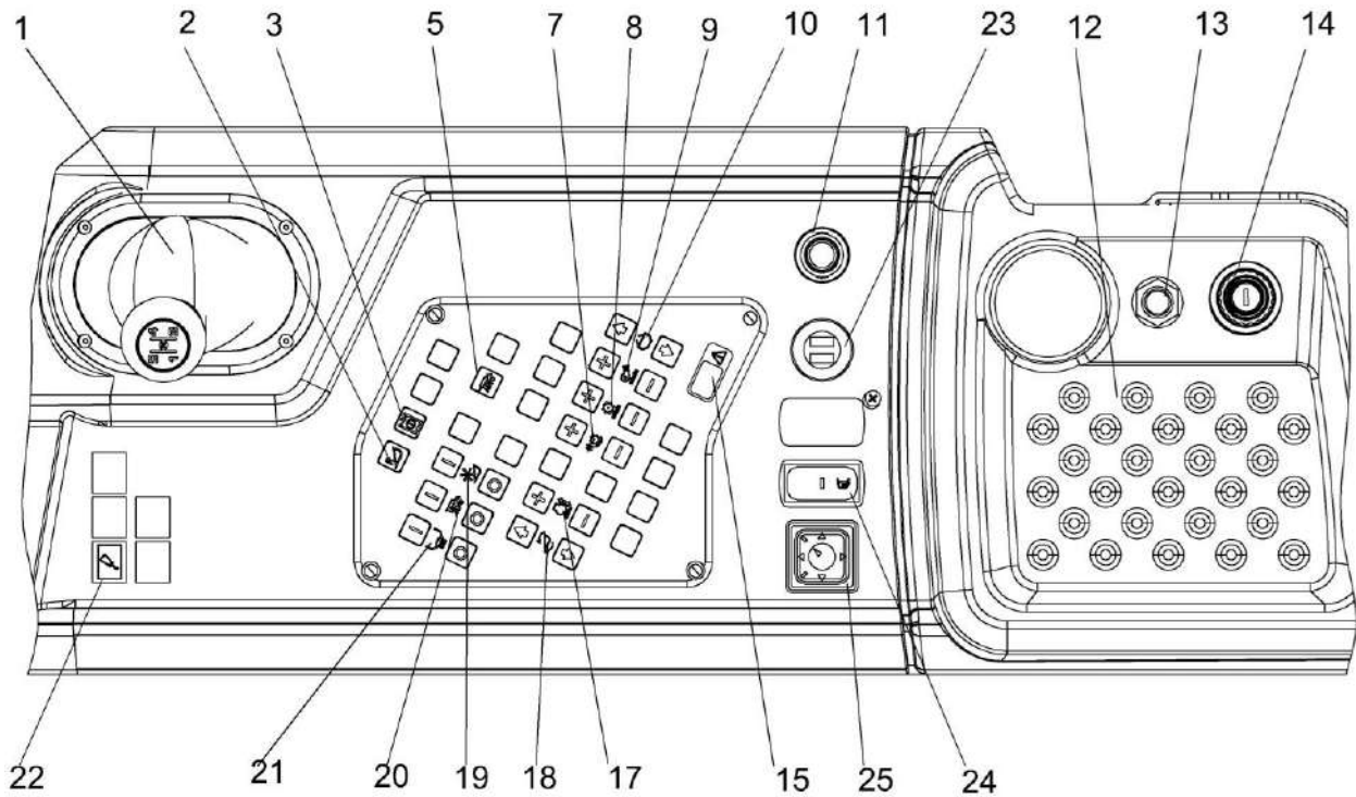
Рисунок 1.28 – Пульт управления комбайна
