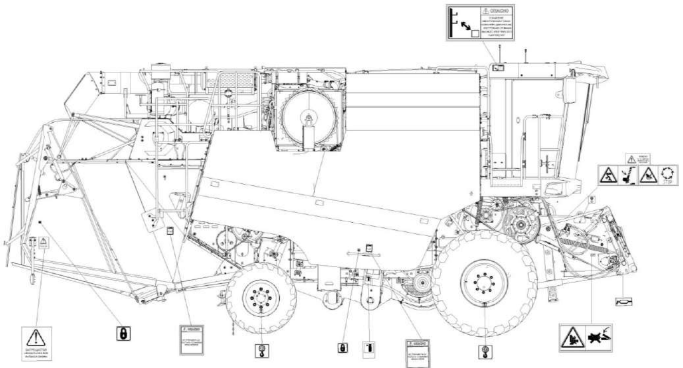
Комбайн (вид справа)
