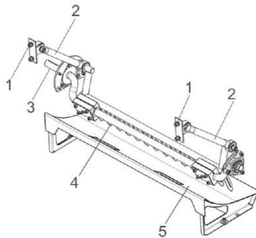
Рисунок 1.15 – Соломонабиватель
