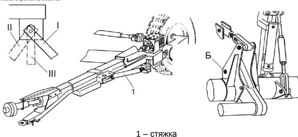
Схема положения сницы относительно рамы комбайна
