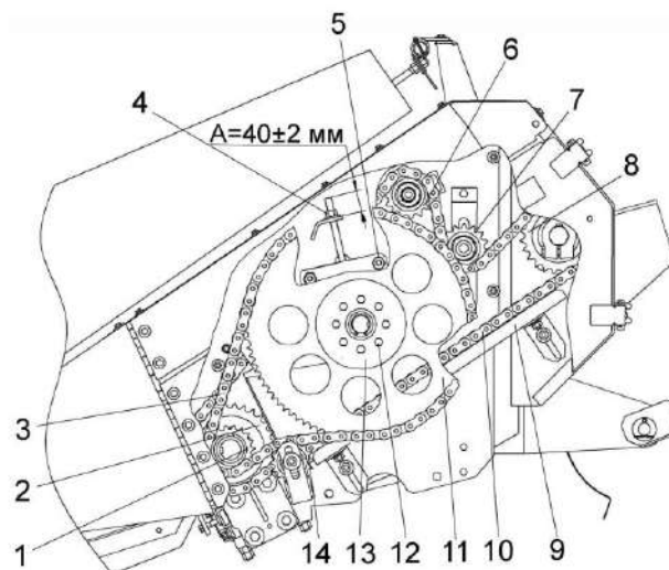
1, 2, 8, 11– звездочки приводные; 3, 10 – цепи; 4, 5 – гайки; 6, 7, 14 – звездочки натяжные; 9 – успокоитель; 12 – болт; 13 – муфта
