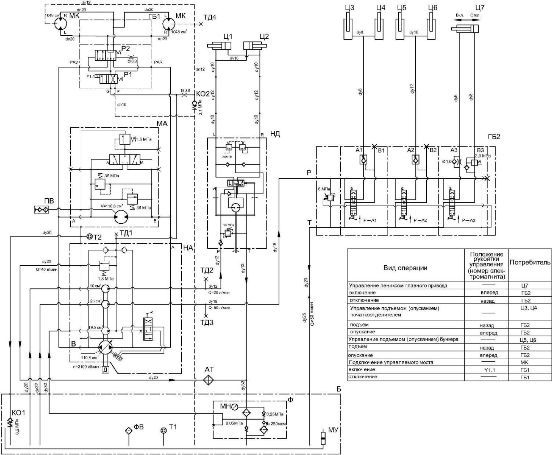
АТ – радиатор масляный; Б – бак масляный; ГБ1 – гидроблок подключения управляемого моста; ГБ2 – гидроблок управления рабочими органами; КО1 – гидроклапан обратный; КО2 – клапан дренажный; МА – гидромотор привода ходовой части; МК – гидромотор привода управляемого моста; МН – манометр; МУ – указатель уровня масла; НА – тандем насосов; НД – насос-дозатор; ПВ – полумуфта внутренняя; P1, P2 – гидрораспределители; Т1 – датчик аварийной температуры жидкости; Т2 – датчик указателя температуры жидкости; ТД1, ТД2, ТД3, ТД4 – соединение резьбовое с колпачком; Ф – фильтр; ФВ – фильтр воздушный гидравлический; Ц1, Ц2 – гидроцилиндры поворота управляемых колес; Ц3, Ц4 – гидроцилиндры подъема (опускания) початкоотделителя; Ц5, Ц6 – гидроцилиндры подъема (опускания) бункера; Ц7 – гидроцилиндр управления ленинсом главного привода
