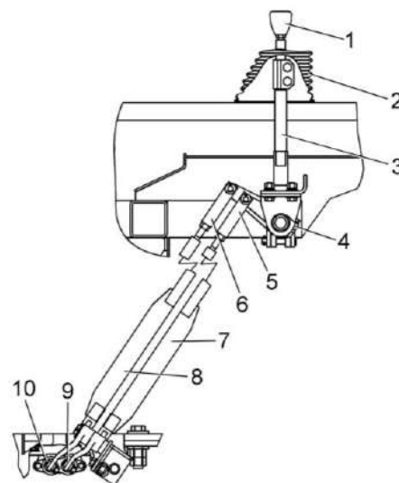
1 – рукоятка; 2 – чехол; 3 – рычаг; 4 – блок переключения; 5, 6 – вилки; 7, 8 – тяги; 9, 10 – штоки
