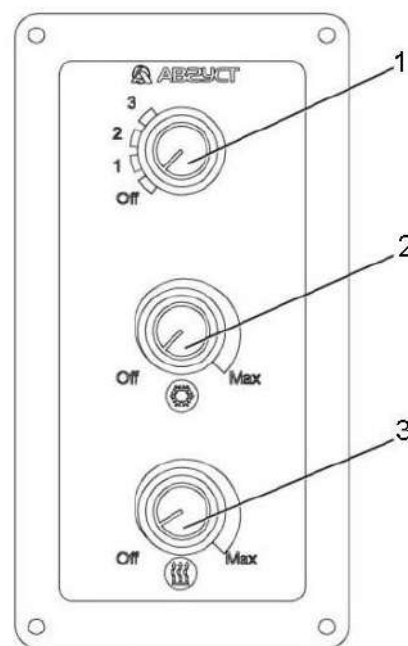
1 – ручка выключателя управления вентилятором; 2 – ручка выключателя управления термостатом кондиционера; 3 – ручка выключателя управления термостатом отопителя
