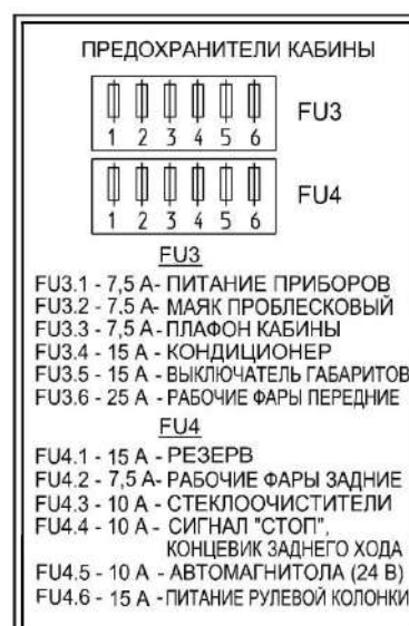
Рисунок 1.23 – Предохранители кабины
