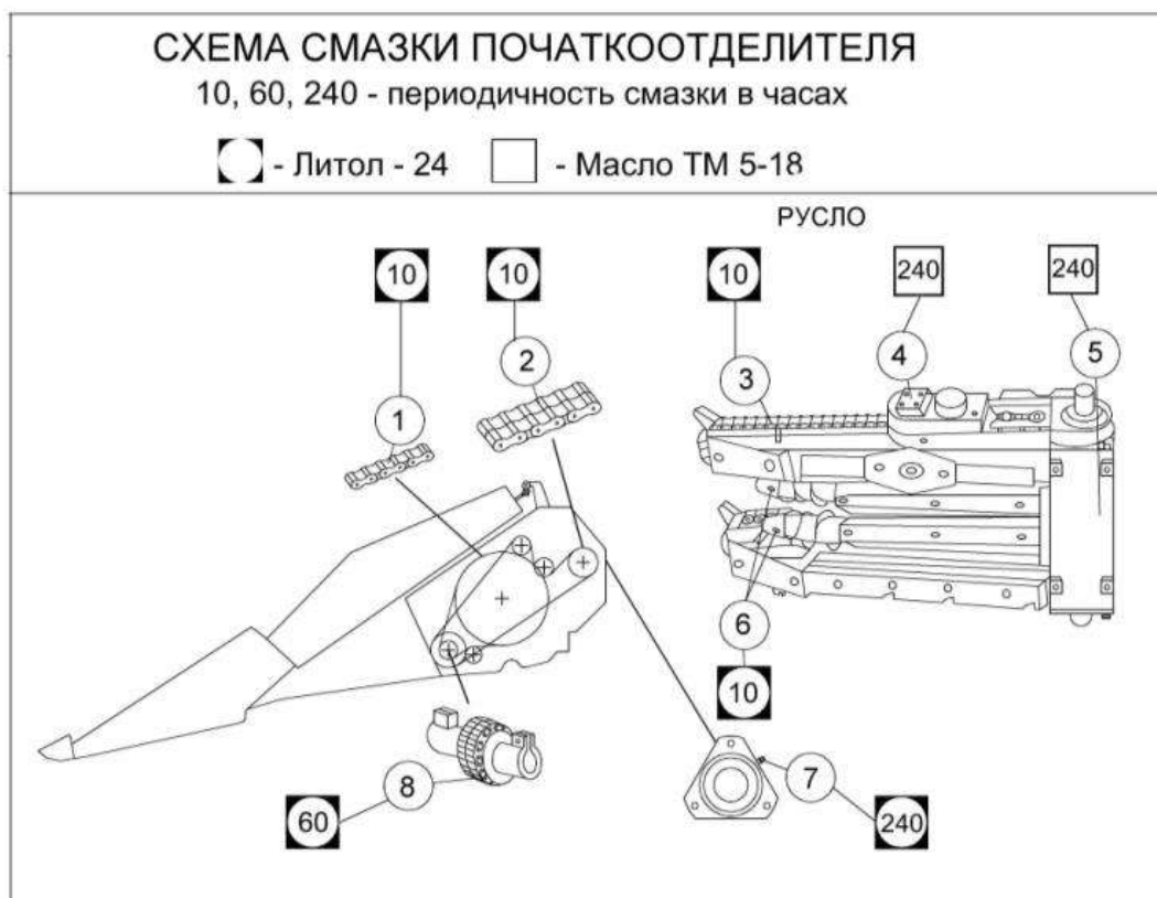
Рисунок 3.3 – Схема смазки початкоотделителя
