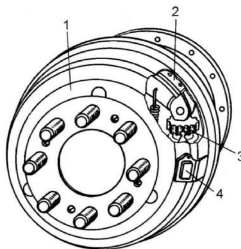
1 — барабан тормозной; 2 — колодка тормозная; 3 — колпачок; 4 — крышка
