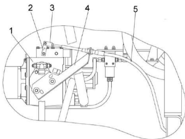
1 – гидронасос привода ходовой части; 2 – рычаг; 3 – вилка; 4 – кронштейн; 5 – трос
