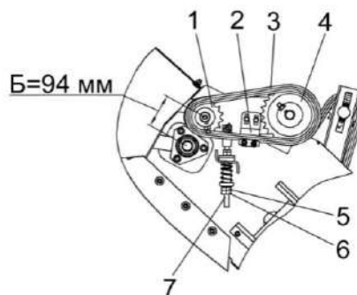
1, 4 – звездочки; 2 – успокоитель; 3 – цепь; 5, 6 – гайки; 7 – тяга
