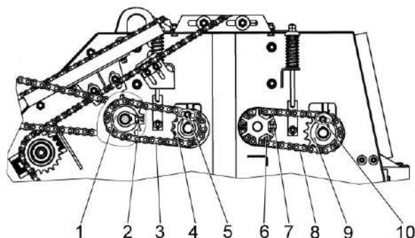
Рисунок 2.10 – Регулировки приводов устройства початкоочистительного, правая сторона
