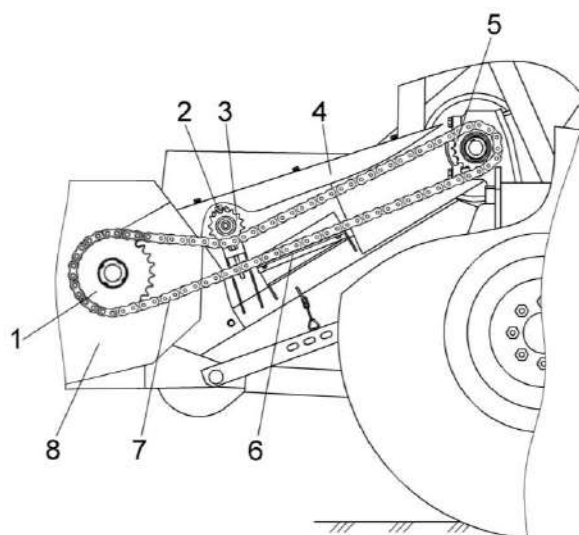
1, 5 – звездочки приводные; 2 – болт натяжной; 3 – звездочка натяжная; 4 – рама навески; 6 – успокоитель; 7 – цепь; 8 – початкоотделитель
