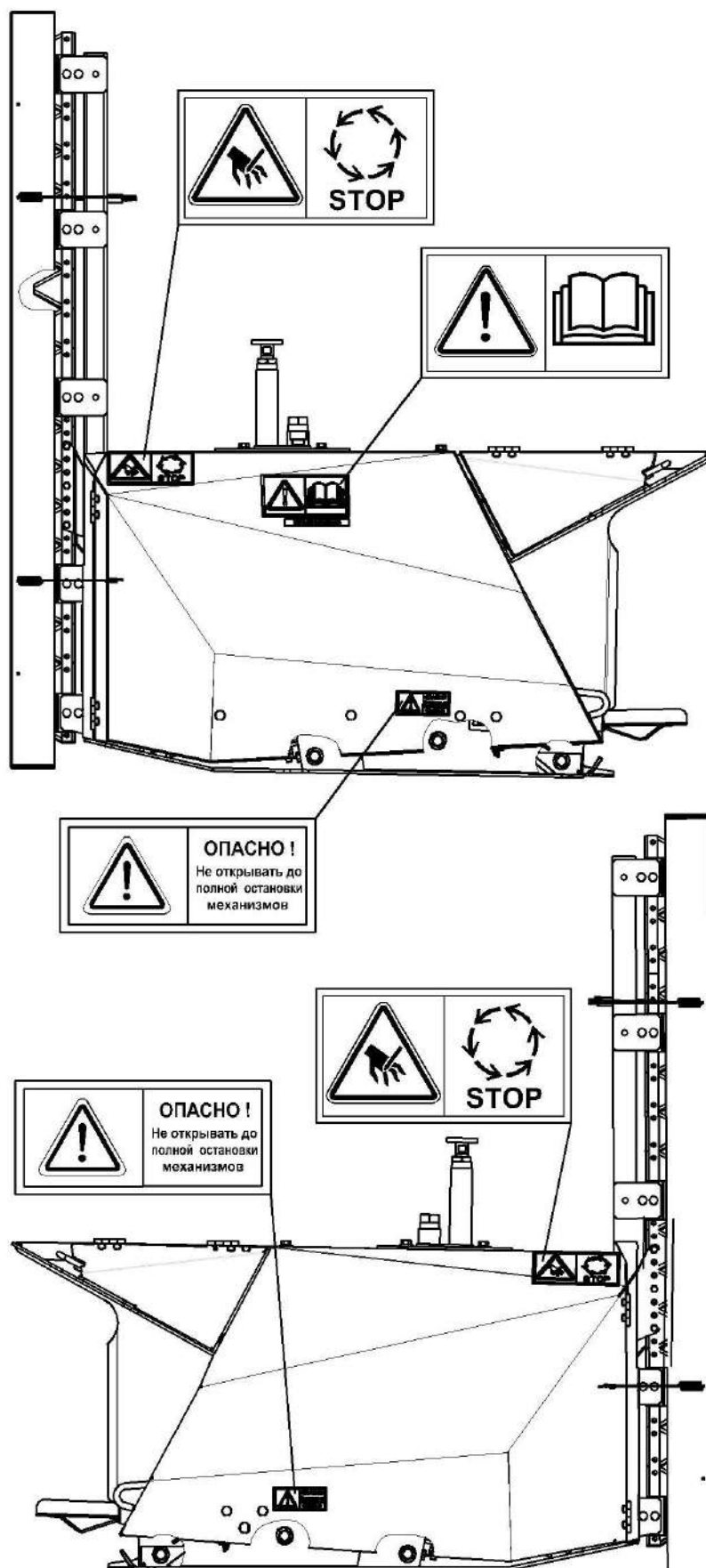
Расположение табличек на приспособлении
