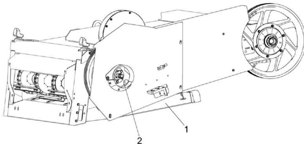
Рисунок 2.2 – Наклонная камера
