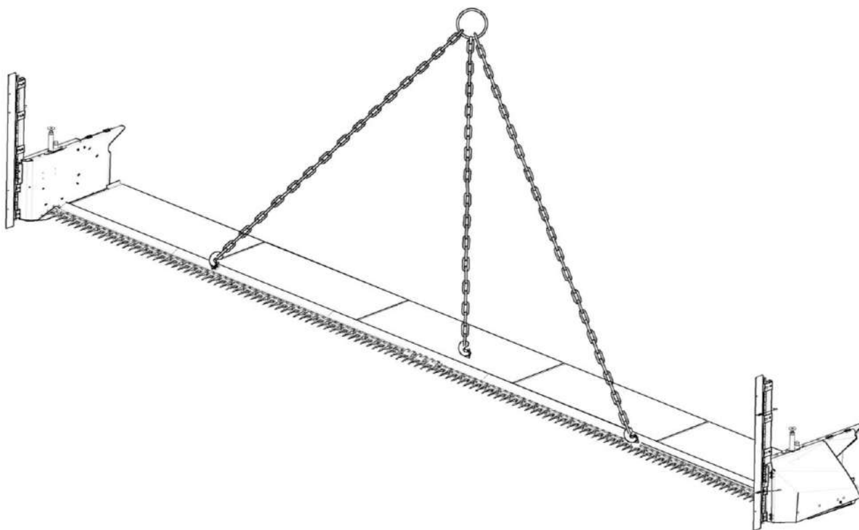
Рисунок 6.1 – Схема строповки
